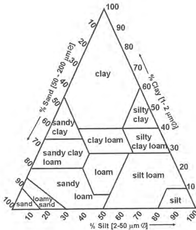
Ilustración VI-4: Triángulo de clasificación por contenido de arena (sand), limo (silt) y arcilla (clay), migajón (loam)
