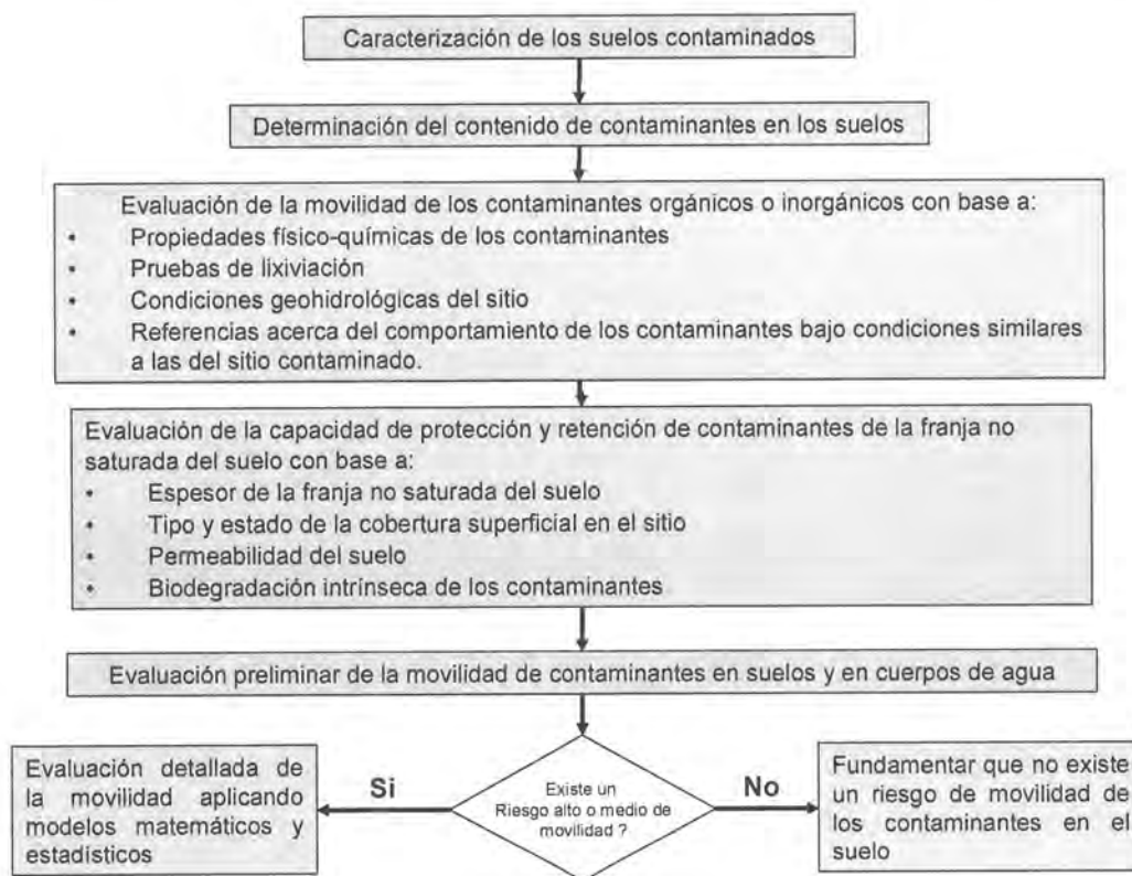
Ilustración VI-2: Estrategia para la evaluación de la movilidad de contaminantes en suelos.
