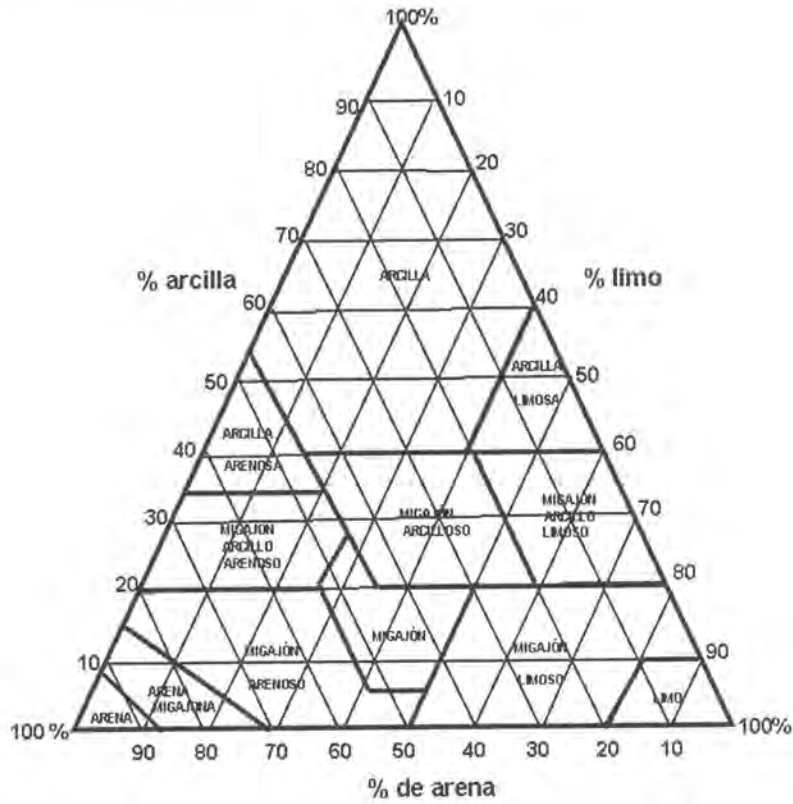
Triángulo de texturas (Soil Survey Manual, 1975)
