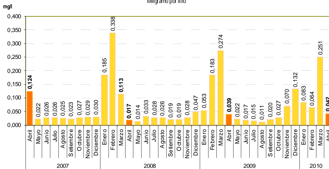
Gráfico N° 10 Lima Metropolitana: Concentración promedio de plomo (Pb) en el río Rímac, 2007-2010 Miligramo por litro
