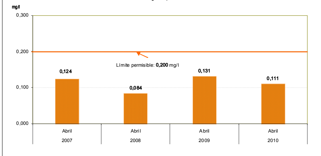
Gráfico N° 19 Lima Metropolitana: Concentración máxima de aluminio (Al) en las plantas de tratamiento 1 y 2 de SEDAPAL, 2007-2010 Miligramo por litro
