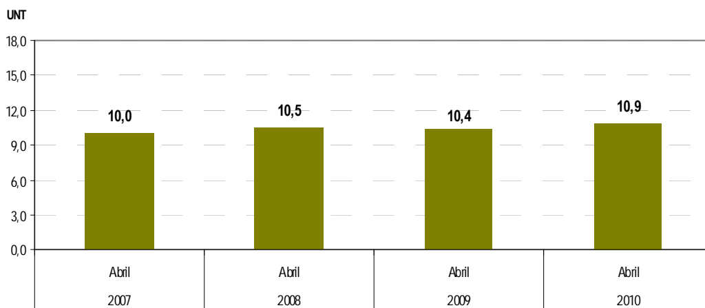
Gráfico: N° 31 Lima Metropolitana: Nivel máximo de turbiedad en el río Rímac, 2007-2010
