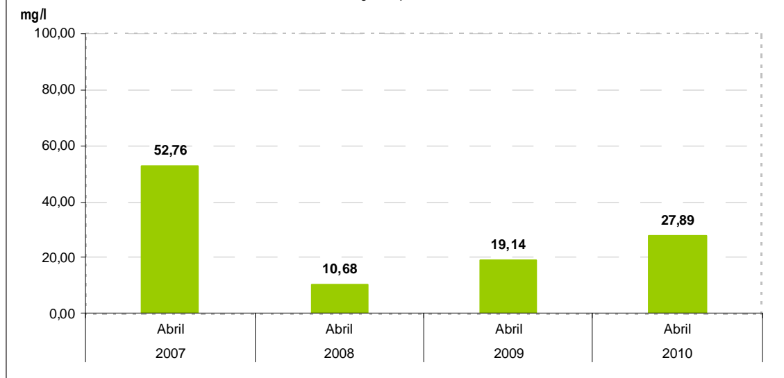
Gráfico N° 5 Lima Metropolitana: Concentración máxima de hierro total (Fe) en el río Rímac, 2007-2010 Miligramo por litro
