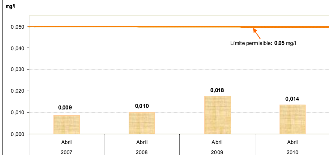
Gráfico N° 11 Lima Metropolitana: Concentración máxima de plomo (Pb) en las plantas de tratamiento 1 y 2 de SEDAPAL, 2007-2010 Miligramo por litro
