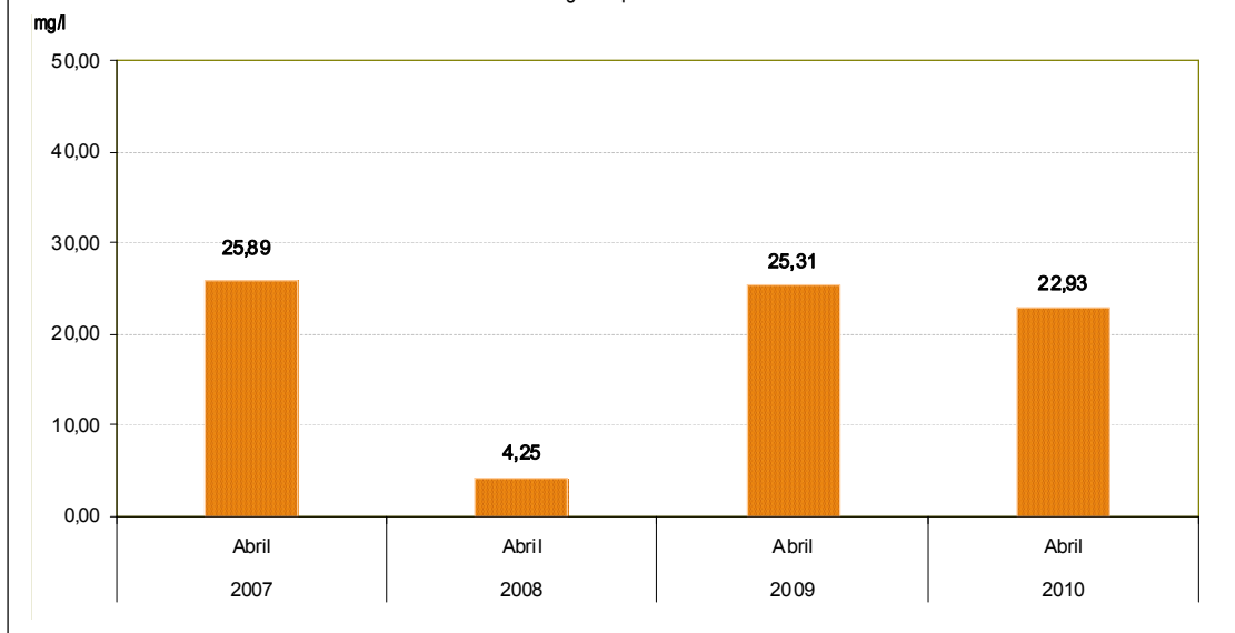
Gráfico N° 17 Lima Metropolitana: Concentración máxima de aluminio (Al) en el río Rímac, 2007-2010 Miligramo por litro
