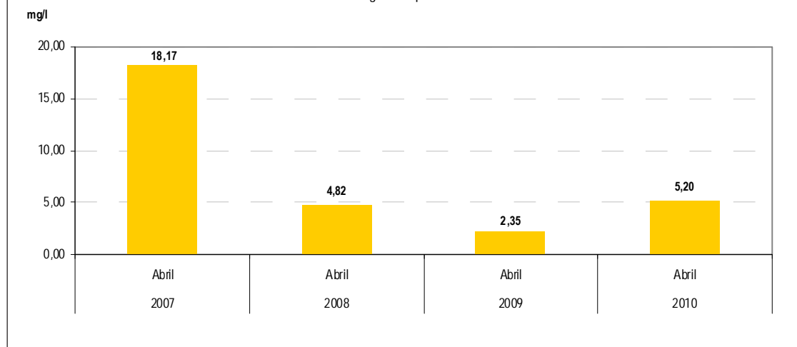
Gráfico N° 21 Lima Metropolitana: Concentración máxima de materia orgánica en el río Rímac, 2007-2010 Miligramos por litro
