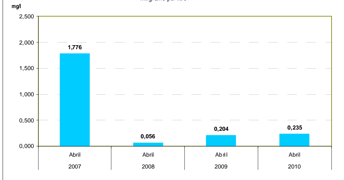
Gráfico N° 9 Lima Metropolitana: Concentración máxima de plomo (Pb) en el río Rímac, 2007-2010 Miligramo por litro
