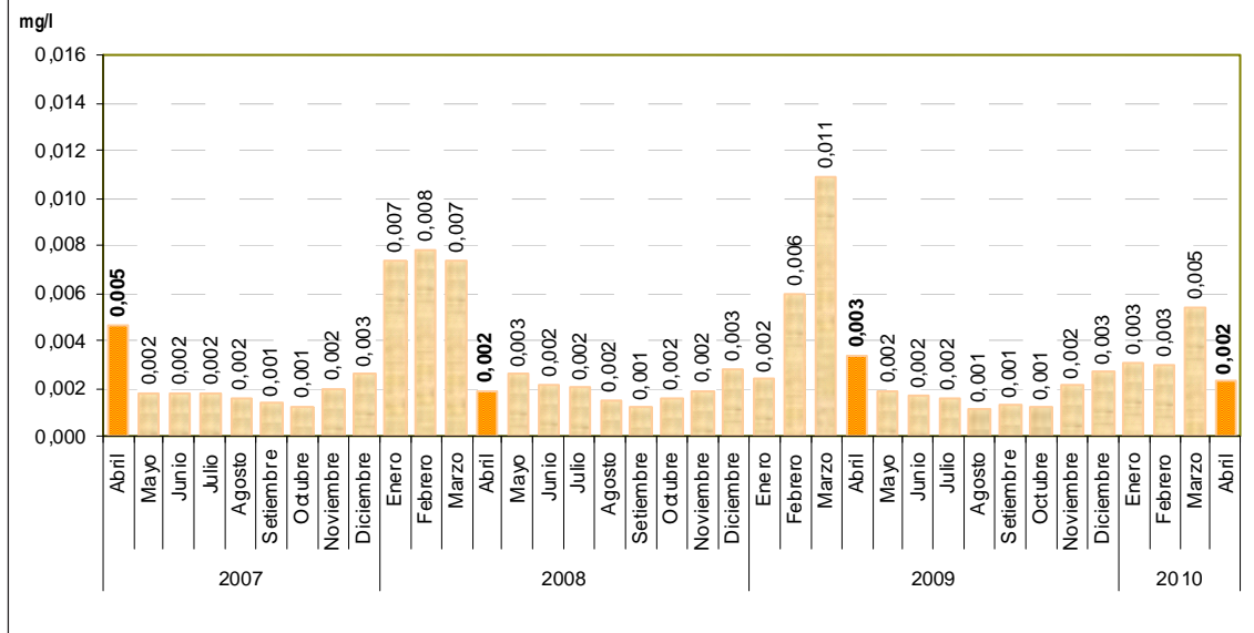
Gráfico N° 14 Lima Metropolitana: Concentración promedio de cadmio (Cd) en el río Rímac, 2007-2010 Miligramo por litro
