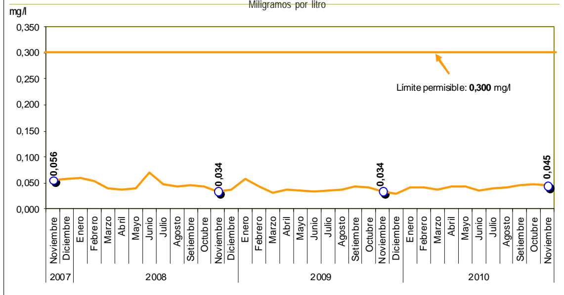
Gráfico N° 8 Lima Metropolitana: Concentración promedio de hierro total (Fe) en las plantas de tratamiento 1 y 2 de SEDAPAL, 2007-2010 Miligramos por litro
