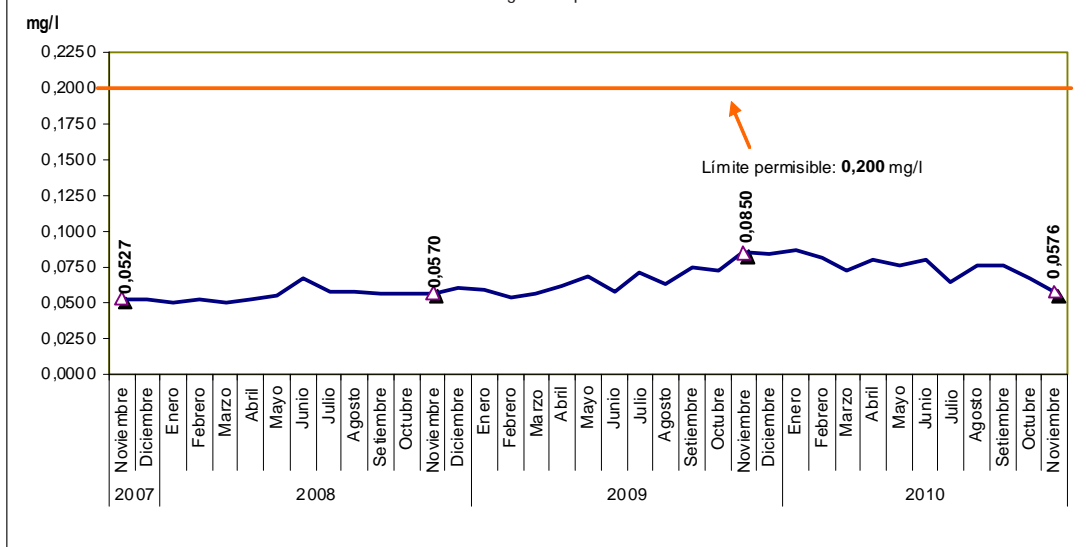
Gráfico N° 20 Lima Metropolitana: Concentración promedio de aluminio (Al) en las plantas de tratamiento 1 y 2 de SEDAPAL, 2007-2010 Miligramos por litro
