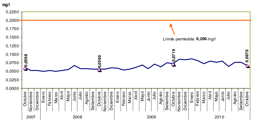
Gráfico N° 20 Lima Metropolitana: Concentración promedio de aluminio (Al) en las plantas de tratamiento 1 y 2 de SEDAPAL, 2007-2010 Miligramos por litro
