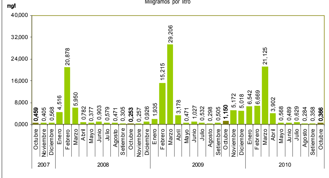
Gráfico N° 18 Lima Metropolitana: Concentración promedio de aluminio (Al) en el río Rímac, 2007-2010 Miligramos por litro
