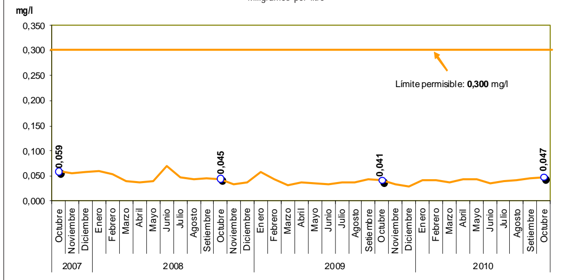
Gráfico N° 8 Lima Metropolitana: Concentración promedio de hierro total (Fe) en las plantas de tratamiento 1 y 2 de SEDAPAL, 2007-2010 Miligramos por litro
