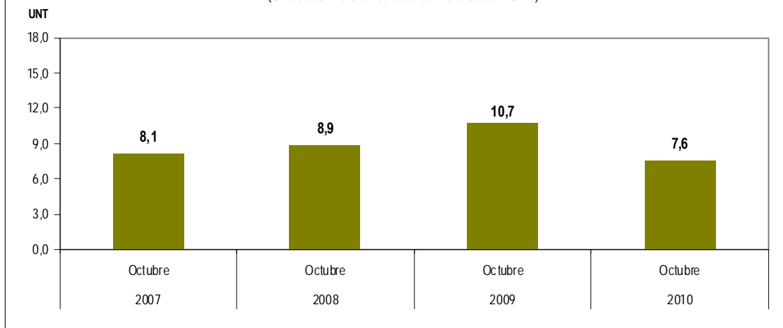
Gráfico N° 31 Lima Metropolitana: Nivel mínimo de turbiedad en el río Rímac, 2007-2010 (Unidades Nefelométricas de Turbiedad - UNT)
