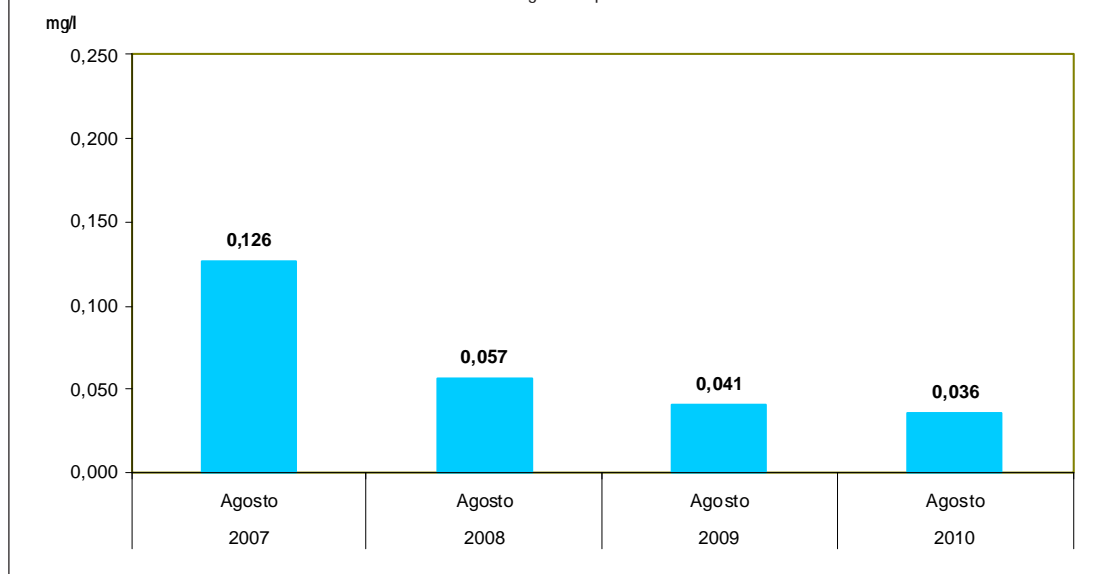
Gráfico N° 9 Lima Metropolitana: Concentración máxima de plomo (Pb) en el río Rímac, 2007-2010 Miligramos por litro
