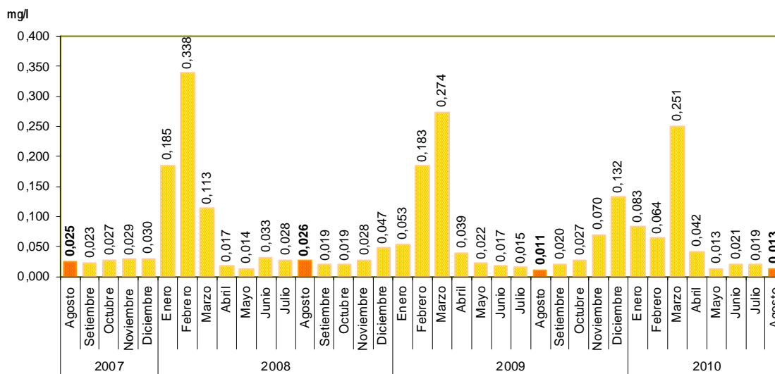
Gráfico N° 10 Lima Metropolitana: Concentración promedio de plomo (Pb) en el río Rímac, 2007-2010 Miligramos por litro
