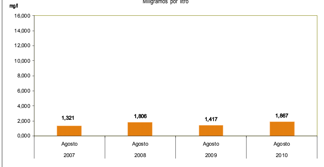
Gráfico N° 17 Lima Metropolitana: Concentración máxima de aluminio (Al) en el río Rímac, 2007-2010 Miligramos por litro
