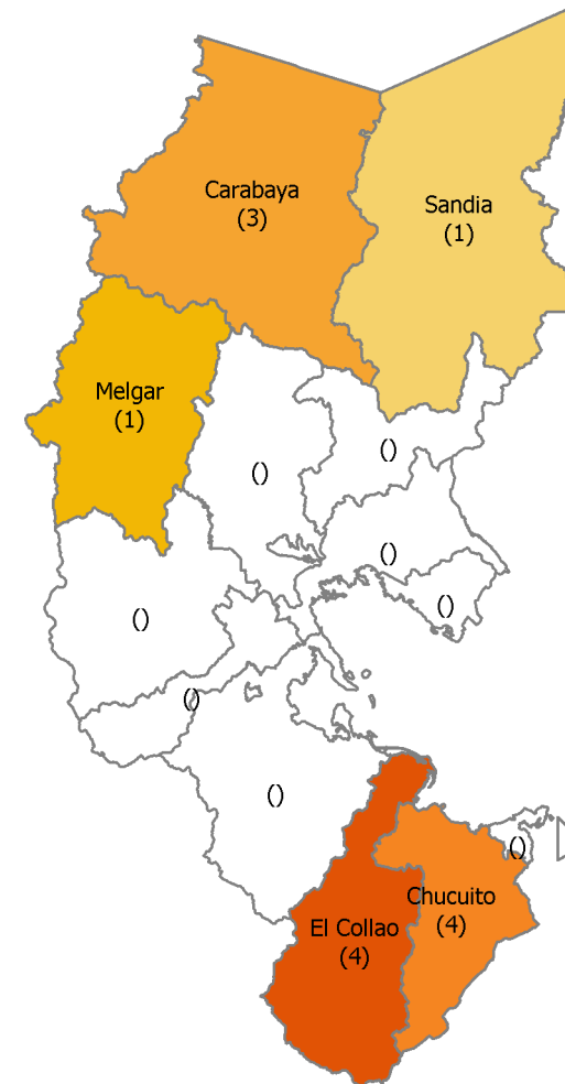
MAPA DE DENSIDAD DE FOCOS DE CALOR POR PROVINCIA Total : 13
