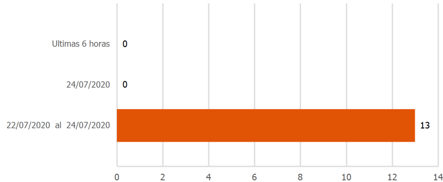
FOCOS DE CALOR Total : 13
