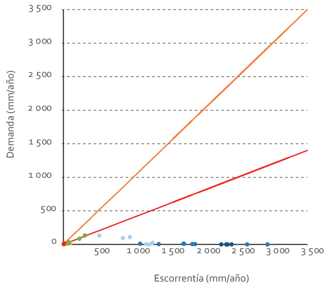
Gráfico 7 Relación entre escorrentía y demanda para todas las cuencas analizadas (mm/año)
