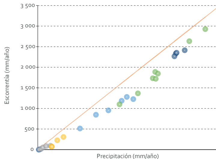
Gráfico 6 Relación entre precipitación y escorrentía para todas las cuencas analizadas
