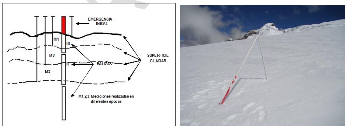
Figura 90. Izquierda: Estructura y emplazamiento de una baliza. Fuente: (Francou & Pouyaud, 2004); Derecha: Baliza Ritacuba Blanco 3, Nevado del Cocuy. Fuente: Fotos de campañas de monitoreo de glaciares colombianos, IDEAM, 2008.
