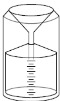
Figura 44. Pluviómetro convencional utilizado para muestreo a base de eventos o con transferencia diaria). A la izquierda esquema del pluviómetro (OIEA/GNIP, 2014), a la
