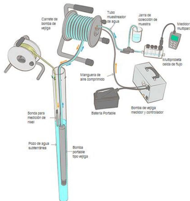
Figura 186. Ejemplo de un muestreo portátil. Fuente: (Geotech Environmental Equipment, 2015)
