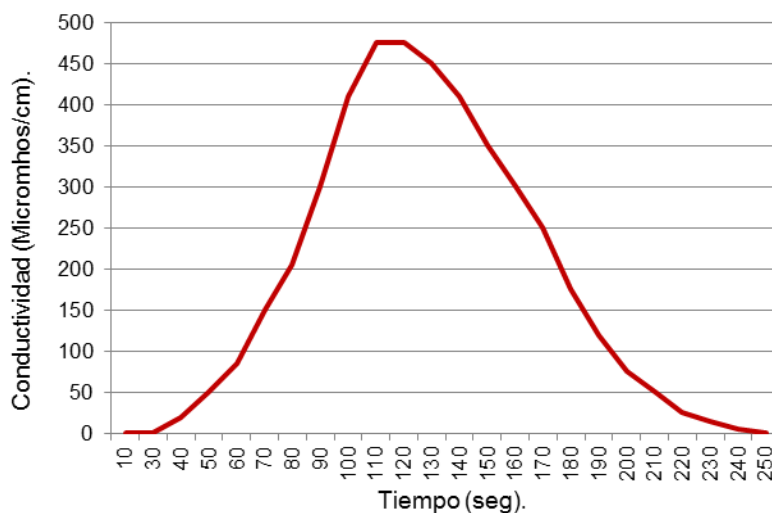
Figura 79. Conductividad según inyección constante. Fuente (IDEAM, 2006).
