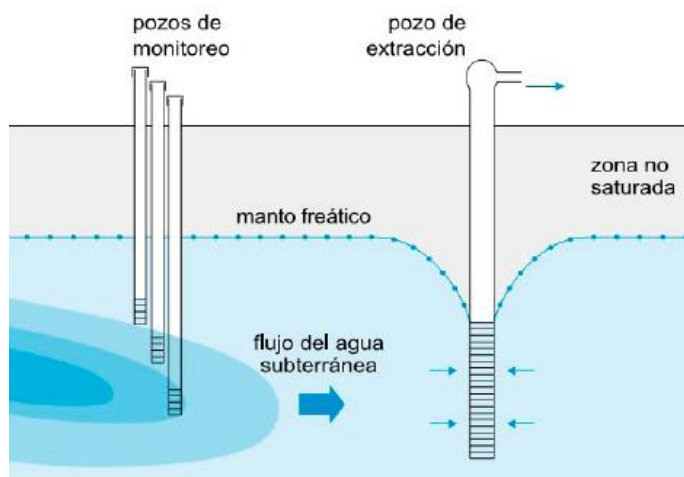
Figura 167. Ubicación de pozos de monitoreo para fuentes de abastecimiento de agua subterránea. Fuente: (Foster S. , Hirata, Gomes, D'Elia, & Paris, 2002).
