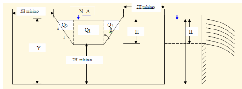
Figura 82. Vertedero trapecial. (IDEAM, 2006)
