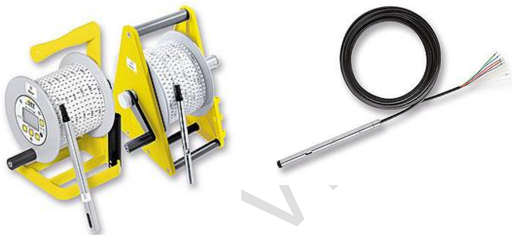
Figura 57. Izquierda: Sonda luminosa cuya operación es de manivela. Derecha: Sonda con sensor de presión. (OTT Hydromet, 2017)
