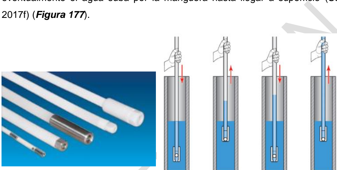
Figura 177. Izquierda: Bomba inercial, Derecha: Mecanismo de operación de la bomba inercial.
