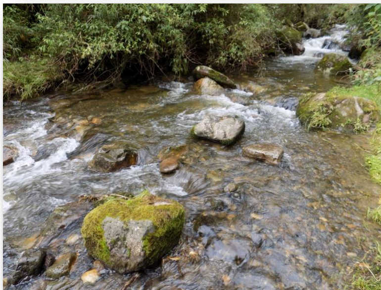
Figura 134. Quebrada Calostros. Se observan las características que se buscan para el muestreo de diatomeas en una corriente vadeable: buena iluminación, zona corriente del río, sustratos abundantes. Fotos por: Luisa Lagos, 2015
