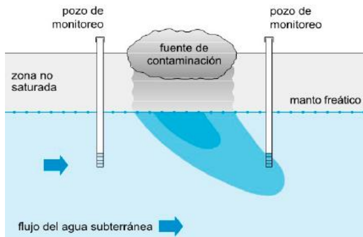
Figura 168. Ubicación de pozos de monitoreo para fuentes de contaminación puntuales. Fuente: (Foster S. , Hirata, Gomes, D'Elia, & Paris, 2002).
