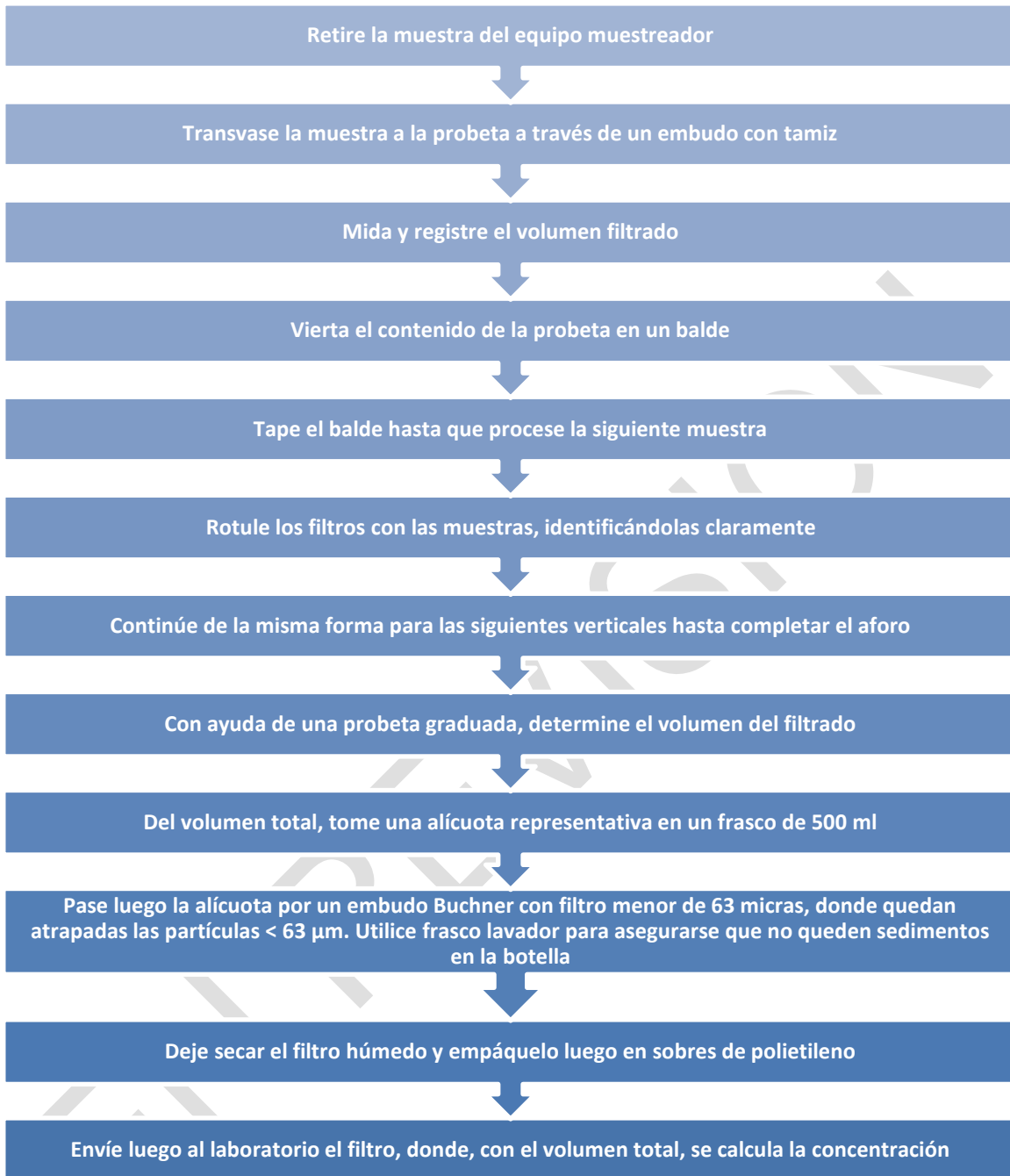
Figura 113. Procedimiento para procesamiento de muestra de bolsa plegable en el sitio
