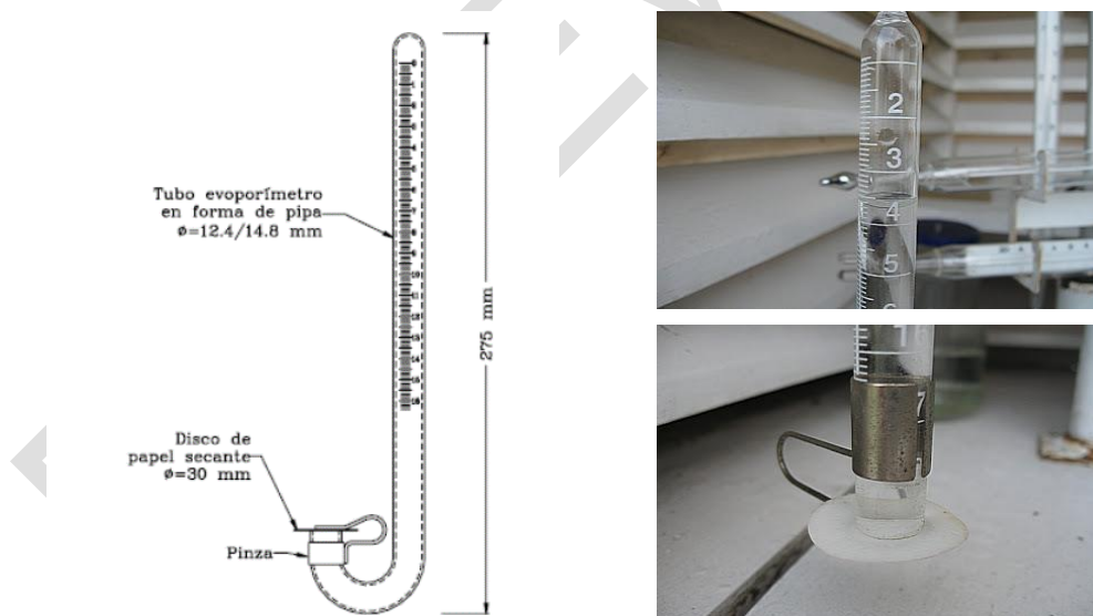
Figura 39. Izquierda: Detalle del evaporímetro Piché. Fuente: (Ruiz Romera & Martínez Santos, 2015). Derecha: Evaporímetro tipo Piche, donde se observa el disco poroso de papel sujeto al evaporímetro mediante una arandela metálica. Fuente: (Pelayo Arce, 2011)
