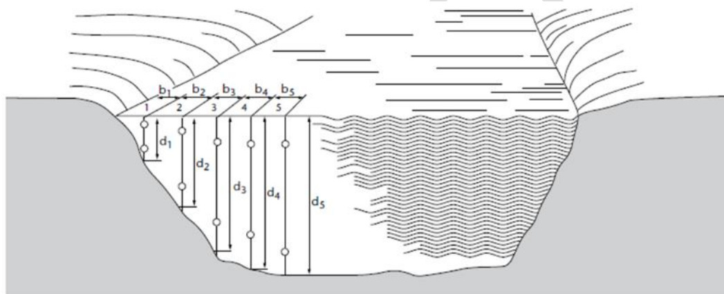
Figura 62. Vista de una sección transversal de una corriente, en la que figura la posición de los puntos de observación. (OMM, 2011)
