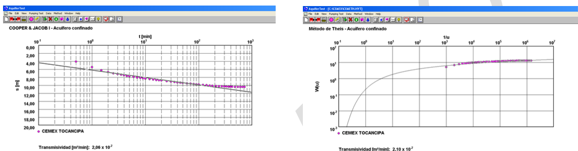
Figura 166. Interpretaciones de prueba de bombeo a caudal constante utilizando el programa Aquifer test , izquierda: método de Cooper & Jacob, derecha: método Theis.
