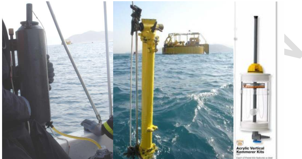
Figura 192. Botellas oceanográficas, Niskin (a) y Nansen (b) Kemmerer (c) usadas para la extracción de muestras de agua, operadas desde una embarcación menor.
