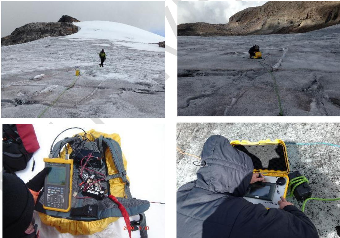
Figura 94. Transmisor utilizado para determinar el espesor del hielo, este envía una señal la cual será reciba por un receptor. Fotos de campañas de monitoreo de glaciares colombianos, IDEAM, 2014.
