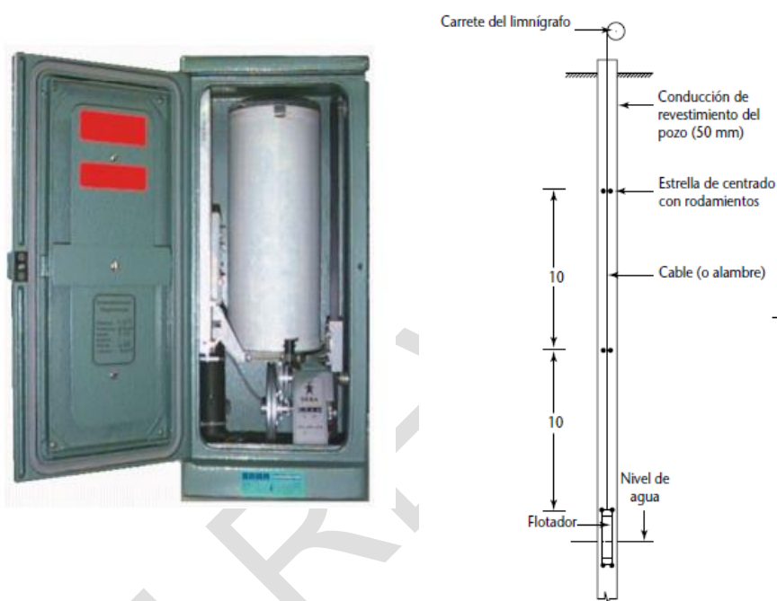
Figura 156. Izquierda: Limnógrafo vertical Fuente: (Ramas Ayala, 2003). Derecha: Mecanismo de funcionamiento para un limnógrafo. Fuente: (OMM, Guía de prácticas hidrológicas, 2011).
