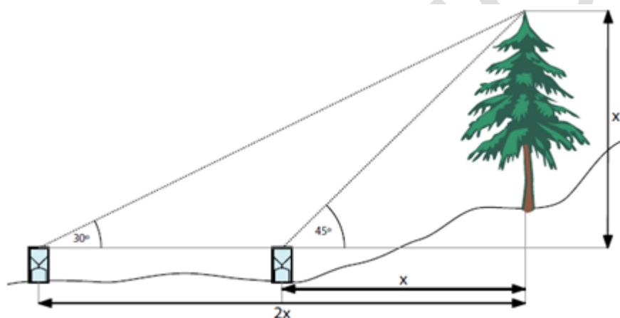
Figura 43. Ubicación del colector minimizando la influencia de estructuras cercanas.
