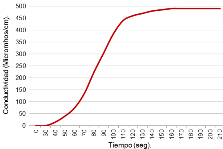
Figura 78. Conductividad según inyección constante. Fuente (IDEAM, 2006).
