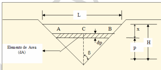
Figura 83. Vertedero Triangular. (IDEAM, 2006)
