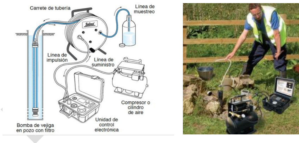
Figura 176. Funcionamiento de la bomba vejiga Fuente: (Solinst, 2017b)
