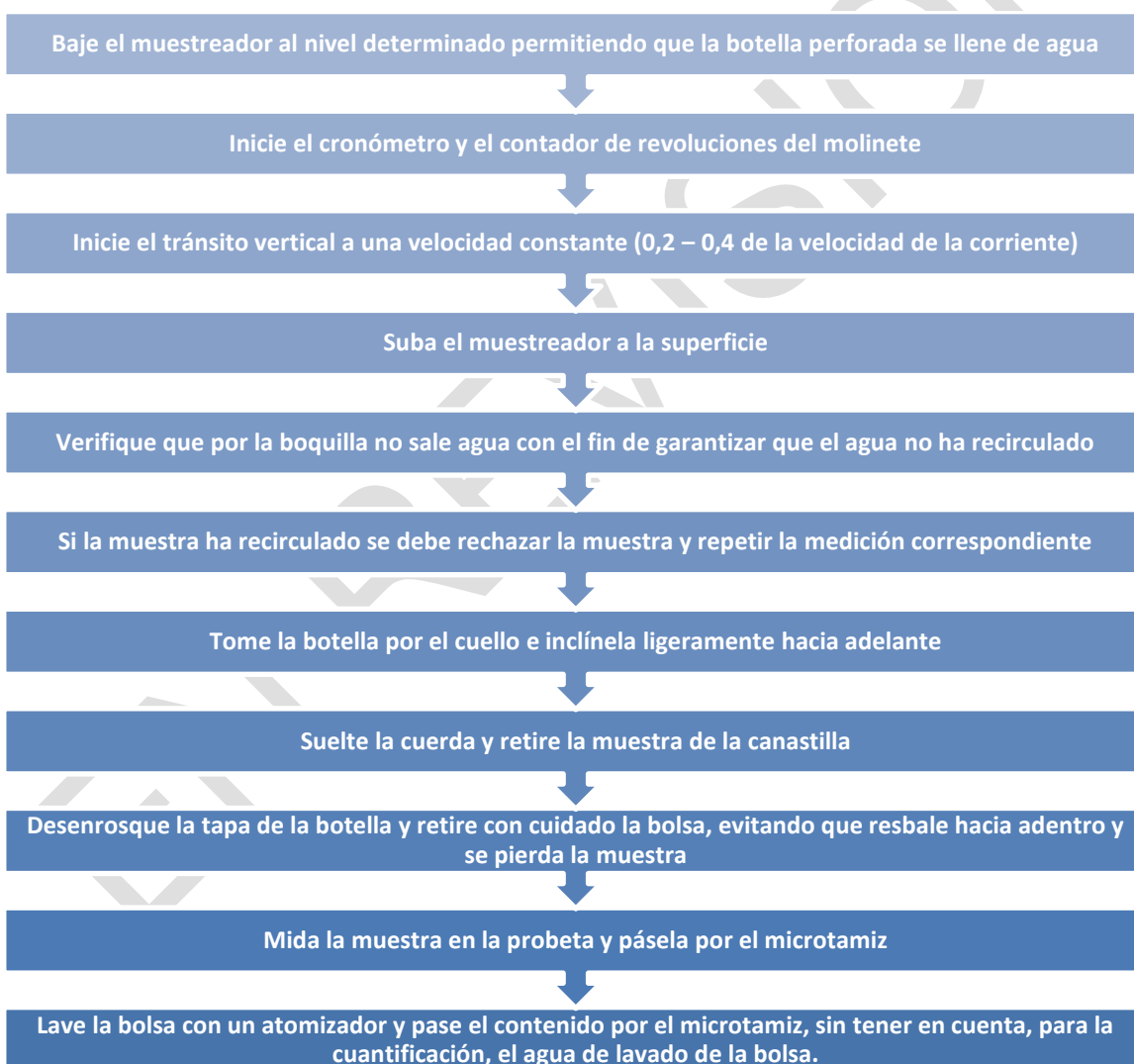
Figura 112. Procedimiento para realizar el aforo sólido integrado con bolsa plegable. Fuente, (EPAM S.A ESP, 2011)
