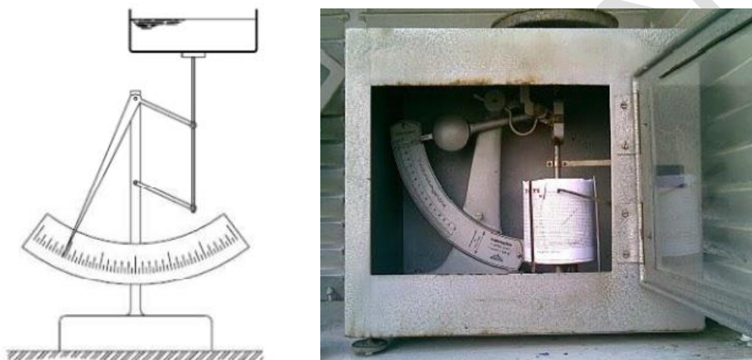
Figura 40. Izquierda: Esquema de evaporímetro tipo Wild. Tomado de (Ruiz Romera & Martínez Santos, 2015). Derecha: Evaporímetro tipo Wild. Tomado de: (Martínez, 2012).
