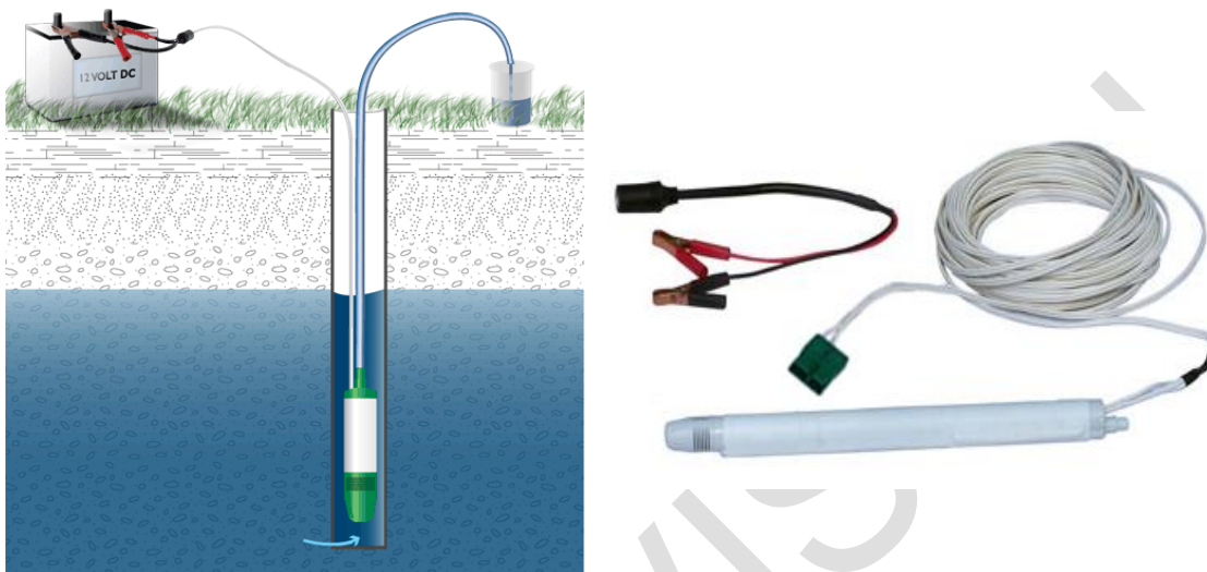
Figura 189. Funcionamiento de bomba eléctrica sumergible. Fuente: (Waterra Pumps Limited, 2016)
