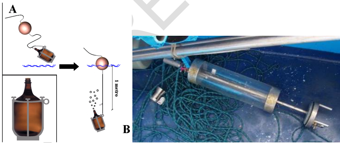
Figura 193. Dispositivo para muestreo de compuestos orgánicos (hidrocarburos y plaguicidas) (A) y botella Ruttner (B).
