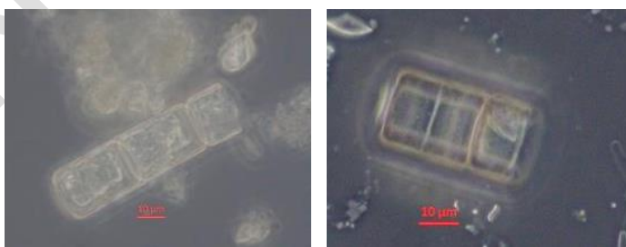
Figura 137. Muestra antes y después de digestión de materia orgánica. En A se observa una muestra antes de realizar la digestión de materia orgánica. En B se observa una muestra luego de la digestión de materia orgánica, con lo que se logra observar en los frústulos el detalle necesario para la determinación taxonómica. Fotos por: Luisa Lagos, 2015
