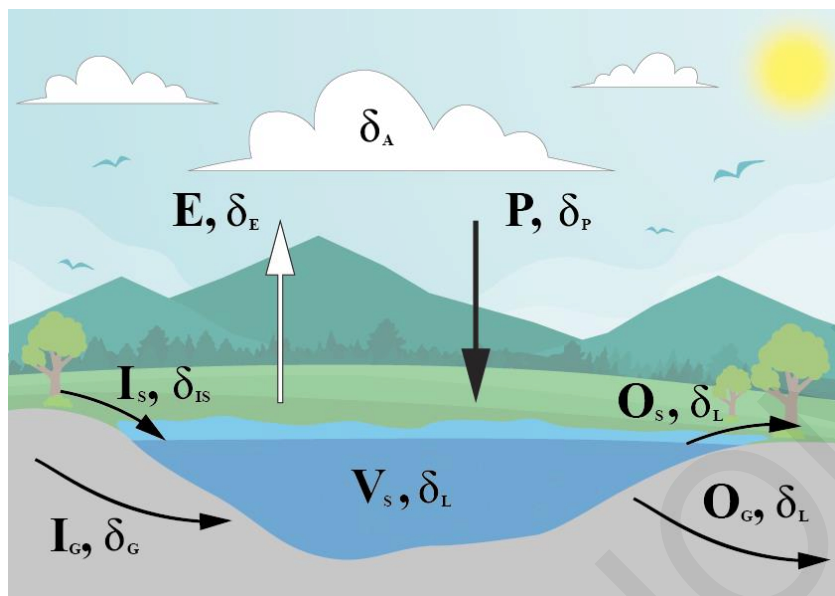
Figura 145. Esquema que describe los componentes del balance hidrológico e isotópico de un sistema lacustre. Los flujos de agua están representados con letras mayúsculas, mientras que su composición isotópica se describe mediante los valores \delta correspondientes. Fuente. (Rozanski, Froehlich, & Mook, 2014)
