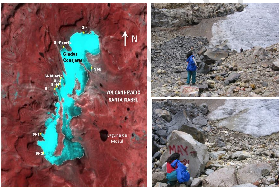
Figura 96. Puntos de retroceso longitudinal monitoreados a 2015 en el volcán nevado Santa Isabel por el IDEAM. (Imagen Spot 2006.). Fuente: Izquierda (Ceballos Liévano, 2015); Derecha: Fotos de campañas de monitoreo de glaciares colombianos, IDEAM, 2005.
