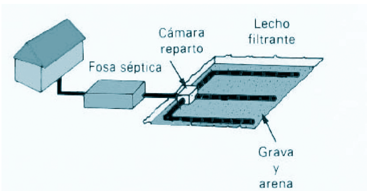
FIGURA 4. Lecho filtrante.
