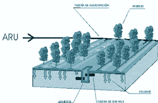
FIGURA 1. Filtro verde.
