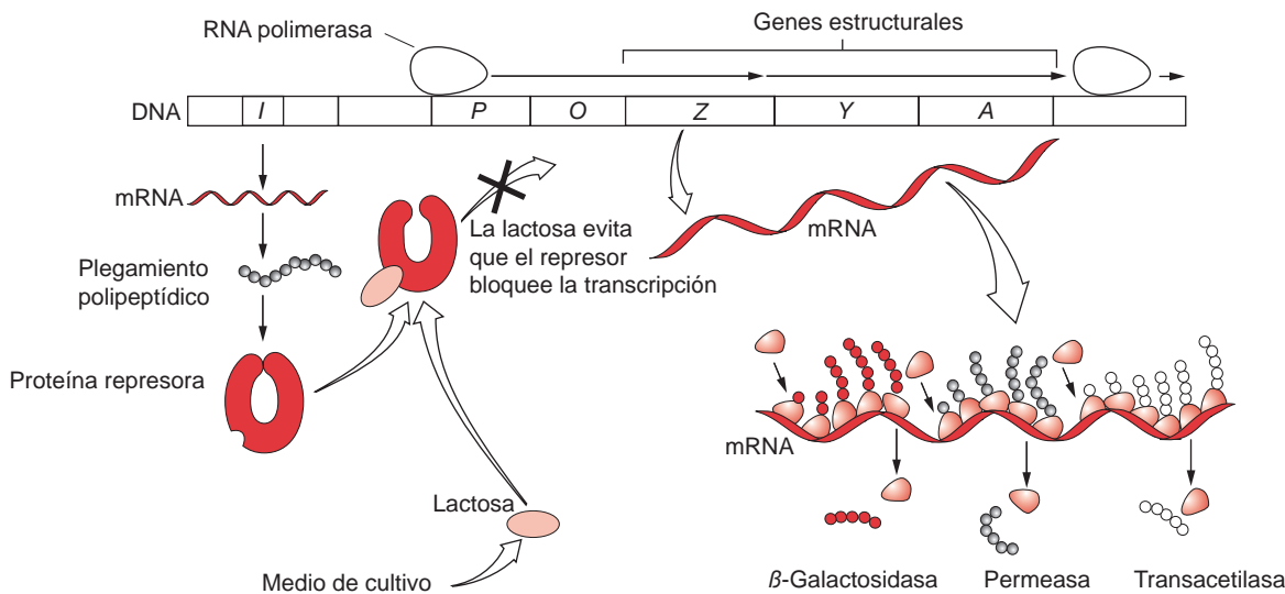
Figura 2.17 El operón lac Mediante el control del operón lac , las células bacterianas pueden regular la expresión génica en respuesta a la disponibilidad de lactosa. En ausencia de lactosa, el represor lac se une al operador bloqueando la transcripción del operón. En presencia de lactosa, ésta se une e inactiva al represor permitiendo que ocurra la transcripción del operón.
