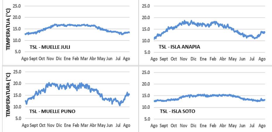
Figura 1. Variación diaria de la Temperatura Superficial del Lago: Muelle Puno, Muelle Juli, Isla Soto e Isla Anapia. Agosto 2019
