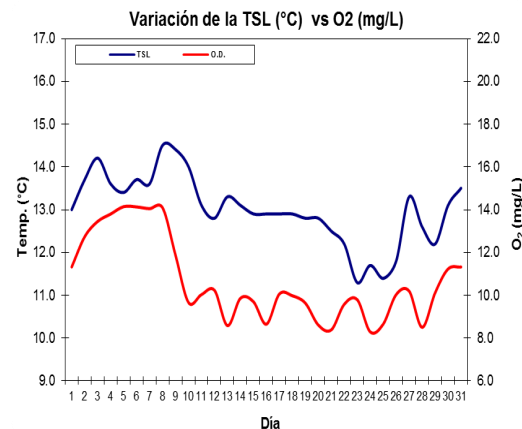
Figura 3. Variación de la TSL versus oxígeno disuelto en la estación Muelle Puno. Agosto 2019
