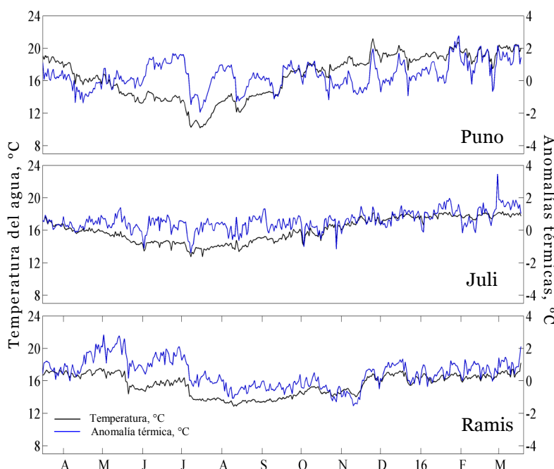
Figura 2. Series de tiempo de la temperatura superficial del agua (°C, línea sólida de color negro) y sus anomalías (°C, línea sólida de color azul) en tres estaciones del Lago Titicaca el 18 de marzo de 2016.
