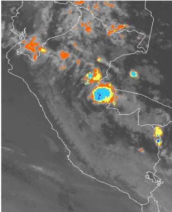
Imagen de Satélite 25/06/13 Hora Local 06:30 AM
