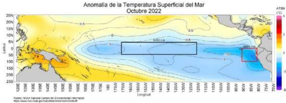
Figura 1: Promedio mensual de las anomalías de TSM en el Pacífico en octubre de 2022. La región Niño 3.4 está delimitada con el recuadro negro y la región Niño 1+2 está delimitada con el recuadro rojo. Fuente: ERSST v5.0.
