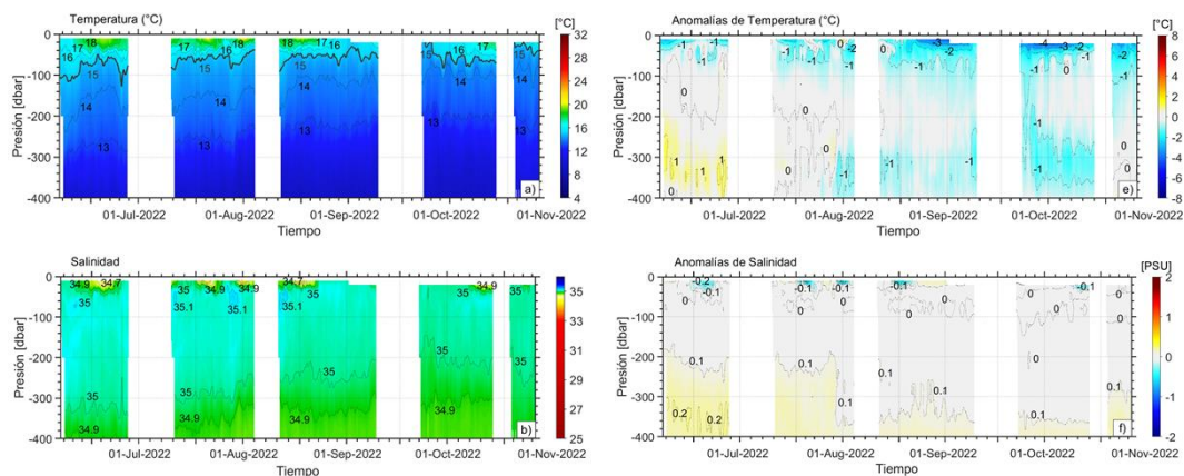
Figura 16. Sección vertical de temperatura ( ^{\circ}\text{C} ), anomalías térmicas ( ^{\circ}\text{C} ), salinidad y anomalías halinas, entre julio y octubre de 2022, registradas por los Gliders Mochica y Chimu frente a Negritos-Talara.
