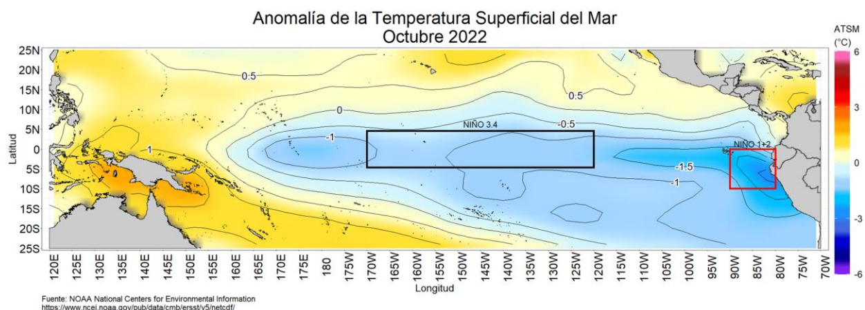
Figura 1: Promedio del mes de octubre 2022 de las anomalías de la TSM en el Pacífico. La región Niño 3.4 está delimitada con el recuadro negro y la región Niño 1+2 está delimitada con el recuadro rojo. Fuente: ERSSTv5.0. Procesamiento: DIHIDRONAV.
