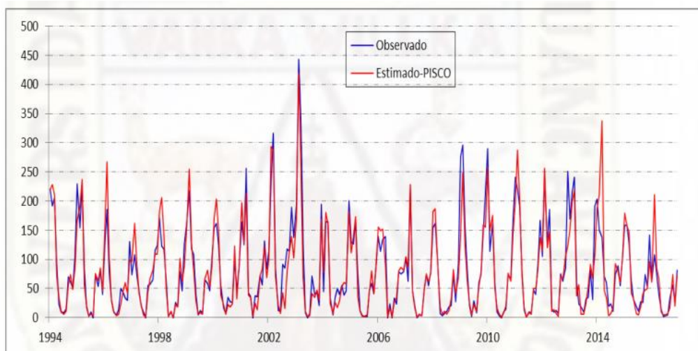
Figura 5 Serie temporal de la precipitación de la estación meteorológica Huancavelica-Senamhi
