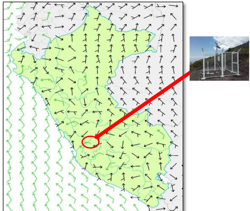
Figura 4 Mapa de viento
