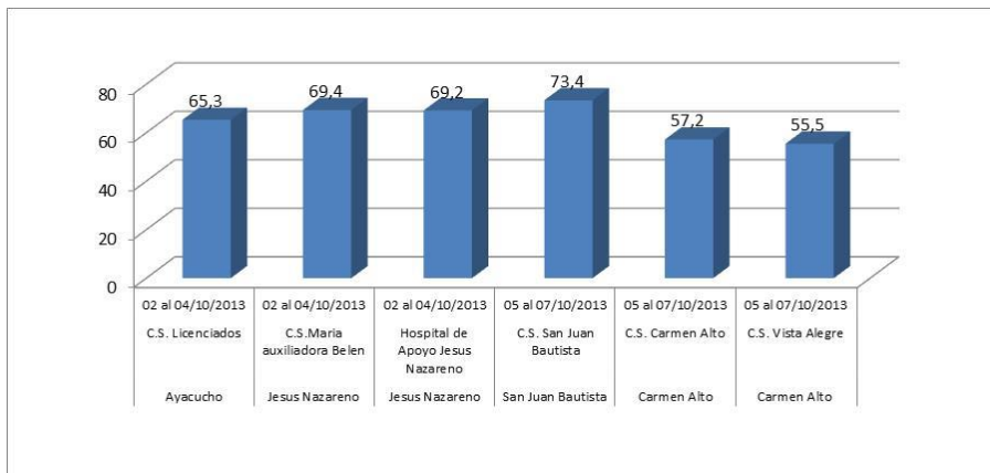
Gráfico N° 49 CONCENTRACIÓN PROMEDIO DE PM10 AYACUCHO 2012. ECA (24 horas)=150ug/m 3
