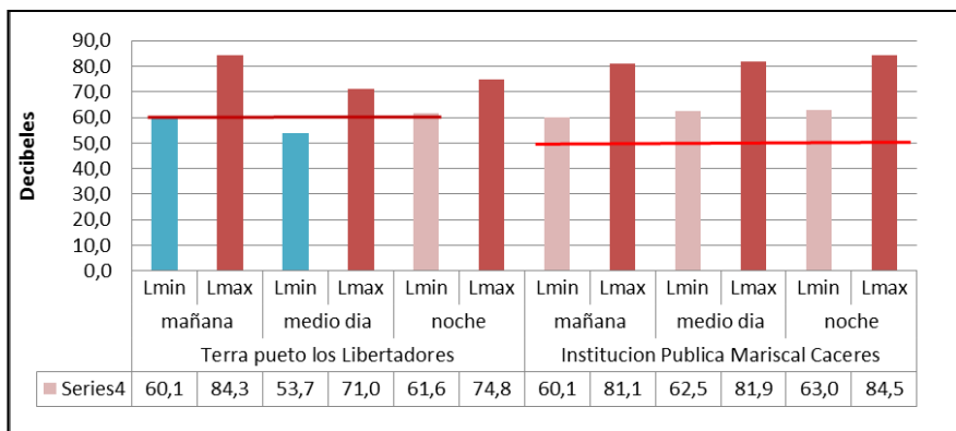
Gráfico N° 51 NIVELES SONOROS REGISTRADOS EN LOS PRINCIPALES PUNTOS CRÍTICOS DE LA PROVINCIA DE HUAMANGA 2015
