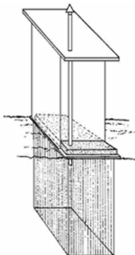
Letrina de hoyo seco ventilado
