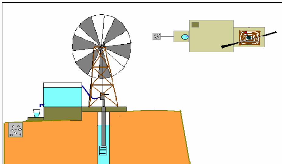
Sistemas típicos con reservorio elevado y apoyado. En el primer caso el nivel de servicio es por conexiones domiciliarias
