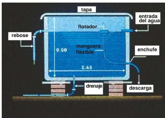
Hipoclorador simple
