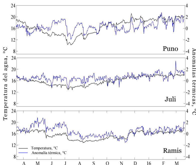
Figura 2. Series de tiempo de la temperatura superficial del agua (°C, línea sólida de color negro) y sus anomalías (°C, línea sólida de color azul) en tres estaciones del Lago Titicaca el 19 de marzo de 2016.
