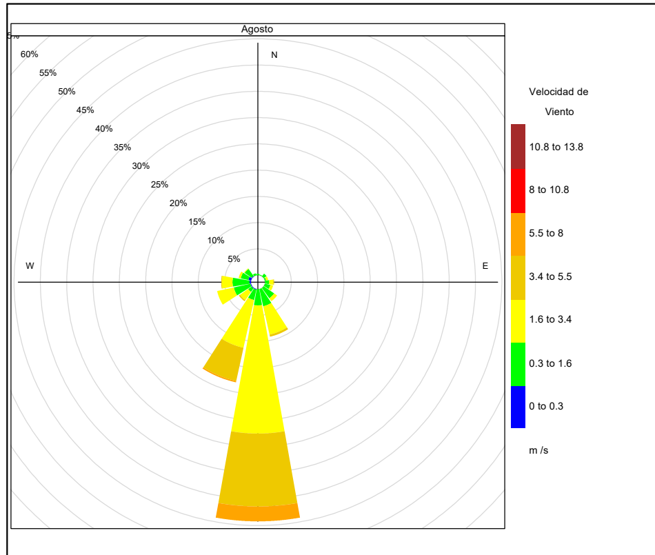
Figura 3.1. Rosa de viento de la estación de monitoreo CA-ILO-01, en agosto de 2022
