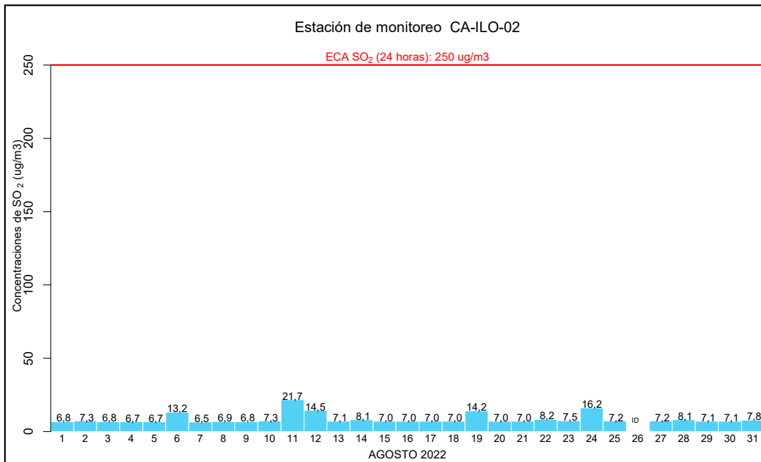
Figura 3.11. Concentraciones de 24 horas de SO 2 en la estación de monitoreo CA-ILO-02, en agosto de 2022
