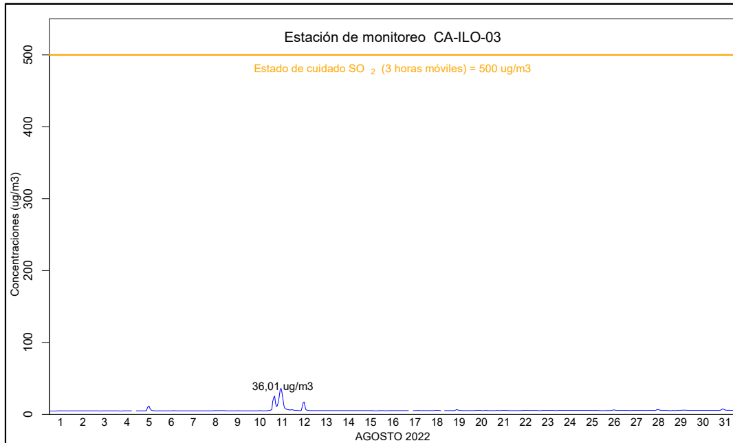
Figura 4.3. Concentraciones de promedio móvil de 3 horas de \text{SO}_2 en la estación de monitoreo CA-ILO-03, en agosto de 2022
