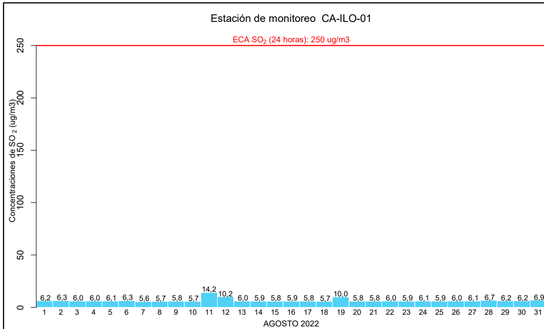
Figura 3.10. Concentraciones de 24 horas de SO 2 en la estación de monitoreo CA-ILO-01, en agosto de 2022
