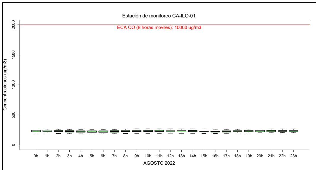
Figura 3.21. Concentraciones de promedio móvil de 8 horas de CO en la estación de monitoreo CA-ILO-01, en agosto de 2022
