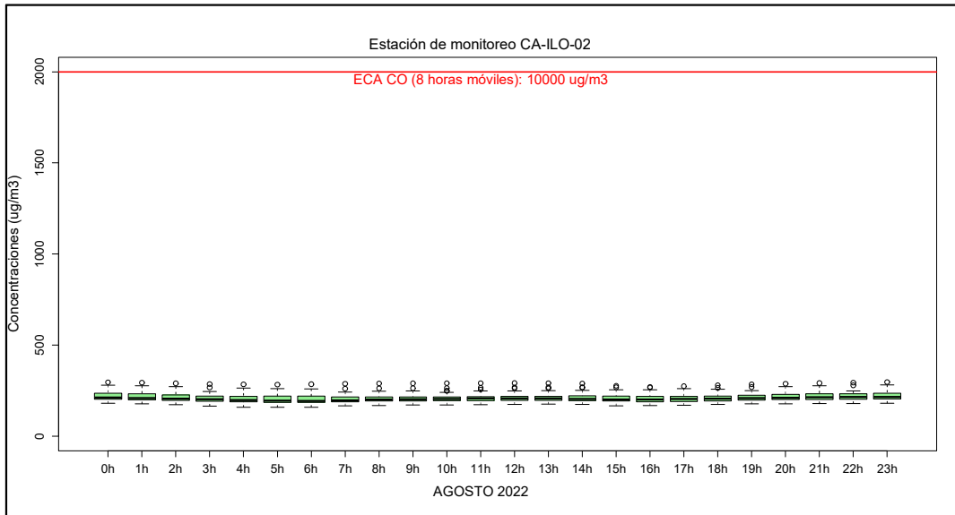
Figura 3.22. Concentraciones de promedio móvil de 8 horas de CO en la estación de monitoreo CA-ILO-02, en agosto de 2022
