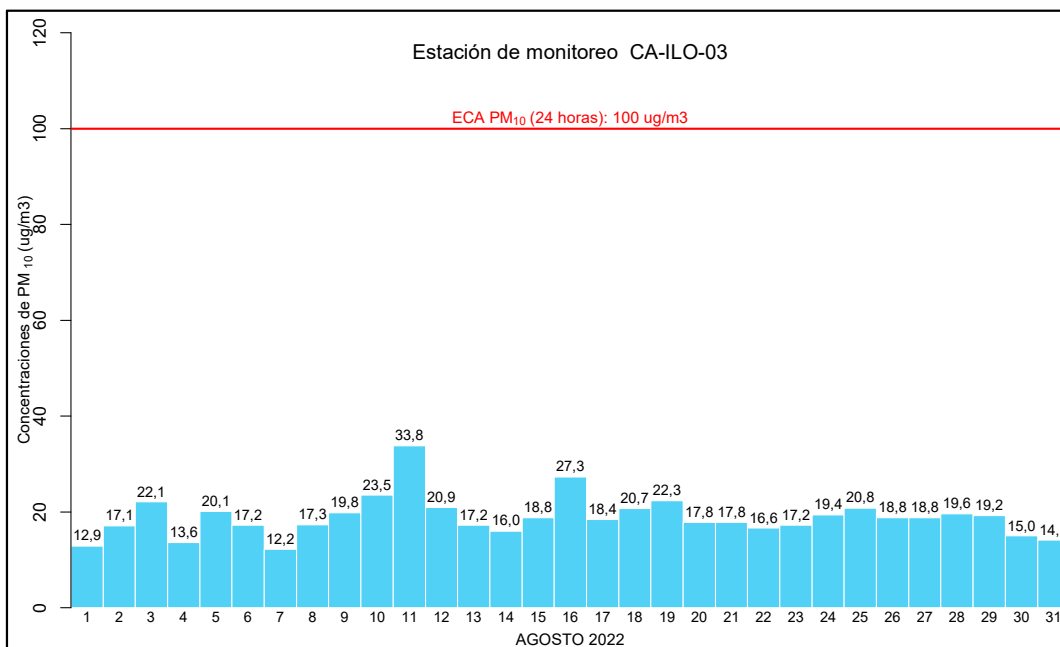
Figura 3.9. Concentraciones de 24 horas de PM 10 en la estación de monitoreo CA-ILO-03, en agosto de 2022
