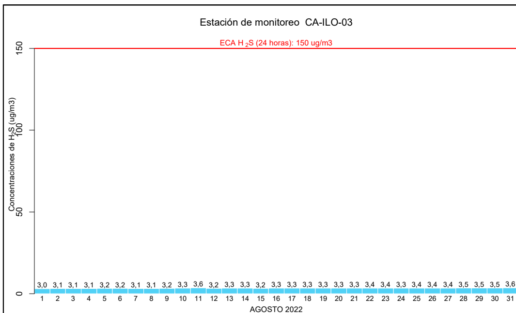
Figura 3.15. Concentraciones de 24 horas de H 2 S en la estación de monitoreo CA-ILO-03, en agosto de 2022.
