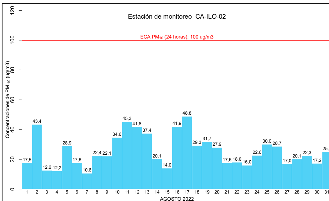
Figura 3.8. Concentraciones de 24 horas de PM 10 en la estación de monitoreo CA-ILO-02, en agosto de 2022
