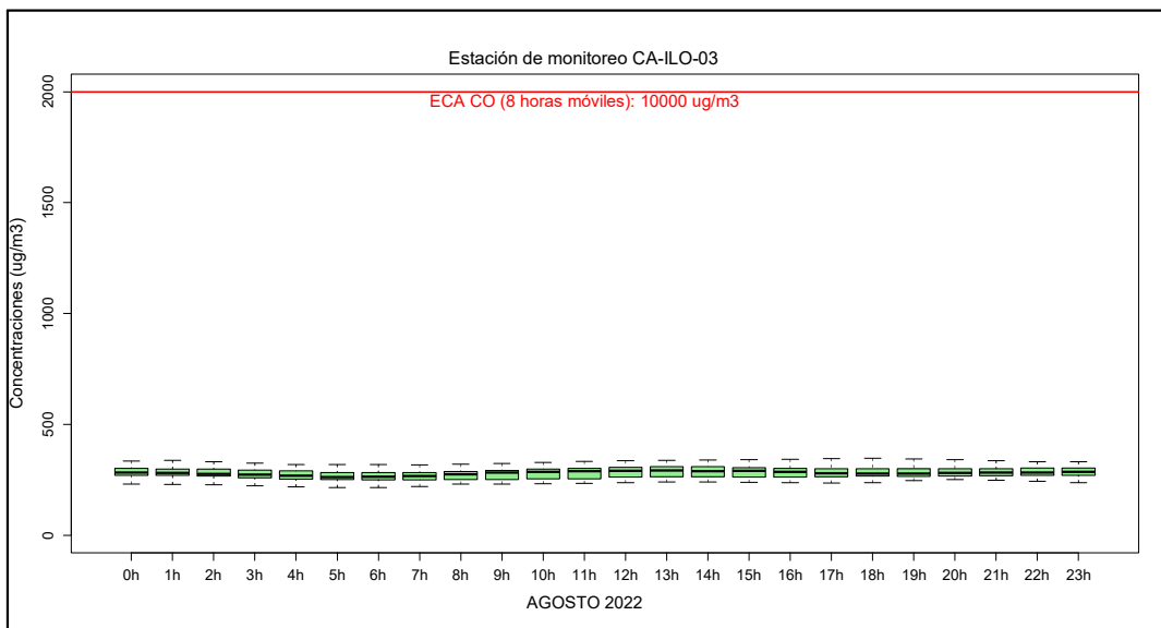
Figura 3.23. Concentraciones de promedio móvil de 8 horas de CO en la estación de monitoreo CA-ILO-03, en agosto de 2022
