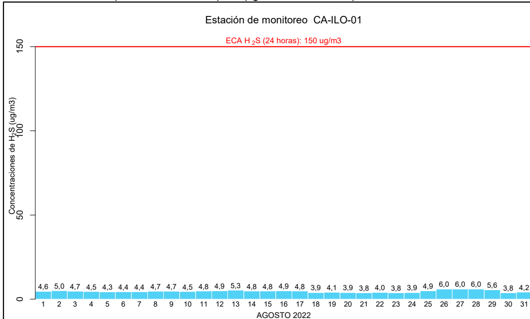
Figura 3.13. Concentraciones de 24 horas de H 2 S en la estación de monitoreo CA-ILO-01, en agosto de 2022
