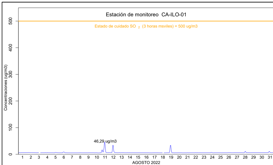
Figura 4.1. Concentraciones de promedio móvil de 3 horas de \text{SO}_2 en la estación de monitoreo CA-ILO-01, en agosto de 2022
