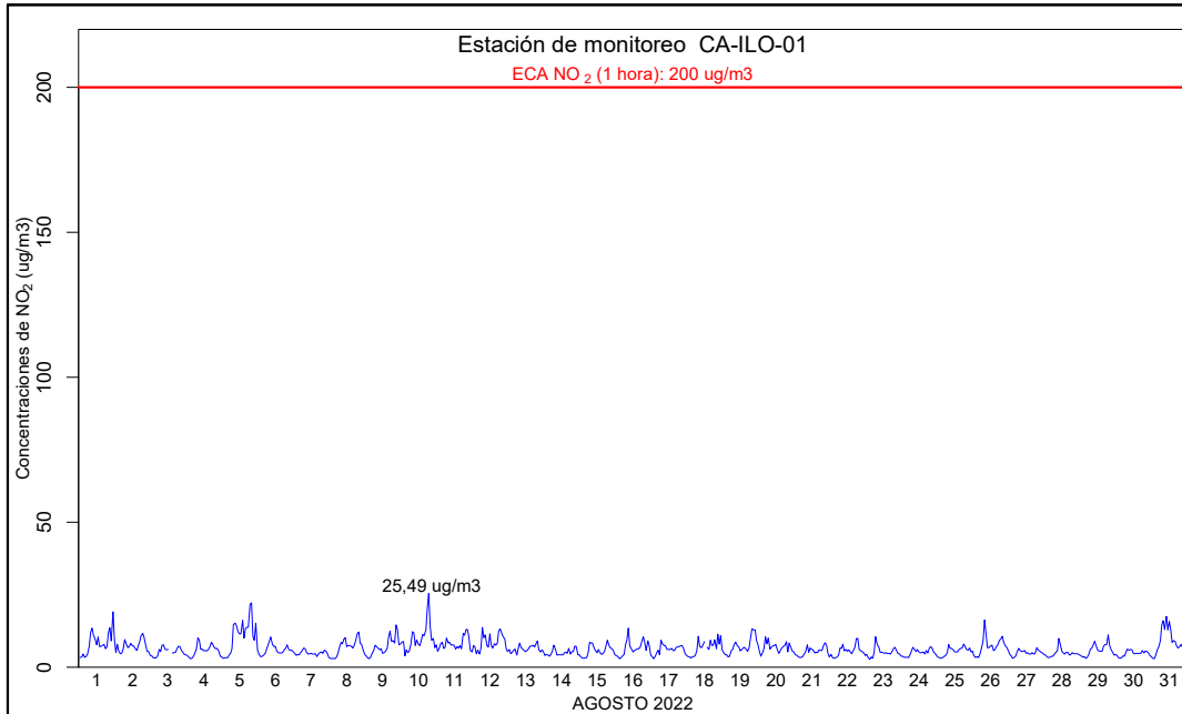
Figura 3.16. Concentraciones de horarias de NO 2 en la estación de monitoreo CA-ILO-01, en agosto de 2022.
