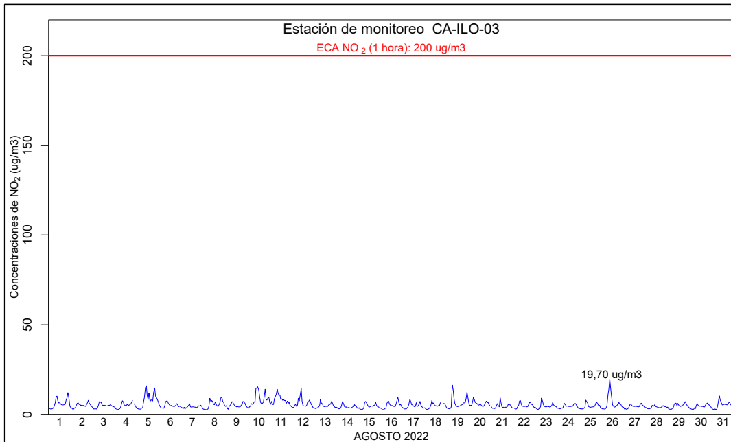
Figura 3.17. Concentraciones de horarias de NO 2 en la estación de monitoreo CA-ILO-03, en agosto de 2022.
