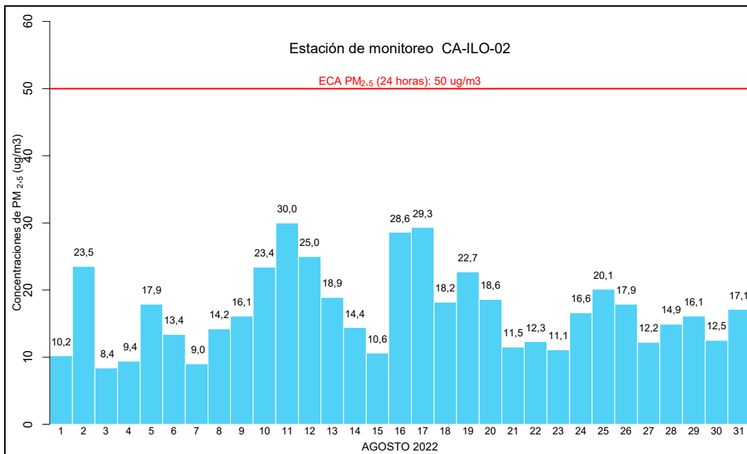
Figura 3.5. Concentraciones de 24 horas de PM 2.5 en la estación de monitoreo CA-ILO-02, en agosto de 2022
