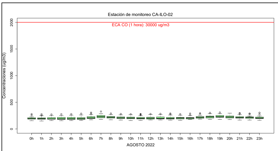
Figura 3.19. Concentraciones horarias de CO, estación de monitoreo CA-ILO-02, agosto del 2022
