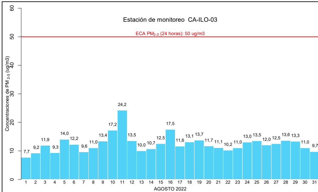
Figura 3.6. Concentraciones de 24 horas de PM 2,5 en la estación de monitoreo CA-ILO-03, en agosto de 2022
