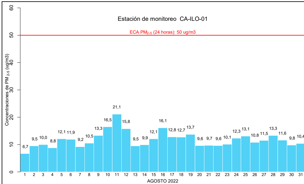
Figura 3.4. Concentraciones de 24 horas de PM 2.5 en la estación de monitoreo CA-ILO-01, en agosto de 2022
