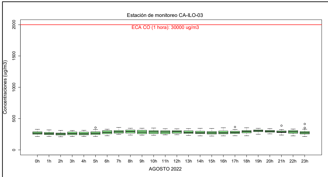
Figura 3.20. Concentraciones horarias de CO, estación de monitoreo CA-ILO-03, agosto del 2022
