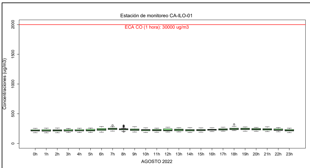
Figura 3.18. Concentraciones horarias de CO, estación de monitoreo CA-ILO-01, agosto del 2022
