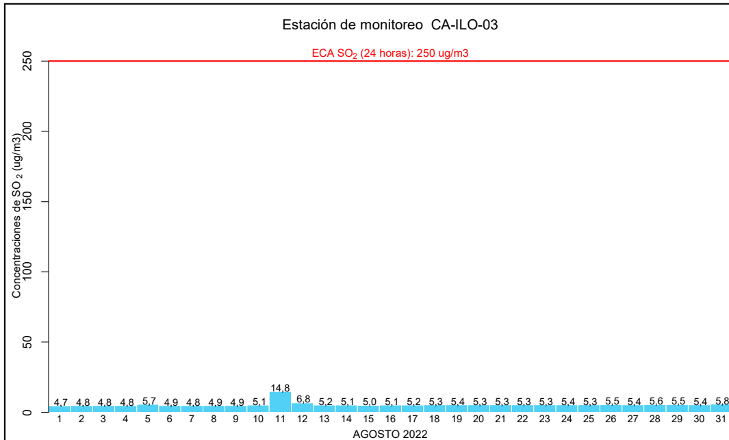
Figura 3.12. Concentraciones de 24 horas de SO 2 en la estación de monitoreo CA-ILO-03, en agosto de 2022.
