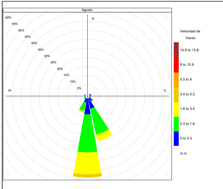
Figura 3.3. Rosa de viento de la estación de monitoreo CA-ILO-03, en agosto de 2022
