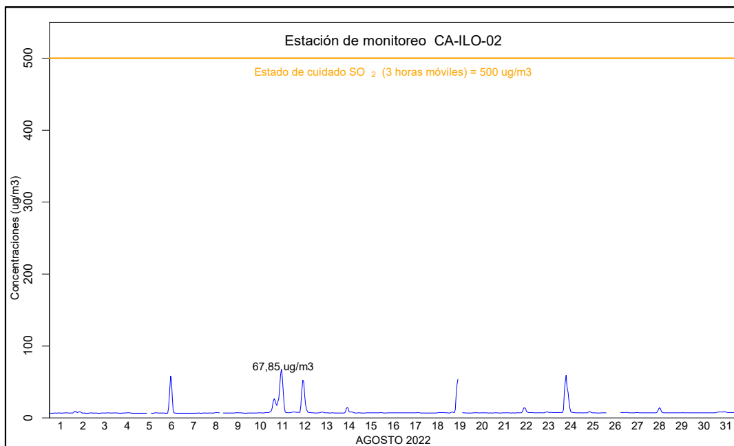
Figura 4.2. Concentraciones de promedio móvil de 3 horas de \text{SO}_2 en la estación de monitoreo CA-ILO-02, en agosto de 2022
