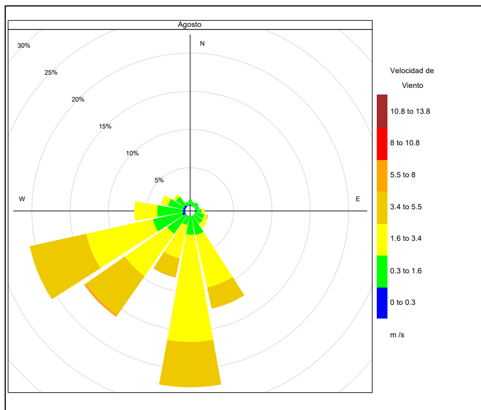
Figura 3.2. Rosa de viento de la estación de monitoreo CA-ILO-02, en agosto de 2022
