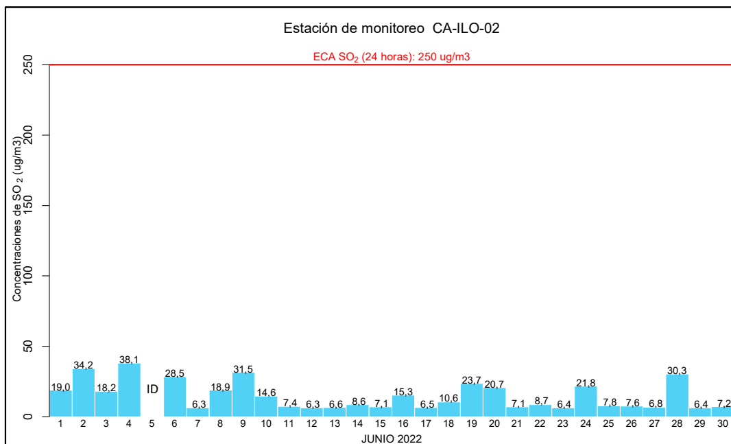
Figura 3.11. Concentraciones de 24 horas de SO 2 en la estación de monitoreo CA-ILO-02, en junio de 2022
