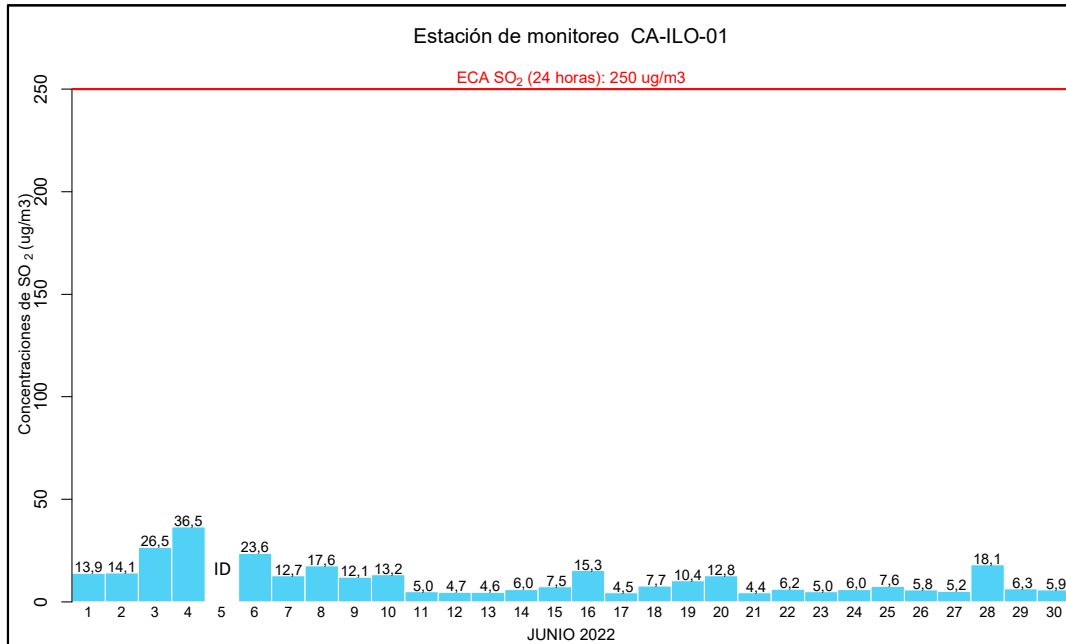
Figura 3.10. Concentraciones de 24 horas de SO 2 en la estación de monitoreo CA-ILO-01, en junio de 2022
