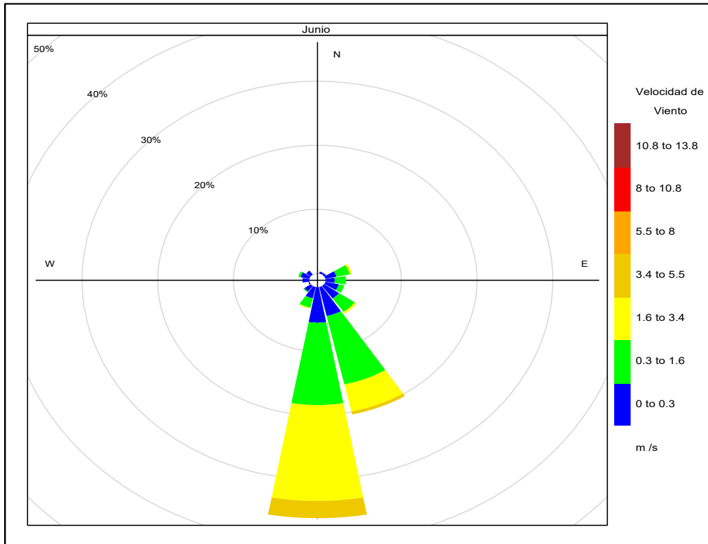
Figura 3.3. Rosa de viento de la estación de monitoreo CA-ILO-03, en junio de 2022
