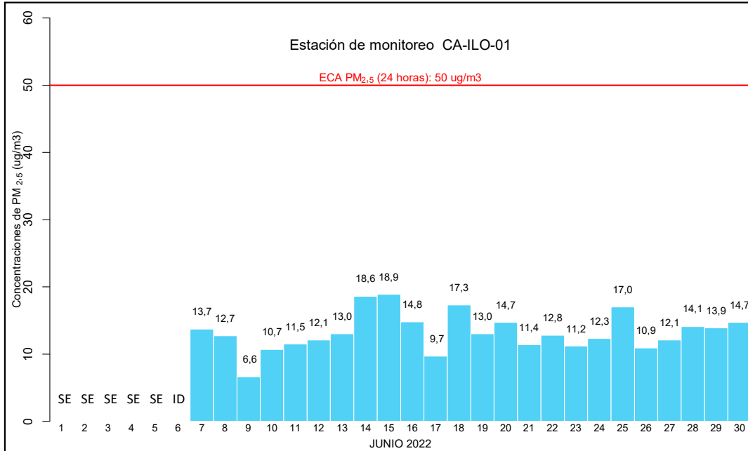
Figura 3.4. Concentraciones de 24 horas de PM 2.5 en la estación de monitoreo CA-ILO-01, en junio de 2022
