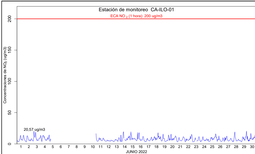
Figura 3.16. Concentraciones de horarias de NO 2 en la estación de monitoreo CA-ILO-01, en junio de 2022
