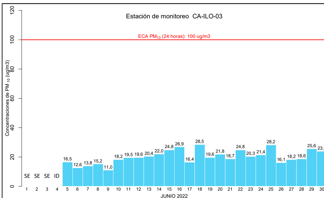
Figura 3.9. Concentraciones de 24 horas de PM 10 en la estación de monitoreo CA-ILO-03, en junio de 2022
