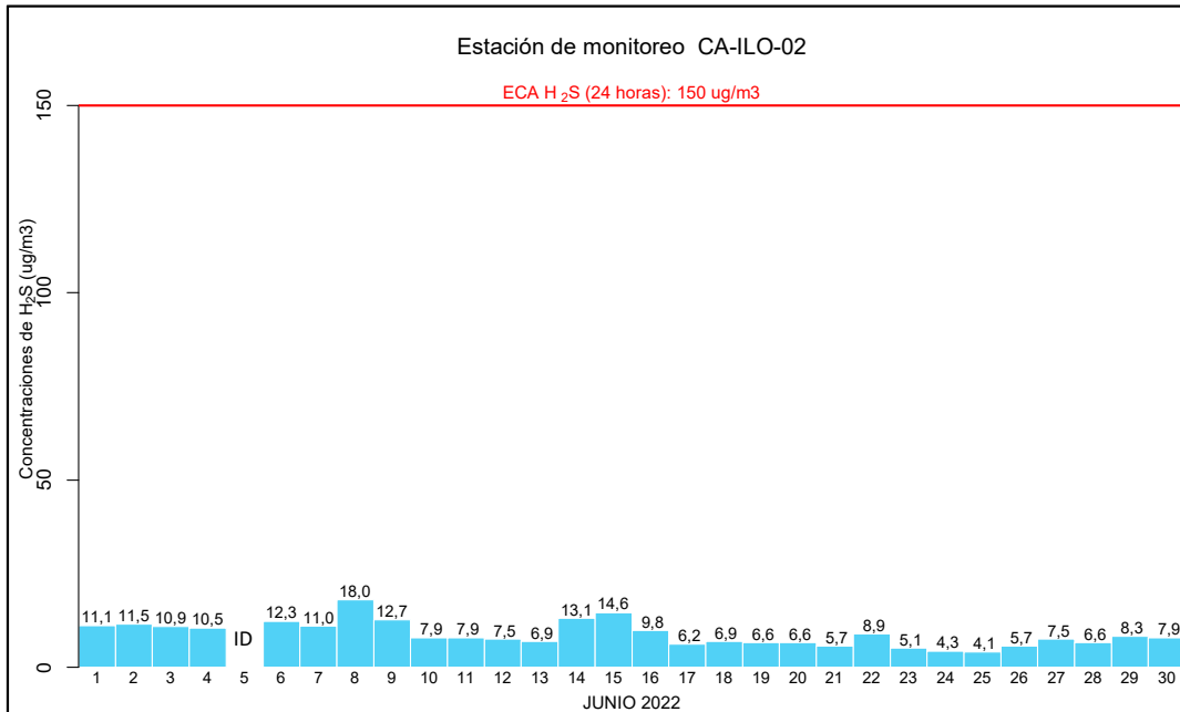
Figura 3.14. Concentraciones de 24 horas de H 2 S en la estación de monitoreo CA-ILO-02, en junio de 2022
