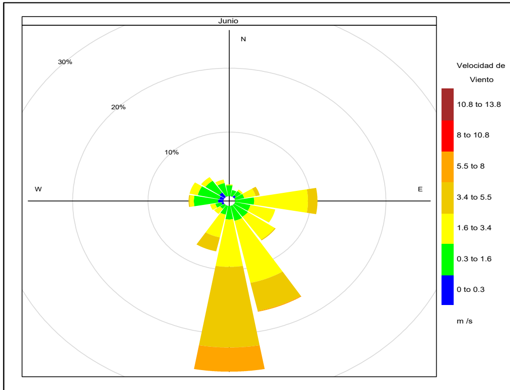
Figura 3.1. Rosa de viento de la estación de monitoreo CA-ILO-01, en junio de 2022
