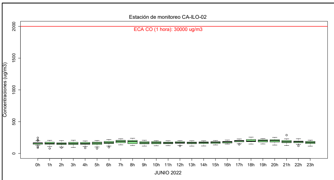
Figura 3.19. Concentraciones horarias de CO, estación de monitoreo CA-ILO-02, junio del 2022
