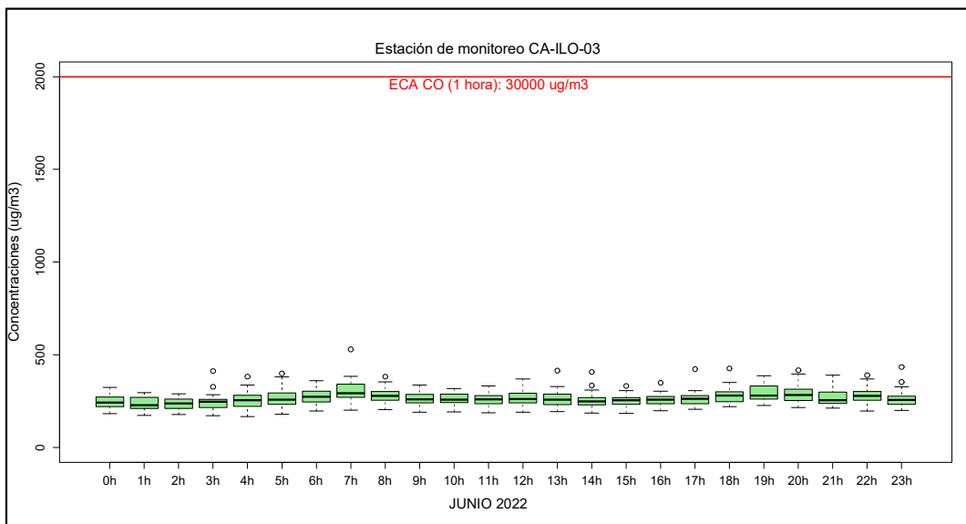
Figura 3.20. Concentraciones horarias de CO, estación de monitoreo CA-ILO-03, junio del 2022
