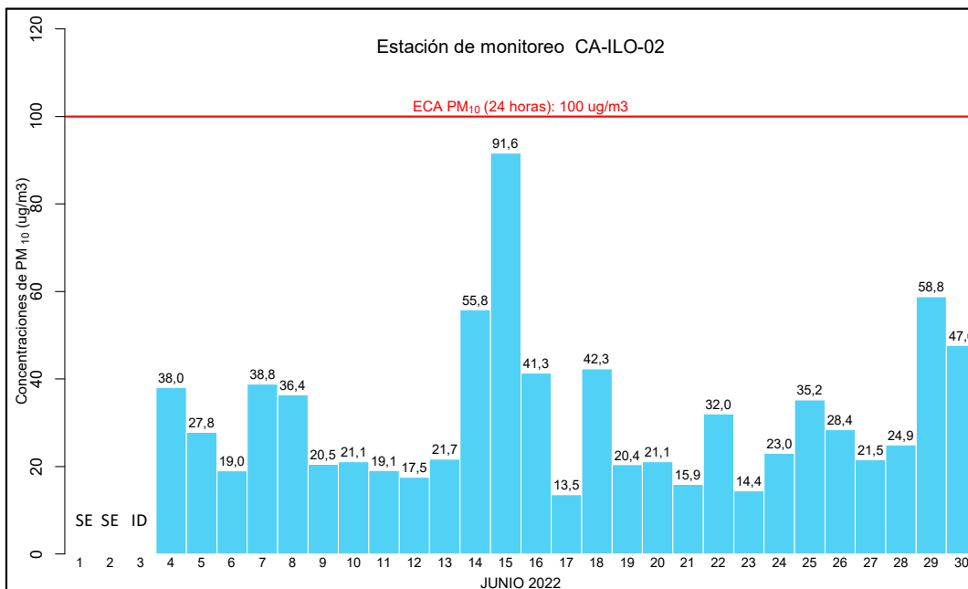
Figura 3.8. Concentraciones de 24 horas de PM 10 en la estación de monitoreo CA-ILO-02, en junio de 2022
