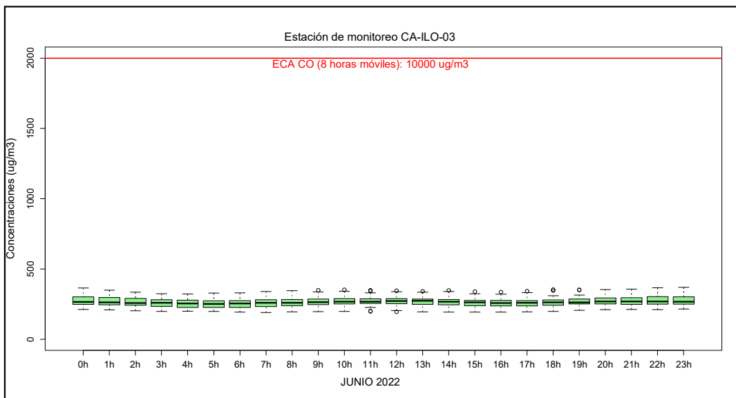
Figura 3.23. Concentraciones de promedio móvil de 8 horas de CO en la estación de monitoreo CA-ILO-03, en junio de 2022
