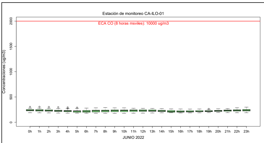
Figura 3.21. Concentraciones de promedio móvil de 8 horas de CO en la estación de monitoreo CA-ILO-01, en junio de 2022
