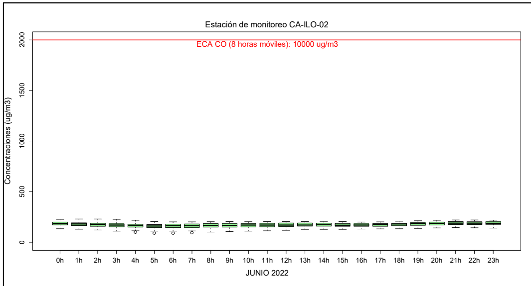
Figura 3.22. Concentraciones de promedio móvil de 8 horas de CO en la estación de monitoreo CA-ILO-02, en junio de 2022
