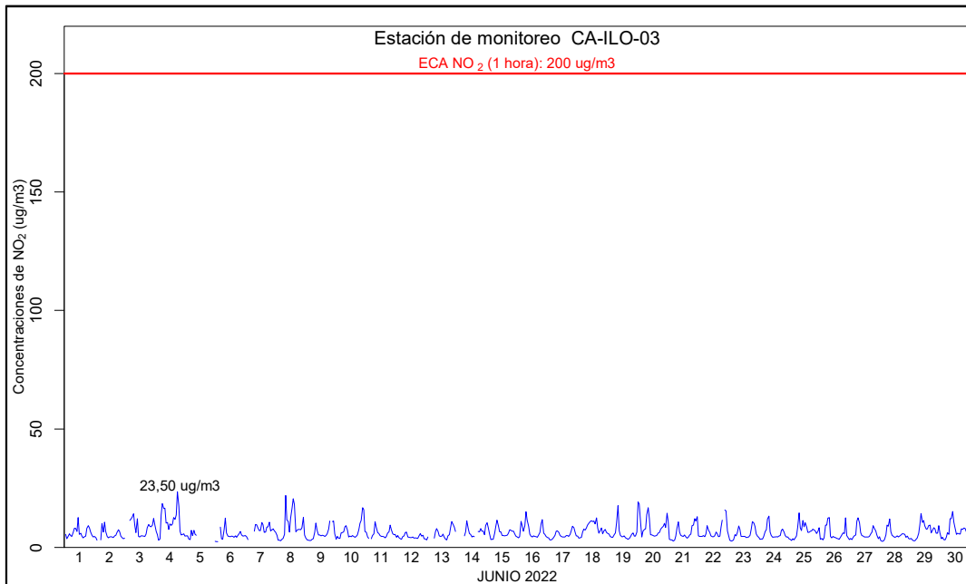
Figura 3.17. Concentraciones de horarias de NO 2 en la estación de monitoreo CA-ILO-03, en junio de 2022
