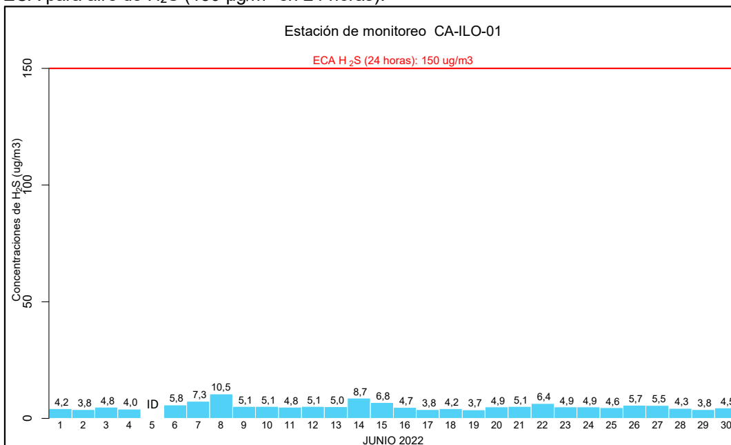
Figura 3.13. Concentraciones de 24 horas de H 2 S en la estación de monitoreo CA-ILO-01, en junio de 2022
