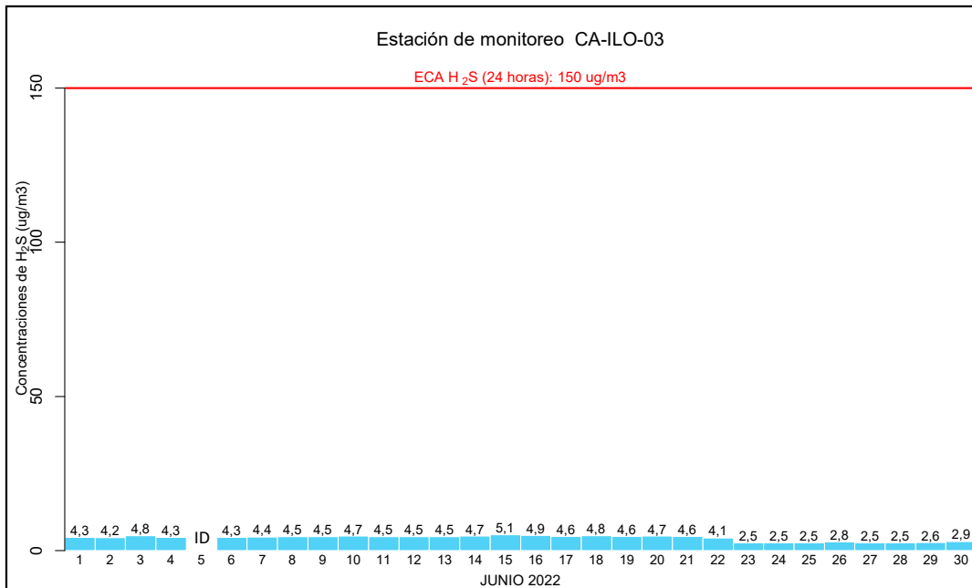
Figura 3.15. Concentraciones de 24 horas de H 2 S en la estación de monitoreo CA-ILO-03, en junio de 2022
