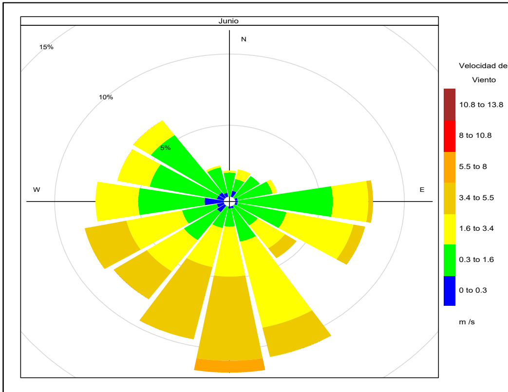
Figura 3.2. Rosa de viento de la estación de monitoreo CA-ILO-02, en junio de 2022
