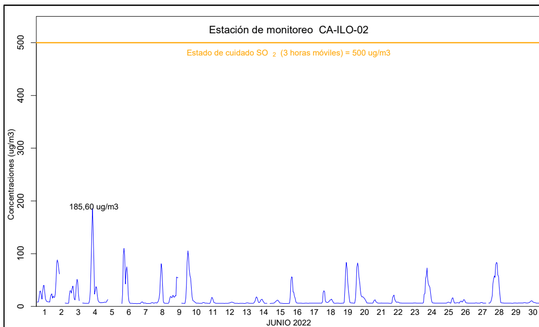
Figura 4.2. Concentraciones de promedio móvil de 3 horas de SO 2 en la estación de monitoreo CA-ILO-02, en junio de 2022
