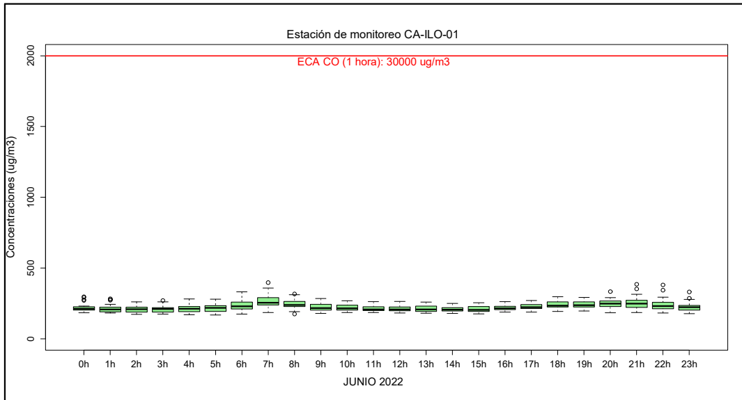
Figura 3.18. Concentraciones horarias de CO, estación de monitoreo CA-ILO-01, junio del 2022
