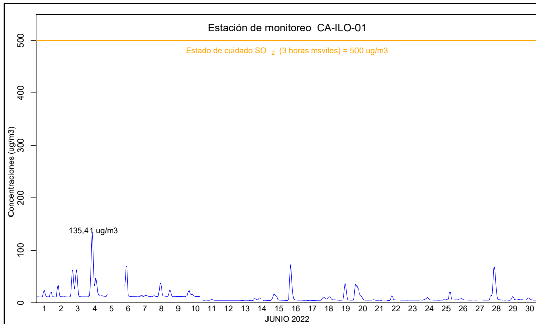
Figura 4.1. Concentraciones de promedio móvil de 3 horas de SO 2 en la estación de monitoreo CA-ILO-01, en junio de 2022
