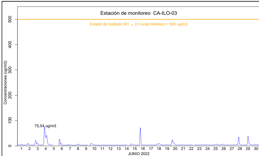
Figura 4.3. Concentraciones de promedio móvil de 3 horas de \text{SO}_2 en la estación de monitoreo CA-ILO-03, en junio de 2022
