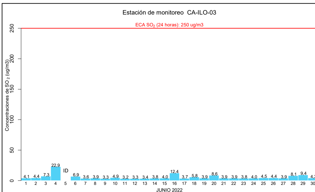
Figura 3.12. Concentraciones de 24 horas de SO 2 en la estación de monitoreo CA-ILO-03, en junio de 2022
