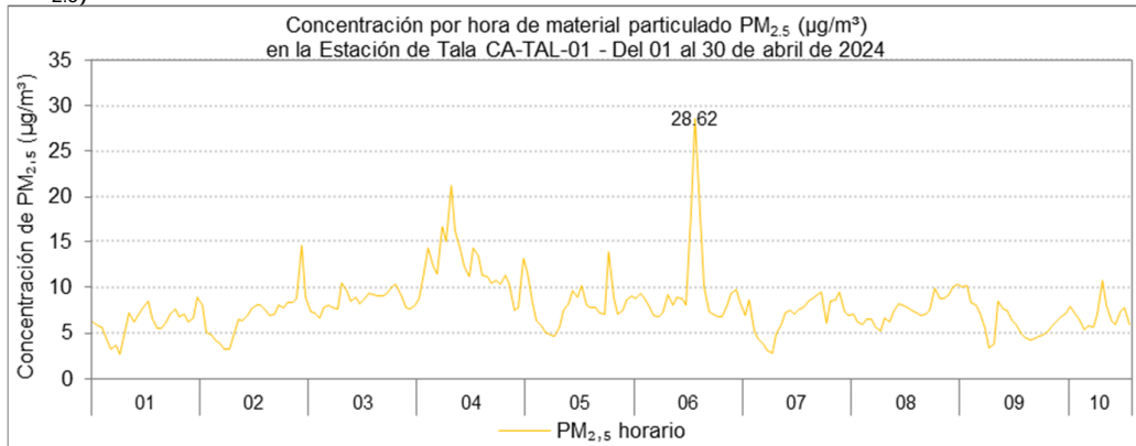
Figura 3.6. Concentración hora de PM_{2,5} en la estación de Tala, del 1 al 10 de abril de 2024
