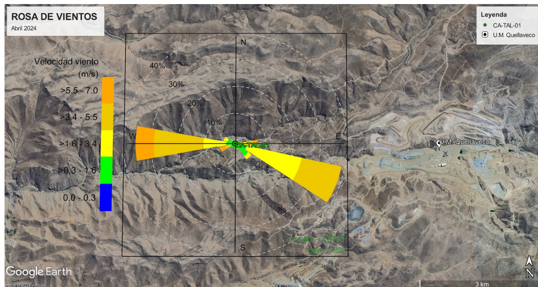
Figura 3.1. Rosa de vientos de la estación de monitoreo CA-TAL-01 (ubicada en Tala), del mes de abril de 2024
