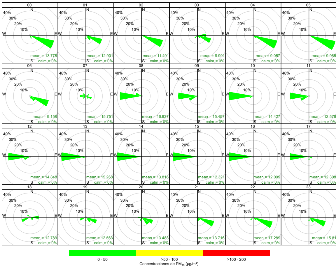
Figura 3.5. Rosas de concentración por horas para el PM 10 , de las 00:00 hasta las 23:00 horas, del mes de abril de 2024.
