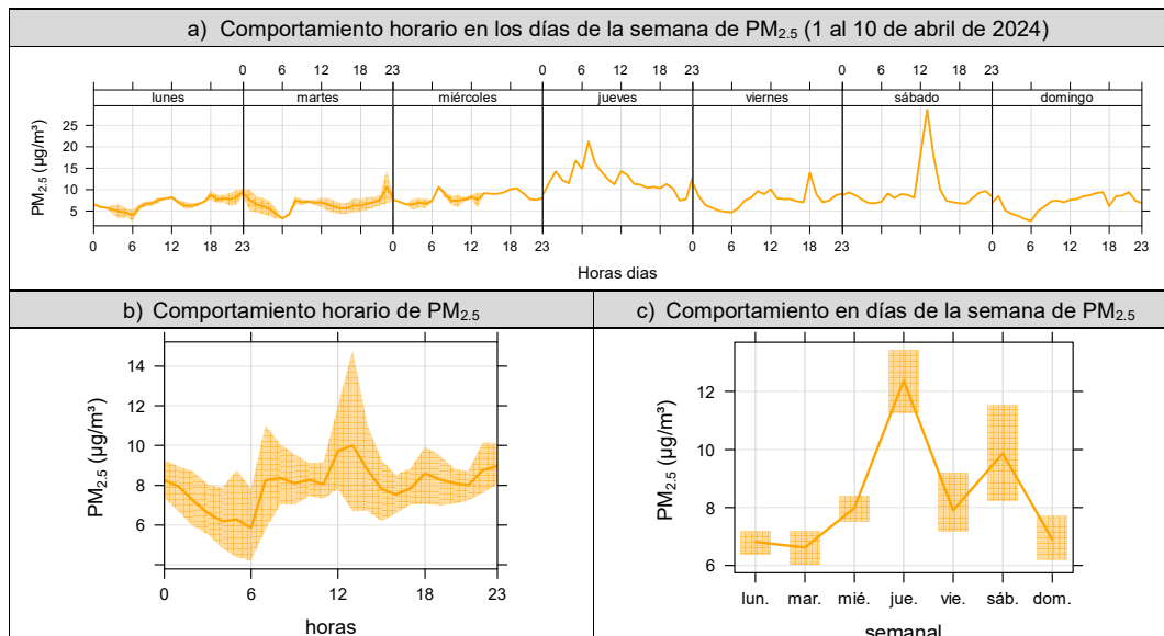
Figura 3.7. Concentraciones promedio (a) horario y por días de la semana, b) horario y c) por días de la semana de PM_{2,5} en la estación de monitoreo CA-TAL-01 (ubicada en Tala), del mes de abril de 2024.
