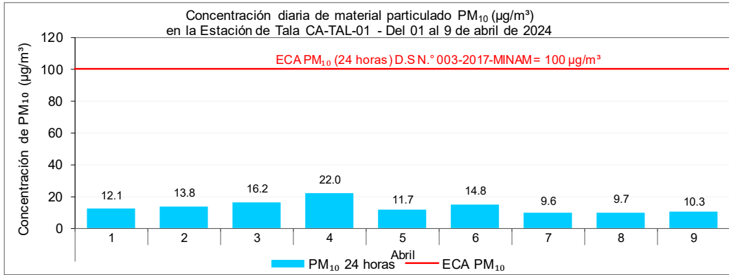
Figura 3.4. Concentración de 24 horas de PM 10 en estación de Tala, 1 al 9 de abril de 2024.
