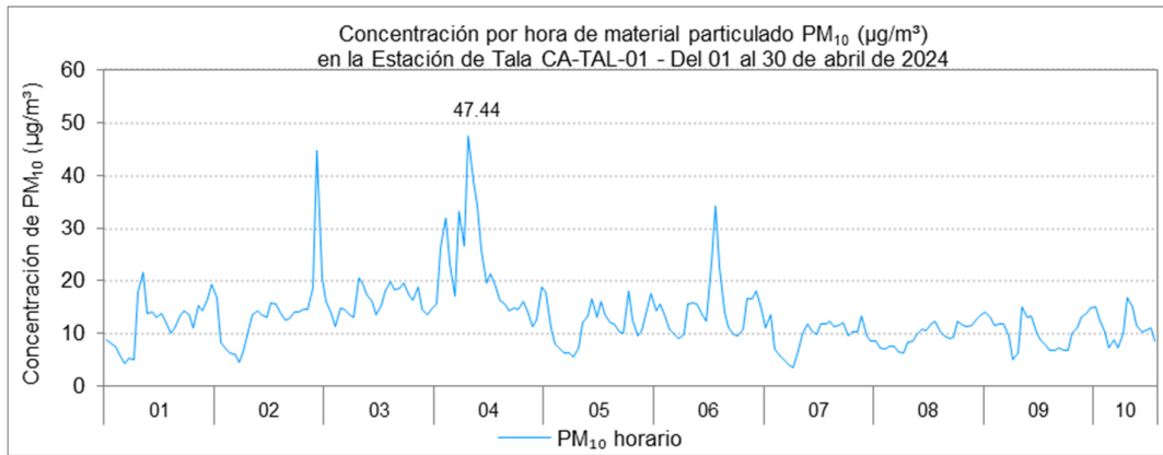
Figura 3.2. Concentración hora de PM_{10} en la estación de Tala, del 1 al 10 de abril de 2024
