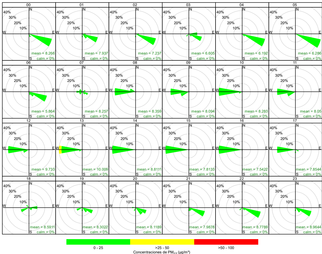
Figura 3.9. Rosas de concentración por horas para PM 2,5 , de 00:00 a 23:00 horas, abril de 2024
