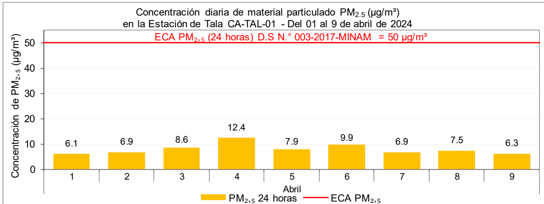
Figura 3.8. Concentración de 24 horas de PM_{2,5} en la estación de Tala, 1 al 9 de abril de 2024.
