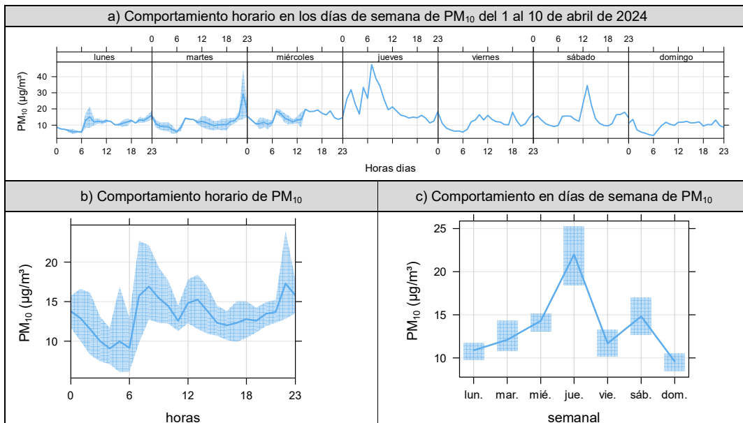
Figura 3.3. Concentraciones promedio (a) horario y por días de la semana, (b) horario y (c) por días de la semana de PM_{10} en la estación de monitoreo CA-TAL-01 (ubicada en Tala), del mes de abril de 2024
