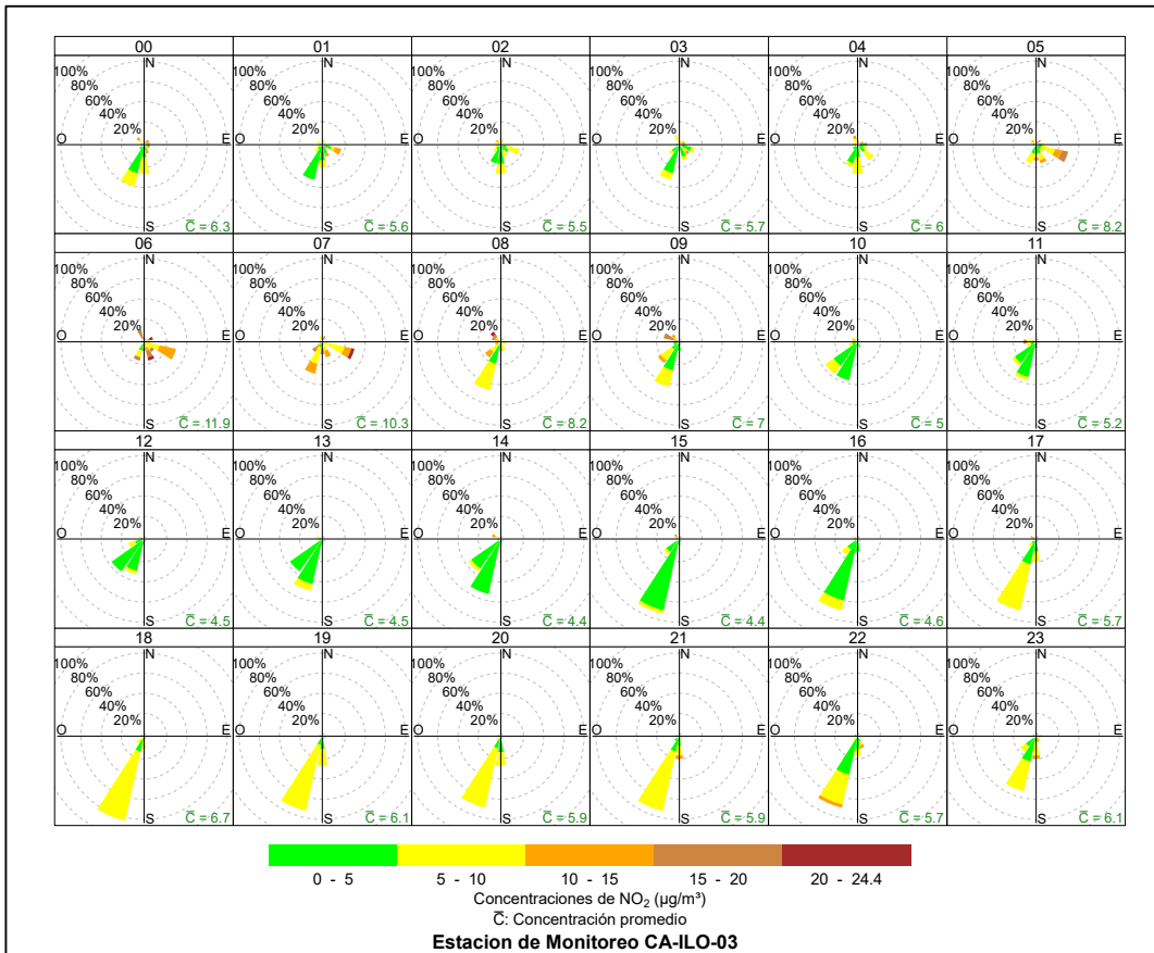
Figura 3.8.30. Rosa de concentración horaria del NO 2 en la estación de monitoreo CA-ILO-03, abril de 2024
