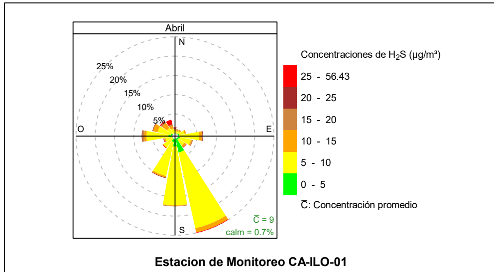
Figura 3.8.19. Rosa de concentración del H 2 S en la estación de monitoreo CA-ILO-01, abril de 2024
