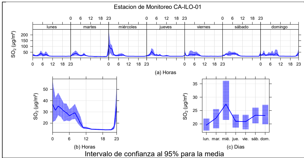
Figura 3.9.7. Concentraciones promedio horarios de SO 2 en la estación de monitoreo CA-ILO-01, de abril de 2024
