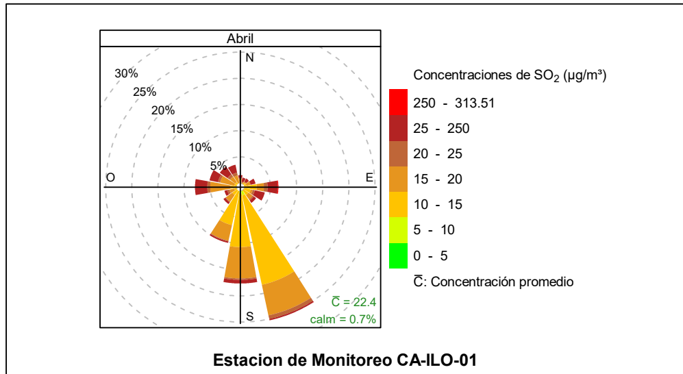
Figura 3.8.13. Rosa de concentración del SO 2 en la estación de monitoreo CA-ILO-01, abril de 2024
