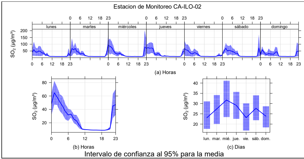
Figura 3.9.8. Concentraciones promedio horarios de SO 2 en la estación de monitoreo CA-ILO-02, de abril de 2024
