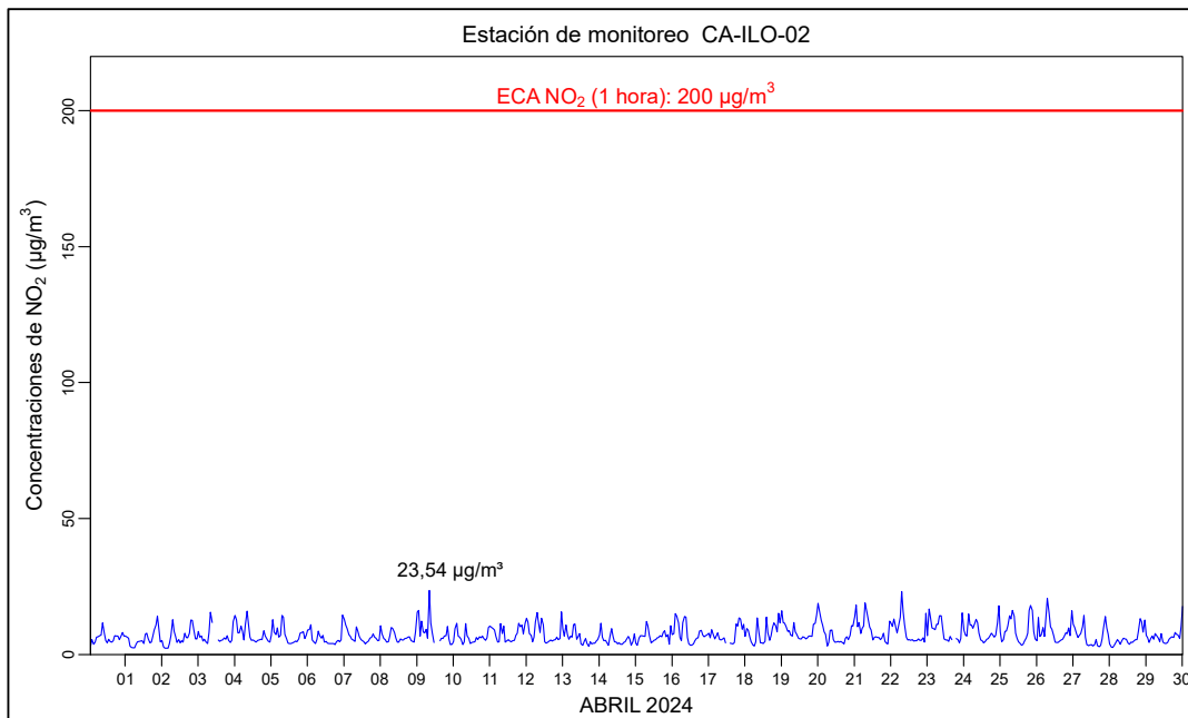
Figura 3.6.2. Concentraciones de horarias de NO 2 en la estación de monitoreo CA-ILO-02, abril de 2024.
