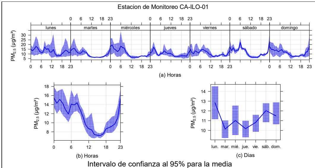
Figura 3.9.1. Concentraciones promedio horarias de PM_{2.5} en la estación de monitoreo CA-ILO-01, de abril de 2024
