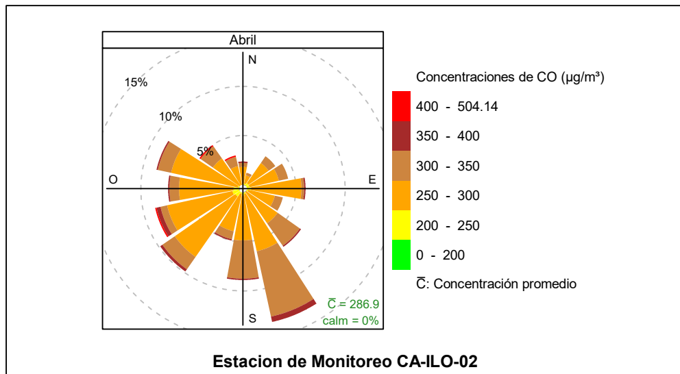
Figura 3.8.32. Rosa de concentración del CO en la estación de monitoreo CA-ILO-02, abril de 2024
