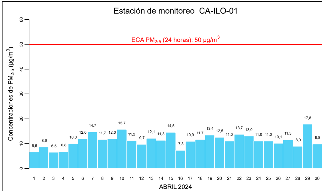
Figura 3.2.1. Concentraciones de 24 horas de PM 2,5 en la estación de monitoreo CA-ILO-01, abril de 2024
