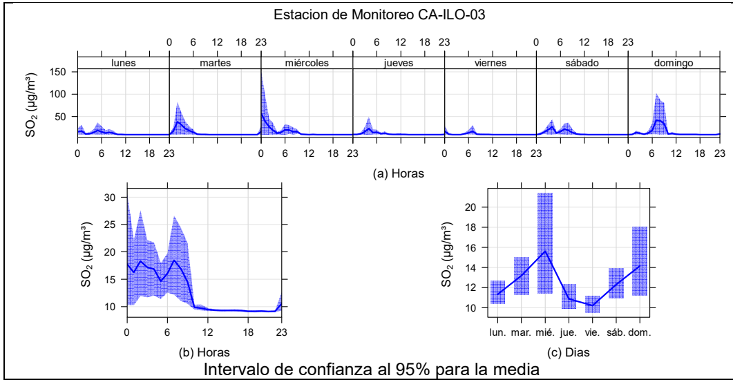
Figura 3.9.9. Concentraciones promedio horarios de SO 2 en la estación de monitoreo CA-ILO-03, de abril de 2024
