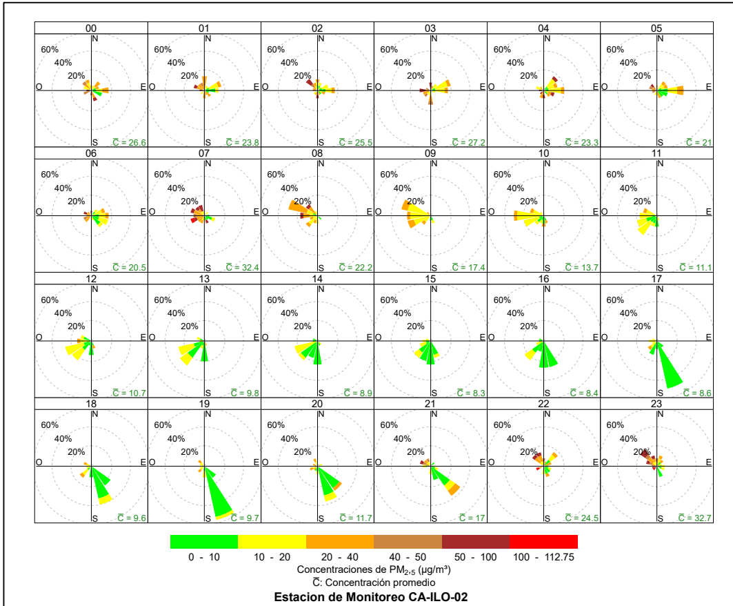
Figura 3.8.5. Rosa de concentración horaria del PM 2.5 en la estación de monitoreo CA-ILO-02, abril de 2024
