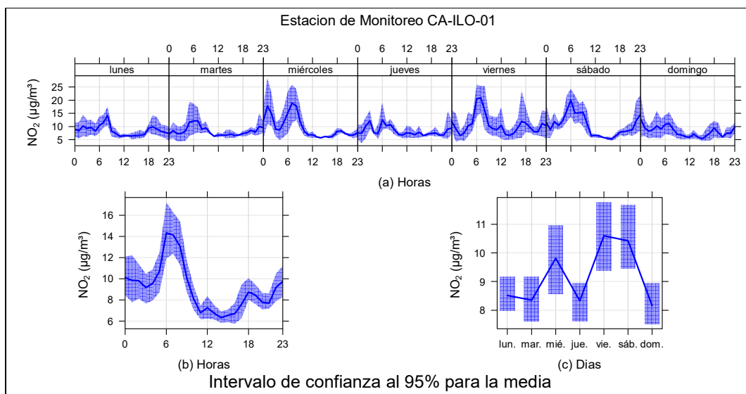
Figura 3.9.13. Concentraciones promedio horarias de NO 2 en la estación de monitoreo CA-ILO-01, de abril de 2024
