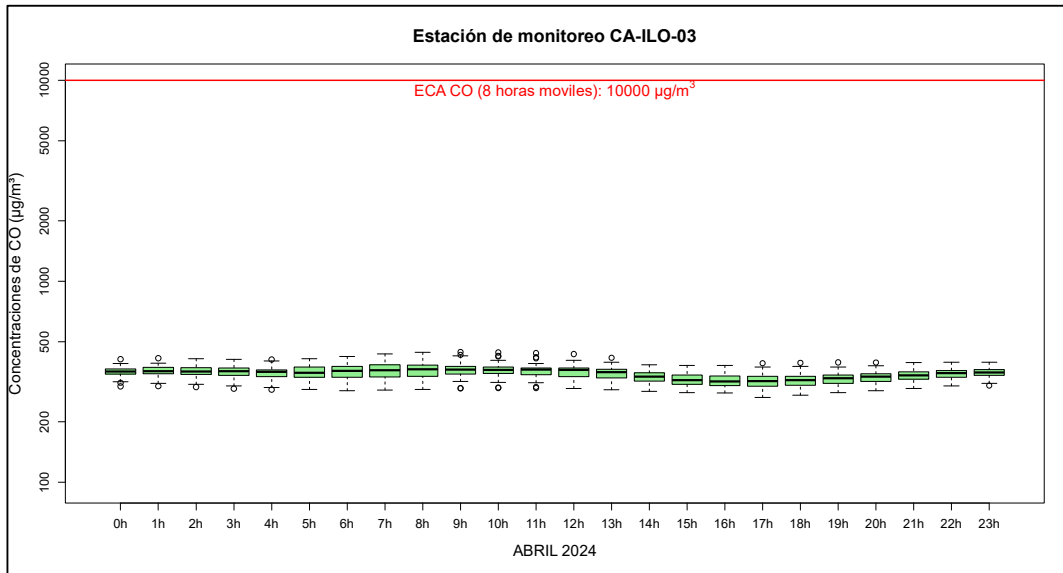
Figura 3.7.6. Concentraciones de promedio móvil de 8 horas de CO en la estación de monitoreo CA-ILO-03, abril de 2024
