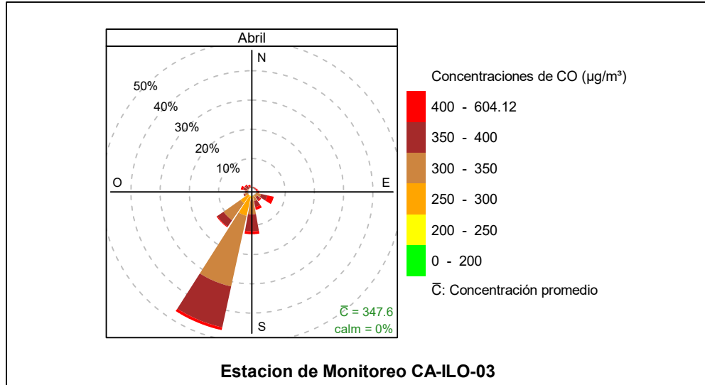
Figura 3.8.33. Rosa de concentración del CO en la estación de monitoreo CA-ILO-03, abril de 2024
