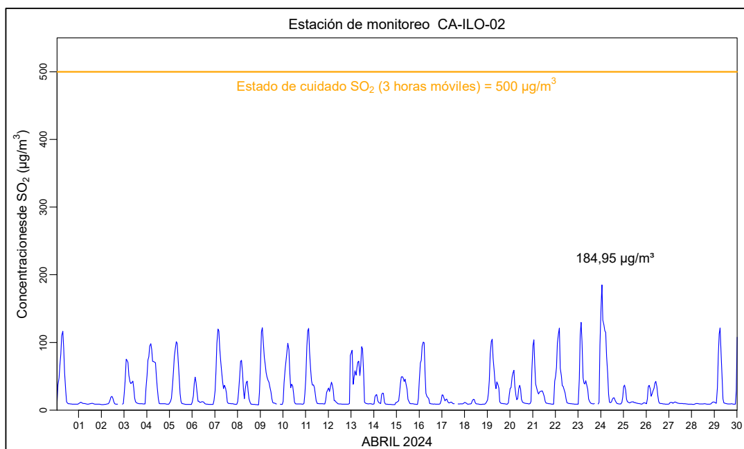
Figura 3.10.2. Concentraciones de promedio móvil de 3 horas de SO 2 en la estación de monitoreo CA-ILO-02, en abril de 2024
