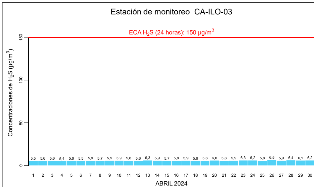
Figura 3.5.3. Concentraciones de 24 horas de H 2 S en la estación de monitoreo CA-ILO-03, abril de 2024.
