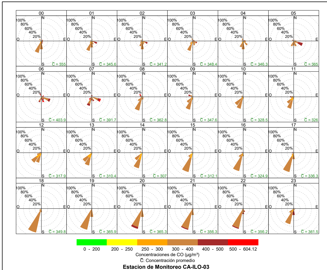
Figura 3.8.36. Rosa de concentración horaria del CO en la estación de monitoreo CA-ILO-03, abril de 2024
