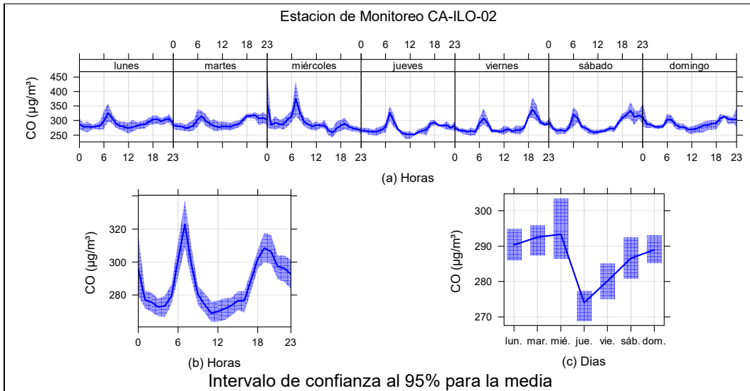
Figura 3.9.17. Concentraciones promedio horarias de CO en la estación de monitoreo CA-ILO-02, de abril de 2024
