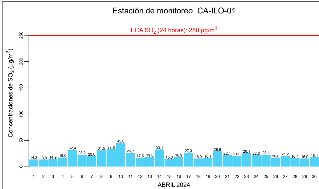
Figura 3.4.1. Concentraciones de 24 horas de SO 2 en la estación de monitoreo CA-ILO-01, abril de 2024
