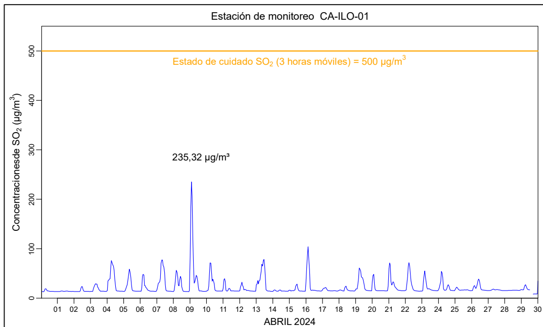
Figura 3.10.1. Concentraciones de promedio móvil de 3 horas de SO 2 en la estación de monitoreo CA-ILO-01, en abril de 2024
