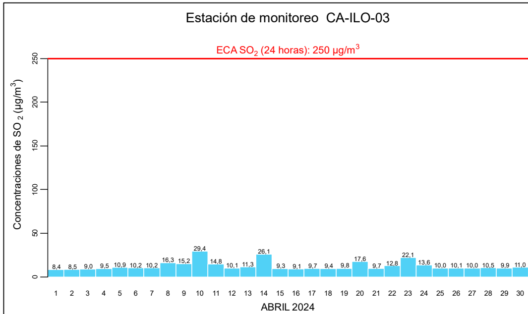
Figura 3.4.3. Concentraciones de 24 horas de SO 2 en la estación de monitoreo CA-ILO-03, abril de 2024.
