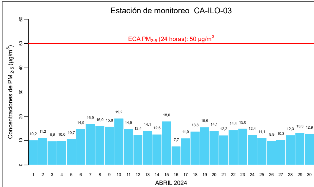
Figura 3.2.3. Concentraciones de 24 horas de PM 2,5 en la estación de monitoreo CA-ILO-03, abril de 2024
