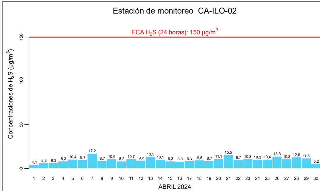
Figura 3.5.2. Concentraciones de 24 horas de H 2 S en la estación de monitoreo CA-ILO-02, abril de 2024
