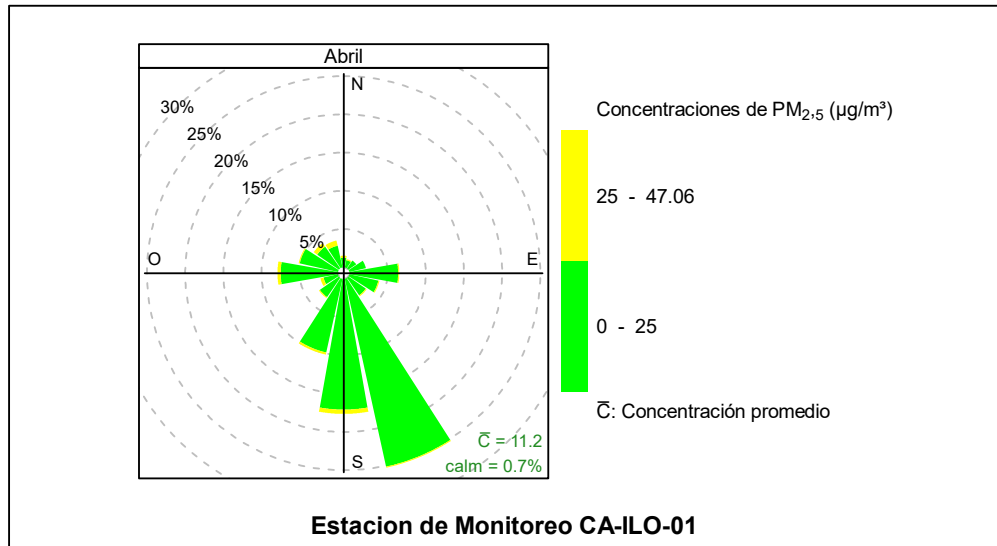
Figura 3.8.1. Rosa de concentración del PM 2,5 en la estación de monitoreo CA-ILO-01, abril del 2024
