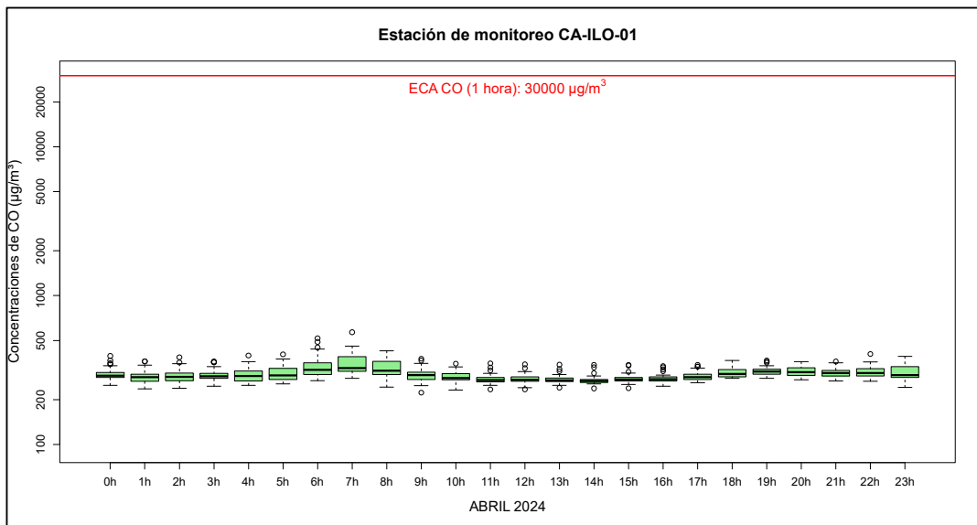
Figura 3.7.1. Concentraciones horarias de CO en la estación de monitoreo CA-ILO-01, abril de 2024
