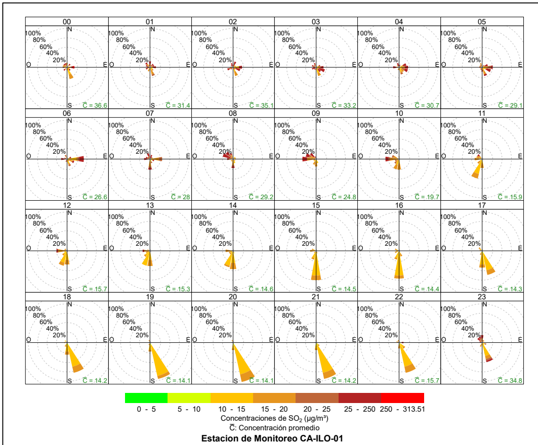
Figura 3.8.16. Rosa de concentración horaria del SO 2 en la estación de monitoreo CA-ILO-01, abril de 2024
