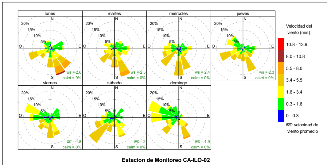
Figura 3.1.5. Rosa de viento por días de la semana de la estación de monitoreo CA-ILO-02, abril de 2024
