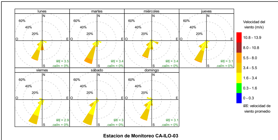
Figura 3.1.8. Rosa de viento por días de la semana de la estación de monitoreo CA-ILO-03, abril de 2024
