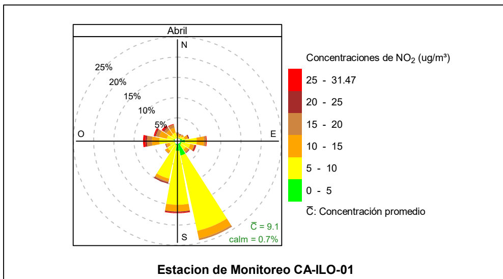
Figura 3.8.25. Rosa de concentración del NO 2 en la estación de monitoreo CA-ILO-01, abril de 2024
