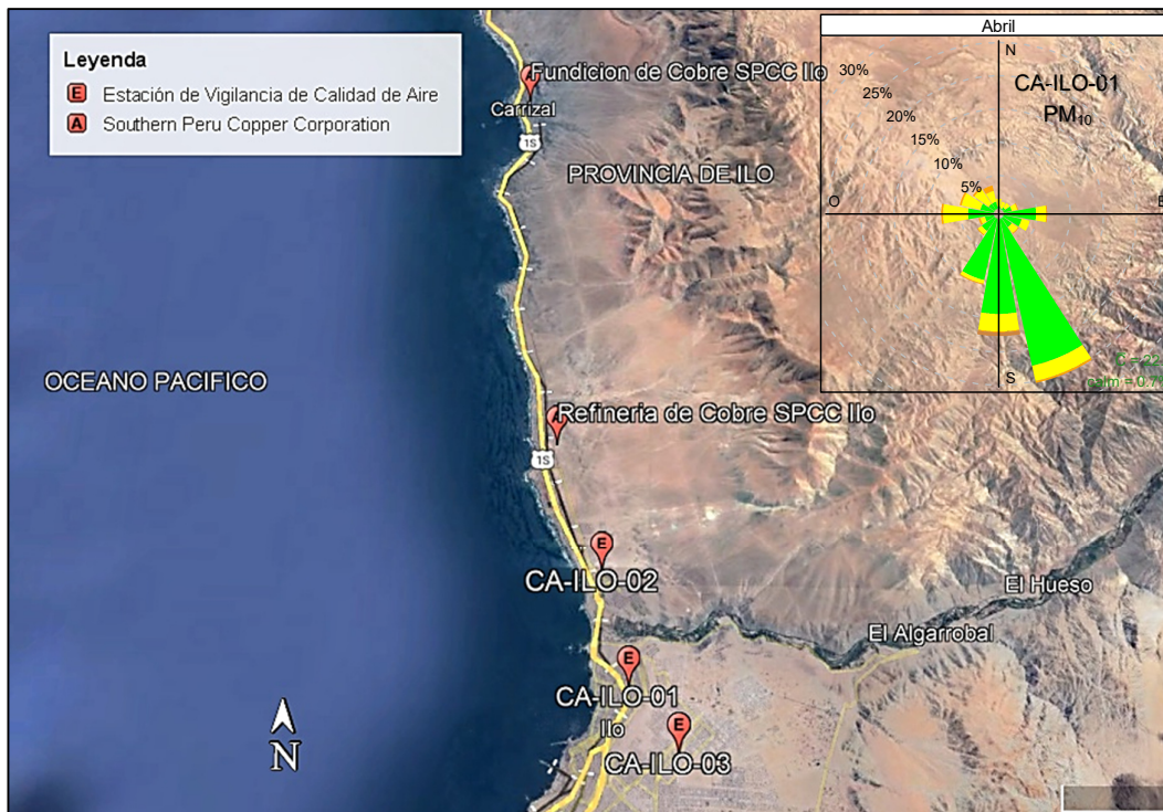
Figura 3.8.7.a. Ubicación de las estaciones de Vigilancia respecto al administrado Southern Peru Copper Corporation
