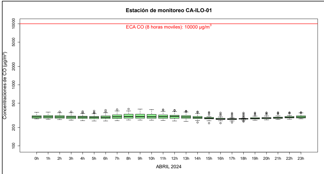
Figura 3.7.4. Concentraciones de promedio móvil de 8 horas de CO en la estación de monitoreo CA-ILO-01, abril de 2024
