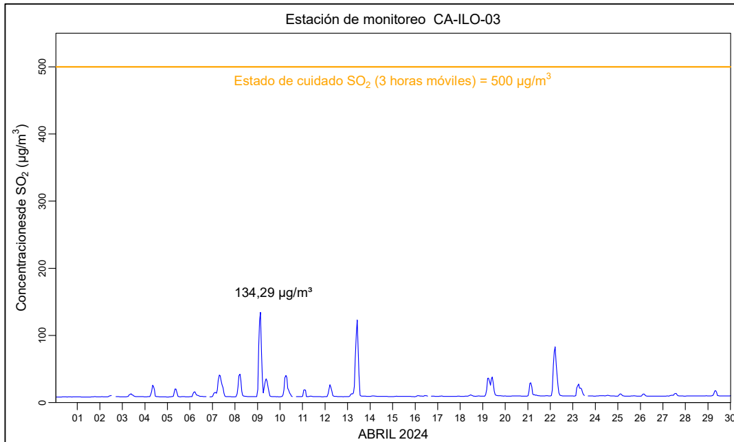
Figura 3.10.3. Concentraciones de promedio móvil de 3 horas de \text{SO}_2 en la estación de monitoreo CA-ILO-03, en abril de 2024
