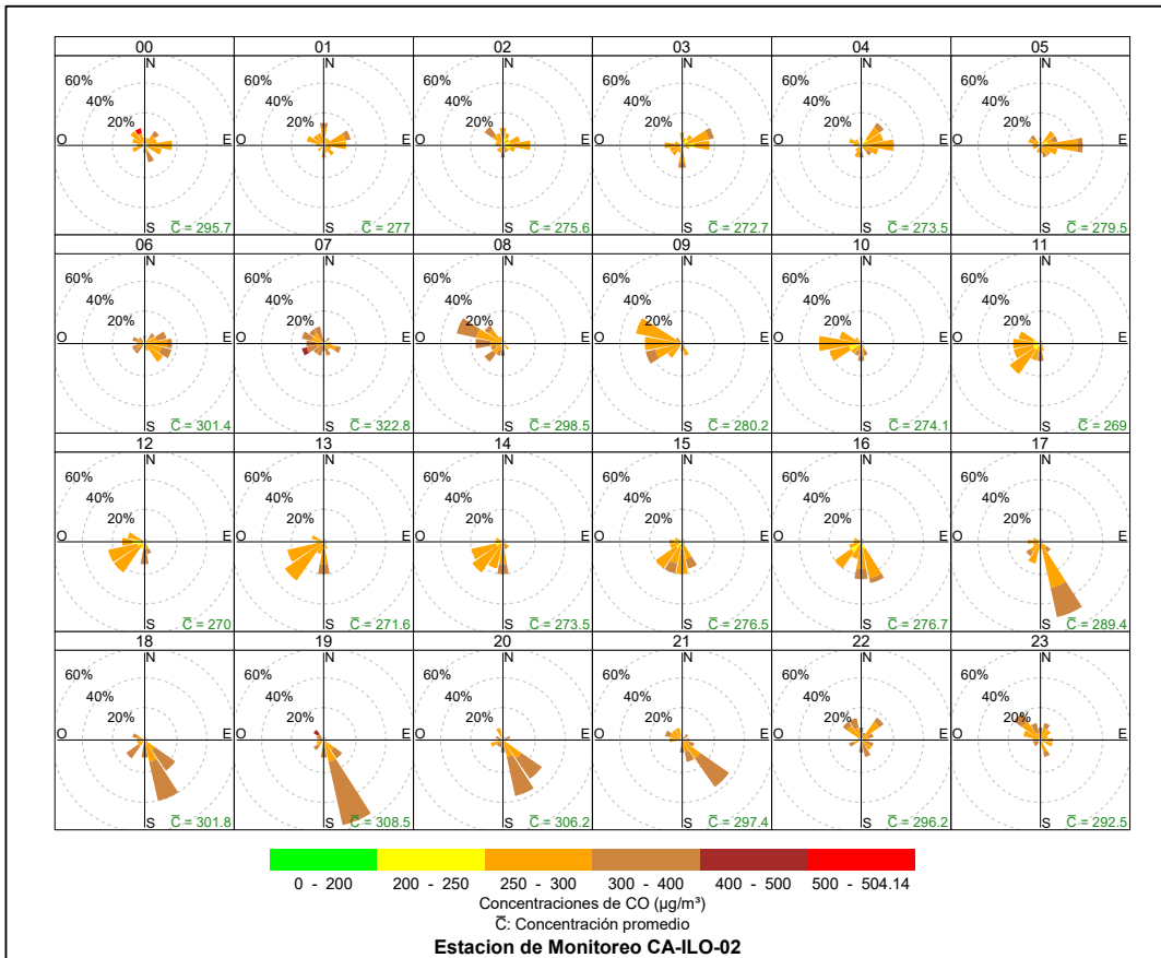
Figura 3.8.35. Rosa de concentración horaria del CO en la estación de monitoreo CA-ILO-02, abril de 2024
