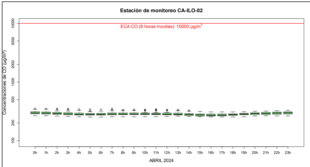
Figura 3.7.5. Concentraciones de promedio móvil de 8 horas de CO en la estación de monitoreo CA-ILO-02, abril de 2024
