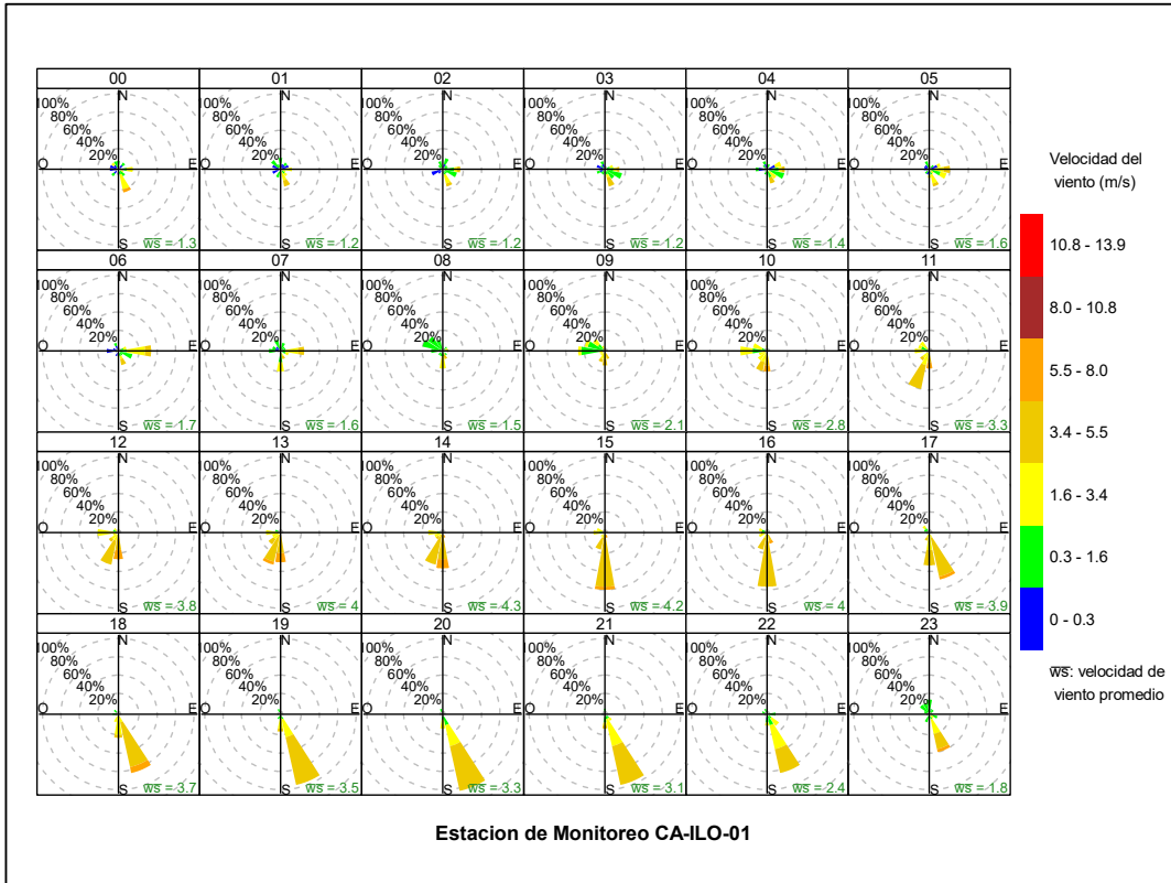
Figura 3.1.3. Rosa de viento horaria de la estación de monitoreo CA-ILO-01, abril de 2024
