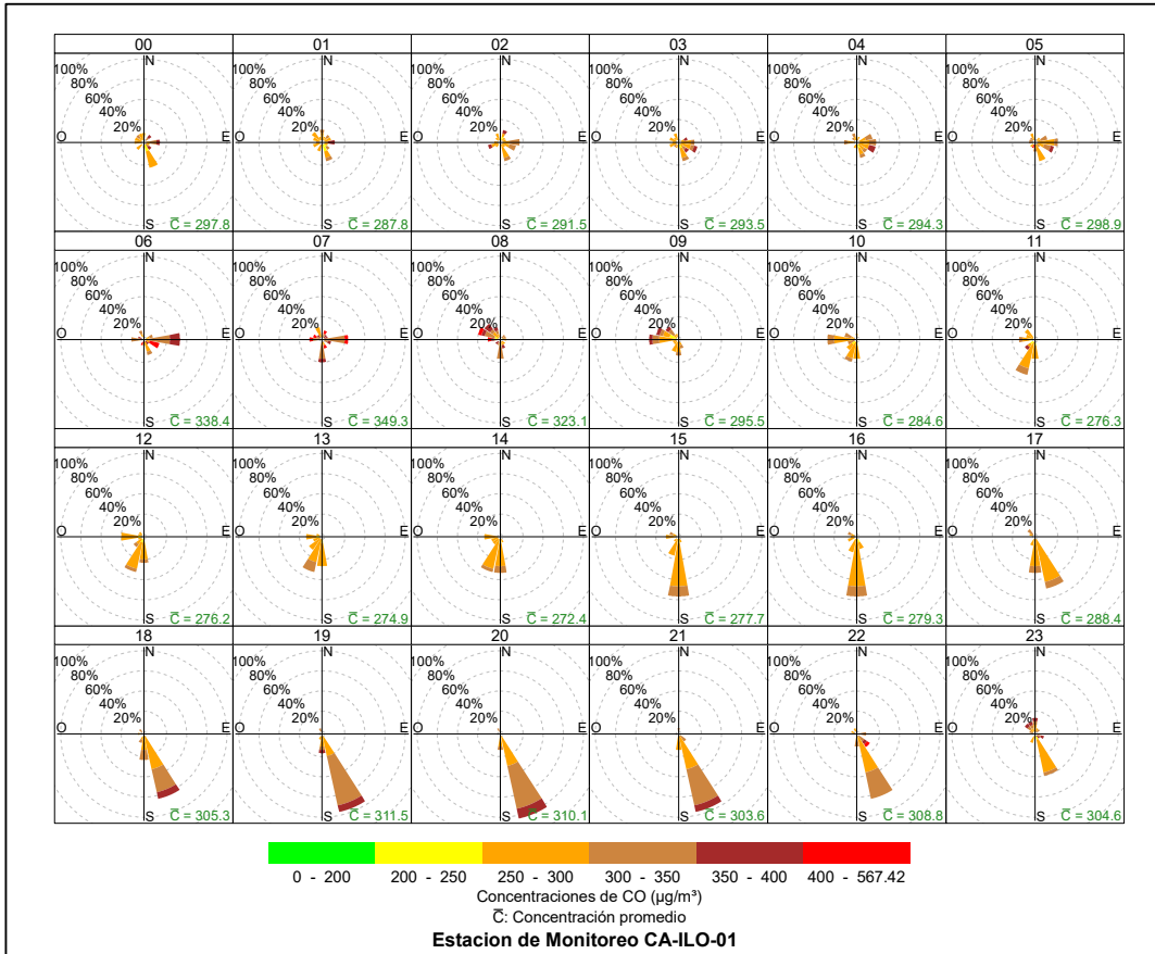
Figura 3.8.34. Rosa de concentración horaria del CO en la estación de monitoreo CA-ILO-01, abril de 2024
