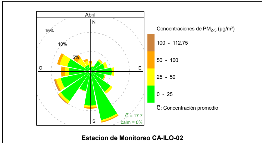
Figura 3.8.2. Rosa de concentración del PM_{2.5} en la estación de monitoreo CA-ILO-02, abril del 2024
