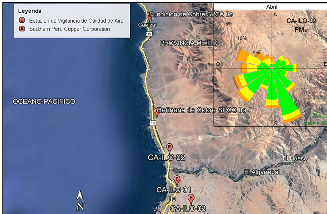
Figura 3.8.8.a. Ubicación de las estaciones de Vigilancia respecto al administrado Southern Peru Copper Corporation
