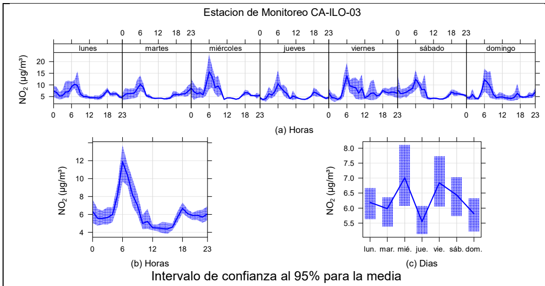
Figura 3.9.15. Concentraciones promedio horarias de \text{NO}_2 en la estación de monitoreo CA-ILO-03, de abril de 2024
