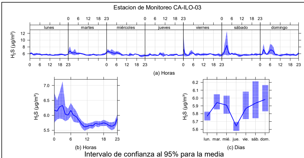
Figura 3.9.12. Concentraciones promedio horarias de H 2 S en la estación de monitoreo CA-ILO-03, de abril de 2024
