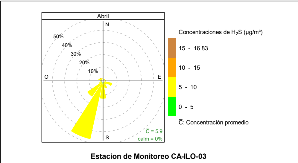
Figura 3.8.21. Rosa de concentración del H 2 S en la estación de monitoreo CA-ILO-03, abril de 2024
