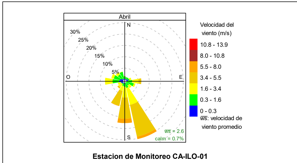
Figura 3.1.1. Rosa de viento de la estación de monitoreo CA-ILO-01, abril de 2024 2
