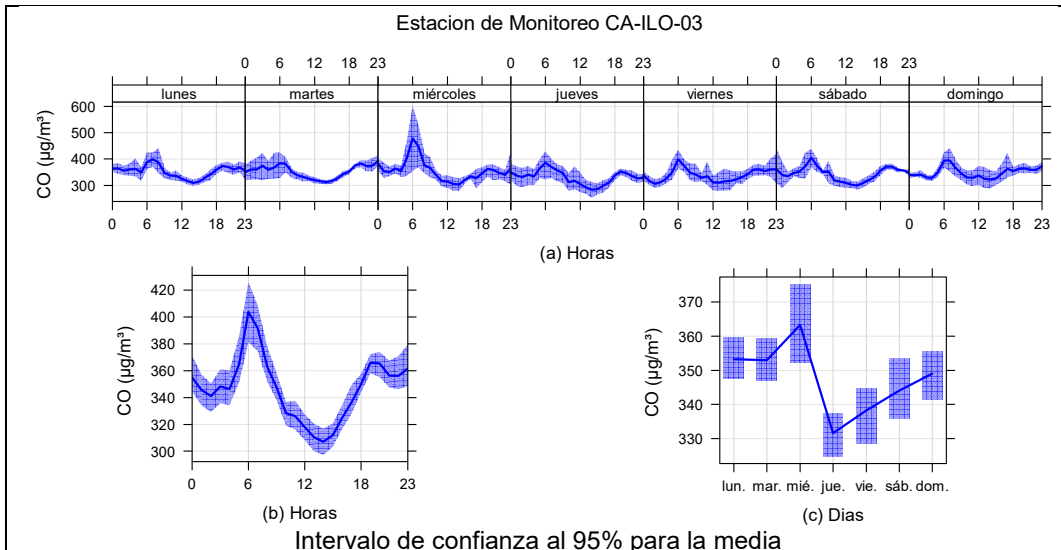
Figura 3.9.18. Concentraciones promedio horarias de CO en la estación de monitoreo CA-ILO-03, de abril de 2024
