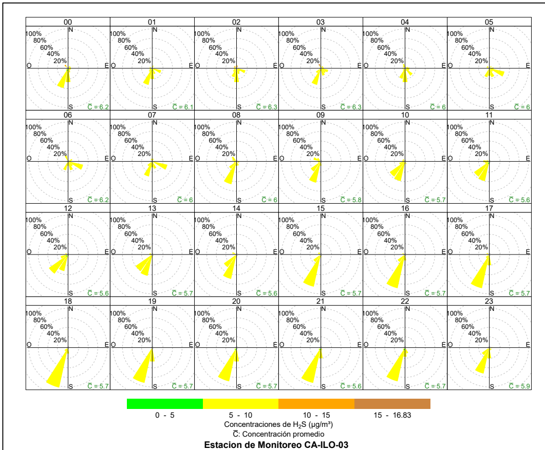
Figura 3.8.24. Rosa de concentración horaria del H 2 S en la estación de monitoreo CA-ILO-03, abril de 2024
