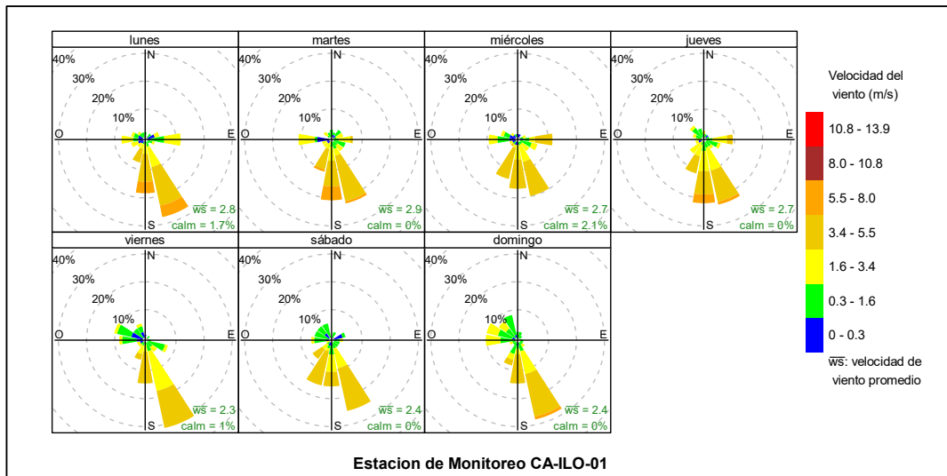
Figura 3.1.2. Rosa de viento por días de la semana de la estación de monitoreo CA-ILO-01, abril de 2024
