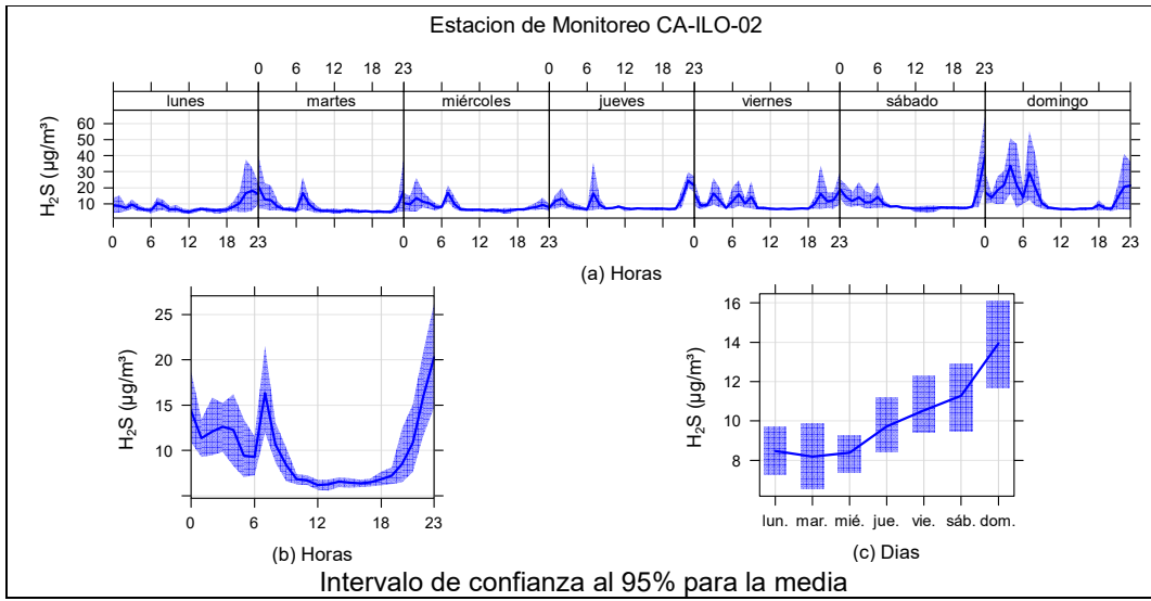
Figura 3.9.11. Concentraciones promedio horarias de H 2 S en la estación de monitoreo CA-ILO-02, de abril de 2024
