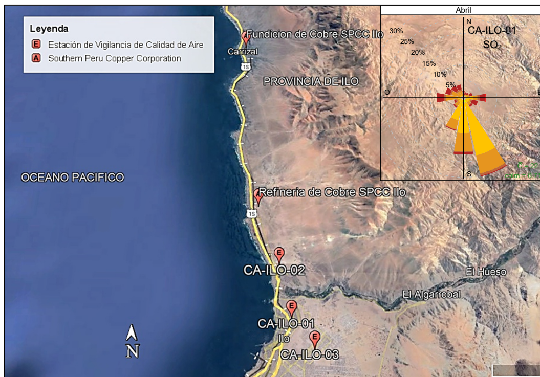
Figura 3.8.13. Rosa de concentración del SO 2 en la estación de monitoreo CA-ILO-01, abril de 2024
