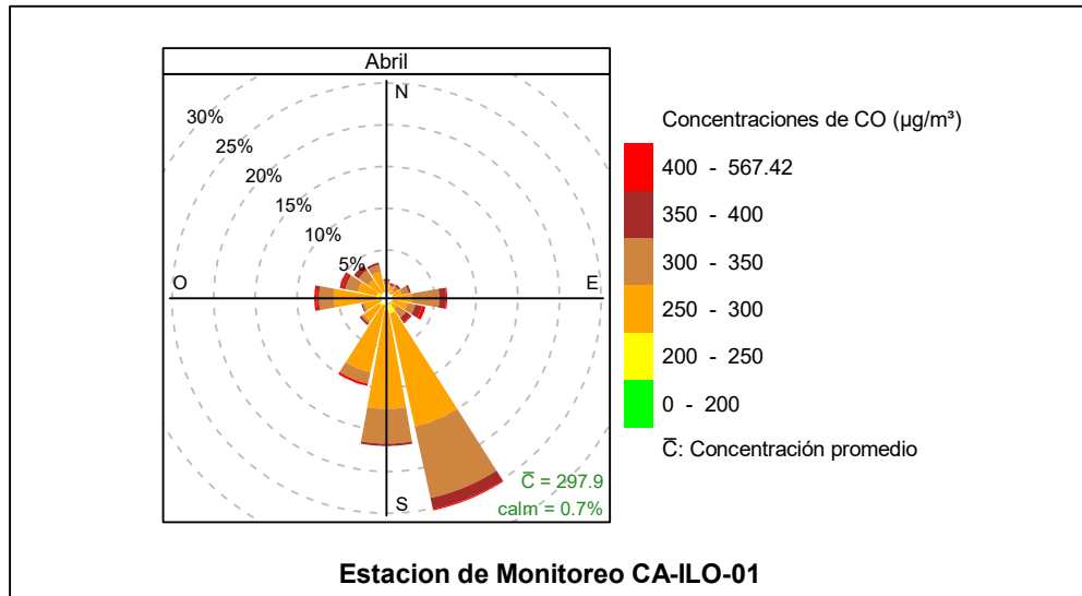
Figura 3.8.31. Rosa de concentración del CO en la estación de monitoreo CA-ILO-01, abril de 2024
