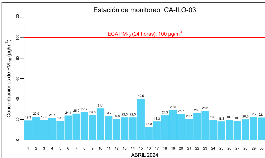
Figura 3.3.3. Concentraciones de 24 horas de PM 10 en la estación de monitoreo CA-ILO-03, abril de 2024
