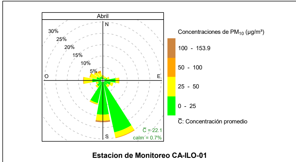
Figura 3.8.7. Rosa de concentración del PM 10 en la estación de monitoreo CA-ILO-01, abril de 2024
