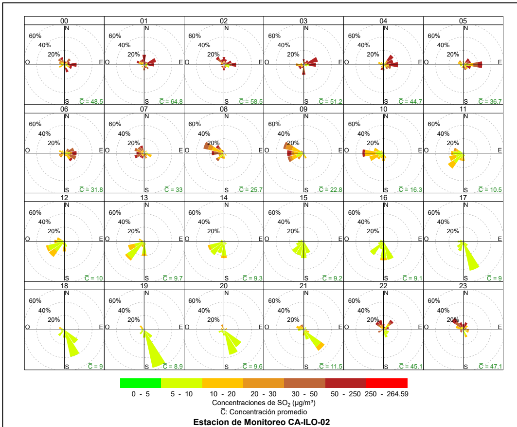
Figura 3.8.17. Rosa de concentración horaria del SO 2 en la estación de monitoreo CA-ILO-02, abril de 2024
