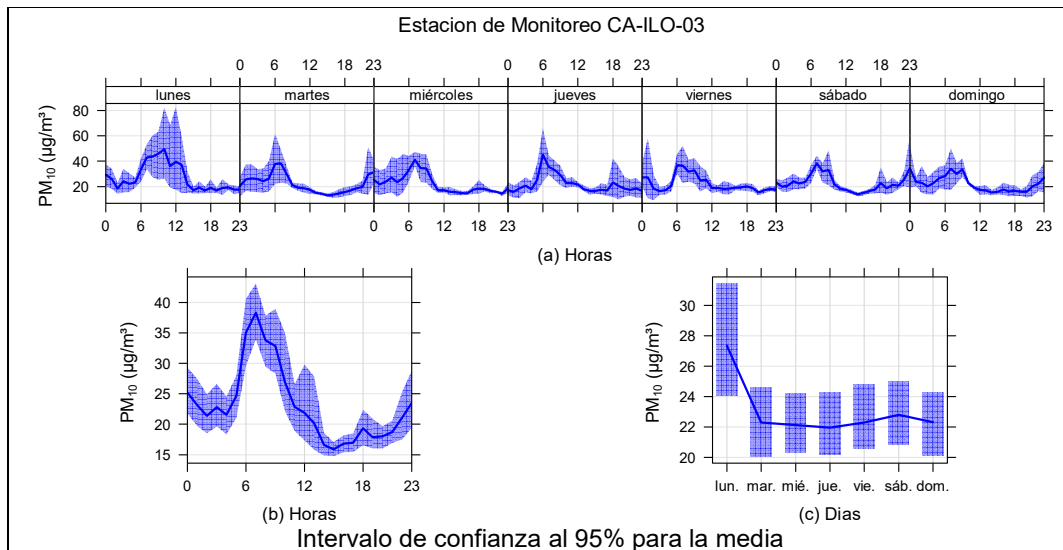
Figura 3.9.6. Concentraciones promedio horarias de PM_{10} en la estación de monitoreo CA-ILO-03, de abril de 2024
