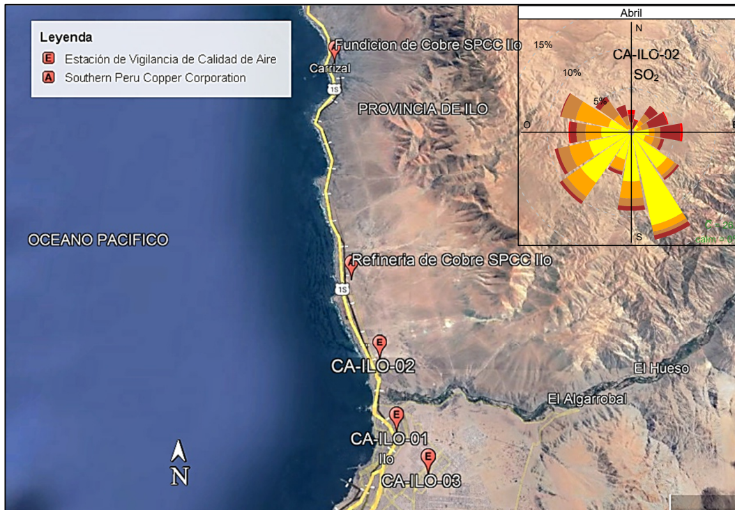
Figura 3.8.14.a. Ubicación de las estaciones de Vigilancia respecto al administrado Southern Peru Copper Corporation
