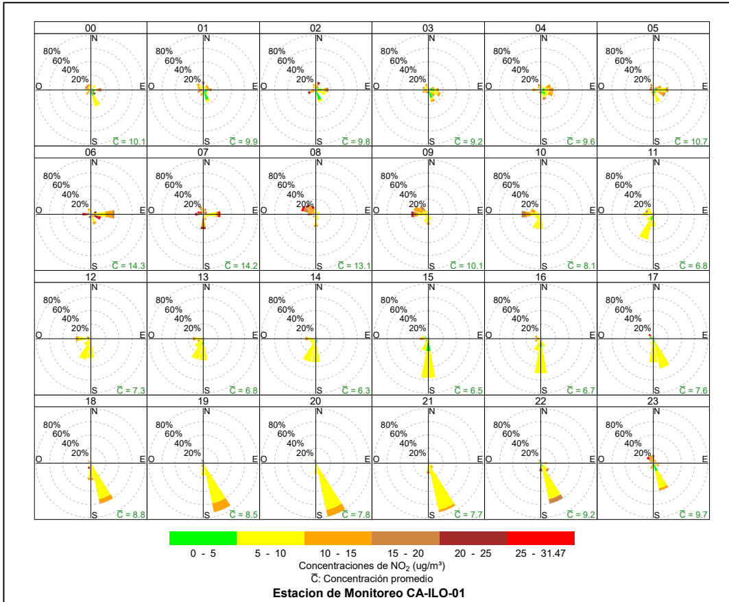
Figura 3.8.28. Rosa de concentración horaria del NO 2 en la estación de monitoreo CA-ILO-01, abril de 2024
