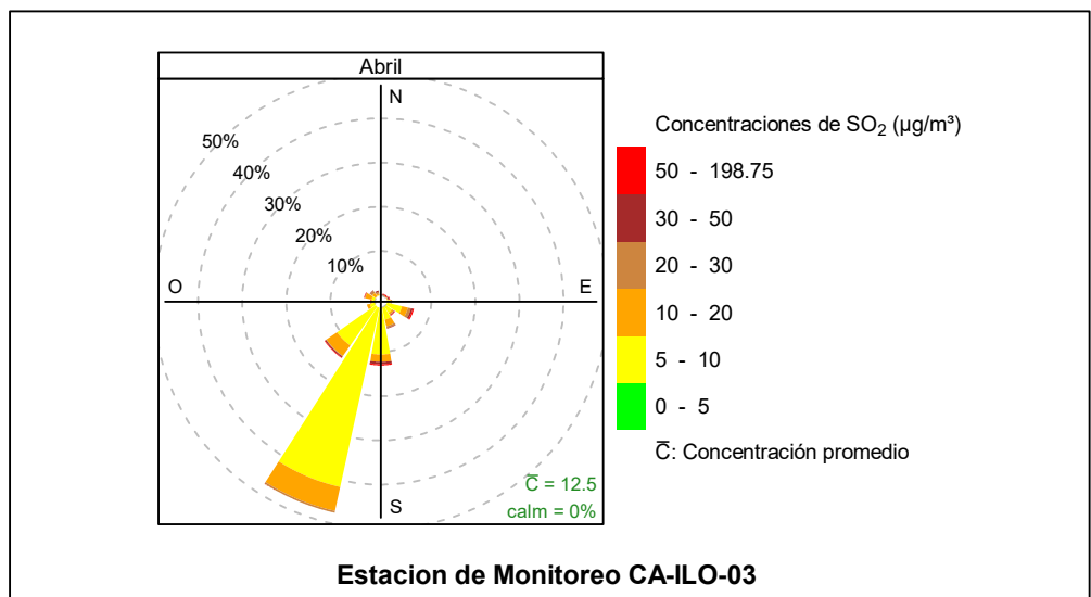
Figura 3.8.15. Rosa de concentración del \text{SO}_2 en la estación de monitoreo CA-ILO-03, abril de 2024
