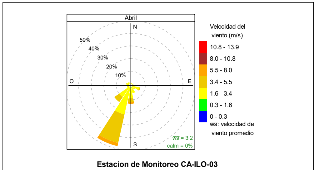
Figura 3.1.7. Rosa de viento de la estación de monitoreo CA-ILO-03, abril de 2024 6
