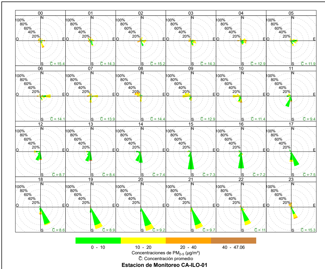
Figura 3.8.4. Rosa de concentración horaria del PM 2.5 en la estación de monitoreo CA-ILO-01, abril de 2024
