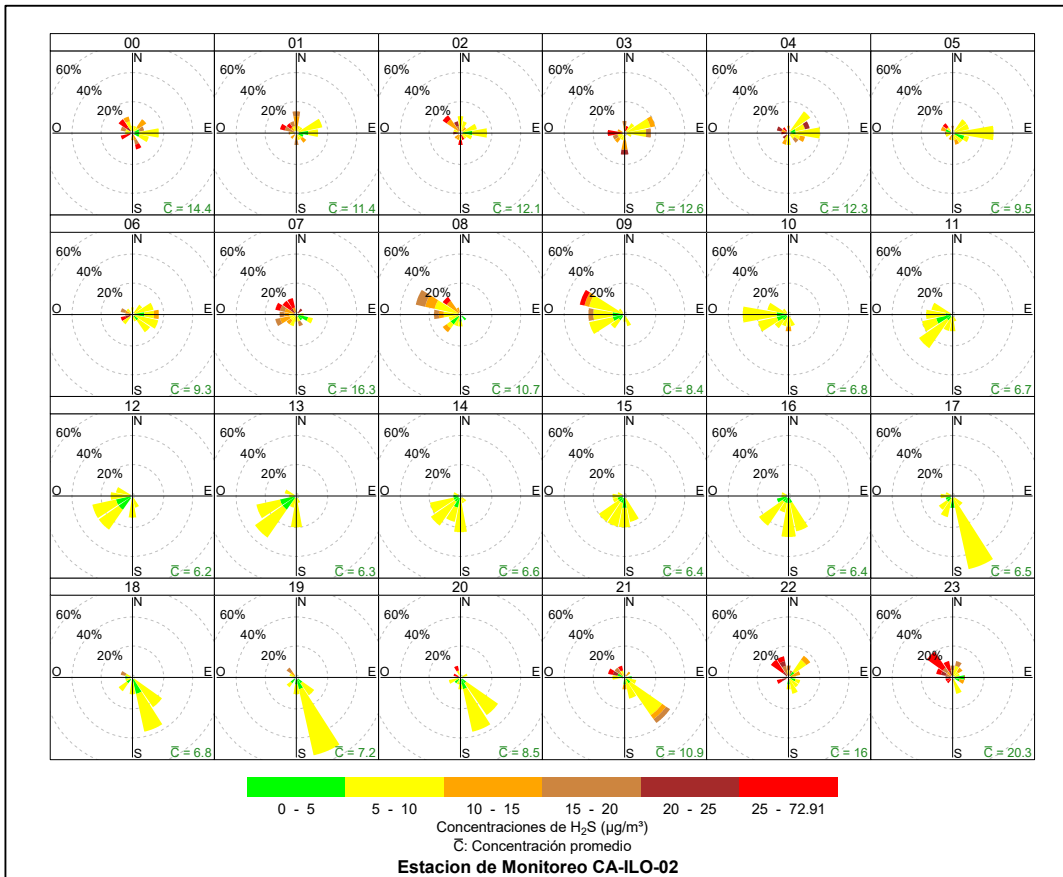
Figura 3.8.23. Rosa de concentración horaria del H 2 S en la estación de monitoreo CA-ILO-02, abril de 2024
