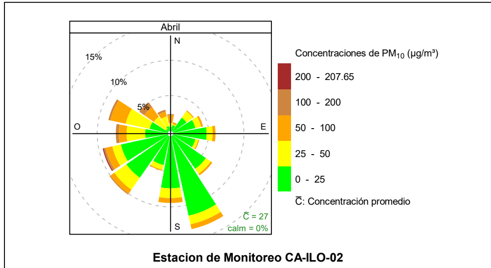
Figura 3.8.8. Rosa de concentración del \text{PM}_{10} en la estación de monitoreo CA-ILO-02, abril de 2024
