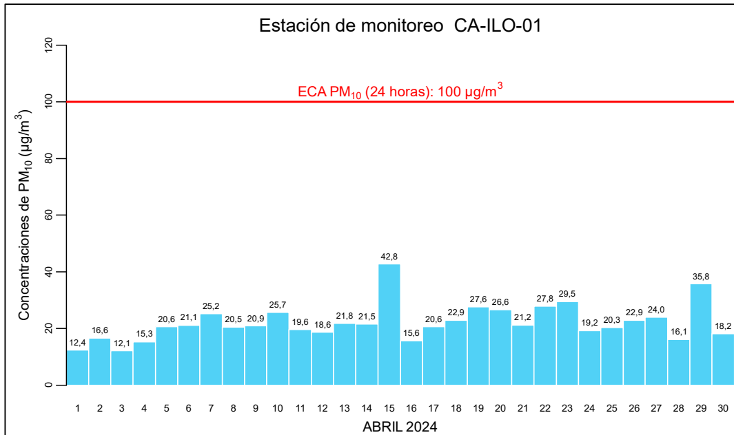
Figura 3.3.1. Concentraciones de 24 horas de PM 10 en la estación de monitoreo CA-ILO-01, abril de 2024
