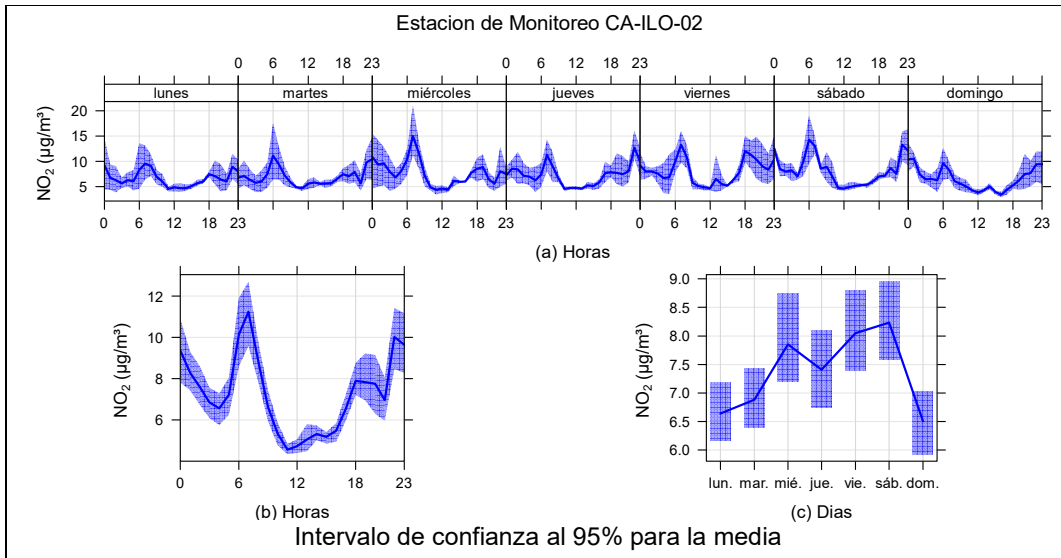
Figura 3.9.14. Concentraciones promedio horarias de \text{NO}_2 en la estación de monitoreo CA-ILO-02, de abril de 2024
