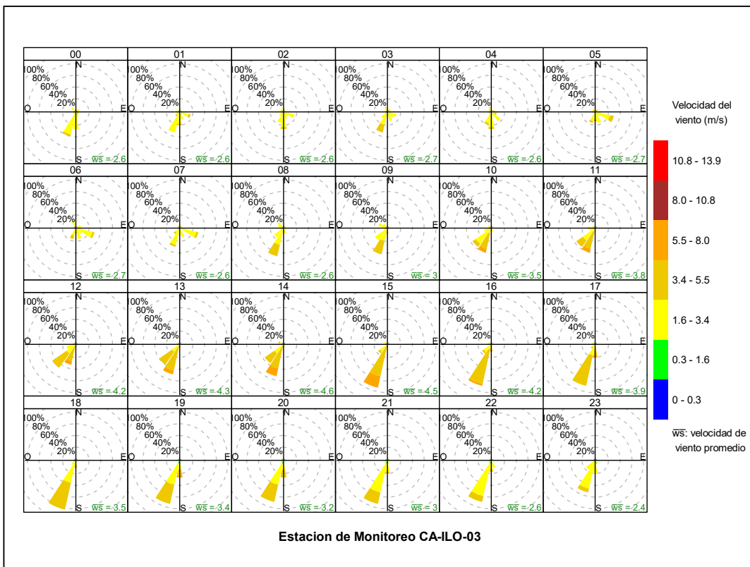
Figura 3.1.9. Rosa de viento horaria de la estación de monitoreo CA-ILO-03, abril de 2024
