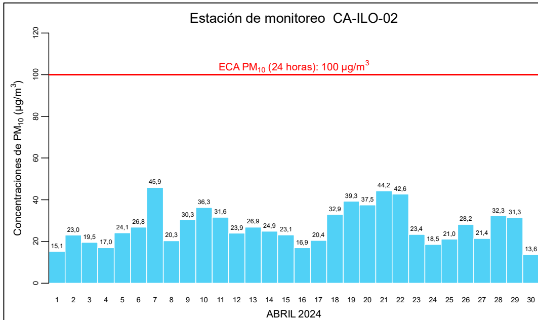
Figura 3.3.2. Concentraciones de 24 horas de PM 10 en la estación de monitoreo CA-ILO-02, abril de 2024
