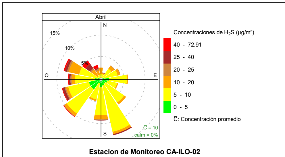
Figura 3.8.20. Rosa de concentración del H 2 S en la estación de monitoreo CA-ILO-02, abril de 2024
