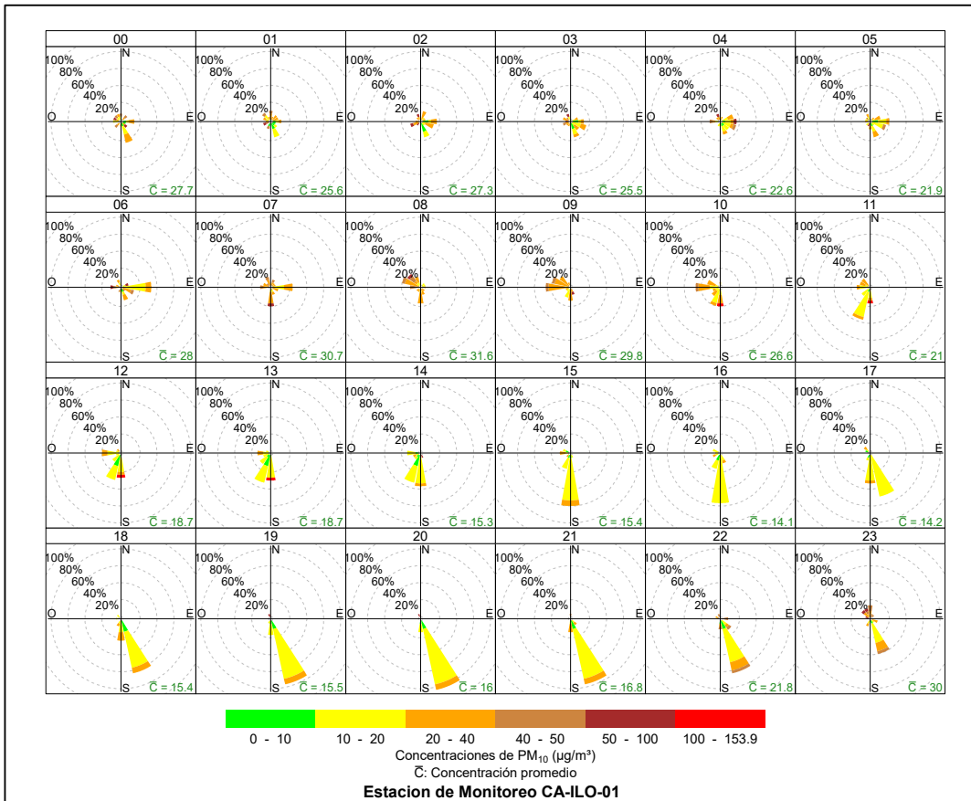
Figura 3.8.10. Rosa de concentración horaria del \text{PM}_{10} en la estación de monitoreo CA-ILO-01, abril de 2024
