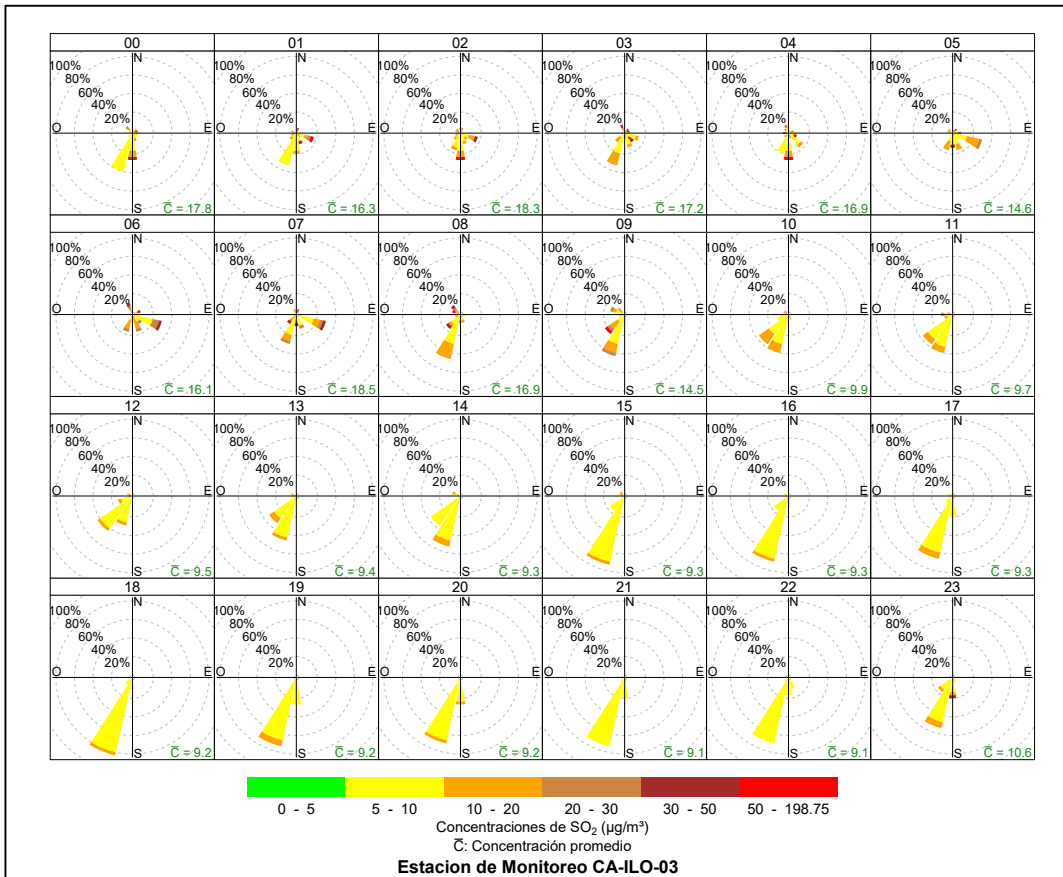
Figura 3.8.18. Rosa de concentración horaria del SO 2 en la estación de monitoreo CA-ILO-03, abril de 2024
