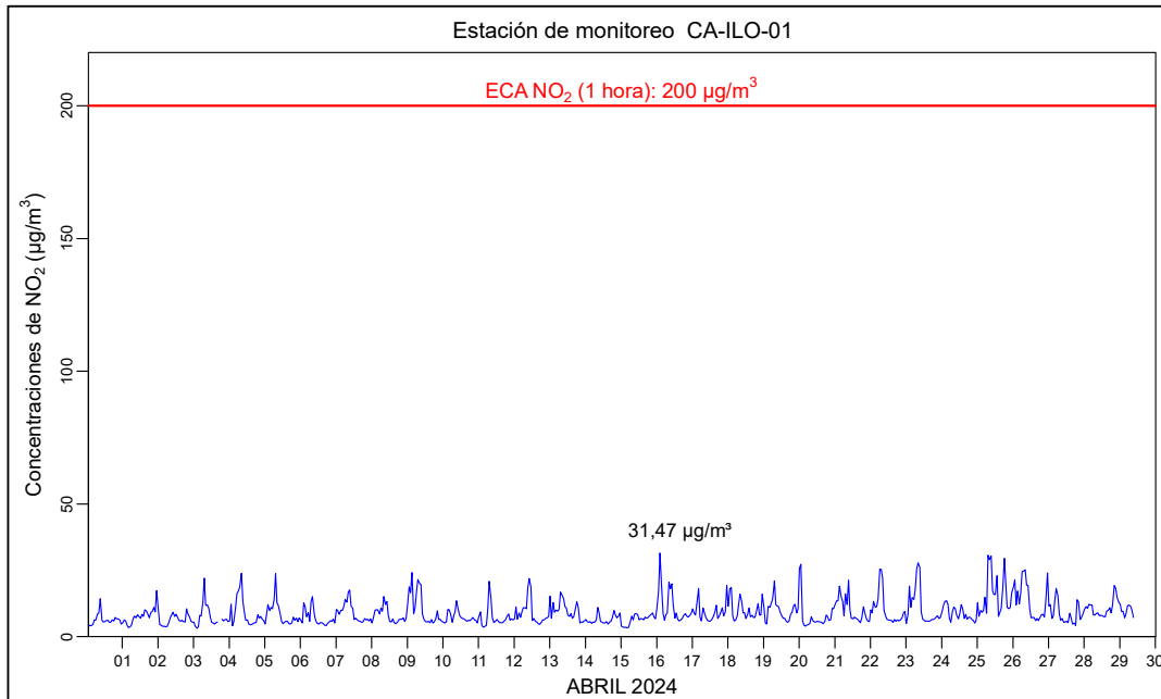
Figura 3.6.1. Concentraciones de horarias de NO 2 en la estación de monitoreo CA-ILO-01, abril de 2024.
