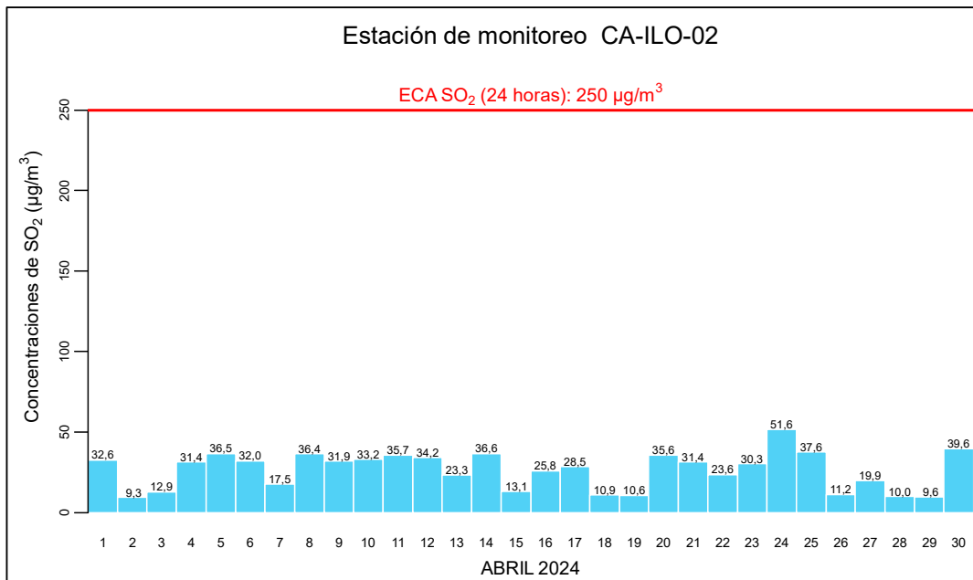
Figura 3.4.2. Concentraciones de 24 horas de SO 2 en la estación de monitoreo CA-ILO-02, abril de 2024
