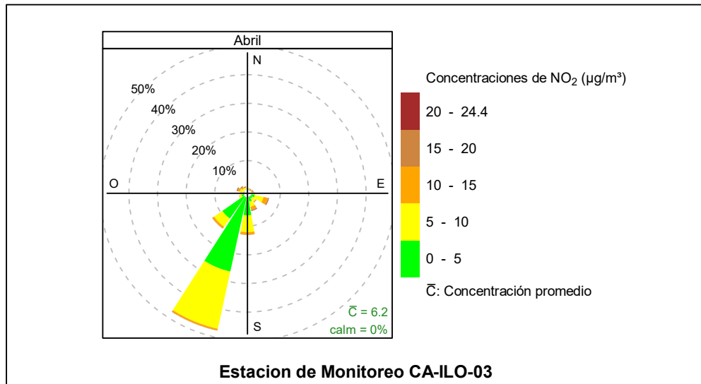
Figura 3.8.27. Rosa de concentración del NO 2 en la estación de monitoreo CA-ILO-03, abril de 2024
