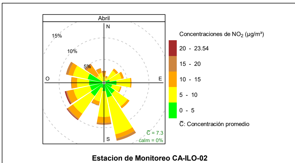
Figura 3.8.26. Rosa de concentración del NO 2 en la estación de monitoreo CA-ILO-02, abril de 2024
