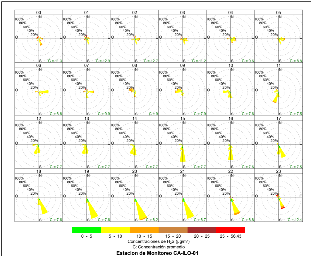
Figura 3.8.22. Rosa de concentración horaria del H 2 S en la estación de monitoreo CA-ILO-01, abril de 2024
