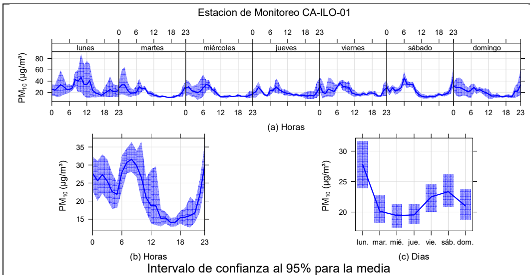
Figura 3.9.4. Concentraciones promedio horarios de PM_{10} en la estación de monitoreo CA-ILO-01, de abril de 2024
