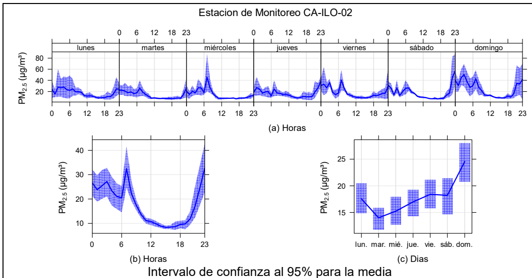
Figura 3.9.2. Concentraciones promedio horarias de PM_{2.5} en la estación de monitoreo CA-ILO-02, de abril de 2024
