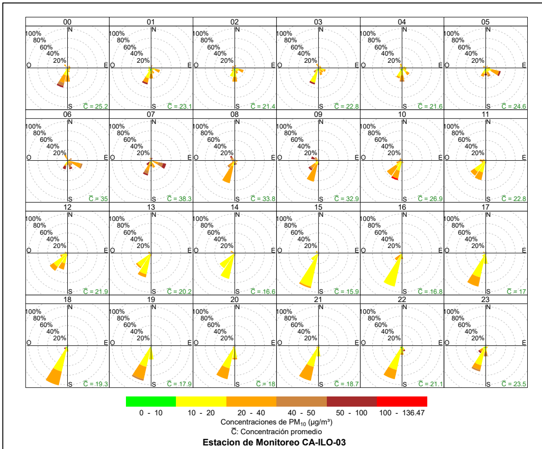
Figura 3.8.12. Rosa de concentración horaria del PM 10 en la estación de monitoreo CA-ILO-03, abril de 2024
