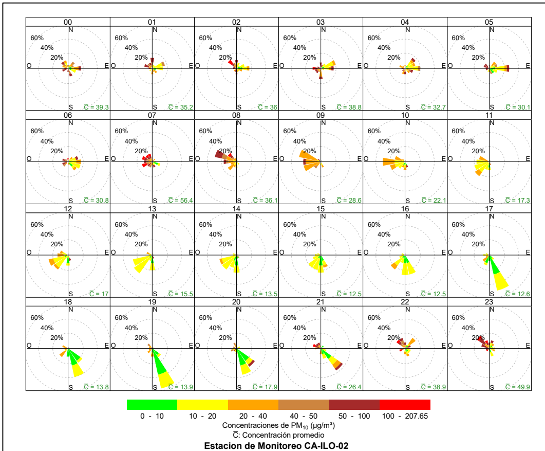
Figura 3.8.11. Rosa de concentración horaria del PM 10 en la estación de monitoreo CA-ILO-02, abril de 2024
