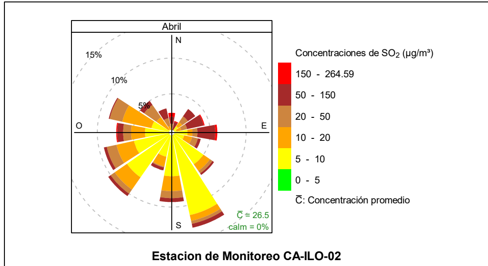
Figura 3.8.14. Rosa de concentración del \text{SO}_2 en la estación de monitoreo CA-ILO-02, abril de 2024
