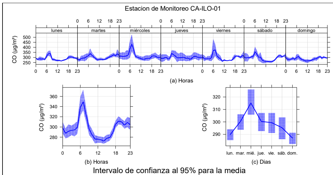
Figura 3.9.16. Concentraciones promedio horarias de CO en la estación de monitoreo CA-ILO-01, de abril de 2024
