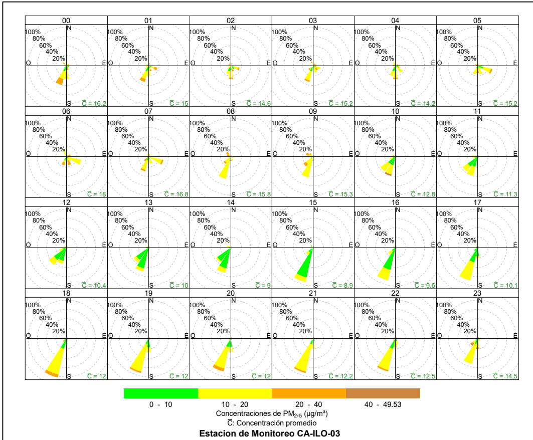
Figura 3.8.6. Rosa de concentración horaria del PM_{2.5} en la estación de monitoreo CA-ILO-03, abril de 2024
