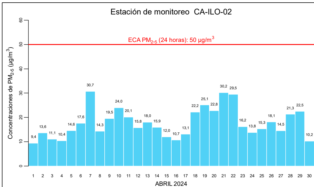
Figura 3.2.2. Concentraciones de 24 horas de PM 2,5 en la estación de monitoreo CA-ILO-02, abril de 2024
