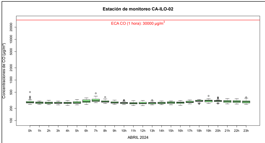
Figura 3.7.2. Concentraciones horarias de CO en la estación de monitoreo CA-ILO-02, abril de 2024
