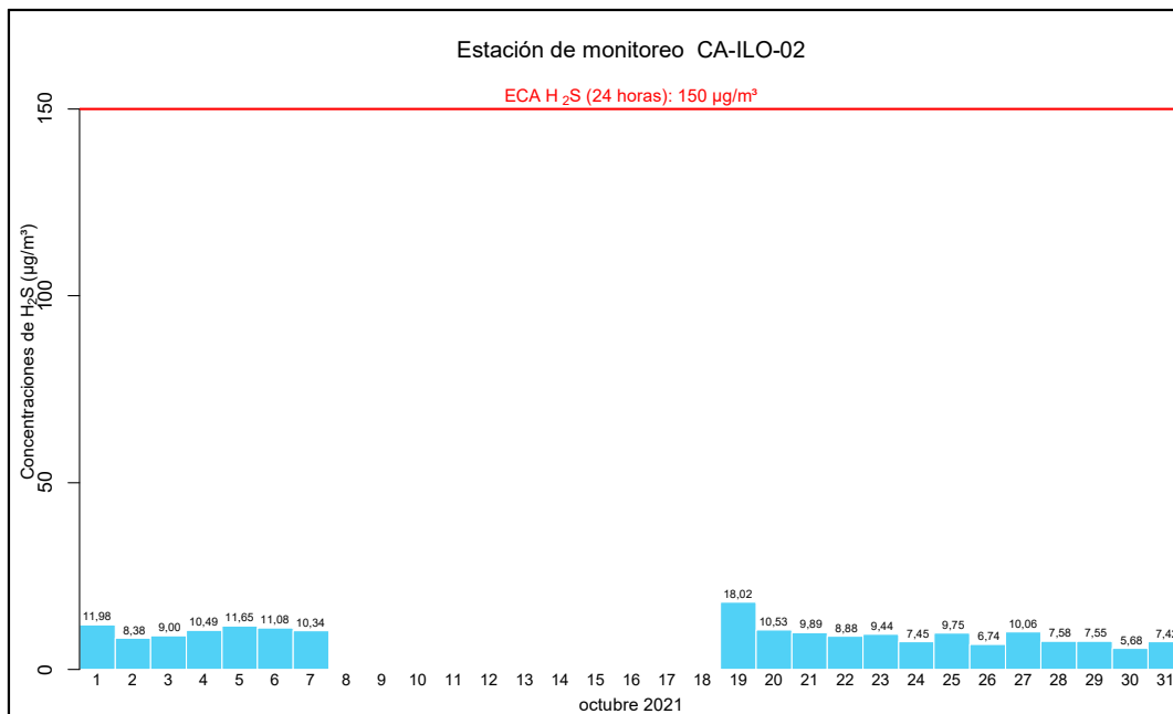
Figura 4.12. Concentraciones de 24 horas de H 2 S en la estación de monitoreo CA-ILO-02, en octubre de 2021 6
