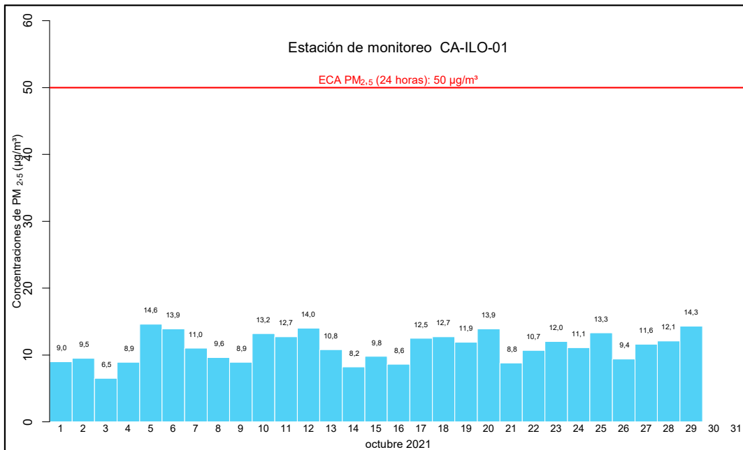
Figura 4.4. Concentraciones de 24 horas de PM 2,5 en la estación de monitoreo CA-ILO-01, en octubre de 2021 1
