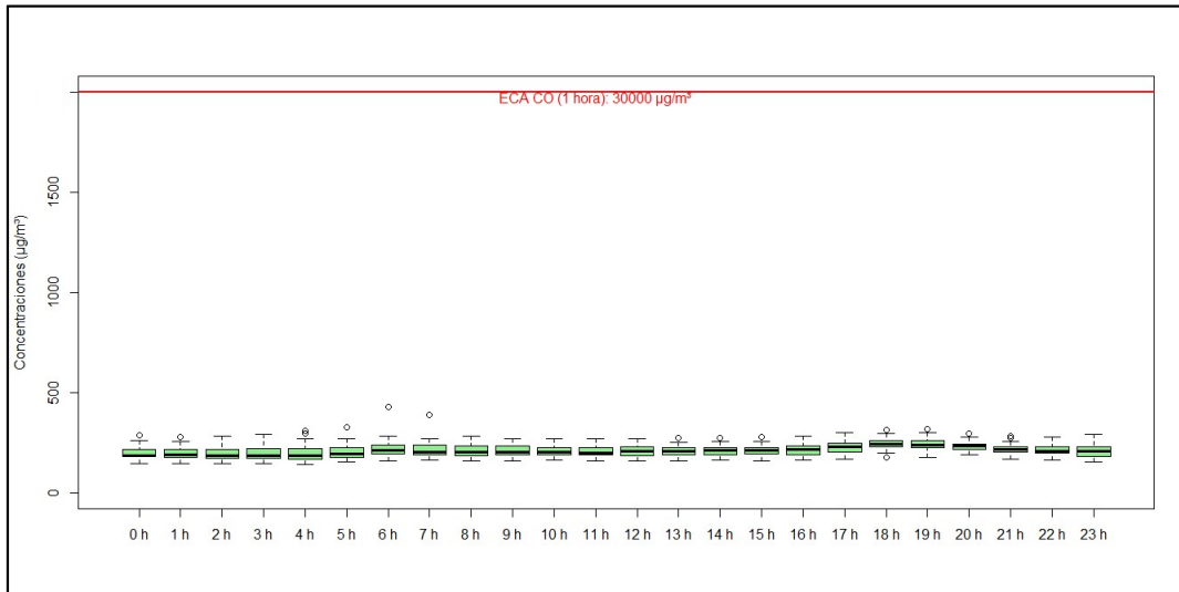
Figura 4.18. Concentraciones de horarias de CO en la estación de monitoreo CA-ILO-02, en octubre de 2021
