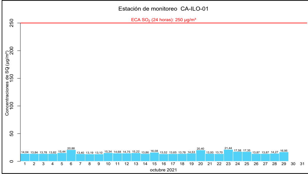
Figura 4.8. Concentraciones de 24 horas de SO 2 en la estación de monitoreo CA-ILO-01, en octubre de 2021 3
