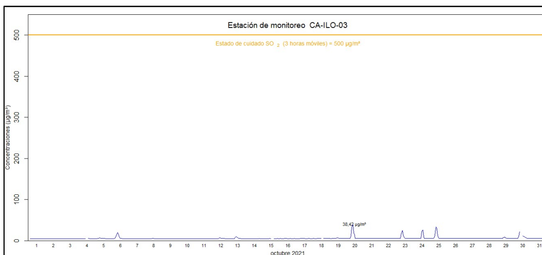
Figura 4.25. Concentraciones de promedio móvil de 3 horas de SO 2 en la estación de monitoreo CA-ILO-03, en octubre de 2021
