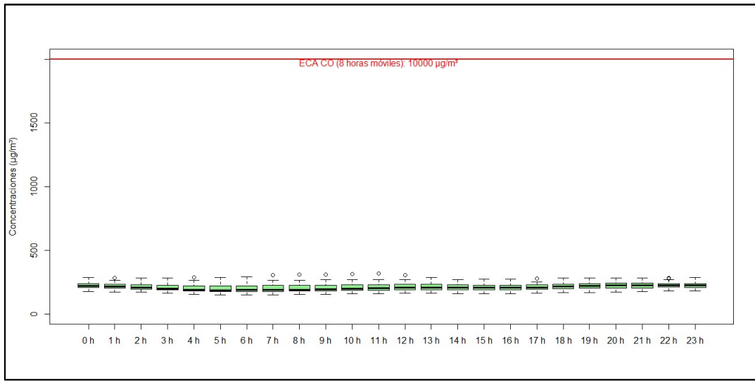
Figura 4.21. Concentraciones de promedio móvil de 8 horas de CO en la estación de monitoreo CA-ILO-02, en octubre de 2021
