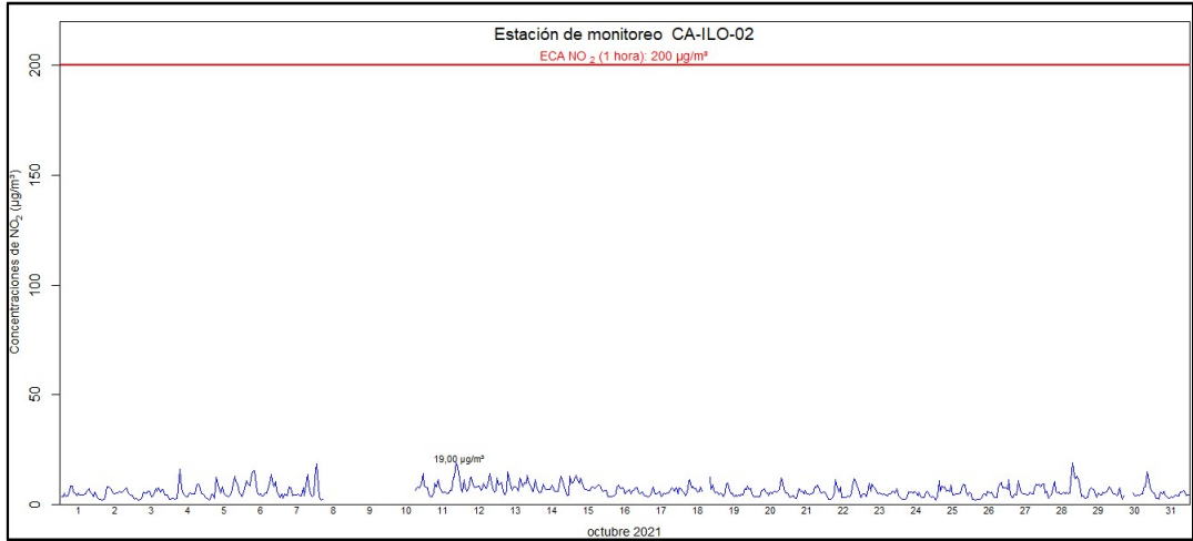
Figura 4.15. Concentraciones de horarias de NO 2 en la estación de monitoreo CA-ILO-02, en octubre de 2021 8
