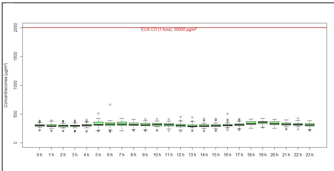
Figura 4.19. Concentraciones de horarias de CO en la estación de monitoreo CA-ILO-03, en octubre de 2021
