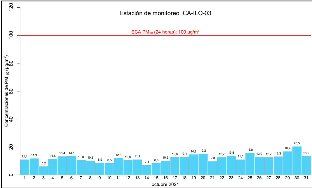
Figura 4.7. Concentraciones de 24 horas de PM 10 en la estación de monitoreo CA-ILO-03, en octubre de 2021
