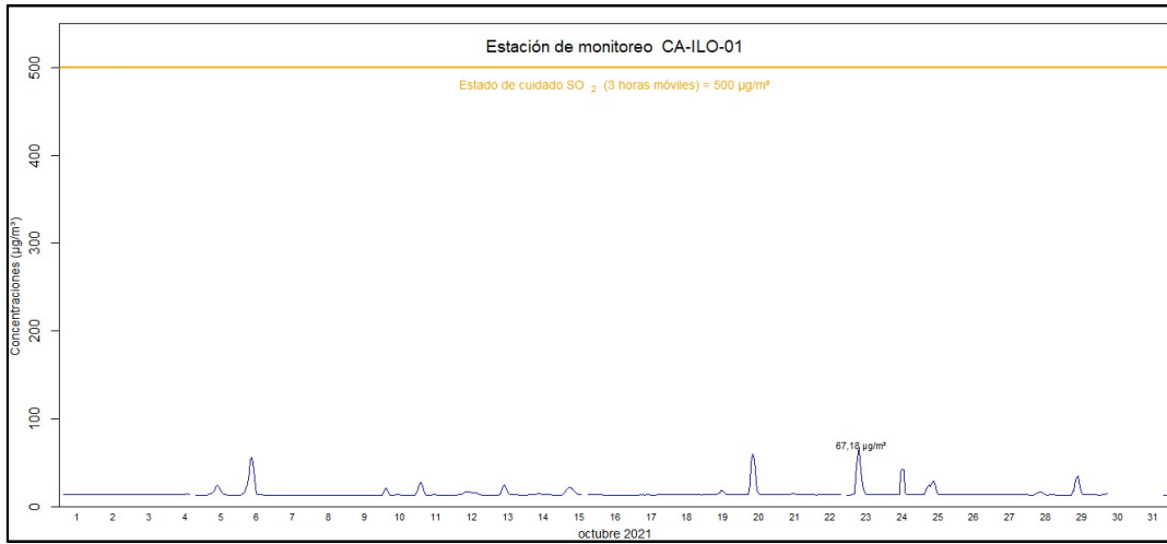
Figura 4.23. Concentraciones de promedio móvil de 3 horas de SO 2 en la estación de monitoreo CA-ILO-01, en octubre de 2021 10
