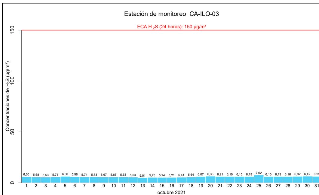
Figura 4.13. Concentraciones de 24 horas de H 2 S en la estación de monitoreo CA-ILO-03, en octubre de 2021
