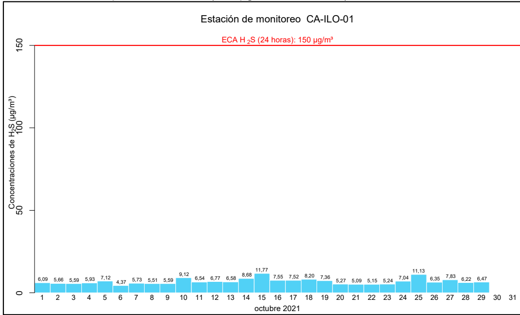
Figura 4.11. Concentraciones de 24 horas de H 2 S en la estación de monitoreo CA-ILO-01, en octubre de 2021 5
