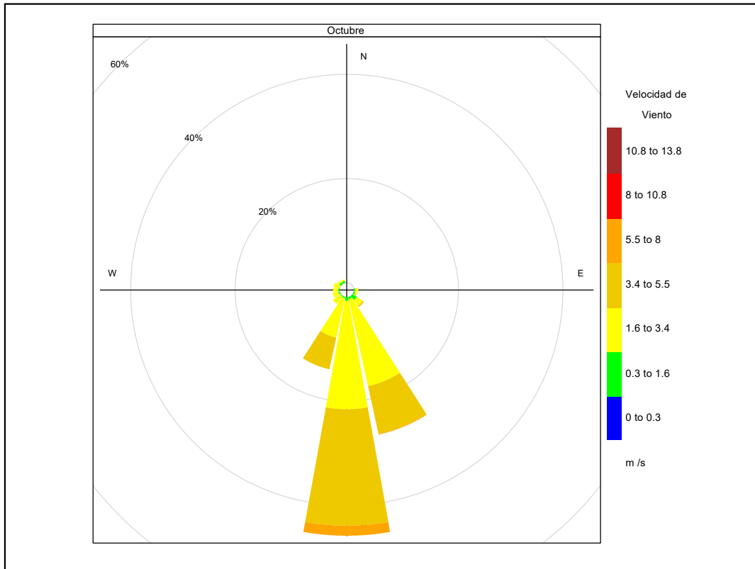
Figura 4.3. Rosa de viento de la estación de monitoreo CA-ILO-03, en octubre de 2021
