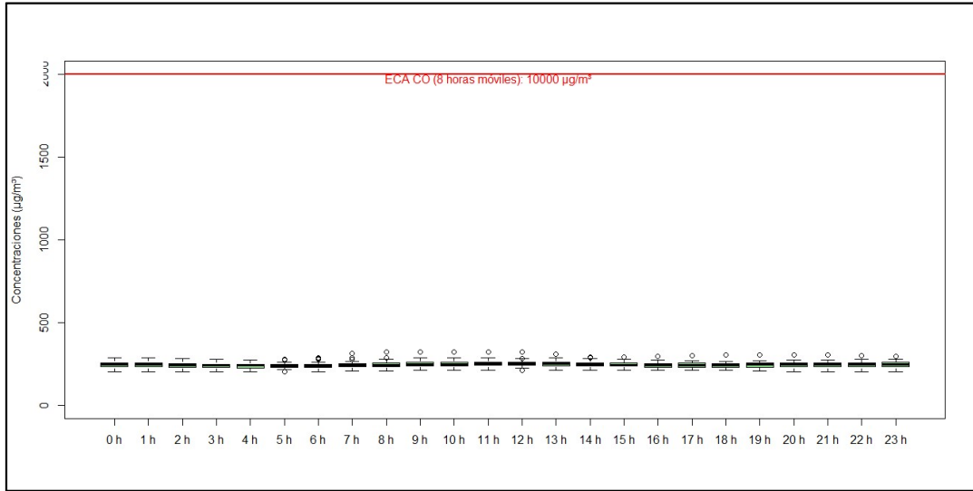
Figura 4.20. Concentraciones de promedio móvil de 8 horas de CO en la estación de monitoreo CA-ILO-01, en octubre de 2021
