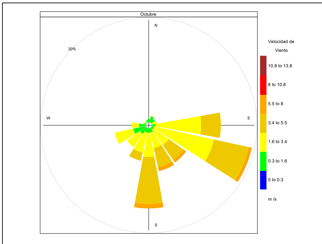
Figura 4.2. Rosa de viento de la estación de monitoreo CA-ILO-02, en octubre de 2021
