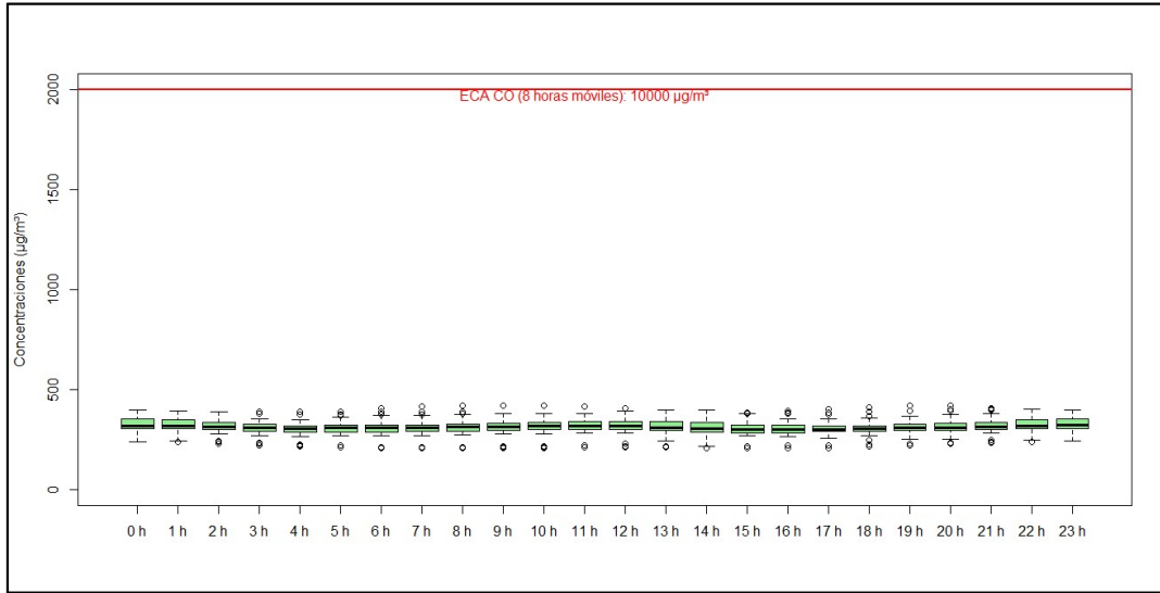
Figura 4.22. Concentraciones de promedio móvil de 8 horas de CO en la estación de monitoreo CA-ILO-03, en octubre de 2021
