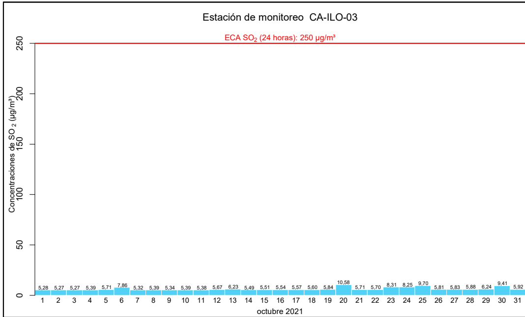
Figura 4.10. Concentraciones de 24 horas de SO 2 en la estación de monitoreo CA-ILO-03, en octubre de 2021
