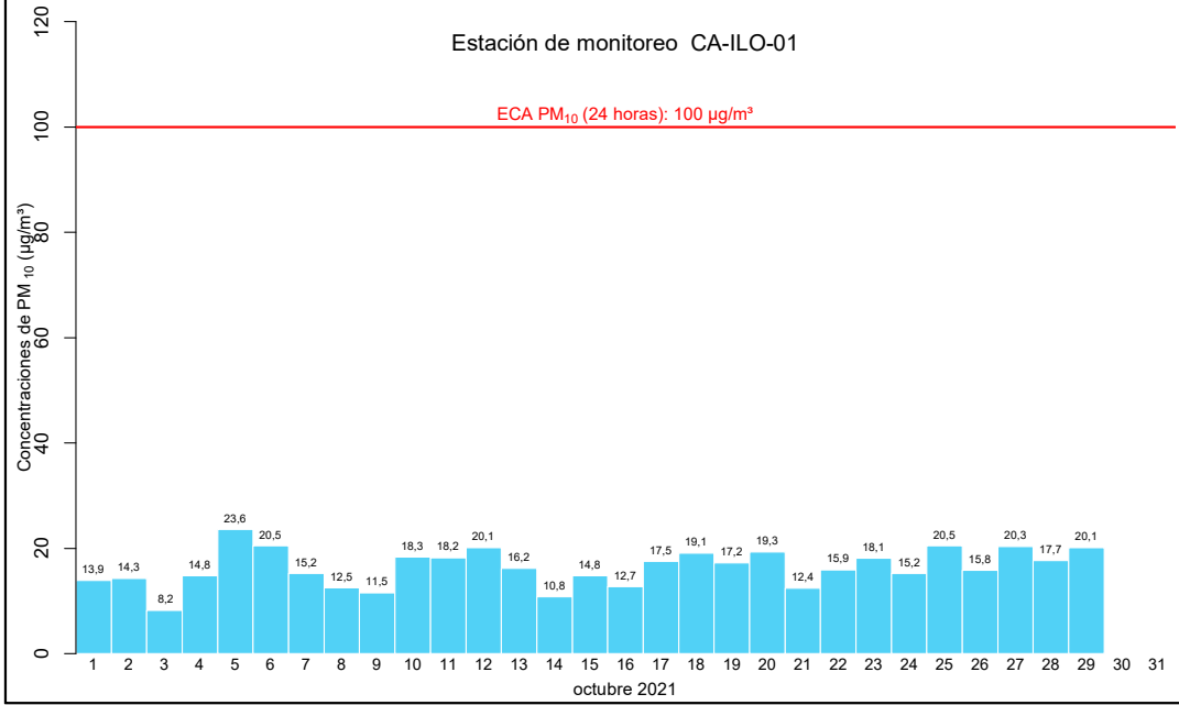
Figura 4.6. Concentraciones de 24 horas de PM 10 en la estación de monitoreo CA-ILO-01, en octubre de 2021 2
