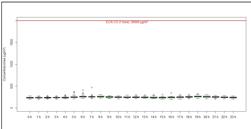
Figura 4.17. Concentraciones de horarias de CO en la estación de monitoreo CA-ILO-01, en octubre de 2021
