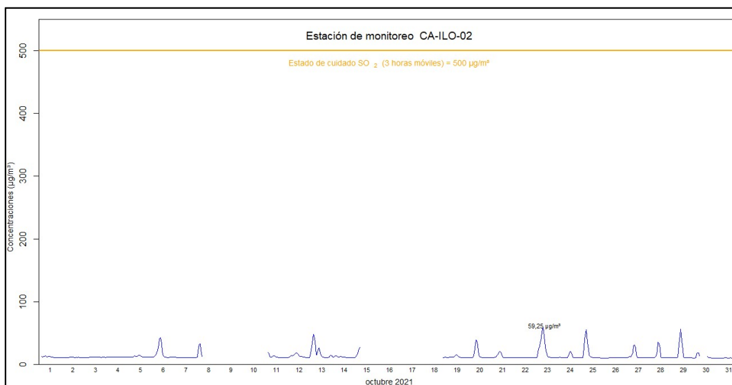
Figura 4.24. Concentraciones de promedio móvil de 3 horas de SO 2 en la estación de monitoreo CA-ILO-02, en octubre de 2021 11
