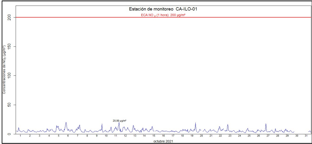
Figura 4.14. Concentraciones de horarias de NO 2 en la estación de monitoreo CA-ILO-01, en octubre de 2021 7
