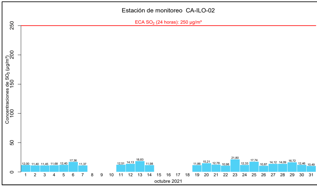
Figura 4.9. Concentraciones de 24 horas de SO 2 en la estación de monitoreo CA-ILO-02, en octubre de 2021 4
