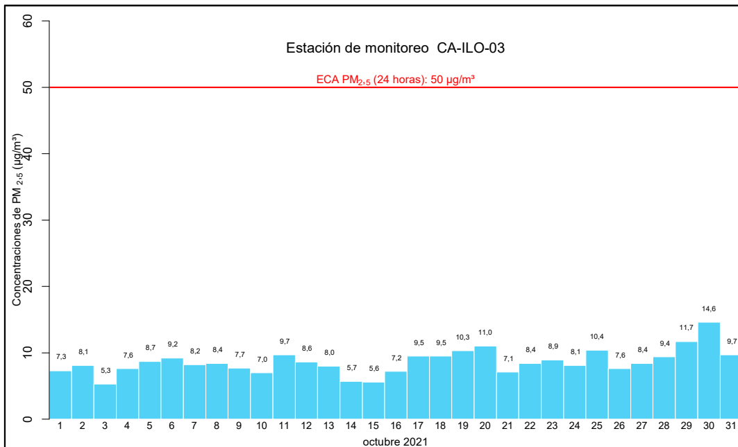
Figura 4.5. Concentraciones de 24 horas de PM 2,5 en la estación de monitoreo CA-ILO-03, en octubre de 2021
