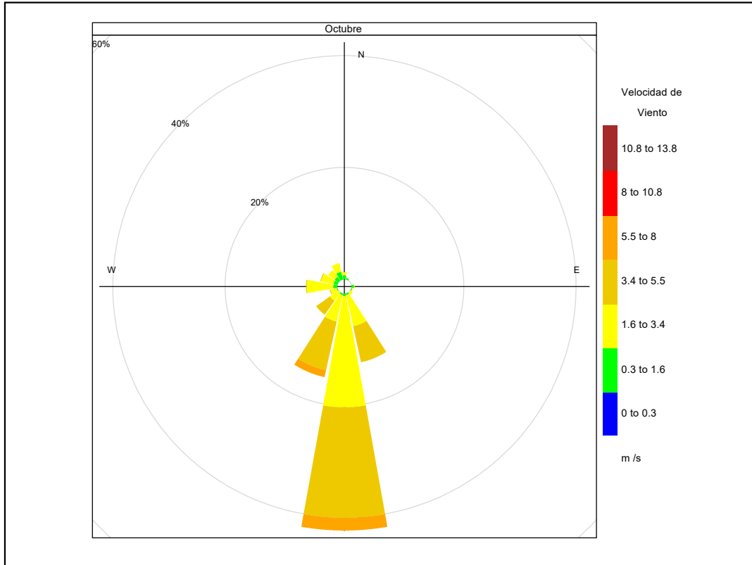
Figura 4.1. Rosa de viento de la estación de monitoreo CA-ILO-01, en octubre de 2021
