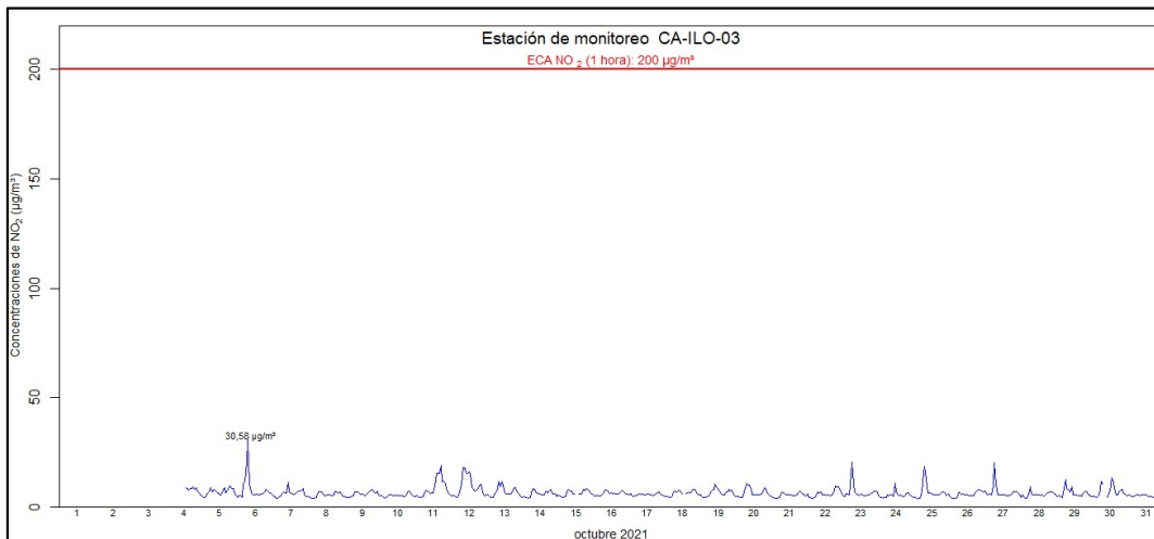
Figura 4.16. Concentraciones de horarias de NO 2 en la estación de monitoreo CA-ILO-03, en octubre de 2021 9
