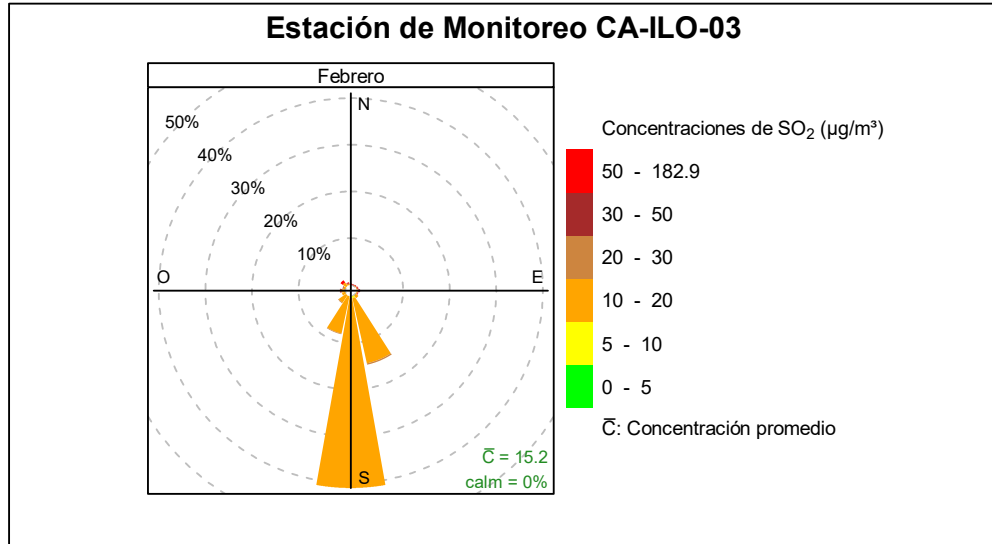
Figura 3.8.10. Rosa de concentración del SO 2 en la estación de monitoreo Ilo - José Pardo (CA-ILO-03), febrero de 2025
