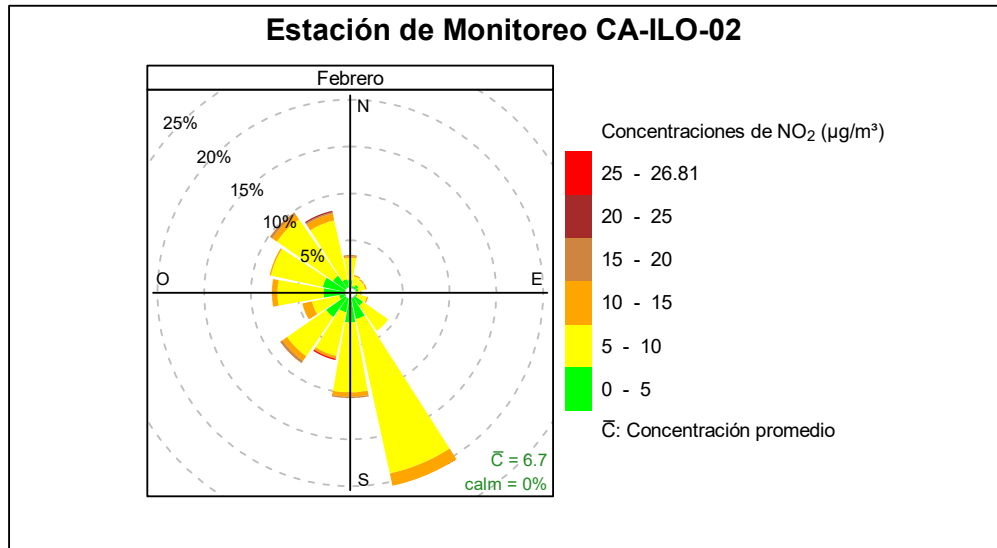
Figura 3.8.17. Rosa de concentración del NO 2 en la estación de monitoreo Ilo - Pacocha (CA-ILO-02), febrero de 2025
