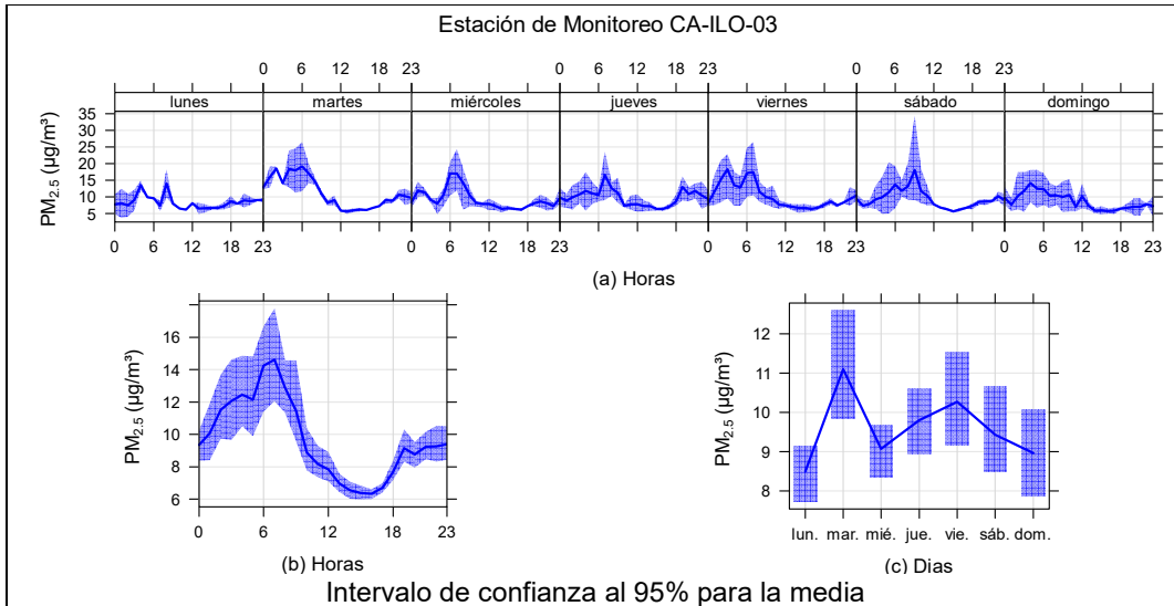
Figura 3.9.3. Concentraciones promedio horarias de PM_{2,5} en la estación de monitoreo Ilo - José Pardo (CA-ILO-03), de febrero de 2025
