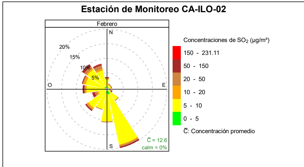
Figura 3.8.9. Rosa de concentración del SO 2 en la estación de monitoreo Ilo - Pacocha (CA-ILO-02), febrero de 2025
