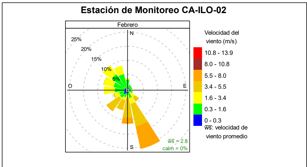
Figura 3.1.1. Rosa de viento de la estación de monitoreo Ilo - Pacocha (CA-ILO-02), febrero de 2025 4
