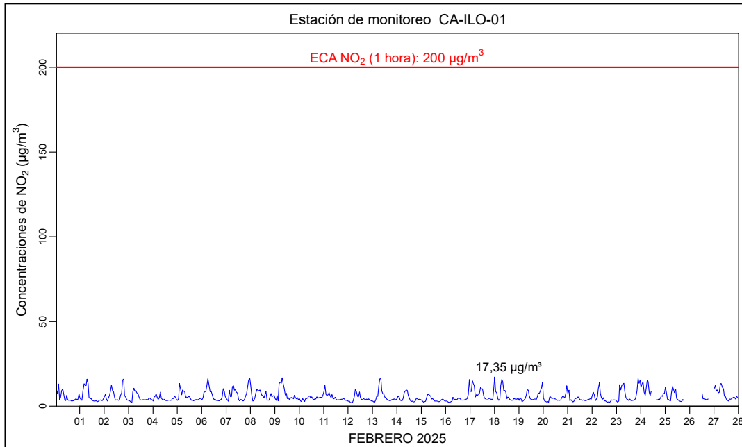
Figura 3.6.1. Concentraciones de horarias de NO 2 en la estación de monitoreo Ilo – Bolognesi (CA-ILO-01), febrero de 2025.
