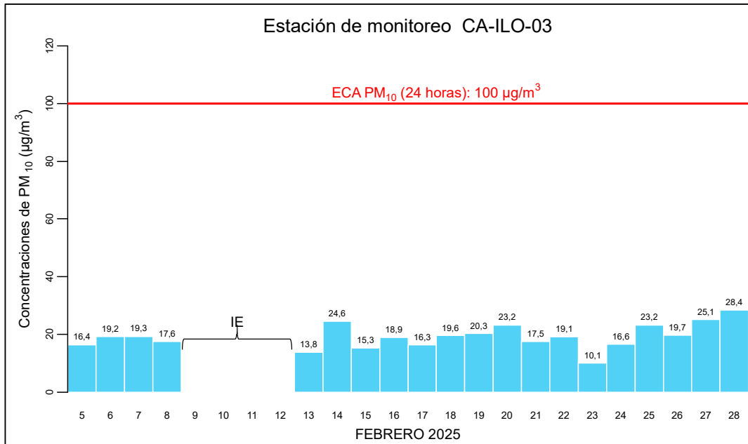
Figura 3.3.3. Concentraciones de 24 horas de PM 10 en la estación de monitoreo Ilo - José Pardo (CA-ILO-03), febrero de 2025
