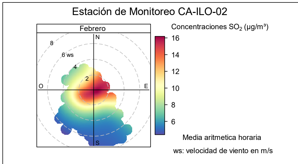
Figura 3.10.1. Grafica polar de las concentraciones promedio de SO 2 en la estación de monitoreo Ilo - Pacocha (CA-ILO-02), febrero de 2025
