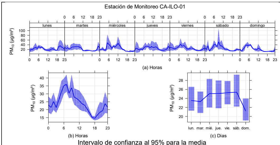
Figura 3.9.4. Concentraciones promedio horarias de PM_{10} en la estación de monitoreo Ilo – Bolognesi (CA-ILO-01), de febrero de 2025
