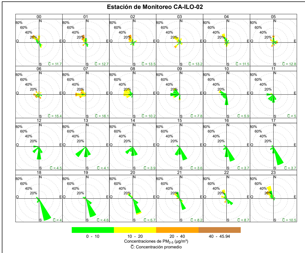
Figura 3.8.3. Rosa de concentración horaria del PM 2.5 en la estación de monitoreo Ilo - Pacocha (CA-ILO-02), febrero de 2025
