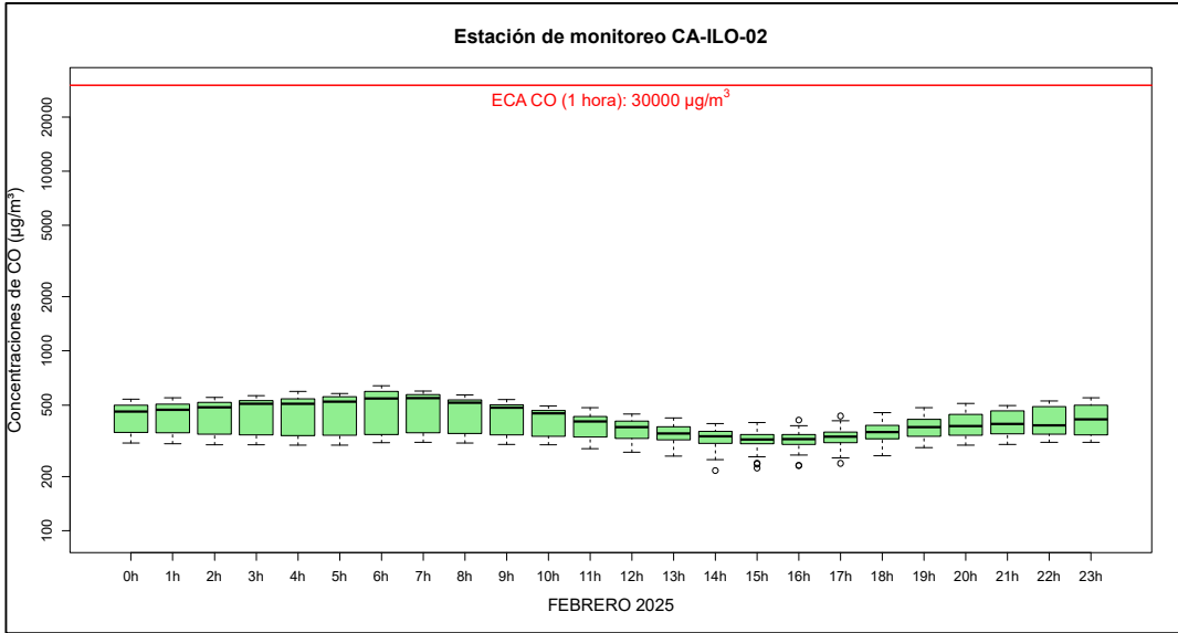
Figura 3.7.1. Concentraciones horarias de CO en la estación de monitoreo Ilo - Pacocha (CA-ILO-02), febrero de 2025
