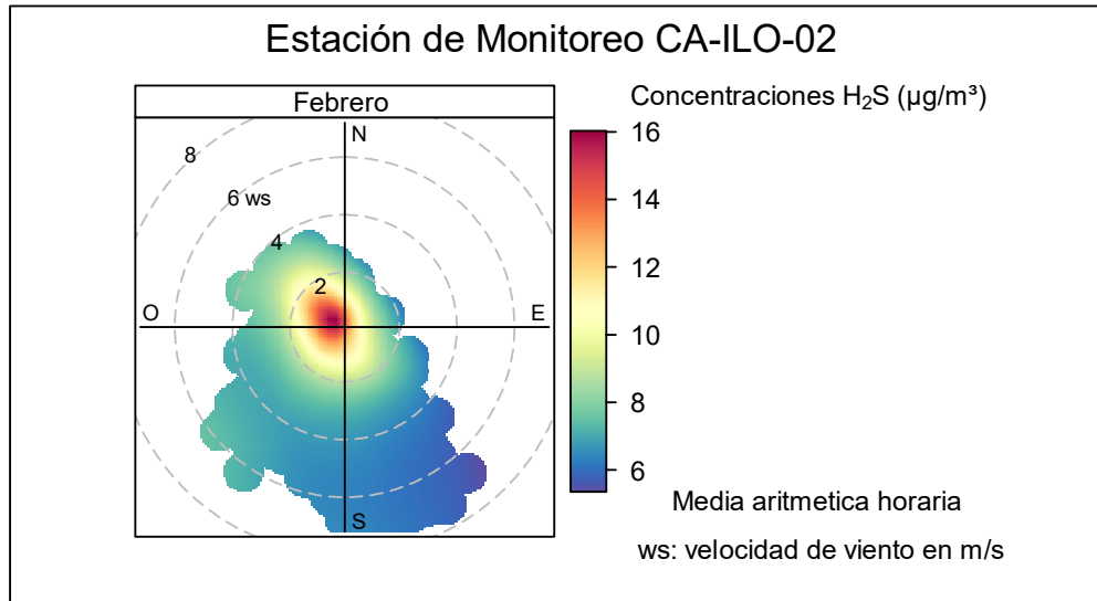
Figura 3.10.4. Grafica polar de las concentraciones promedio de H 2 S en la estación de monitoreo Ilo - Pacocha (CA-ILO-02), febrero de 2025
