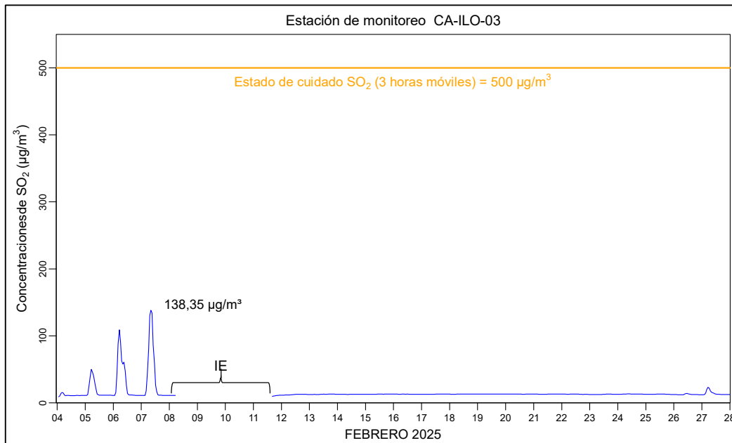
Figura 3.11.3. Concentraciones de promedio móvil de 3 horas de SO 2 en la estación de monitoreo Ilo - José Pardo (CA-ILO-03), en febrero de 2025
