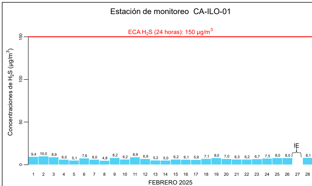
Figura 3.5.1. Concentraciones de 24 horas de H 2 S en la estación de monitoreo Ilo – Bolognesi (CA-ILO-01), febrero de 2025
