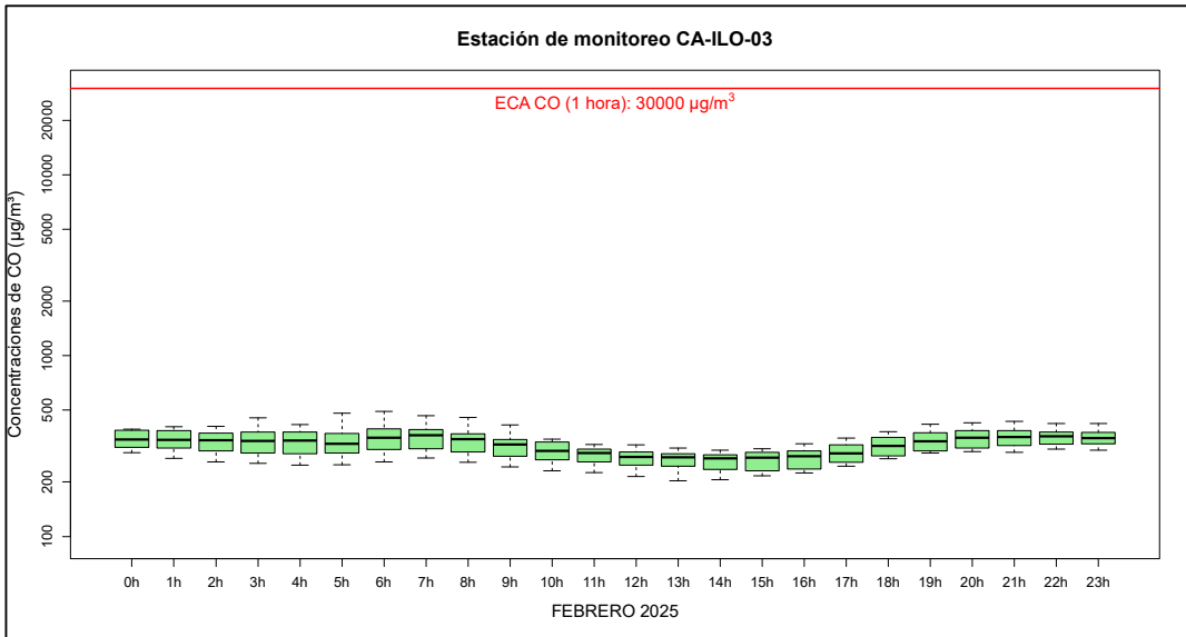
Figura 3.7.2. Concentraciones horarias de CO en la estación de monitoreo Ilo - José Pardo (CA-ILO-03), febrero de 2025
