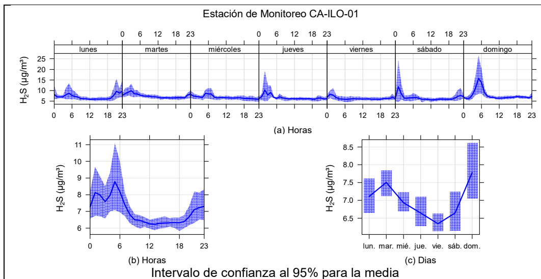
Figura 3.9.10. Concentraciones promedio horarias de H 2 S en la estación de monitoreo Ilo – Bolognesi (CA-ILO-01), de febrero de 2025
