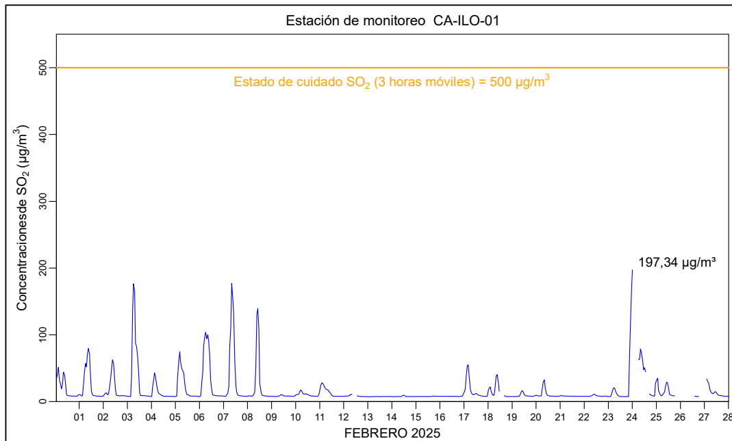
Figura 3.11.1. Concentraciones de promedio móvil de 3 horas de SO 2 en la estación de monitoreo Ilo – Bolognesi (CA-ILO-01), en febrero de 2025
