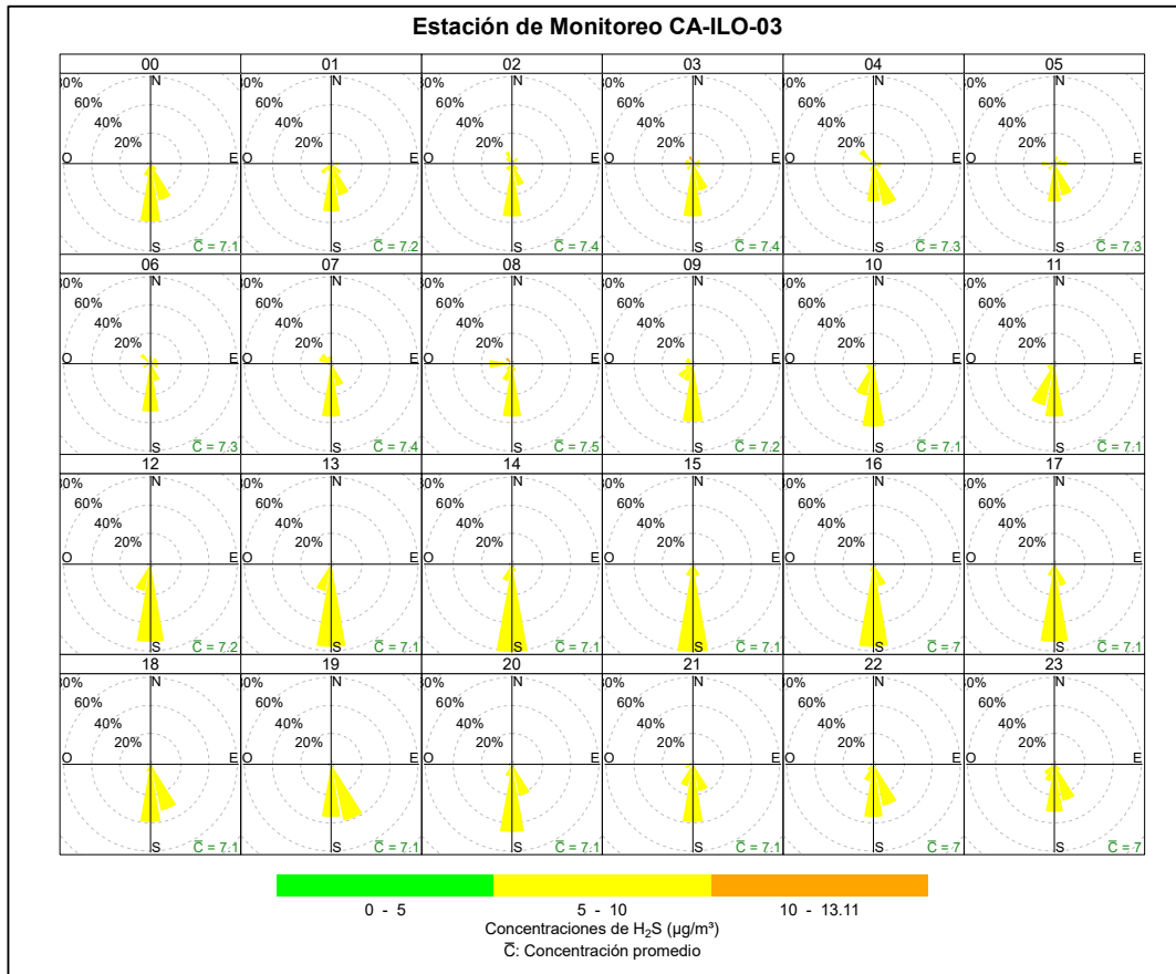
Figura 3.8.16. Rosa de concentración horaria del H 2 S en la estación de monitoreo Ilo - José Pardo (CA-ILO-03), febrero de 2025
