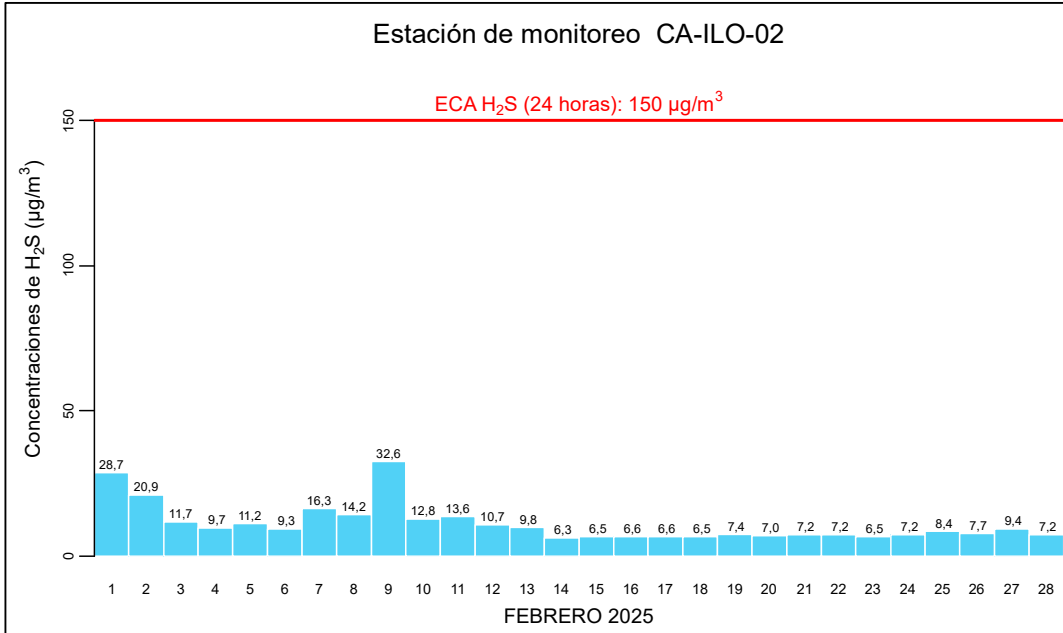
Figura 3.5.2. Concentraciones de 24 horas de H 2 S en la estación de monitoreo Ilo - Pacocha (CA-ILO-02), febrero de 2025
