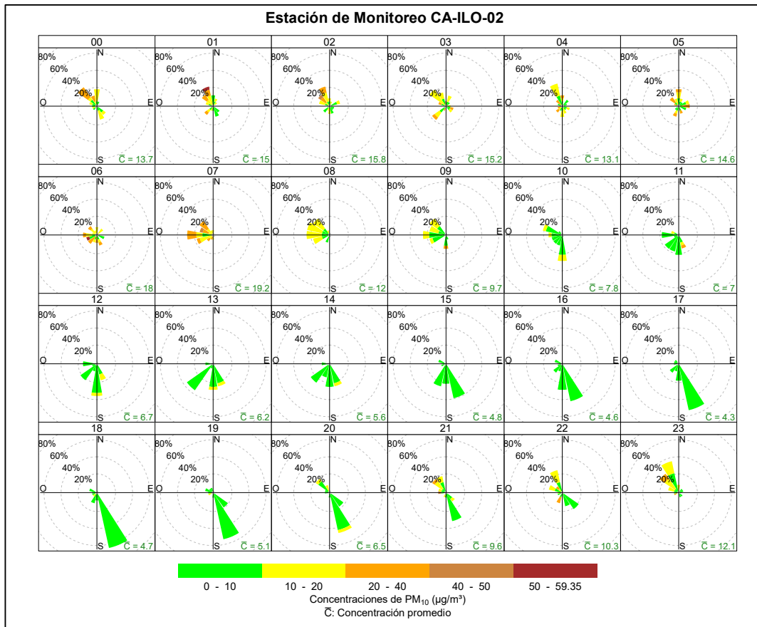
Figura 3.8.7. Rosa de concentración horaria del PM_{10} en la estación de monitoreo Ilo - Pacocha (CA-ILO-02), febrero de 2025
