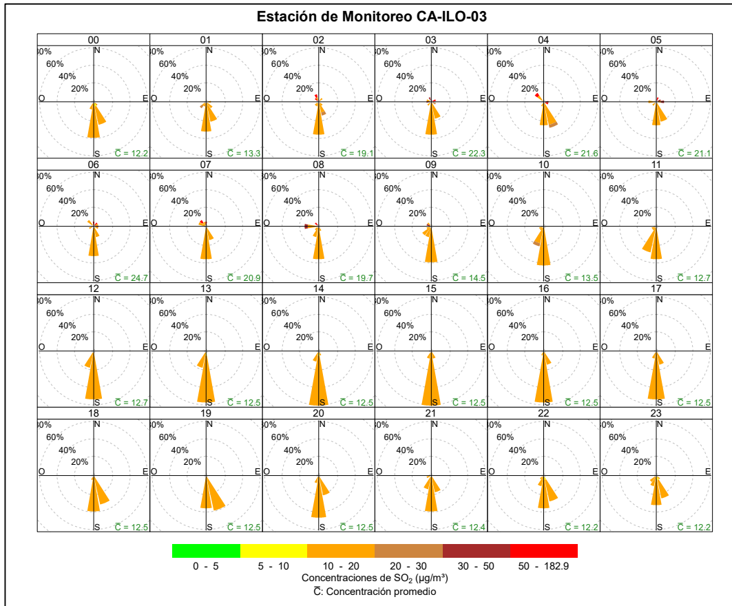
Figura 3.8.12. Rosa de concentración horaria del SO 2 en la estación de monitoreo Ilo - José Pardo (CA-ILO-03), febrero de 2025
