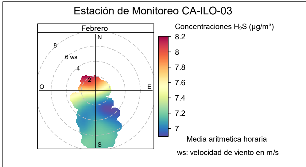
Figura 3.10.5. Grafica polar de las concentraciones promedio de H 2 S en la estación de monitoreo Ilo - José Pardo (CA-ILO-03), febrero de 2025
