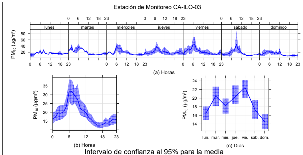
Figura 3.9.6. Concentraciones promedio horarias de PM_{10} en la estación de monitoreo Ilo - José Pardo (CA-ILO-03), de febrero de 2025
