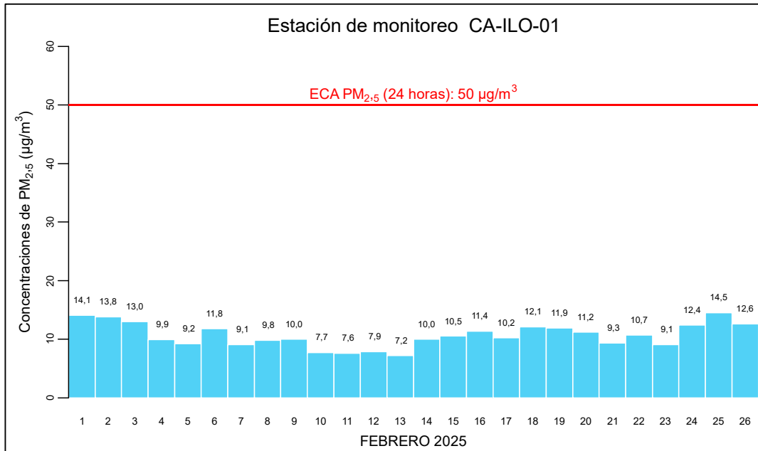
Figura 3.2.1. Concentraciones de 24 horas de PM 2,5 en la estación de monitoreo Ilo – Bolognesi (CA-ILO-01), febrero de 2025
