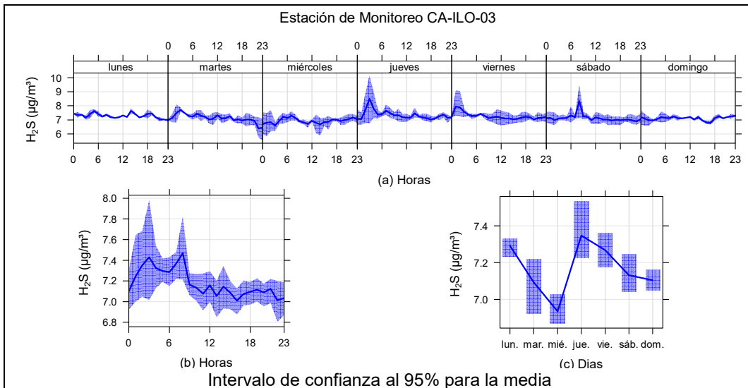
Figura 3.9.12. Concentraciones promedio horarias de H 2 S en la estación de monitoreo Ilo - José Pardo (CA-ILO-03), de febrero de 2025
