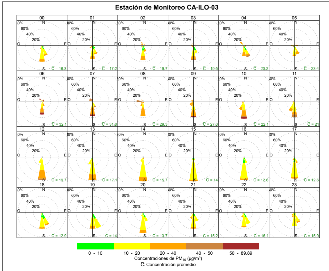
Figura 3.8.8. Rosa de concentración horaria del PM 10 en la estación de monitoreo Ilo - José Pardo (CA-ILO-03), febrero de 2025
