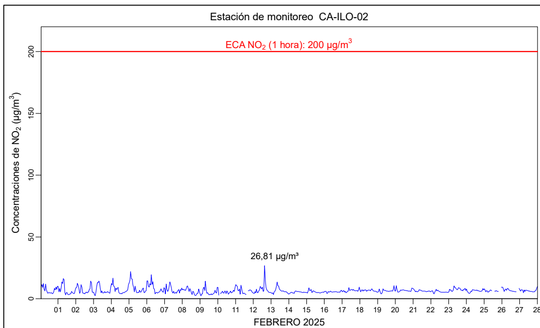
Figura 3.6.2. Concentraciones de horarias de NO 2 en la estación de monitoreo Ilo - Pacocha (CA-ILO-02), febrero de 2025.
