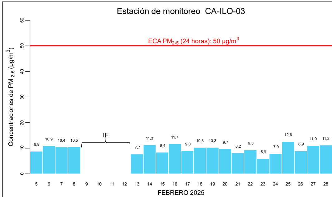
Figura 3.2.3. Concentraciones de 24 horas de PM 2.5 en la estación de monitoreo Ilo - José Pardo (CA-ILO-03), febrero de 2025
