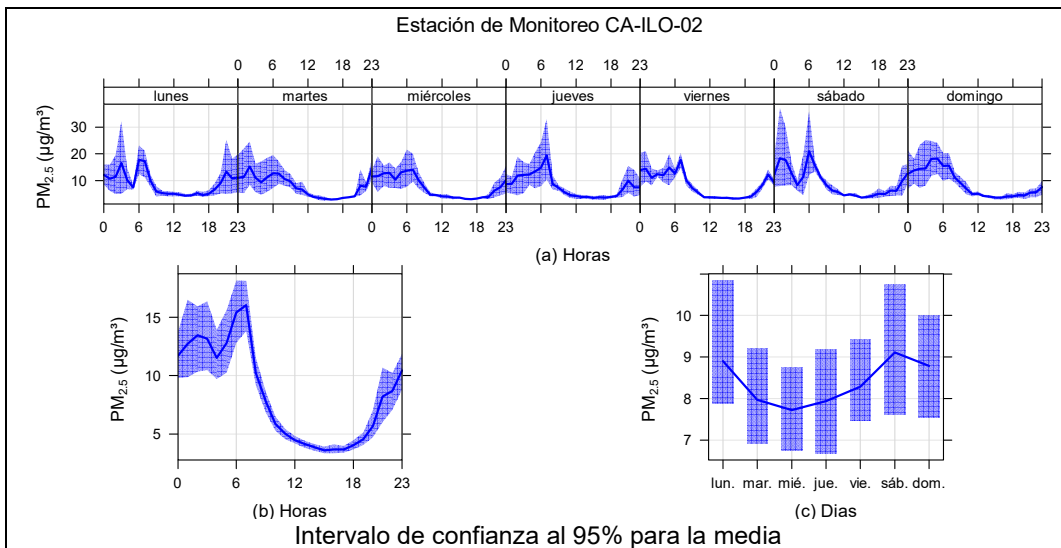
Figura 3.9.2. Concentraciones promedio horarias de PM_{2.5} en la estación de monitoreo Ilo – Pacocha (CA-ILO-02), de febrero de 2025
