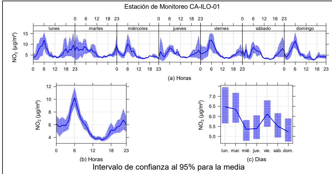
Figura 3.9.13. Concentraciones promedio horarias de NO 2 en la estación de monitoreo Ilo – Bolognesi (CA-ILO-01), de febrero de 2025
