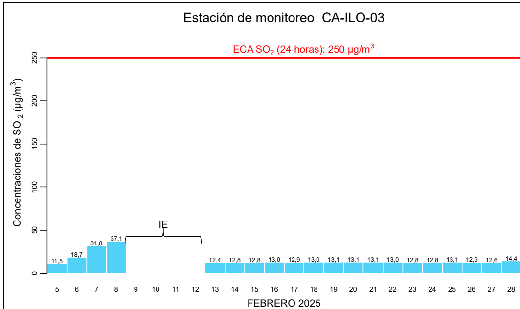
Figura 3.4.3. Concentraciones de 24 horas de SO 2 en la estación de monitoreo Ilo - José Pardo (CA-ILO-03), febrero de 2025
