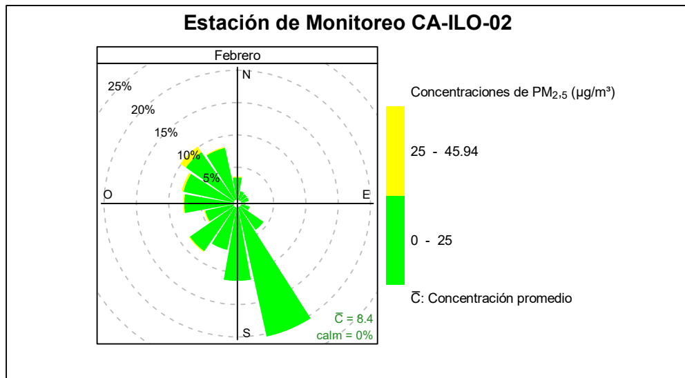
Figura 3.8.1. Rosa de concentración del PM 2,5 en la estación de monitoreo Ilo - Pacocha (CA-ILO-02), febrero del 2025
