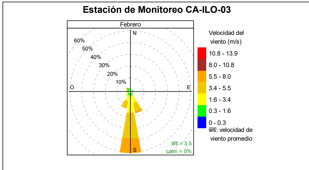
Figura 3.1.3. Rosa de viento de la estación de monitoreo Ilo - José Pardo (CA-ILO-03), febrero de 2025 6
