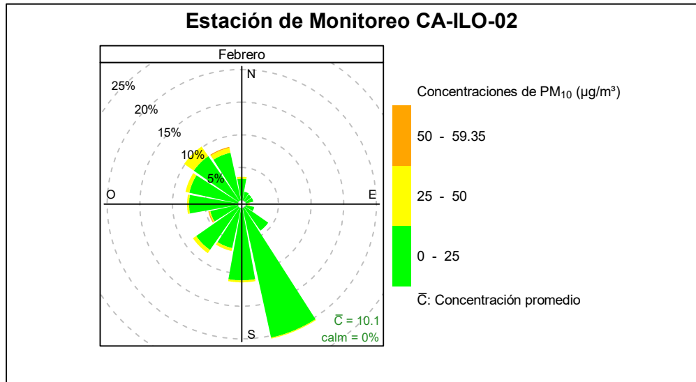
Figura 3.8.5. Rosa de concentración del PM 10 en la estación de monitoreo Ilo - Pacocha (CA-ILO-02), febrero de 2025
