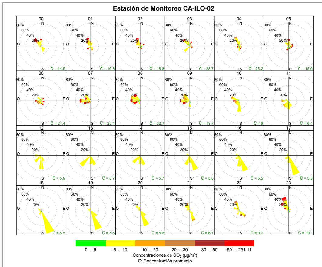
Figura 3.8.11. Rosa de concentración horaria del SO 2 en la estación de monitoreo Ilo - Pacocha (CA-ILO-02), febrero de 2025
