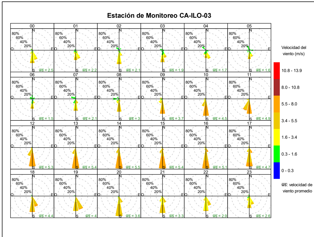
Figura 3.1.4. Rosa de viento horaria de la estación de monitoreo Ilo - José Pardo (CA-ILO-03), febrero de 2025
