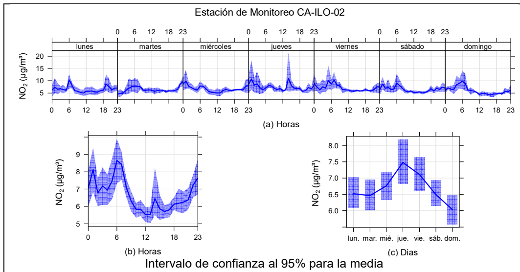
Figura 3.9.14. Concentraciones promedio horarias de NO 2 en la estación de monitoreo Ilo - Pacocha (CA-ILO-02), de febrero de 2025
