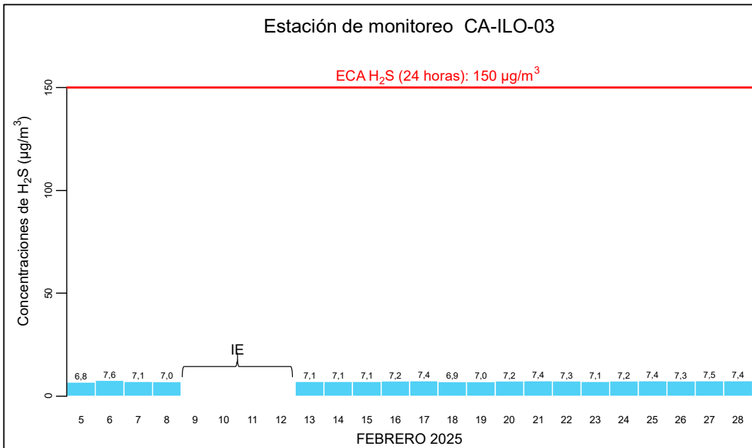
Figura 3.5.3. Concentraciones de 24 horas de H 2 S en la estación de monitoreo Ilo - José Pardo (CA-ILO-03), febrero de 2025
