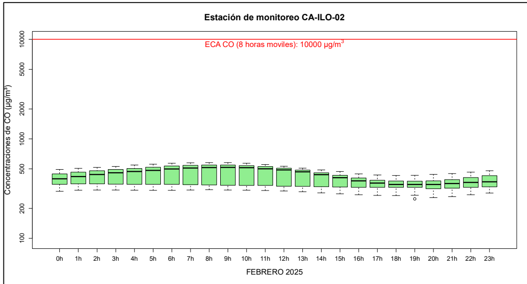
Figura 3.7.3. Concentraciones de promedio móvil de 8 horas de CO en la estación de monitoreo Ilo - Pacocha (CA-ILO-02), febrero de 2025
