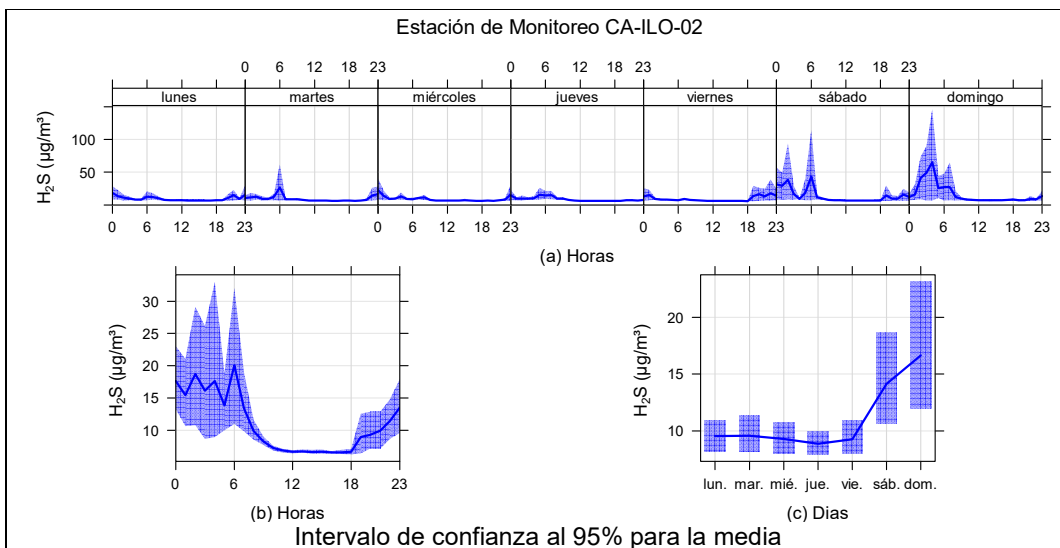
Figura 3.9.11. Concentraciones promedio horarias de H 2 S en la estación de monitoreo Ilo - Pacocha (CA-ILO-02), de febrero de 2025
