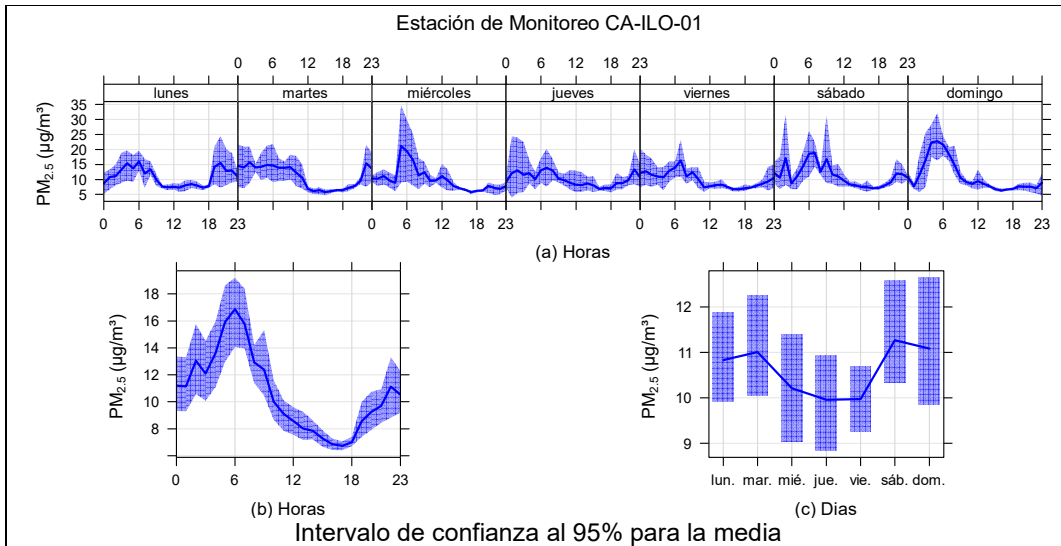
Figura 3.9.1. Concentraciones promedio horarias de PM_{2.5} en la estación de monitoreo Ilo – Bolognesi (CA-ILO-01), de febrero de 2025
