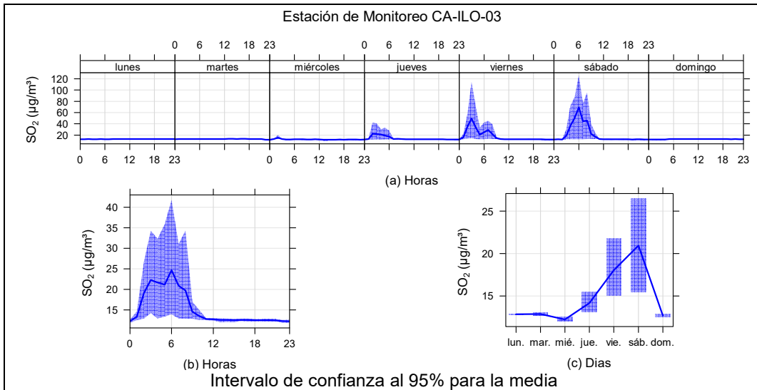
Figura 3.9.9. Concentraciones promedio horarios de SO 2 en la estación de monitoreo Ilo - José Pardo (CA-ILO-03), de febrero de 2025
