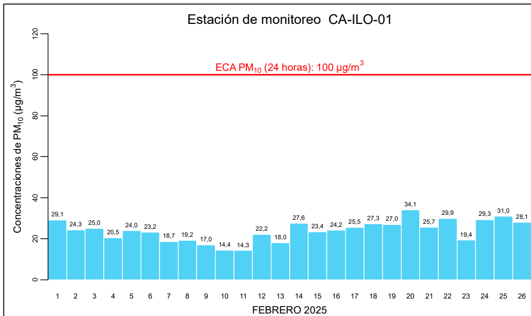
Figura 3.3.1. Concentraciones de 24 horas de PM 10 en la estación de monitoreo Ilo – Bolognesi (CA-ILO-01), febrero de 2025
