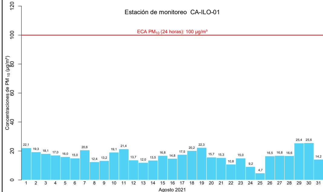
Figura 4.7. Concentraciones de 24 horas de PM 10 en la estación de monitoreo CA-ILO-01, en agosto de 2021
