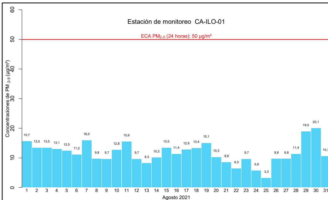
Figura 4.4. Concentraciones de 24 horas de PM 2,5 en la estación de monitoreo CA-ILO-01, en agosto de 2021
