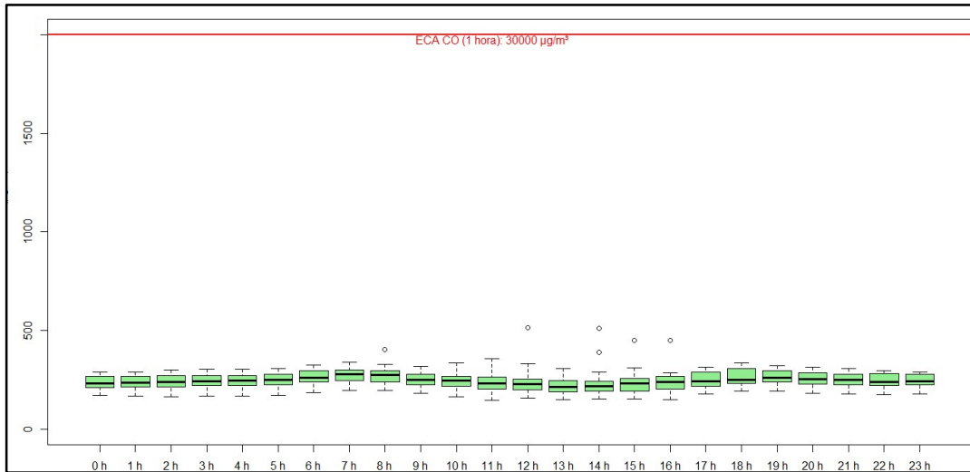
Figura 4.20. Concentraciones de horarias de CO en la estación de monitoreo CA-ILO-02, en agosto de 2021
