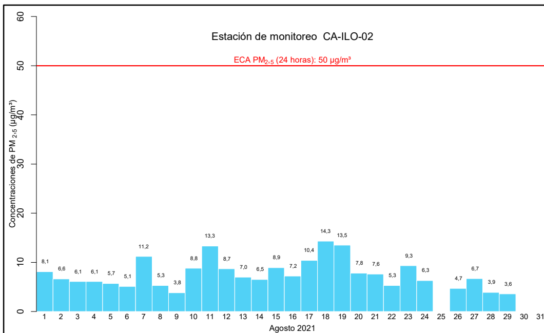
Figura 4.5. Concentraciones de 24 horas de PM 2,5 en la estación de monitoreo CA-ILO-02, en agosto de 2021 1
