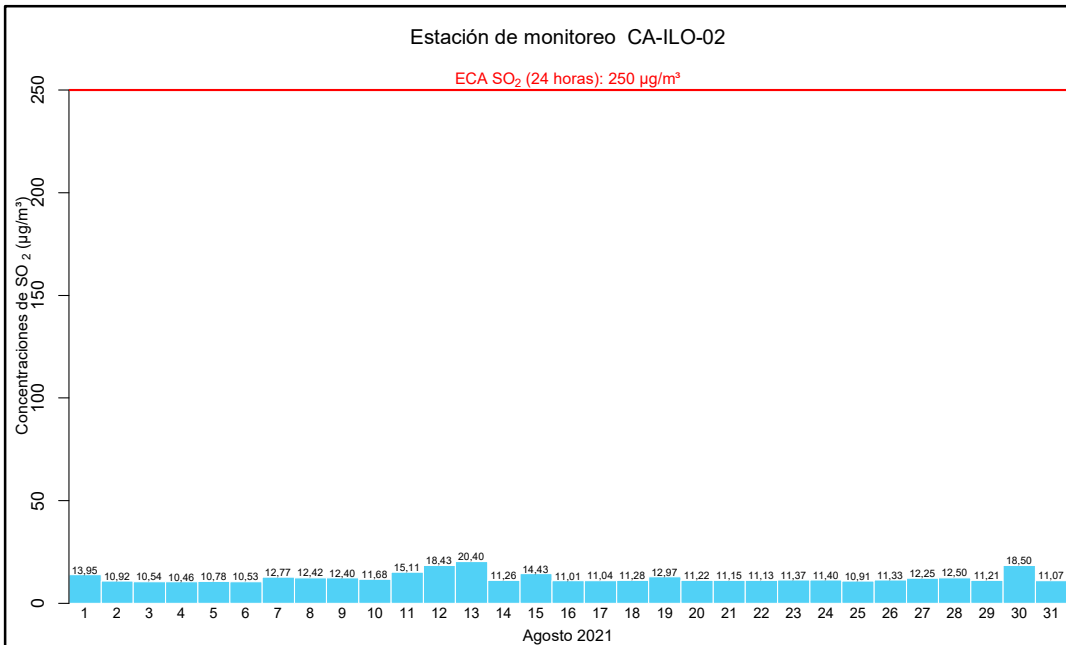
Figura 4.11. Concentraciones de 24 horas de SO 2 en la estación de monitoreo CA-ILO-02, en agosto de 2021
