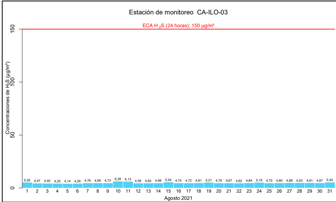
Figura 4.15. Concentraciones de 24 horas de H 2 S en la estación de monitoreo CA-ILO-03, en agosto de 2021
