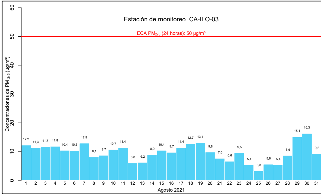
Figura 4.6. Concentraciones de 24 horas de PM 2,5 en la estación de monitoreo CA-ILO-03, en agosto de 2021
