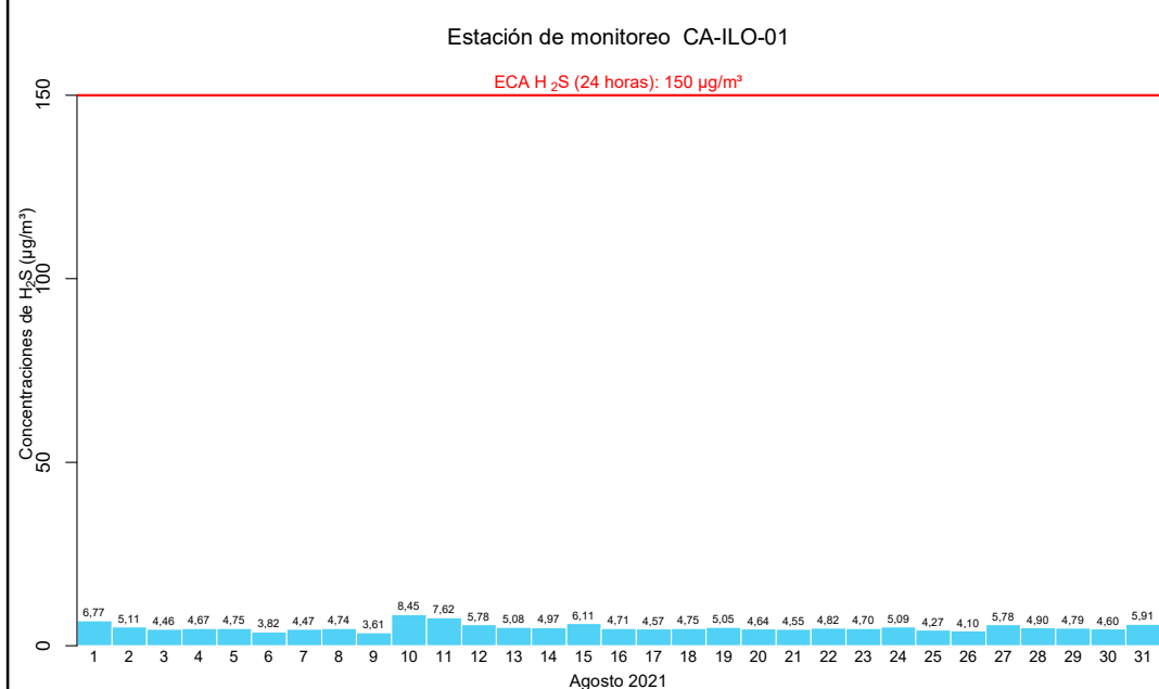
Figura 4.13. Concentraciones de 24 horas de H 2 S en la estación de monitoreo CA-ILO-01, en agosto de 2021
