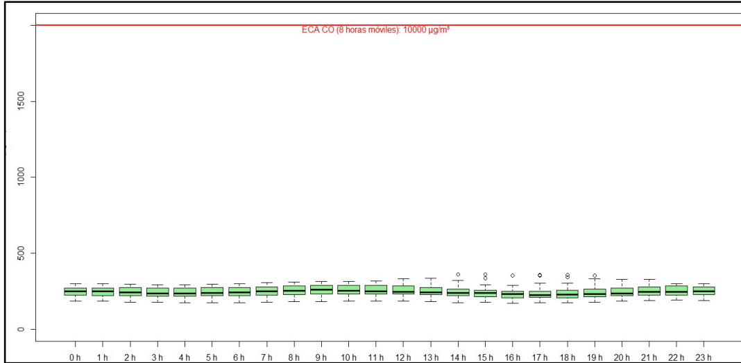
Figura 4.23. Concentraciones de promedio móvil de 8 horas de CO en la estación de monitoreo CA-ILO-02, en agosto de 2021
