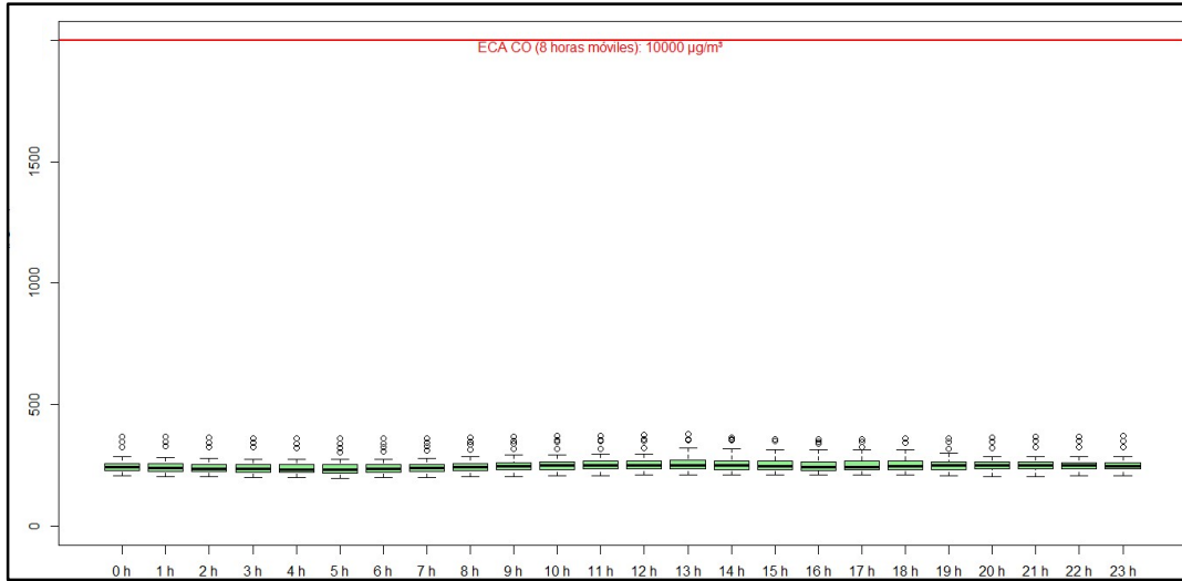
Figura 4.22. Concentraciones de promedio móvil de 8 horas de CO en la estación de monitoreo CA-ILO-01, en agosto de 2021
