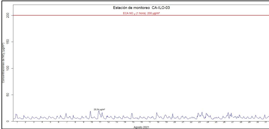
Figura 4.18. Concentraciones de horarias de NO 2 en la estación de monitoreo CA-ILO-03, en agosto de 2021
