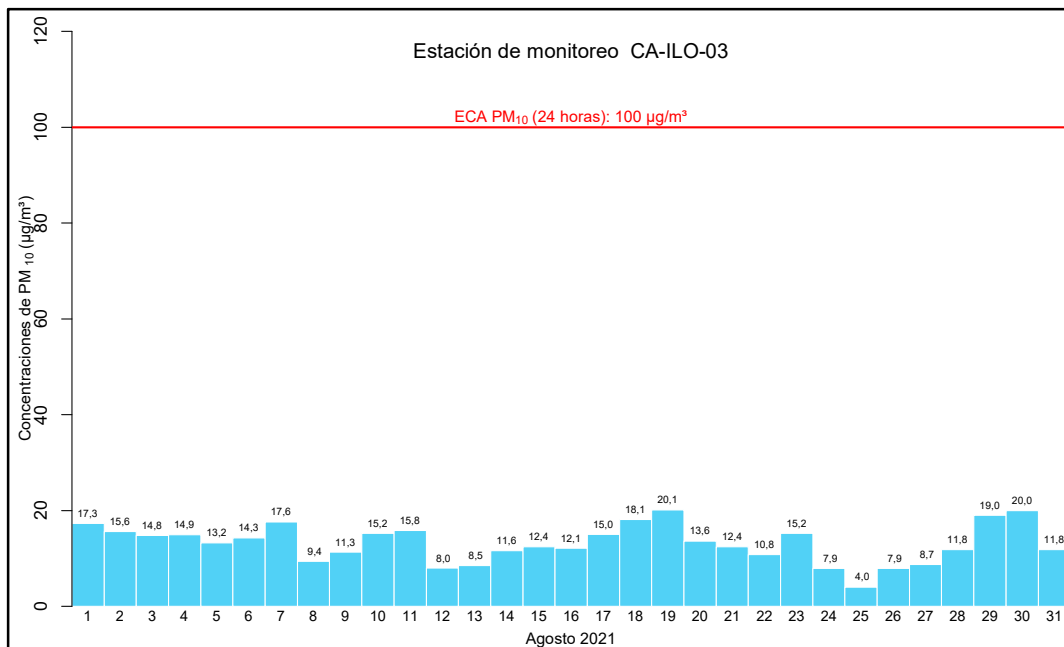
Figura 4.9. Concentraciones de 24 horas de PM 10 en la estación de monitoreo CA-ILO-03, en agosto de 2021
