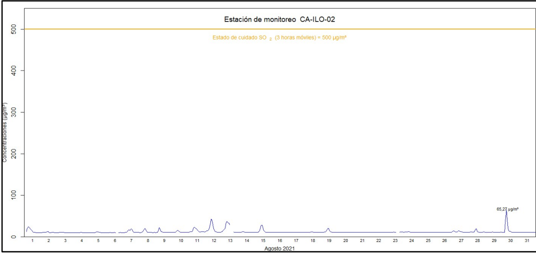
Figura 4.26. Concentraciones de promedio móvil de 3 horas de SO 2 en la estación de monitoreo CA-ILO-02, en agosto de 2021
