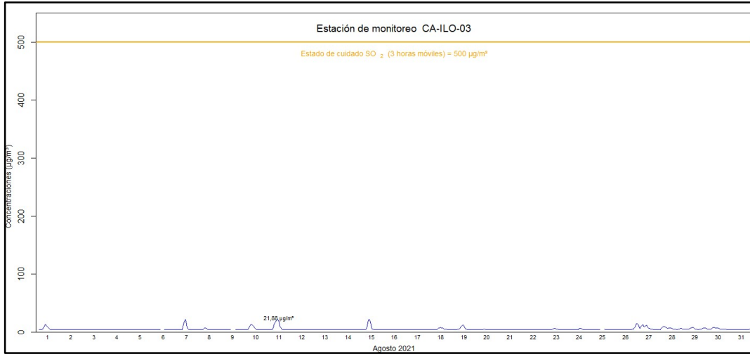
Figura 4.27. Concentraciones de promedio móvil de 3 horas de SO 2 en la estación de monitoreo CA-ILO-03, en agosto de 2021
