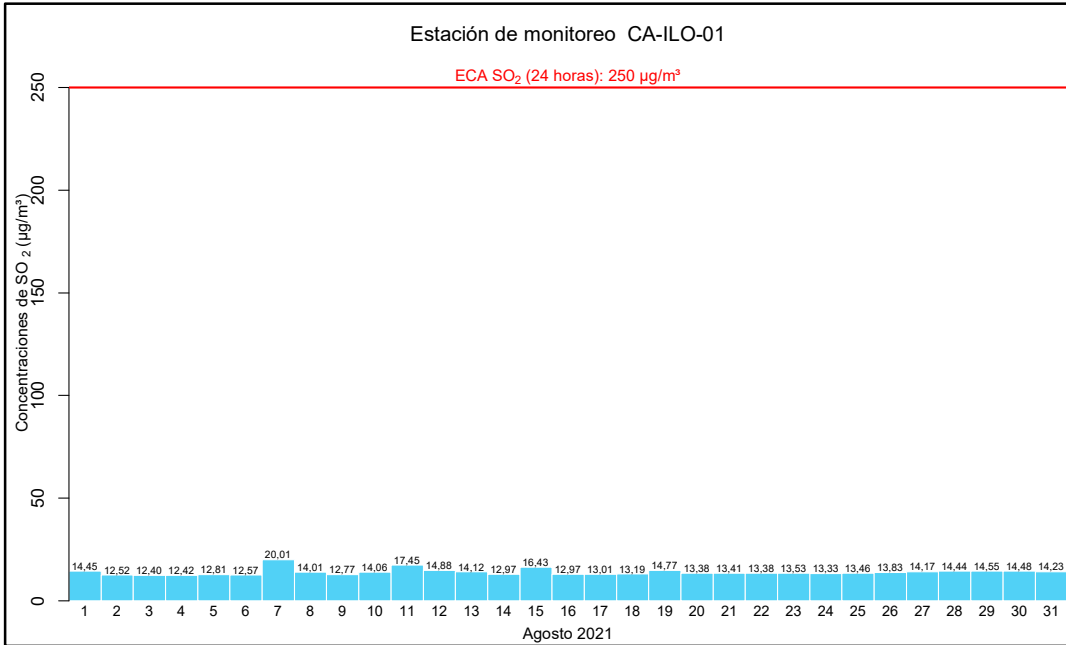
Figura 4.10. Concentraciones de 24 horas de SO 2 en la estación de monitoreo CA-ILO-01, en agosto de 2021
