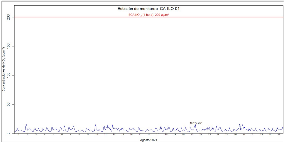
Figura 4.16. Concentraciones de horarias de NO 2 en la estación de monitoreo CA-ILO-01, en agosto de 2021
