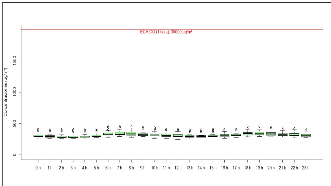
Figura 4.21. Concentraciones de horarias de CO en la estación de monitoreo CA-ILO-03, en agosto de 2021
