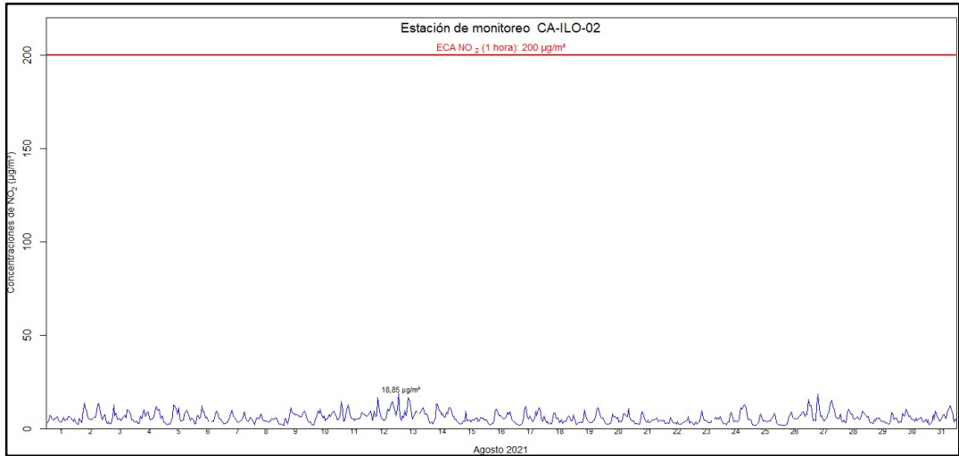
Figura 4.17. Concentraciones de horarias de NO 2 en la estación de monitoreo CA-ILO-02, en agosto de 2021
