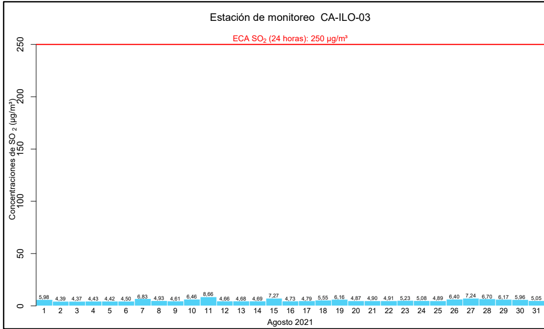
Figura 4.12. Concentraciones de 24 horas de SO 2 en la estación de monitoreo CA-ILO-03, en agosto de 2021
