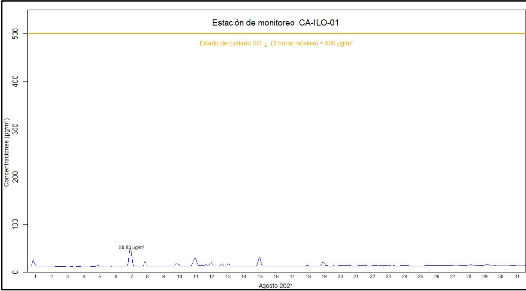
Figura 4.25. Concentraciones de promedio móvil de 3 horas de SO 2 en la estación de monitoreo CA-ILO-01, en agosto de 2021
