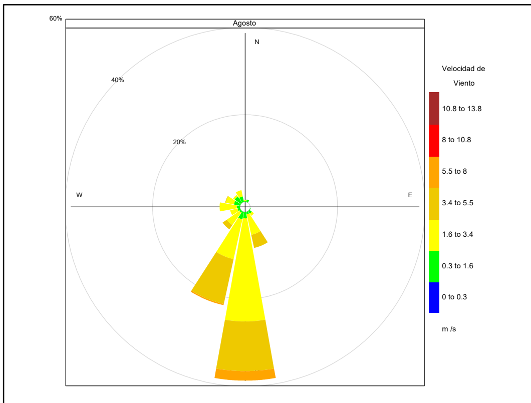
Figura 4.1. Rosa de viento de la estación de monitoreo CA-ILO-01, en agosto de 2021
