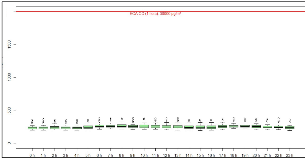
Figura 4.19. Concentraciones de horarias de CO en la estación de monitoreo CA-ILO-01, en agosto de 2021
