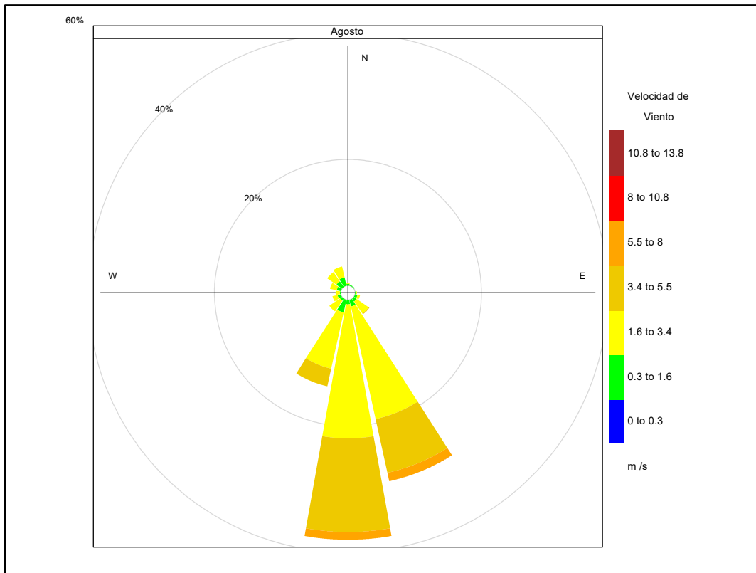
Figura 4.3. Rosa de viento de la estación de monitoreo CA-ILO-03, en agosto de 2021
