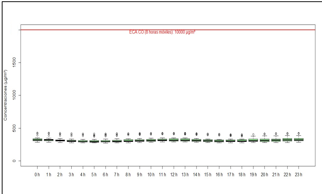
Figura 4.24. Concentraciones de promedio móvil de 8 horas de CO en la estación de monitoreo CA-ILO-03, en agosto de 2021
