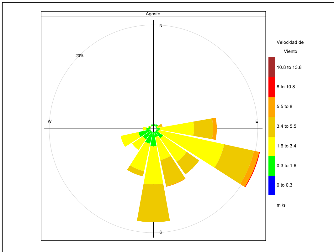
Figura 4.2. Rosa de viento de la estación de monitoreo CA-ILO-02, en agosto de 2021
