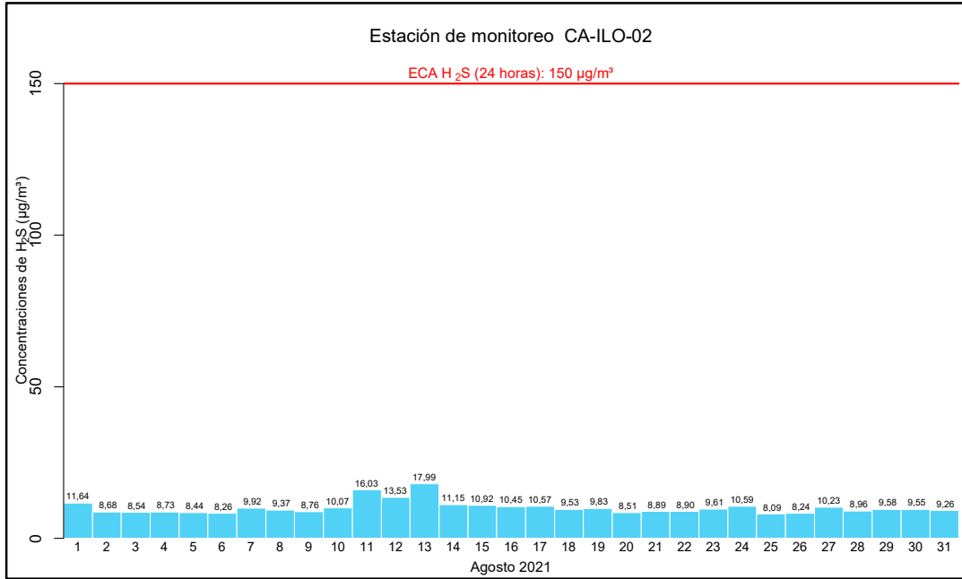
Figura 4.14. Concentraciones de 24 horas de H 2 S en la estación de monitoreo CA-ILO-02, en agosto de 2021
