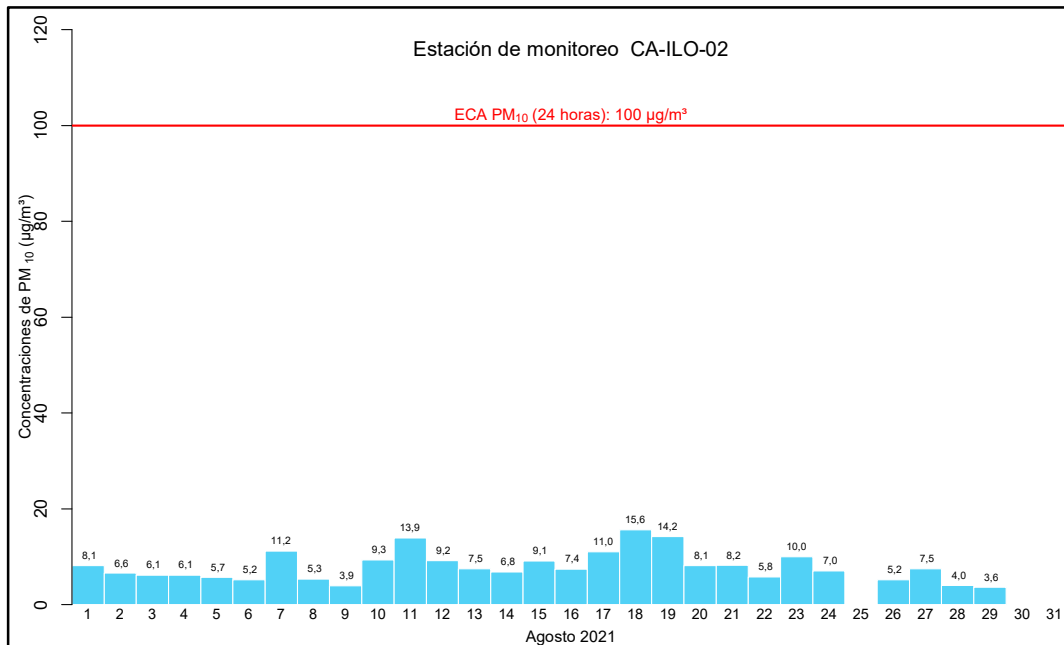
Figura 4.8. Concentraciones de 24 horas de PM 10 en la estación de monitoreo CA-ILO-02, en agosto de 2021 2
