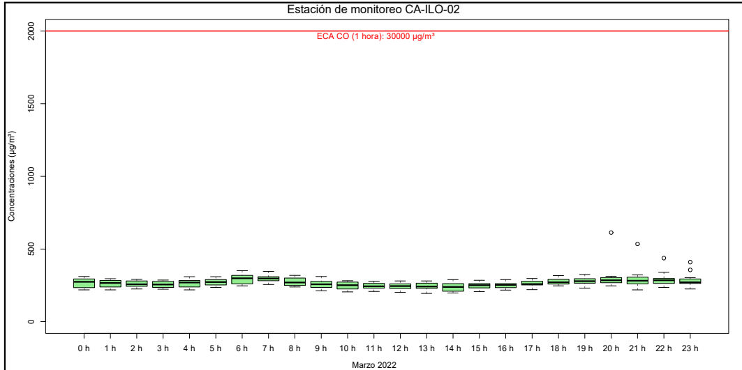
Figura 3.18. Concentraciones horarias de CO, estación de monitoreo CA-ILO-02, marzo del 2022
