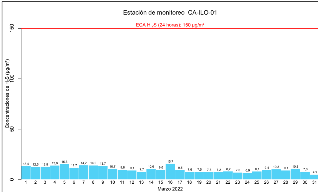
Figura 3.11. Concentraciones de 24 horas de H 2 S en la estación de monitoreo CA-ILO-01, en marzo de 2022
