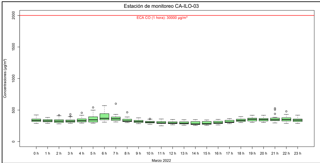
Figura 3.19. Concentraciones horarias de CO, estación de monitoreo CA-ILO-03, marzo del 2022
