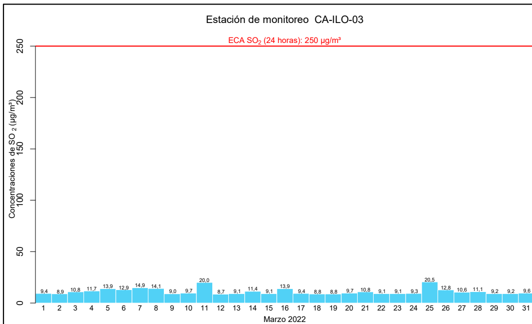
Figura 3.10. Concentraciones de 24 horas de SO 2 en la estación de monitoreo CA-ILO-03, en marzo de 2022
