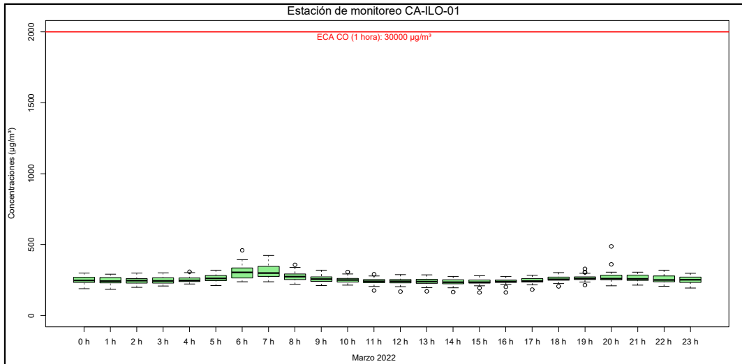
Figura 3.17. Concentraciones horarias de CO, estación de monitoreo CA-ILO-01, marzo del 2022
