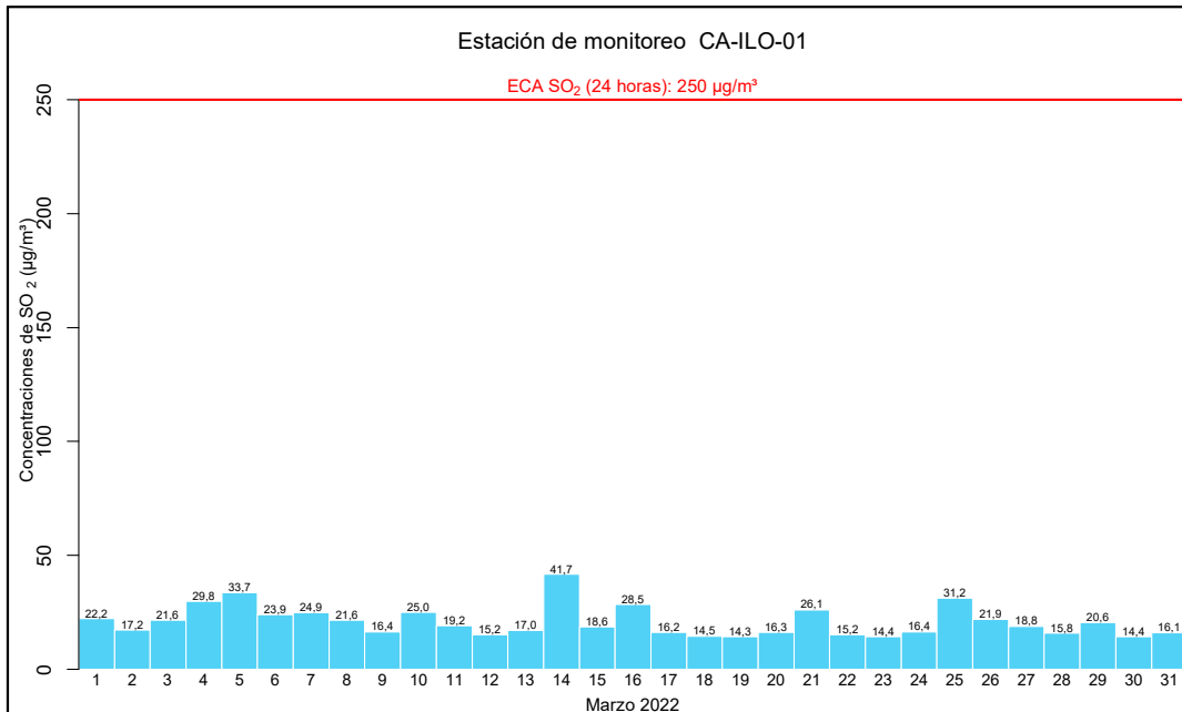
Figura 3.8. Concentraciones de 24 horas de SO 2 en la estación de monitoreo CA-ILO-01, en marzo de 2022
