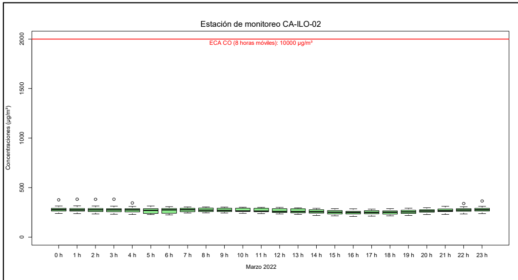
Figura 3.21. Concentraciones de promedio móvil de 8 horas de CO en la estación de monitoreo CA-ILO-02, en marzo de 2022
