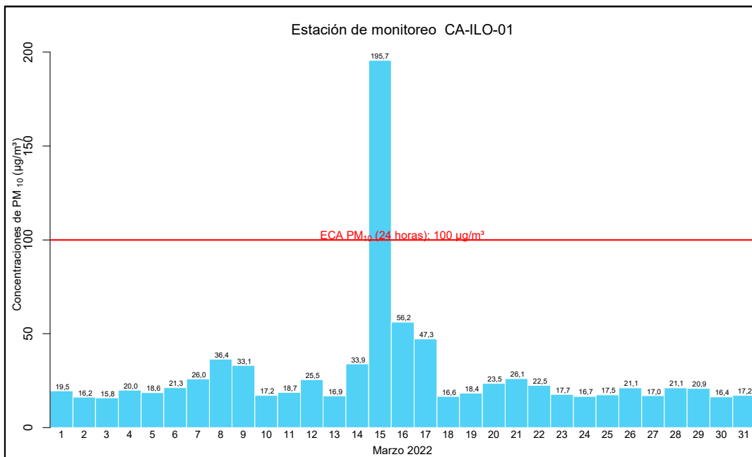
Figura 3.6. Concentraciones de 24 horas de PM 10 en la estación de monitoreo CA-ILO-01, en marzo de 2022
