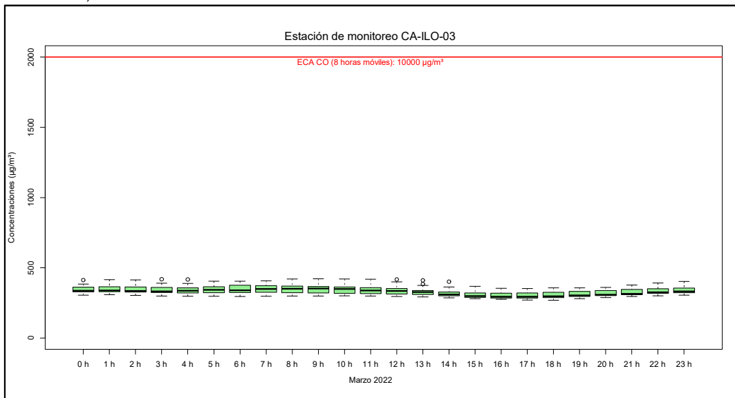
Figura 3.22. Concentraciones de promedio móvil de 8 horas de CO en la estación de monitoreo CA-ILO-03, en marzo de 2022
