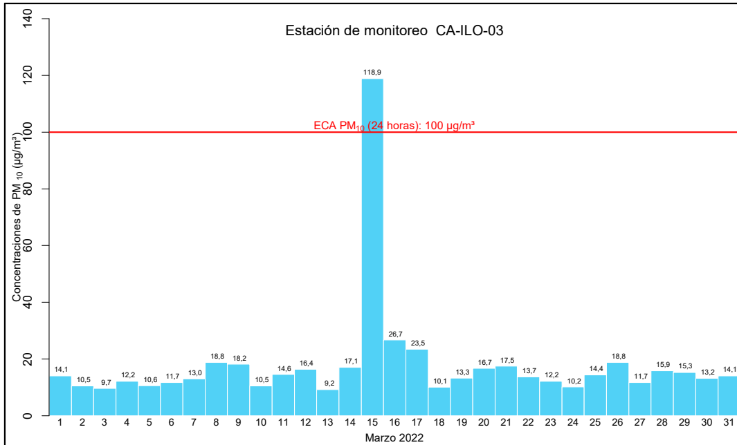
Figura 3.7. Concentraciones de 24 horas de PM 10 en la estación de monitoreo CA-ILO-03, en marzo de 2022
