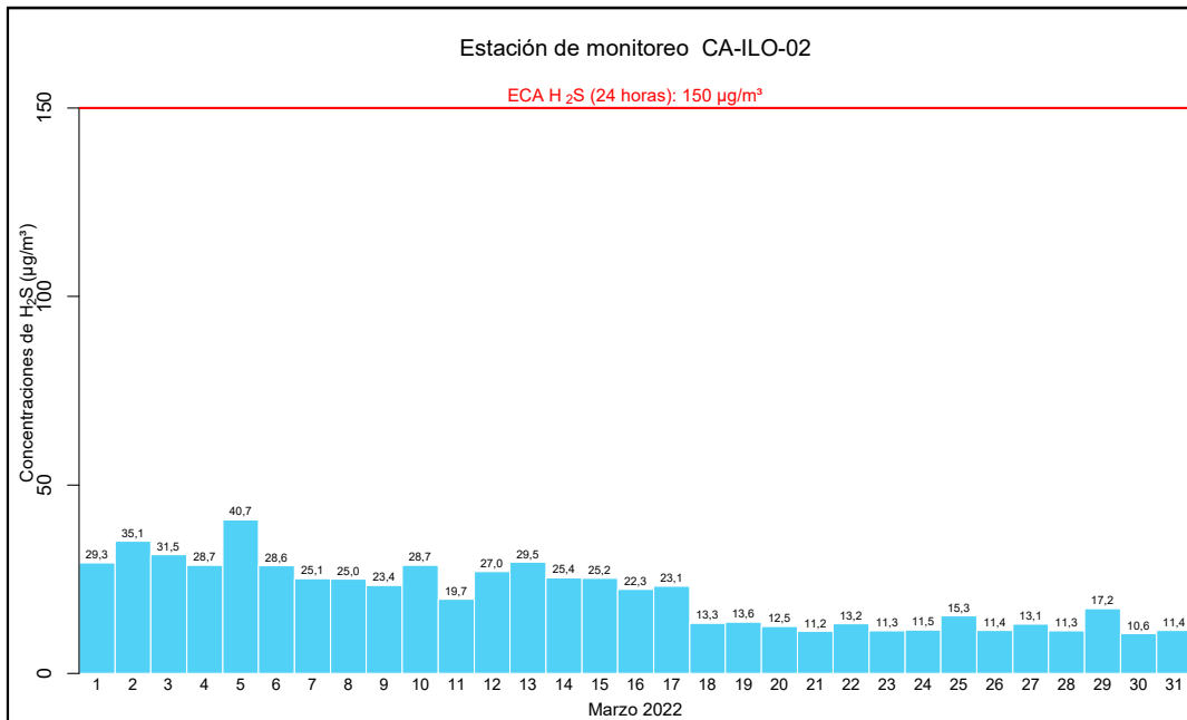
Figura 3.12. Concentraciones de 24 horas de H 2 S en la estación de monitoreo CA-ILO-02, en marzo de 2022
