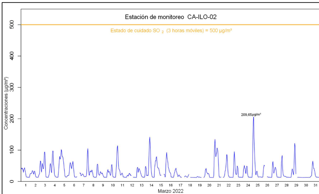
Figura 4.2. Concentraciones de promedio móvil de 3 horas de \text{SO}_2 en la estación de monitoreo CA-ILO-02, en marzo de 2022
