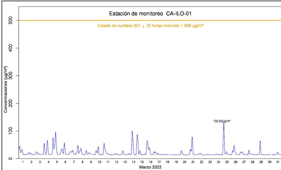
Figura 4.1. Concentraciones de promedio móvil de 3 horas de \text{SO}_2 en la estación de monitoreo CA-ILO-01, en marzo de 2022
