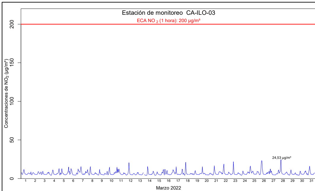
Figura 3.16. Concentraciones de horarias de NO 2 en la estación de monitoreo CA-ILO-03, en marzo de 2022
