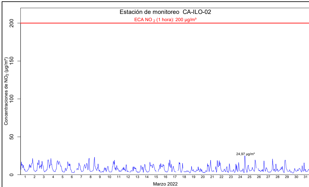
Figura 3.15. Concentraciones de horarias de NO 2 en la estación de monitoreo CA-ILO-02, en marzo de 2022
