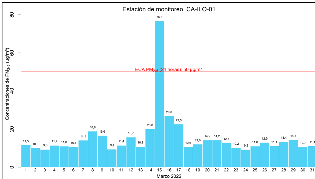
Figura 3.4. Concentraciones de 24 horas de PM 2,5 en la estación de monitoreo CA-ILO-01, en marzo de 2022
