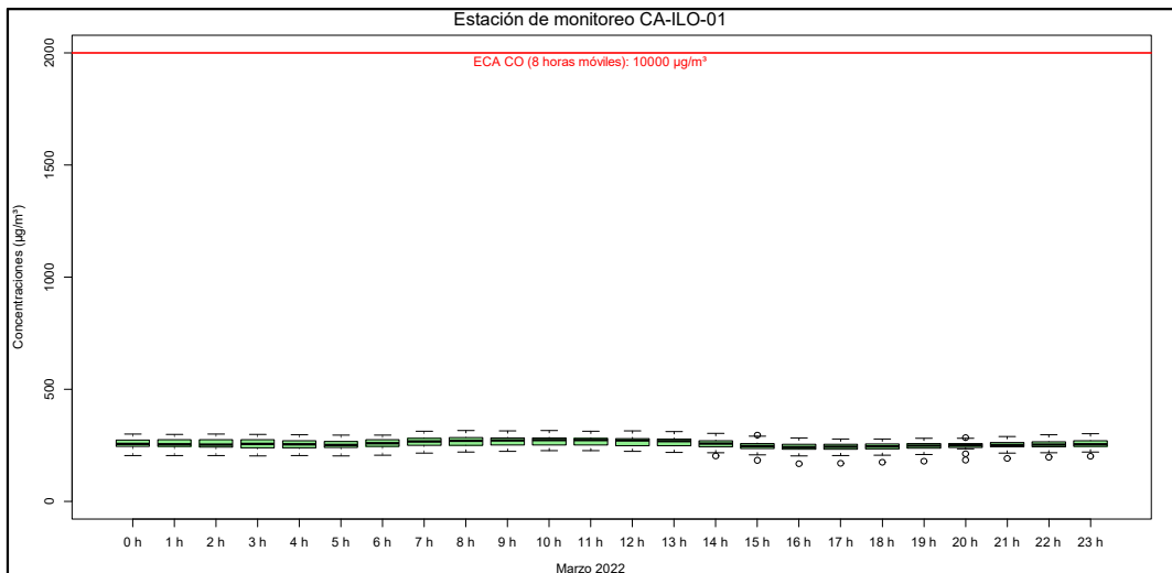
Figura 3.20. Concentraciones de promedio móvil de 8 horas de CO en la estación de monitoreo CA-ILO-01, en marzo de 2022
