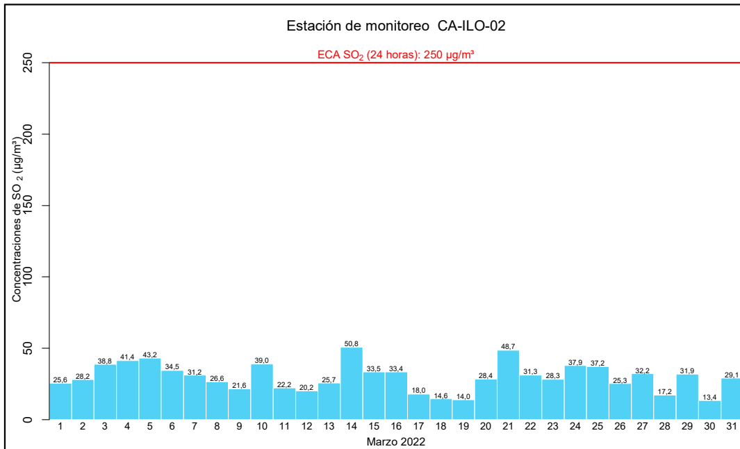
Figura 3.9. Concentraciones de 24 horas de SO 2 en la estación de monitoreo CA-ILO-02, en marzo de 2022
