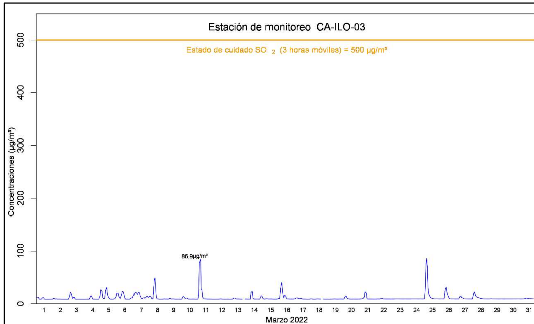
Figura 4.3. Concentraciones de promedio móvil de 3 horas de \text{SO}_2 en la estación de monitoreo CA-ILO-03, en marzo de 2022
