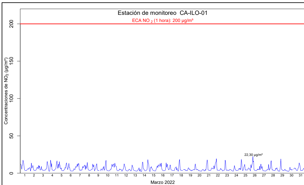
Figura 3.14. Concentraciones de horarias de NO 2 en la estación de monitoreo CA-ILO-01, en marzo de 2022
