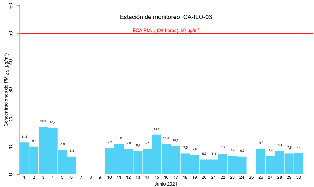
Figura 4.5. Concentraciones de 24 horas de PM 2.5 en la estación de monitoreo CA-ILO-03, en junio de 2021 3
