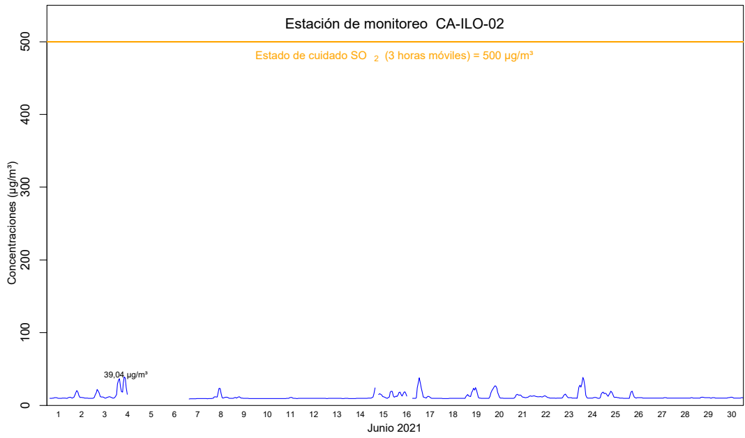
Figura 4.25. Concentraciones de promedio móvil de 3 horas de SO 2 en la estación de monitoreo CA-ILO-02, en junio de 2021 17
