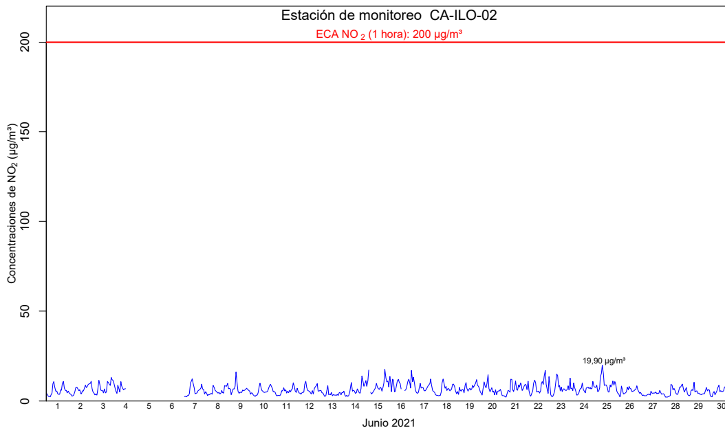
Figura 4.16. Concentraciones de horarias de NO 2 en la estación de monitoreo CA-ILO-02, en junio de 2021 14
