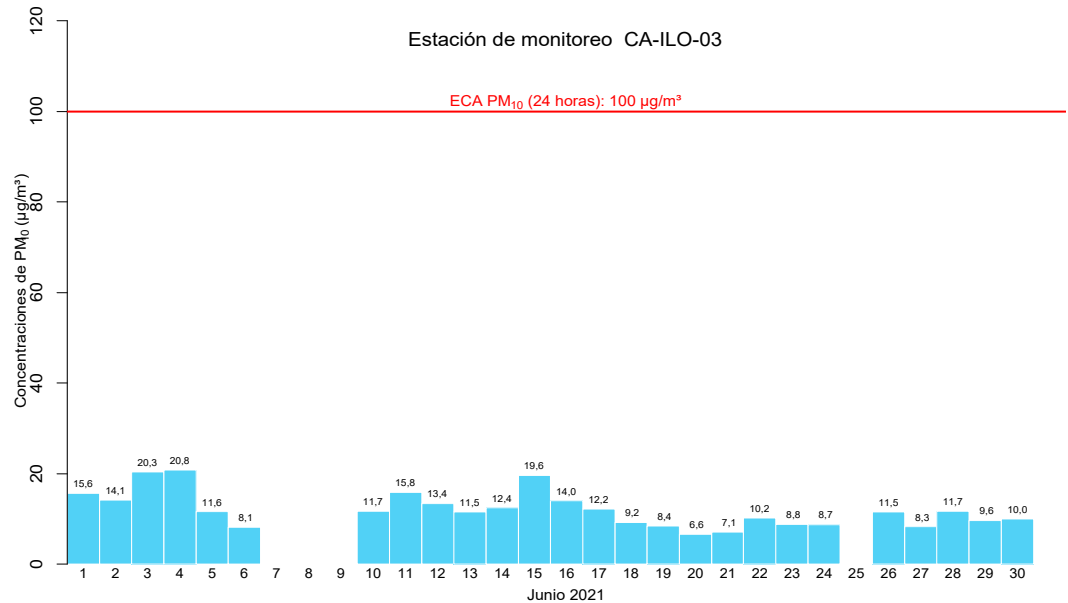
Figura 4.8. Concentraciones de 24 horas de PM 10 en la estación de monitoreo CA-ILO-03, en junio de 2021 6
