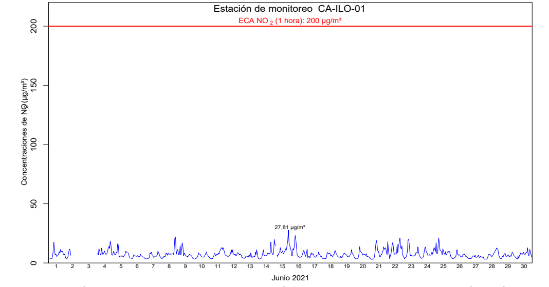
Figura 4.15. Concentraciones de horarias de NO 2 en la estación de monitoreo CA-ILO-01, en junio de 2021 13
