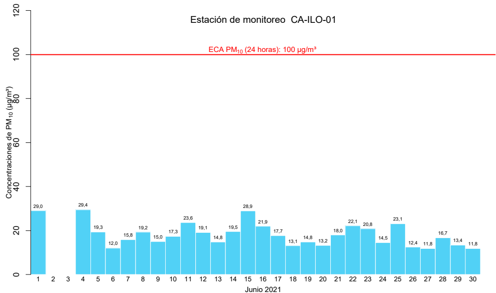
Figura 4.6. Concentraciones de 24 horas de PM 10 en la estación de monitoreo CA-ILO-01, en junio de 2021 4
