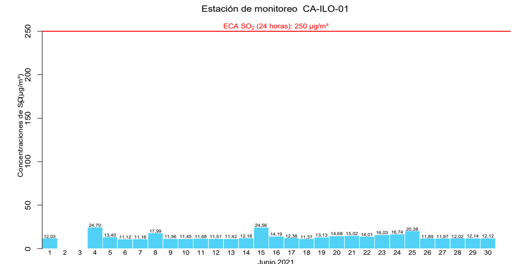
Figura 4.9. Concentraciones de 24 horas de SO 2 en la estación de monitoreo CA-ILO-01, en junio de 2021 7
