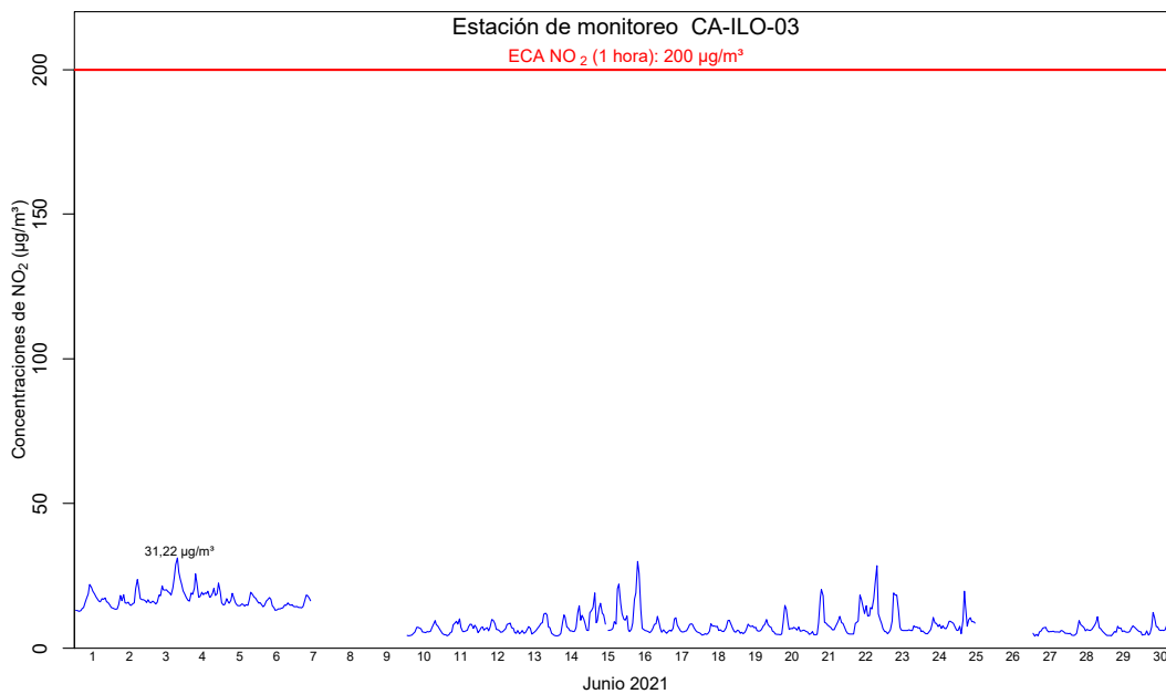
Figura 4.17. Concentraciones de horarias de NO 2 en la estación de monitoreo CA-ILO-03, en junio de 2021 15
