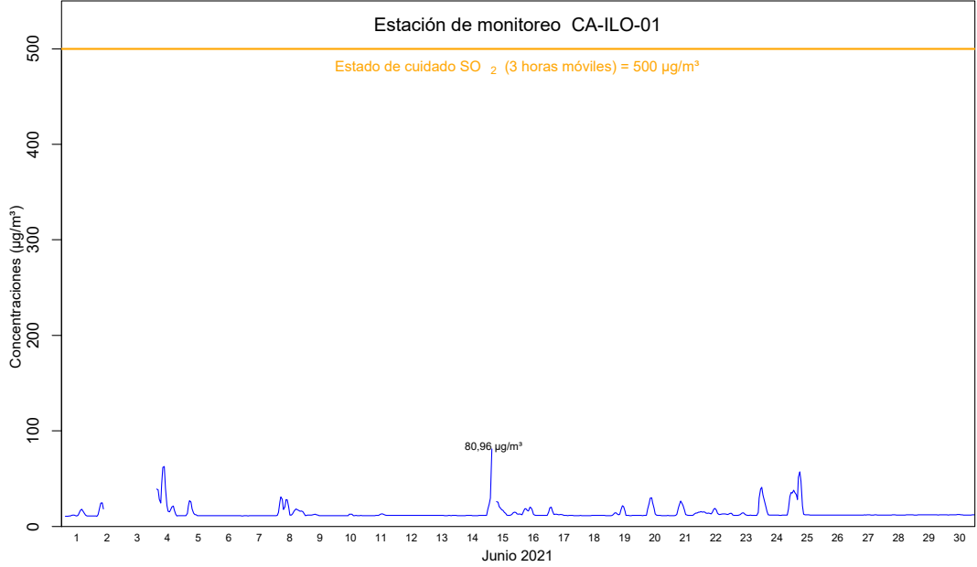
Figura 4.24. Concentraciones de promedio móvil de 3 horas de SO 2 en la estación de monitoreo CA-ILO-01, en junio de 2021 16
