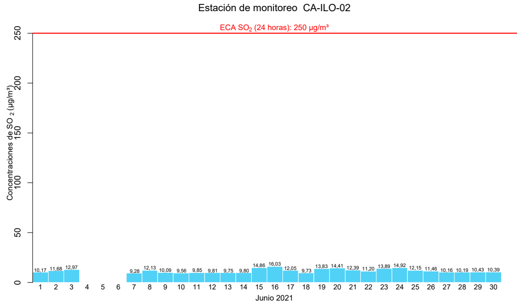
Figura 4.10. Concentraciones de 24 horas de SO 2 en la estación de monitoreo CA-ILO-02, en junio de 2021 8
