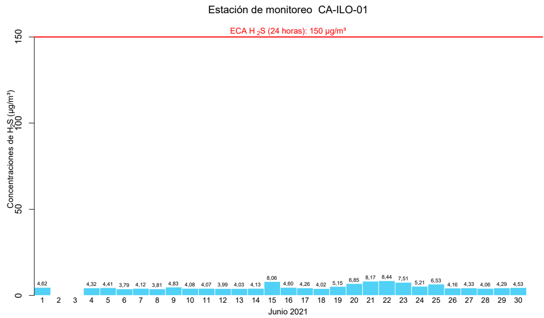
Figura 4.12. Concentraciones de 24 horas de H 2 S en la estación de monitoreo CA-ILO-01, en junio de 2021 10
