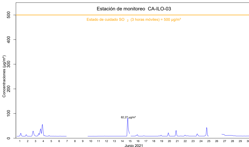
Figura 4.26. Concentraciones de promedio móvil de 3 horas de SO 2 en la estación de monitoreo CA-ILO-03, en junio de 2021 18
