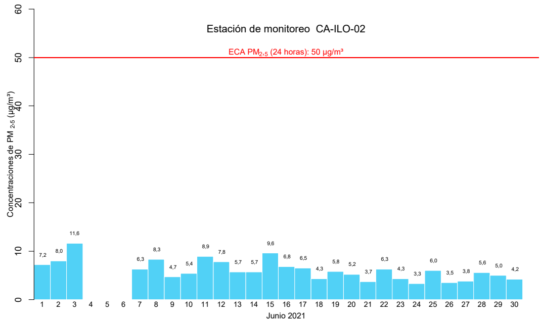
Figura 4.4. Concentraciones de 24 horas de PM 2.5 en la estación de monitoreo CA-ILO-02, en junio de 2021 2
