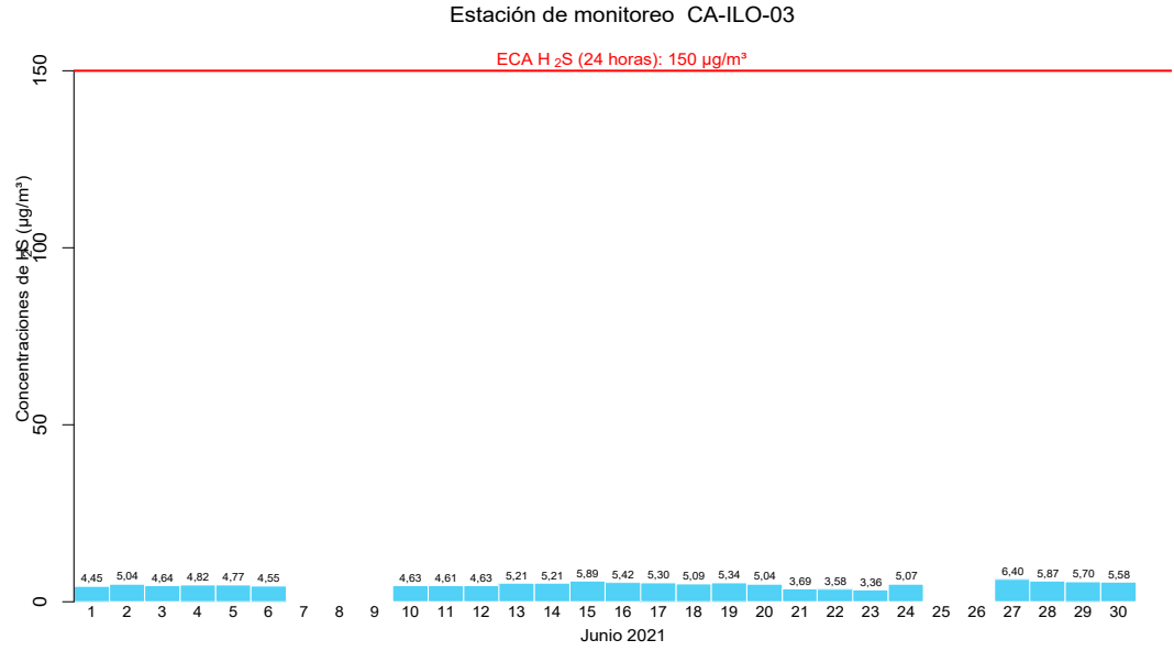
Figura 4.14. Concentraciones de 24 horas de H 2 S en la estación de monitoreo CA-ILO-03, en junio de 2021 12
