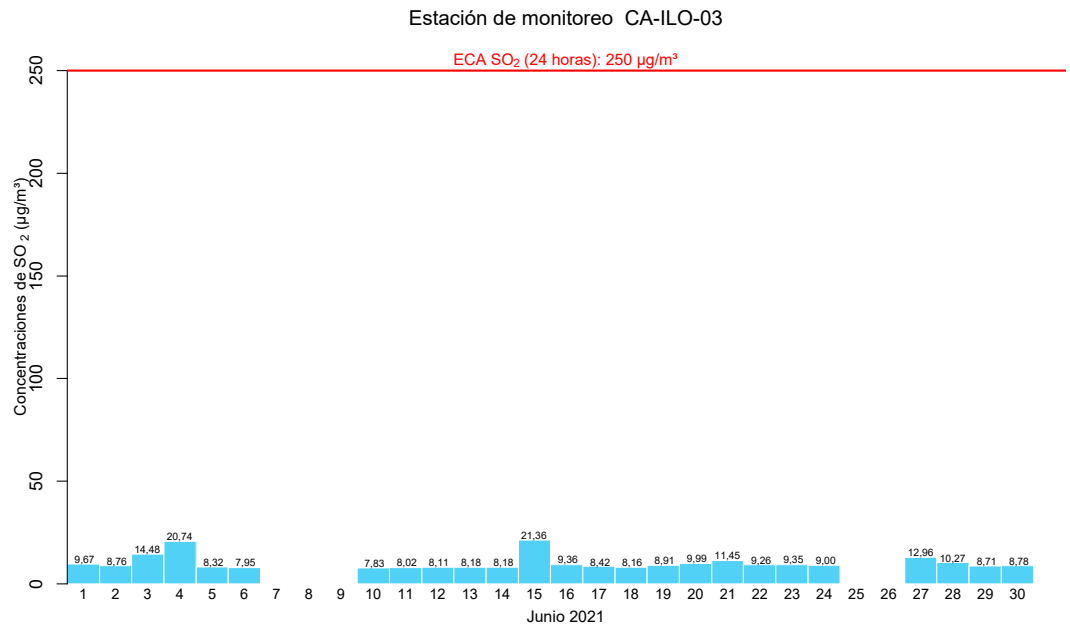
Figura 4.11. Concentraciones de 24 horas de SO 2 en la estación de monitoreo CA-ILO-03, en junio de 2021 9
