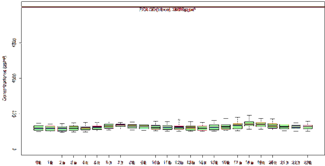
Figura 4.20. Concentraciones de horarias de CO en la estación de monitoreo CA-ILO-03, en junio de 2021
