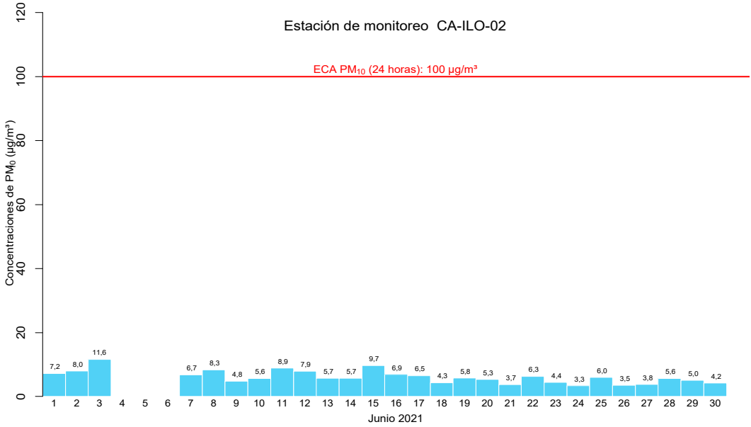
Figura 4.7. Concentraciones de 24 horas de PM 10 en la estación de monitoreo CA-ILO-02, en junio de 2021 5
