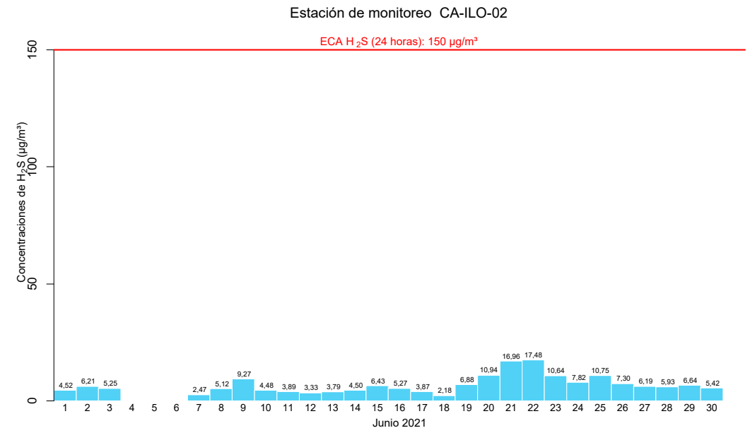
Figura 4.13. Concentraciones de 24 horas de H 2 S en la estación de monitoreo CA-ILO-02, en junio de 2021 11
