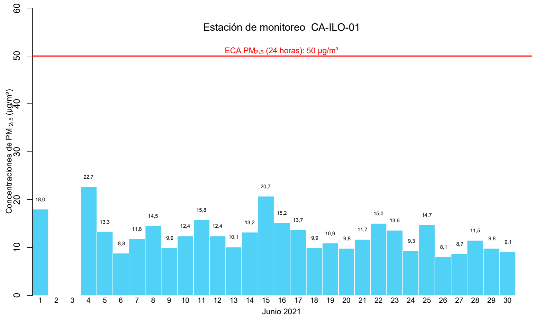
Figura 4.3. Concentraciones de 24 horas de PM 2,5 en la estación de monitoreo CA-ILO-01, en junio de 2021 1
