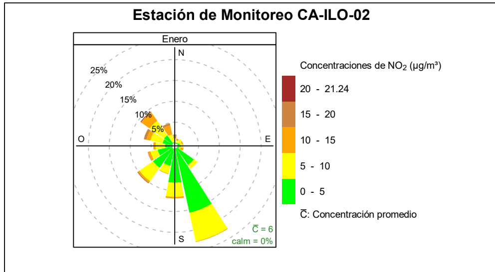
Figura 3.8.9. Rosa de concentración del NO 2 en la estación de monitoreo Ilo - Pacocha (CA-ILO-02), enero de 2025
