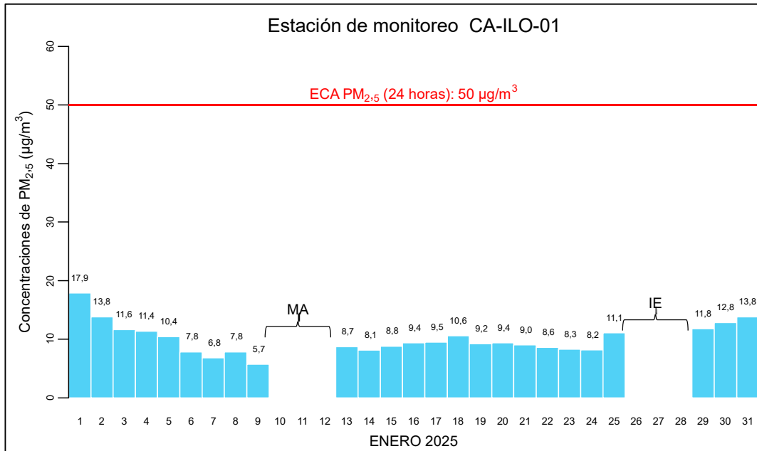
Figura 3.2.1. Concentraciones de 24 horas de PM 2,5 en la estación de monitoreo Ilo – Bolognesi (CA-ILO-01), enero de 2025 MA: Mantenimiento IE: Interrupción eléctrica
