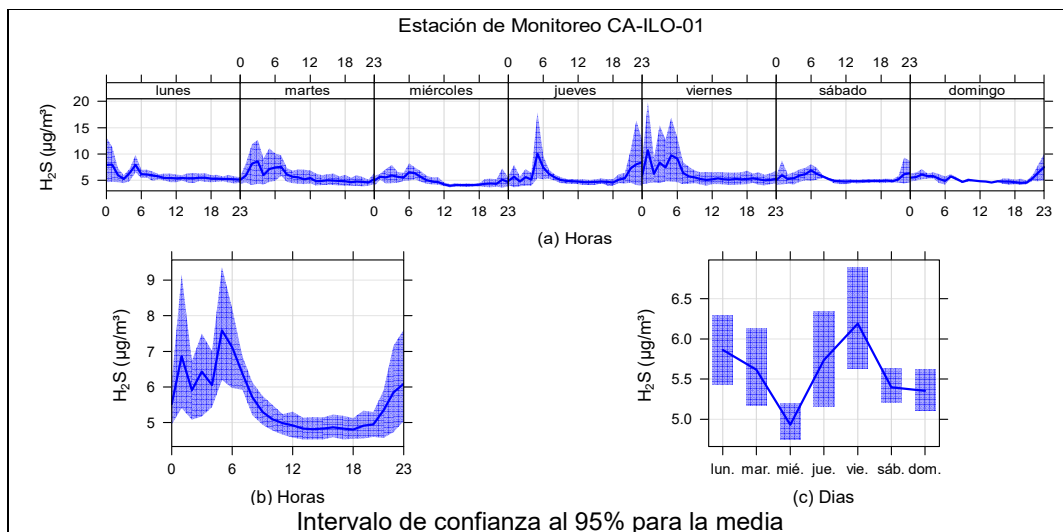
Figura 3.9.7. Concentraciones promedio horarios de H 2 S en la estación de monitoreo Ilo – Bolognesi (CA-ILO-01), de enero de 2025
