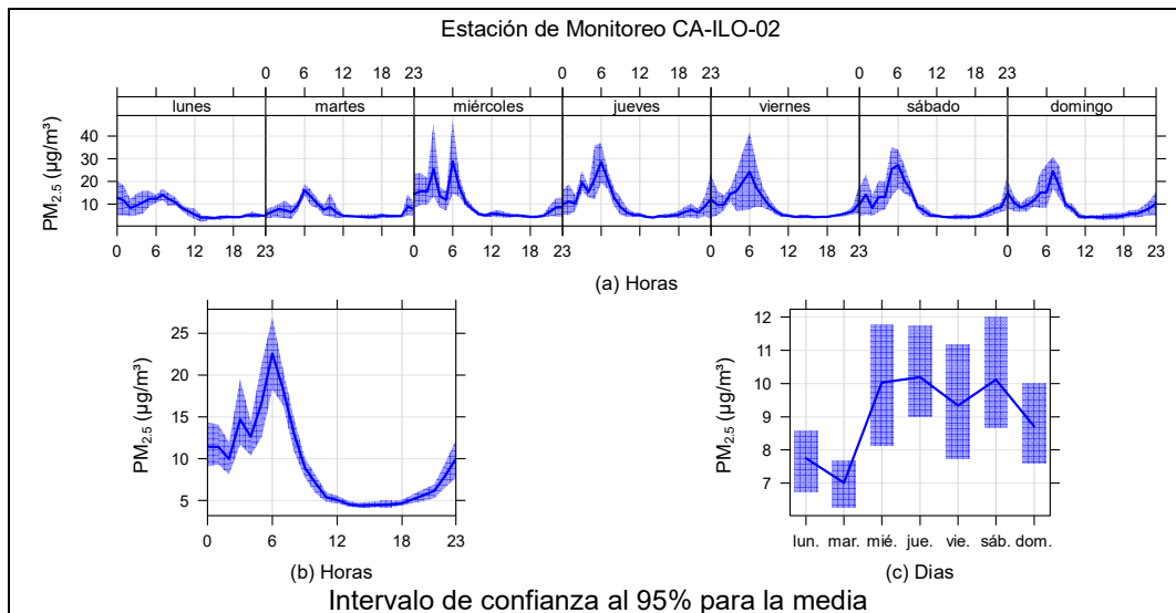
Figura 3.9.2. Concentraciones promedio horarias de PM_{2.5} en la estación de monitoreo Ilo - Pacocha (CA-ILO-02), de enero de 2025
