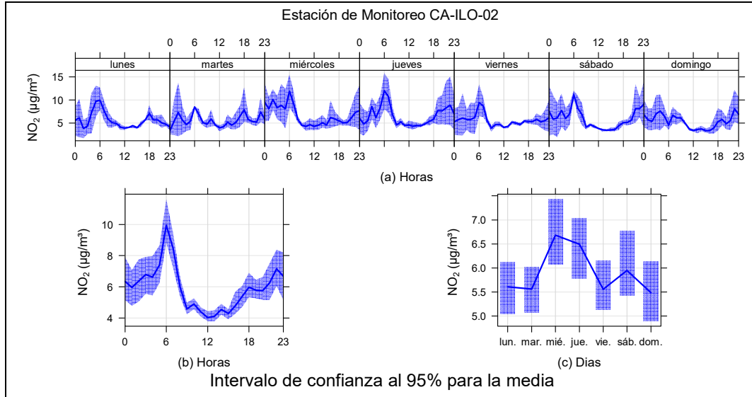
Figura 3.9.10. Concentraciones promedio horarias de \text{NO}_2 en la estación de monitoreo Ilo - Pacocha (CA-ILO-02), de enero de 2025
