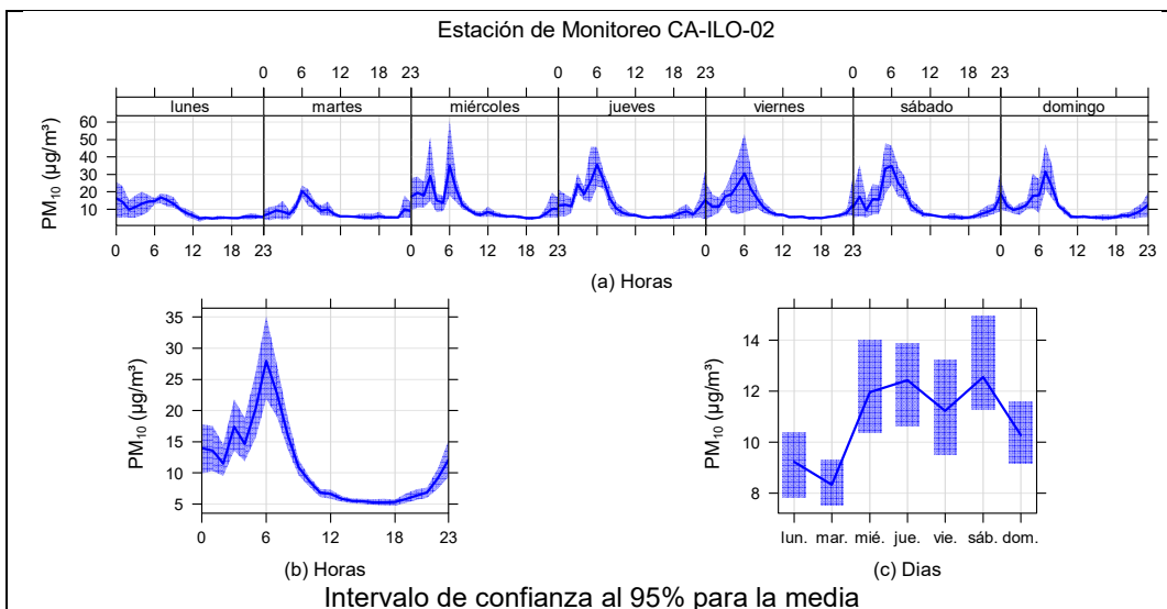
Figura 3.9.4. Concentraciones promedio horarias de PM 10 en la estación de monitoreo Ilo - Pacocha (CA-ILO-02), de enero de 2025
