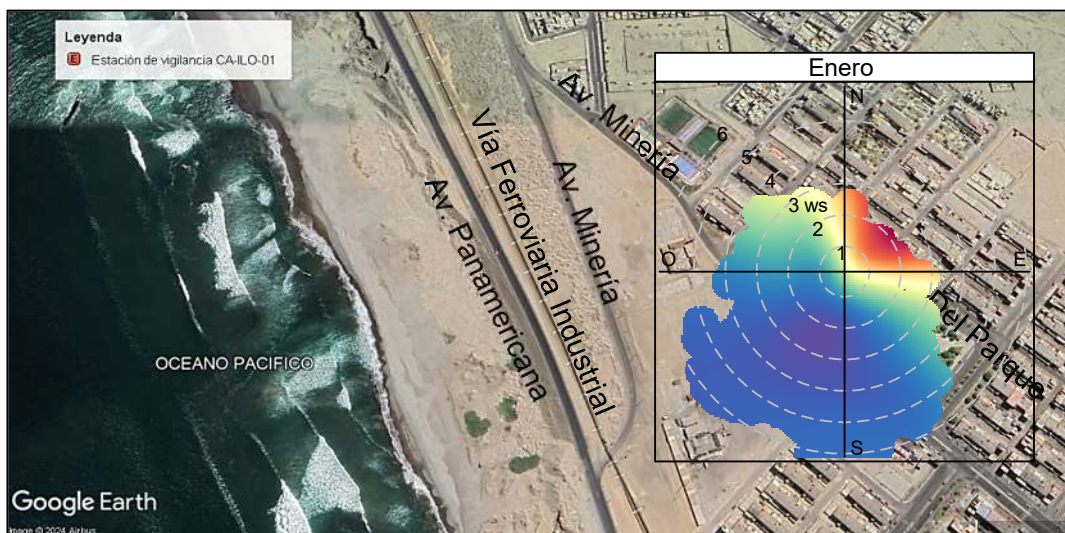
Figura 3.10.2.a Ubicación geográfica de la estación Ilo - Pacocha (CA-ILO-02) respecto a las avenidas principales, mostrando de fondo la gráfica polar correspondiente de la relación geométrica SO_2/NO_x , enero de 2025.
