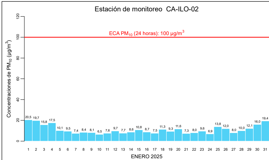
Figura 3.3.2. Concentraciones de 24 horas de PM 10 en la estación de monitoreo Ilo – Pacocha (CA-ILO-02), enero de 2025
