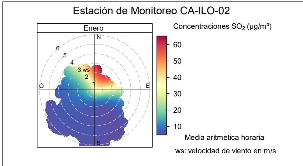
Figura 3.10.1. Gráfica polar de las concentraciones promedio de SO 2 en la estación de monitoreo Ilo - Pacocha (CA-ILO-02), enero de 2025
