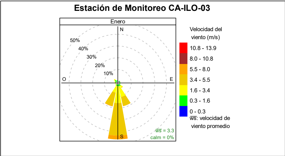
Figura 3.1.3. Rosa de viento de la estación de monitoreo Ilo - José Pardo (CA-ILO-03), enero de 2025 6
