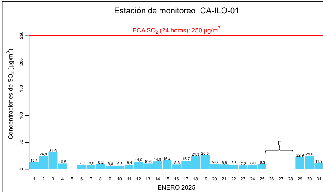
Figura 3.4.1. Concentraciones de 24 horas de SO 2 en la estación de monitoreo Ilo – Bolognesi (CA-ILO-01), enero de 2025 IE: Interrupción eléctrica
