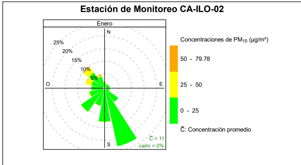
Figura 3.8.3. Rosa de concentración del PM 10 en la estación de monitoreo Ilo - Pacocha (CA-ILO-02), enero de 2025
