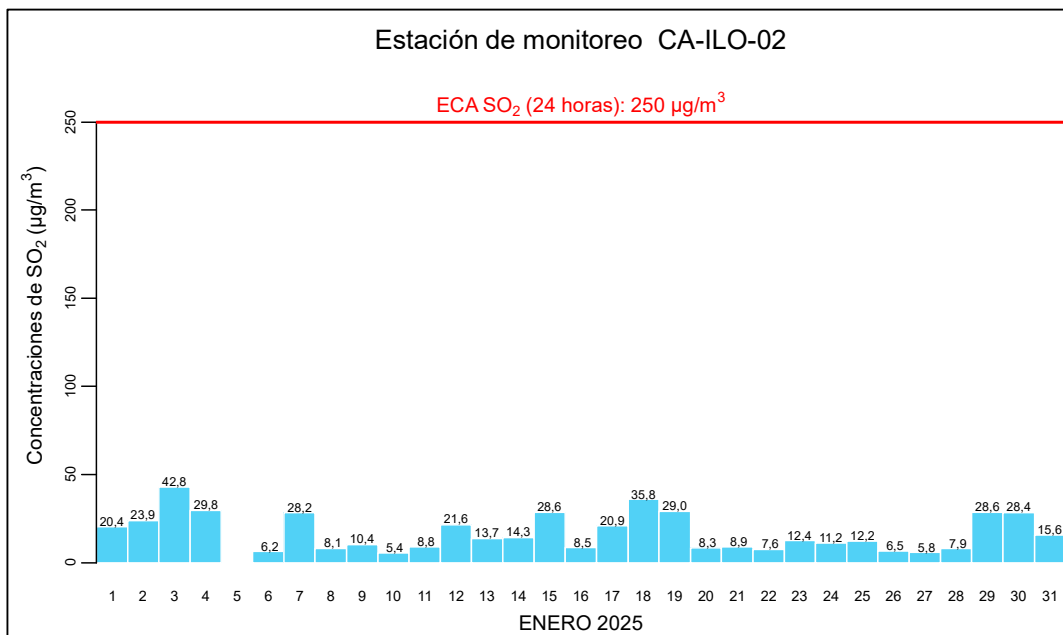
Figura 3.4.2. Concentraciones de 24 horas de SO 2 en la estación de monitoreo Ilo - Pacocha (CA-ILO-02), enero de 2025
