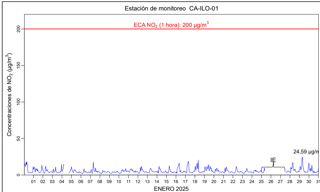
Figura 3.6.1. Concentraciones de horarias de NO 2 en la estación de monitoreo Ilo – Bolognesi (CA-ILO-01), enero de 2025.
