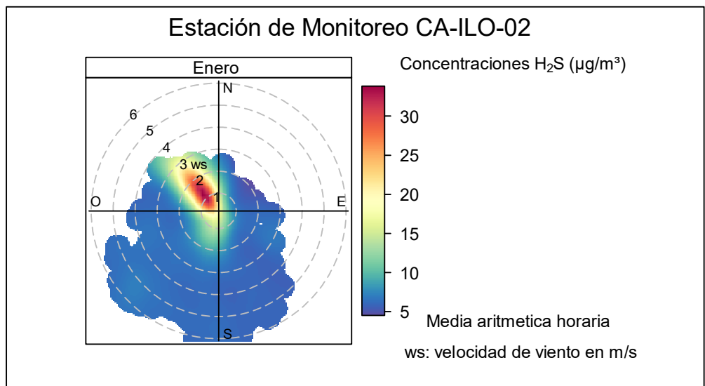
Figura 3.10.3. Gráfica polar de las concentraciones promedios de H 2 S en la estación de monitoreo Ilo - Pacocha (CA-ILO-02), enero de 2025
