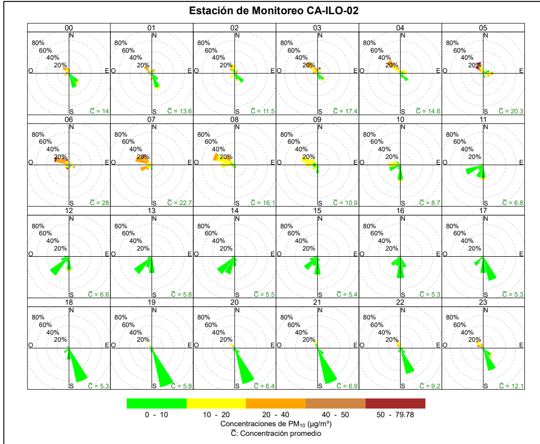
Figura 3.8.4. Rosa de concentración horaria del PM 10 en la estación de monitoreo Ilo - Pacocha (CA-ILO-02), enero de 2025
