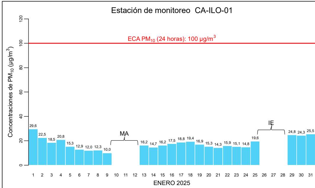
Figura 3.3.1. Concentraciones de 24 horas de PM 10 en la estación de monitoreo Ilo – Bolognesi (CA-ILO-01), enero de 2025
