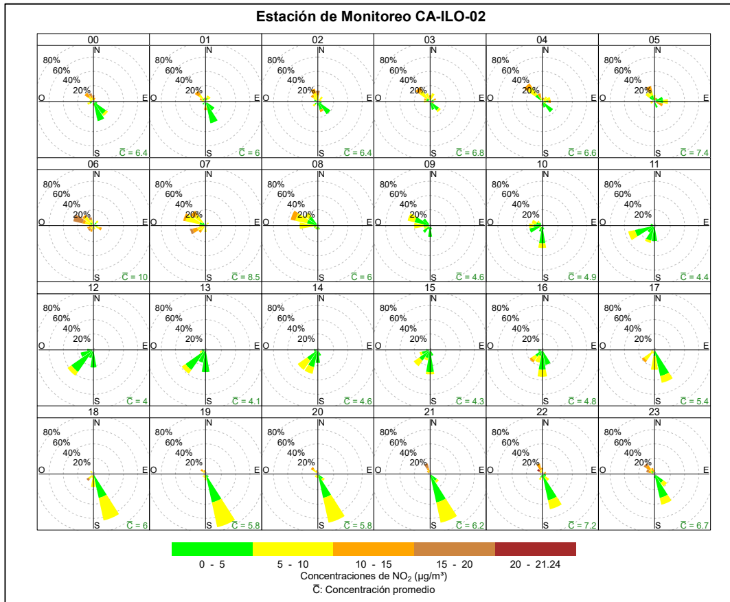
Figura 3.8.10. Rosa de concentración horaria del NO 2 en la estación de monitoreo Ilo - Pacocha (CA-ILO-02), enero de 2025
