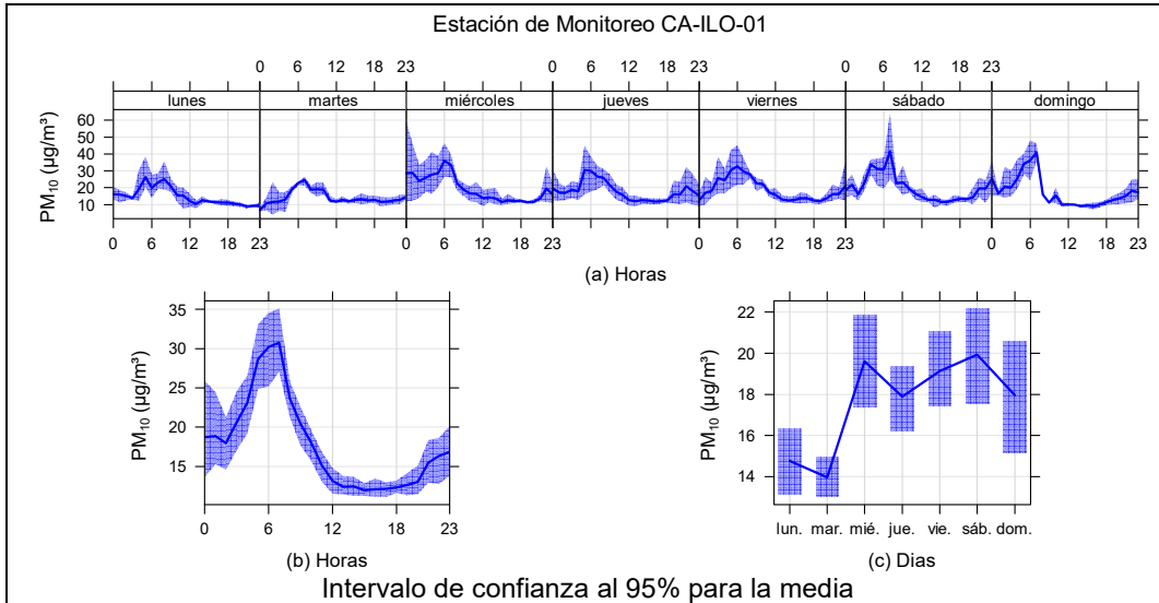
Figura 3.9.3. Concentraciones promedio horarias de PM 10 en la estación de monitoreo Ilo – Bolognesi (CA-ILO-01), de enero de 2025
