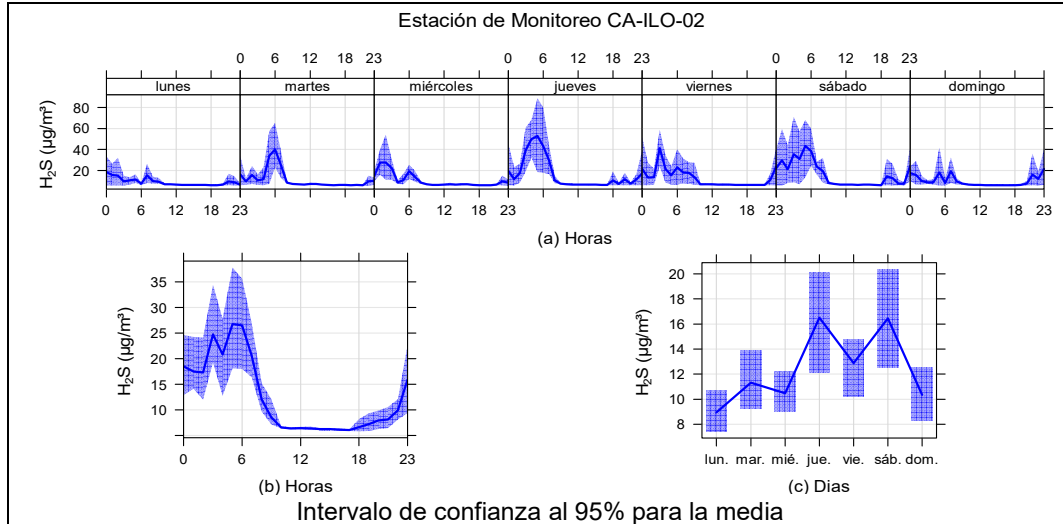
Figura 3.9.8. Concentraciones promedio horarias de H 2 S en la estación de monitoreo Ilo - Pacocha (CA-ILO-02), de enero de 2025
