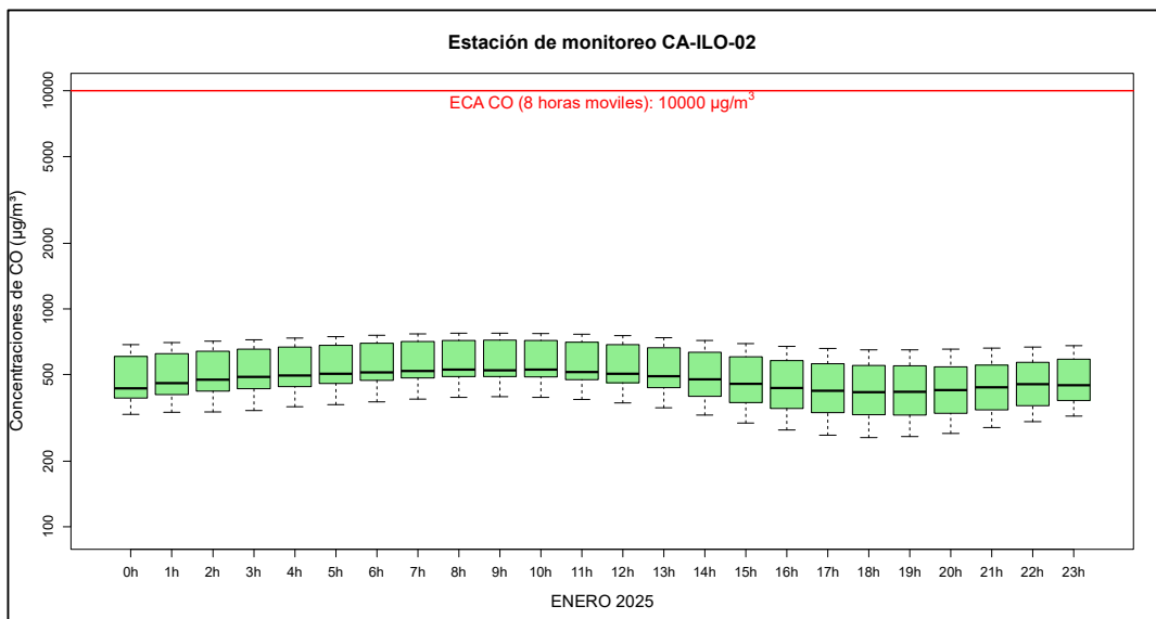
Figura 3.7.2. Concentraciones de promedio móvil de 8 horas de CO en la estación de monitoreo Ilo - Pacocha (CA-ILO-02), enero de 2025
