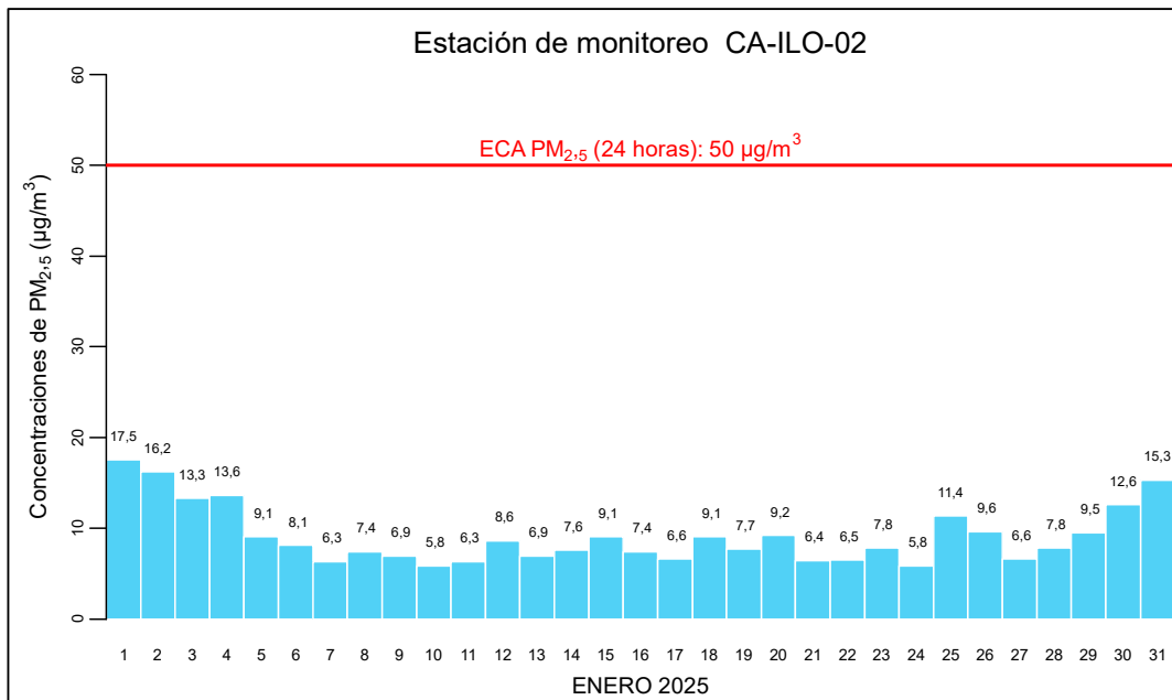
Figura 3.2.2. Concentraciones de 24 horas de PM 2,5 en la estación de monitoreo Ilo – Pacocha (CA-ILO-02), enero de 2025
