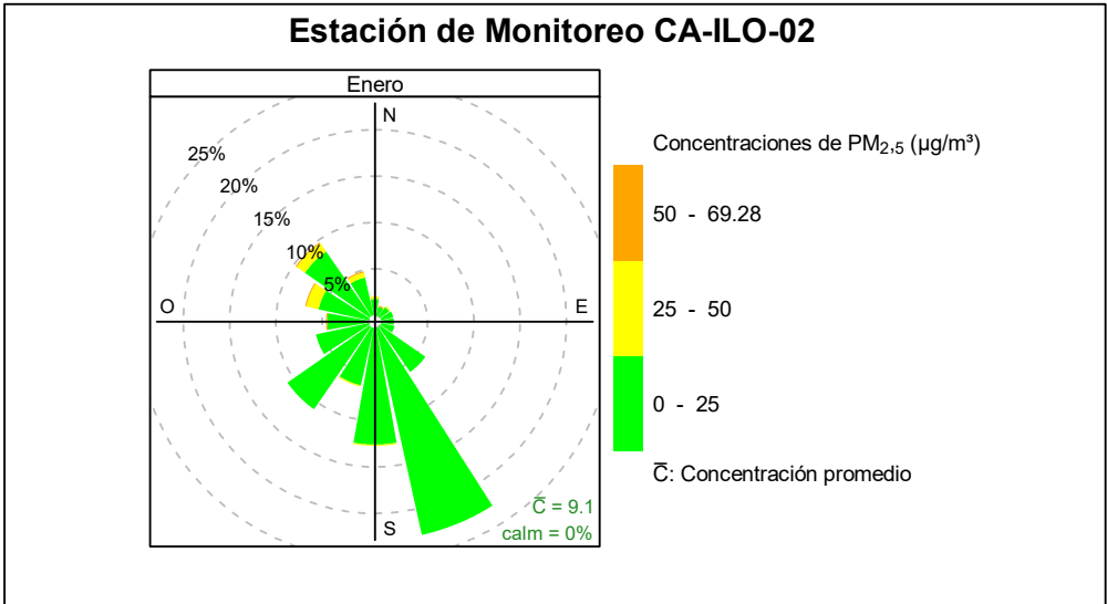
Figura 3.8.1. Rosa de concentración del PM 2,5 en la estación de monitoreo Ilo - Pacocha (CA-ILO-02), enero del 2025
