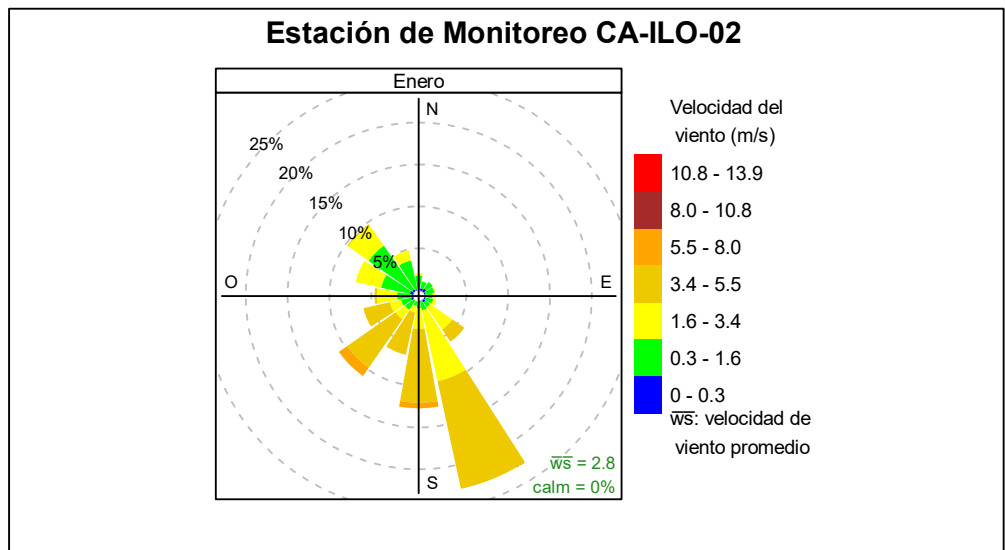
Figura 3.1.1. Rosa de viento de la estación de monitoreo Ilo - Pacocha (CA-ILO-02), enero de 2025 4
