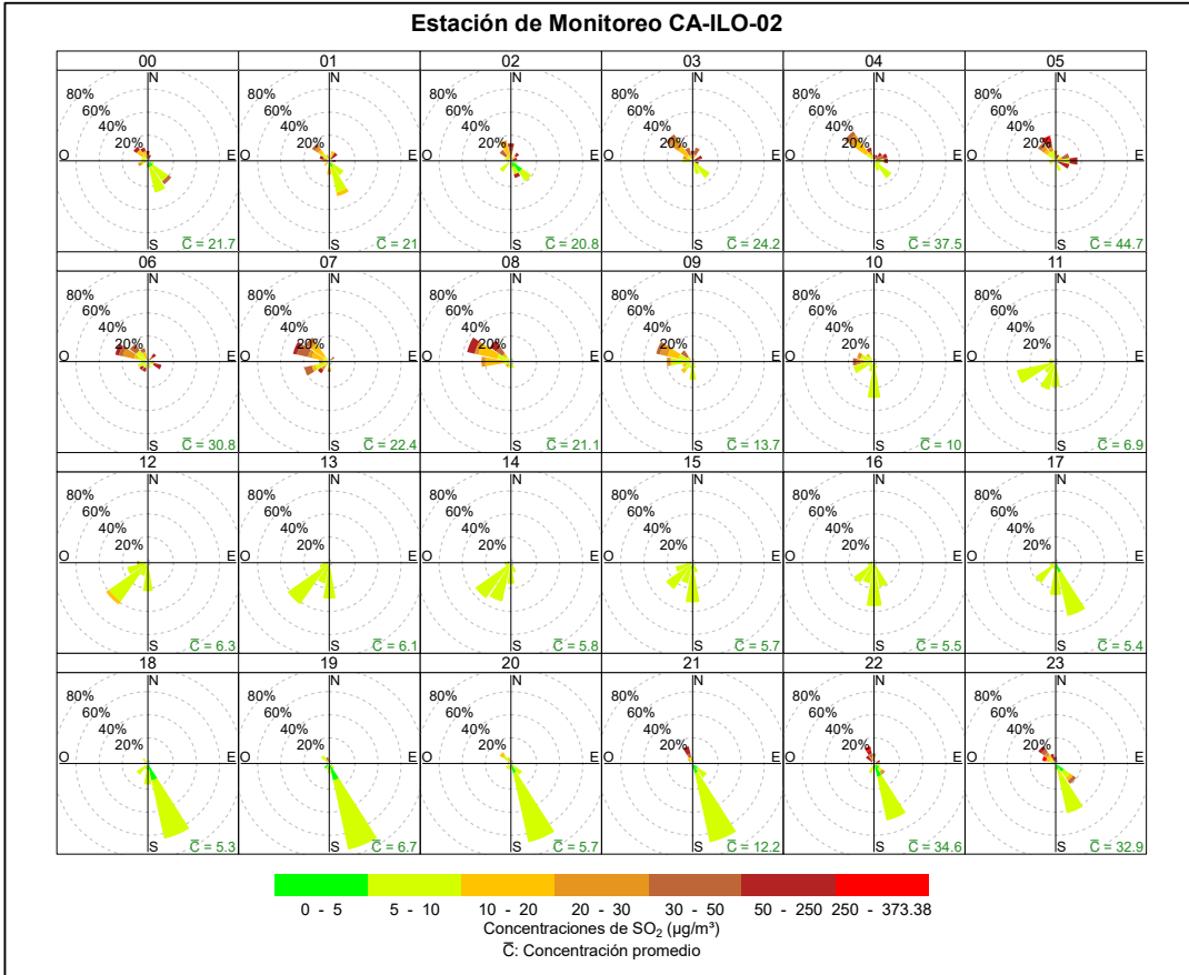
Figura 3.8.6. Rosa de concentración horaria del SO 2 en la estación de monitoreo Ilo - Pacocha (CA-ILO-02), enero de 2025
