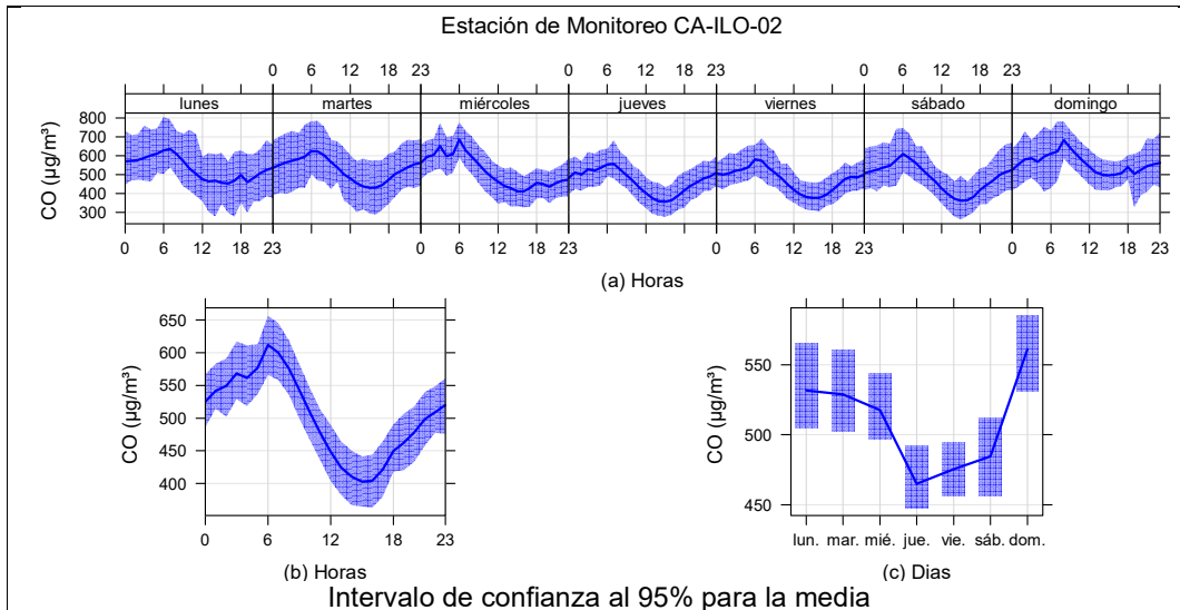
Figura 3.9.11. Concentraciones promedio horarias de CO en la estación de monitoreo Ilo - Pacocha (CA-ILO-02), de enero de 2025
