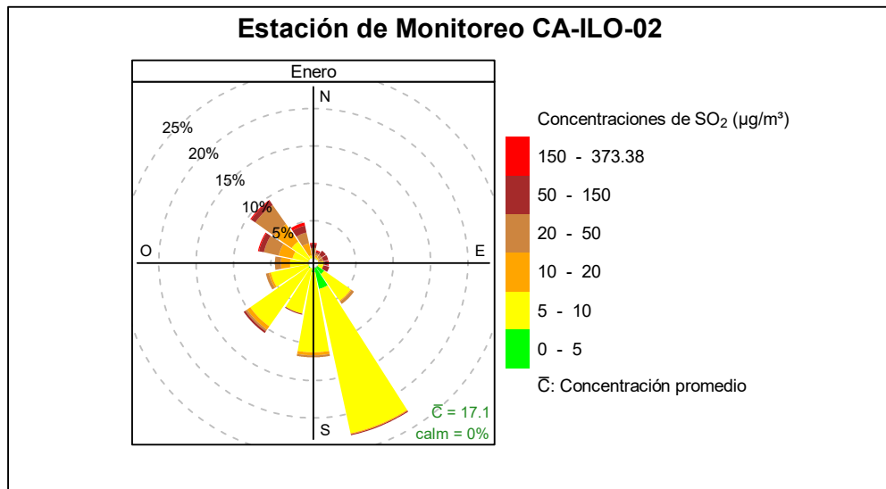
Figura 3.8.5. Rosa de concentración del SO 2 en la estación de monitoreo Ilo - Pacocha (CA-ILO-02), enero de 2025
