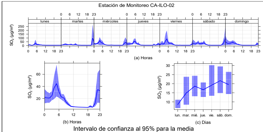
Figura 3.9.6. Concentraciones promedio horarios de SO 2 en la estación de monitoreo Ilo - Pacocha (CA-ILO-02), de enero de 2025.
