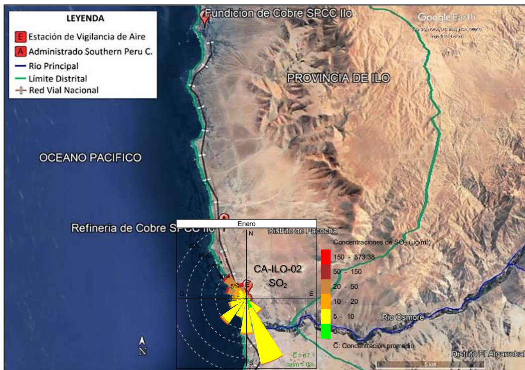
Figura 3.8.5.a. Ubicación de la estación Ilo - Pacocha (CA-ILO-02) respecto al administrado Southern Peru Copper Corporation
