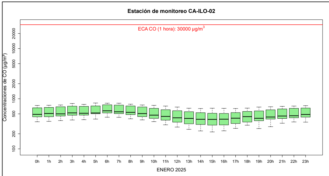
Figura 3.7.1. Concentraciones horarias de CO en la estación de monitoreo Ilo - Pacocha (CA-ILO-02), enero de 2025
