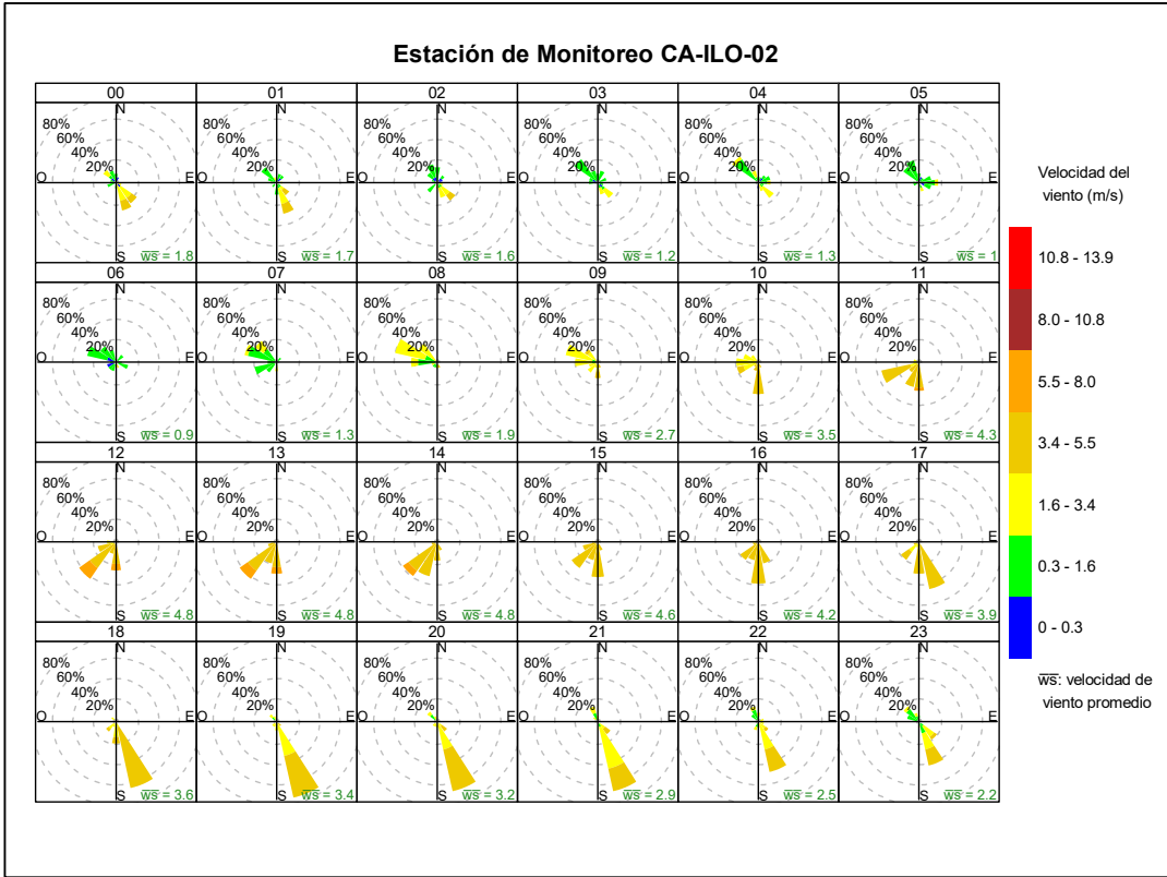
Figura 3.1.2. Rosa de viento horaria de la estación de monitoreo Ilo - Pacocha (CA-ILO-02), enero de 2025
