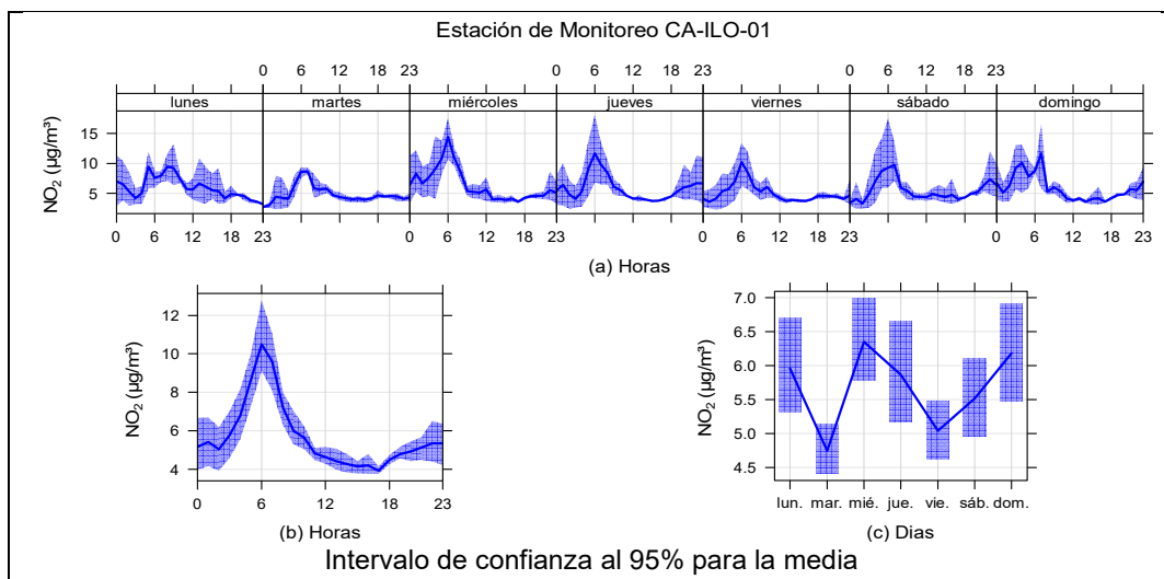
Figura 3.9.9. Concentraciones promedio horarias de NO 2 en la estación de monitoreo Ilo – Bolognesi (CA-ILO-01), de enero de 2025
