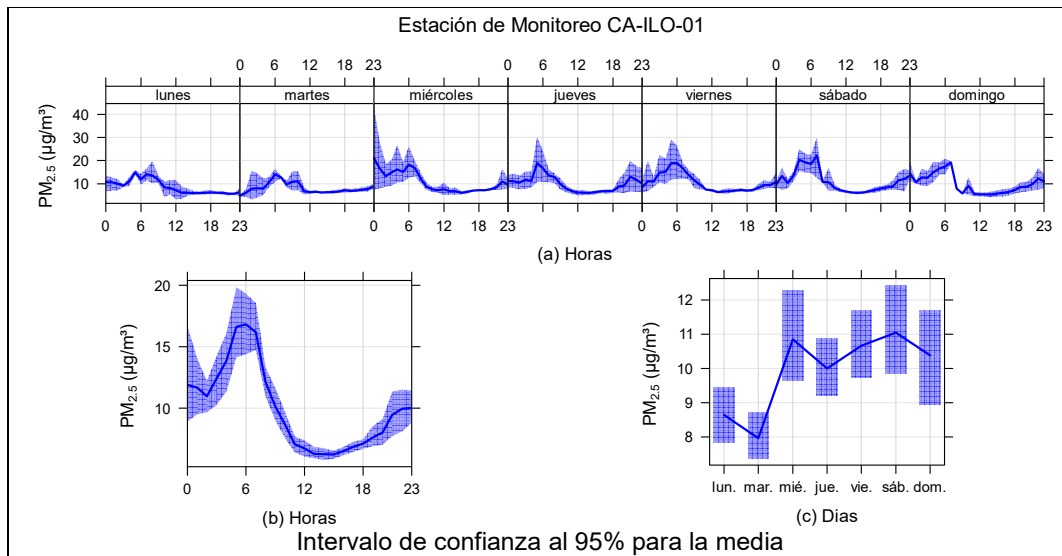
Figura 3.9.1. Concentraciones promedio horarias de PM_{2.5} en la estación de monitoreo Ilo – Bolognesi (CA-ILO-01), de enero de 2025
