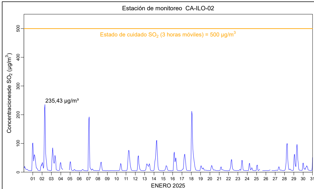
Figura 3.11.2. Concentraciones de promedio móvil de 3 horas de \text{SO}_2 en la estación de monitoreo Ilo - Pacocha (CA-ILO-02), en enero de 2025
