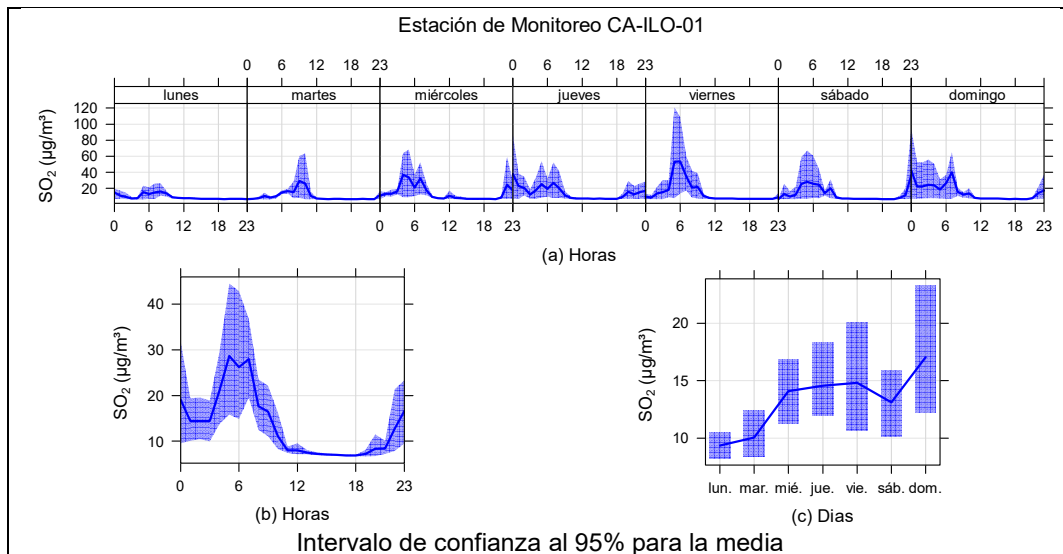
Figura 3.9.5. Concentraciones promedio horarios de SO 2 en la estación de monitoreo Ilo – Bolognesi (CA-ILO-01), de enero de 2025
