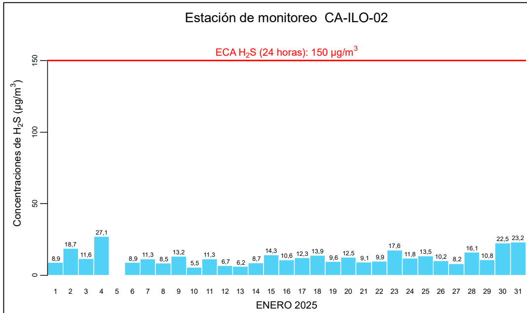
Figura 3.5.2. Concentraciones de 24 horas de H 2 S en la estación de monitoreo Ilo - Pacocha (CA-ILO-02), enero de 2025
