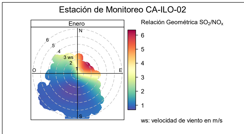
Figura 3.10.2. Gráfica polar de la relación geométrica SO_2/NO_x en la estación de monitoreo Ilo - Pacocha (CA-ILO-02), enero de 2025
