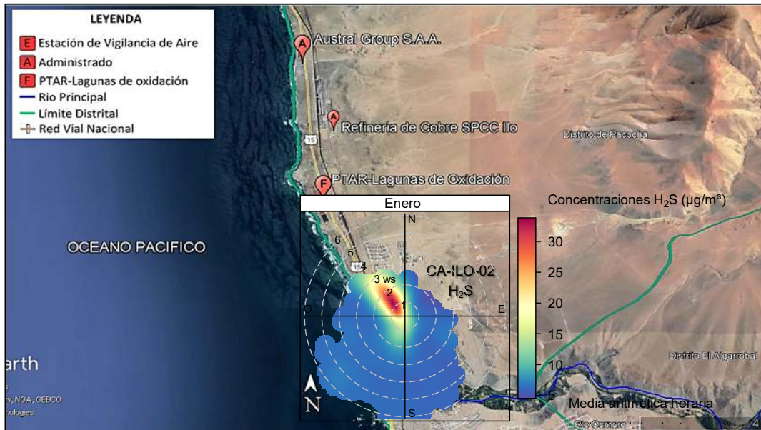
Figura 3.10.3.a Ubicación geográfica de la estación Ilo - Pacocha (CA-ILO-02) respecto a la fábrica de harina de pescado Austral Group S.A.A., mostrando la gráfica polar correspondiente de las concentraciones de H 2 S, enero de 2025.
