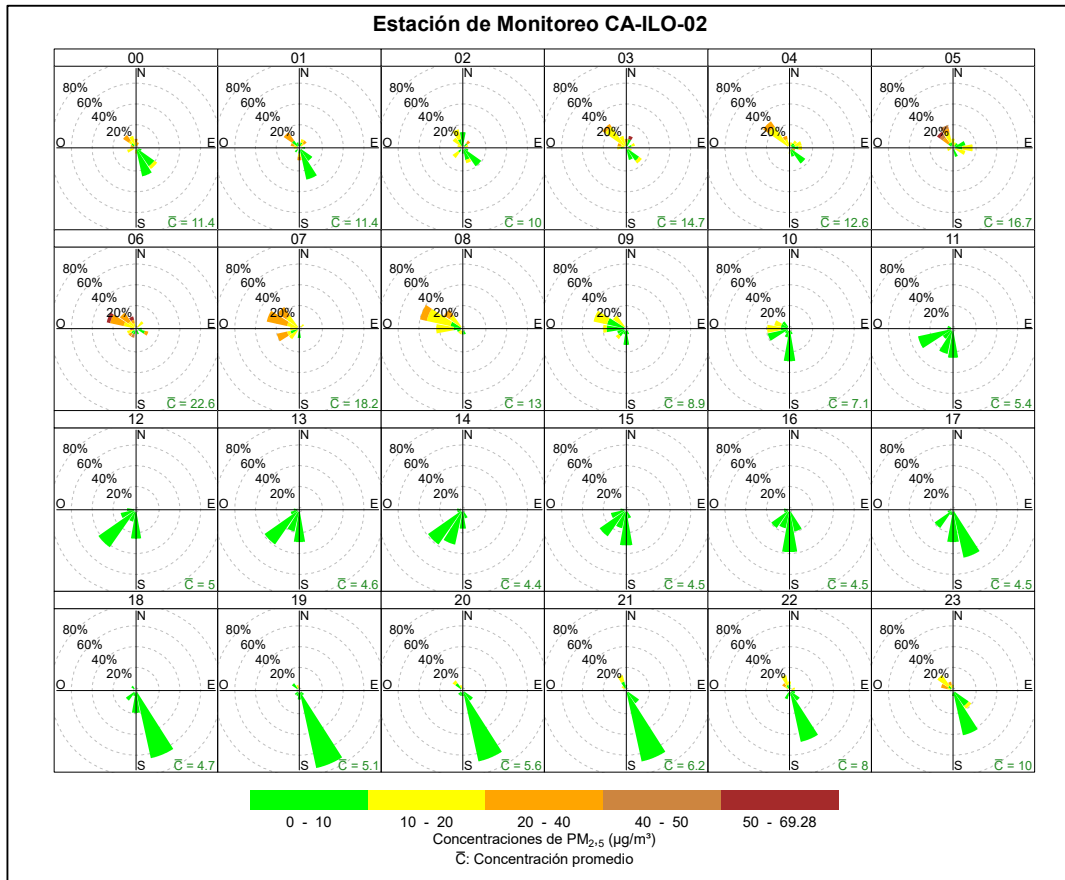
Figura 3.8.2. Rosa de concentración horaria del PM 2.5 en la estación de monitoreo Ilo - Pacocha (CA-ILO-02), enero de 2025
