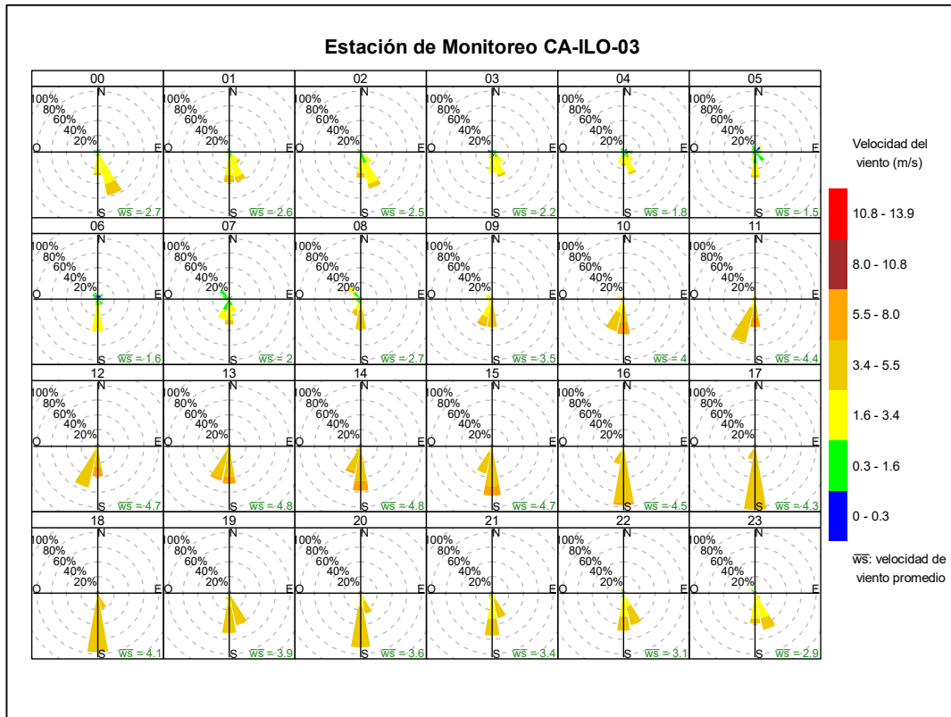
Figura 3.1.4. Rosa de viento horaria de la estación de monitoreo Ilo - José Pardo (CA-ILO-03), enero de 2025
