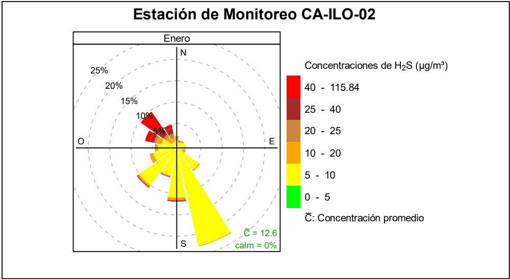
Figura 3.8.7. Rosa de concentración del H 2 S en la estación de monitoreo Ilo - Pacocha (CA-ILO-02), enero de 2025
