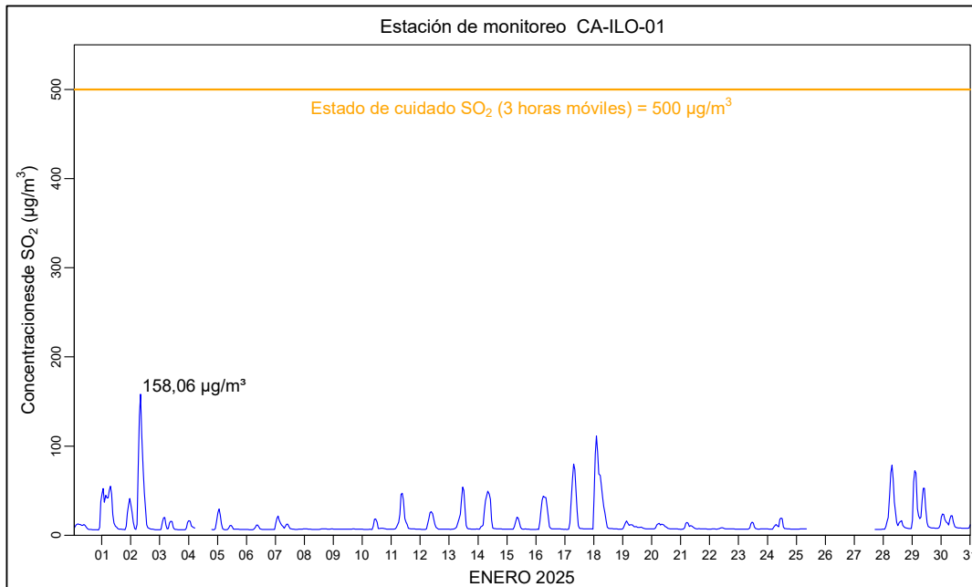
Figura 3.11.1. Concentraciones de promedio móvil de 3 horas de SO 2 en la estación de monitoreo Ilo – Bolognesi (CA-ILO-01), en enero de 2025
