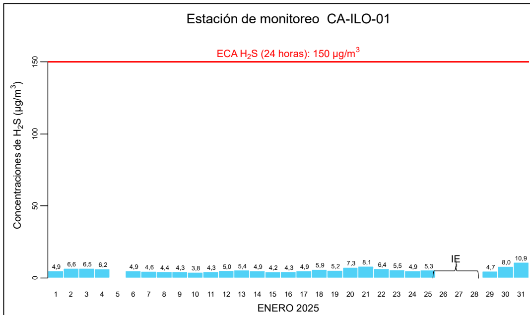
Figura 3.5.1. Concentraciones de 24 horas de H 2 S en la estación de monitoreo Ilo – Bolognesi (CA-ILO-01), enero de 2025 IE: Interrupción eléctrica
