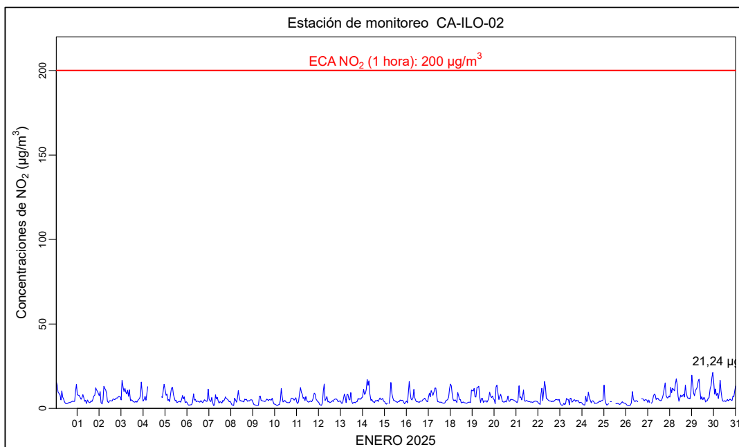
Figura 3.6.2. Concentraciones de horarias de NO 2 en la estación de monitoreo Ilo - Pacocha (CA-ILO-02), enero de 2025.
