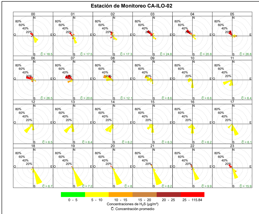
Figura 3.8.8. Rosa de concentración horaria del H 2 S en la estación de monitoreo Ilo - Pacocha (CA-ILO-02), enero de 2025
