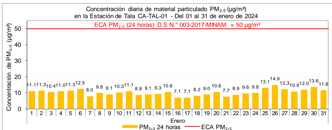
Figura 3.8. Concentración de 24 horas de PM_{2,5} en la estación de Tala, 1 al 31 de enero de 2024.
