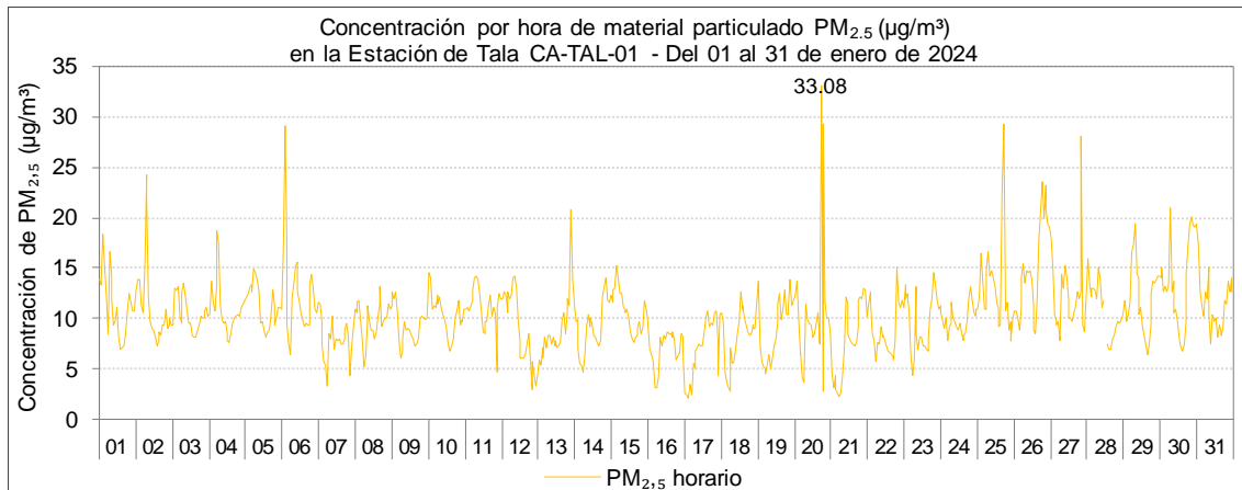
Figura 3.6. Concentración hora de PM 2.5 en la estación de Tala, del 1 al 31 de enero de 2024
