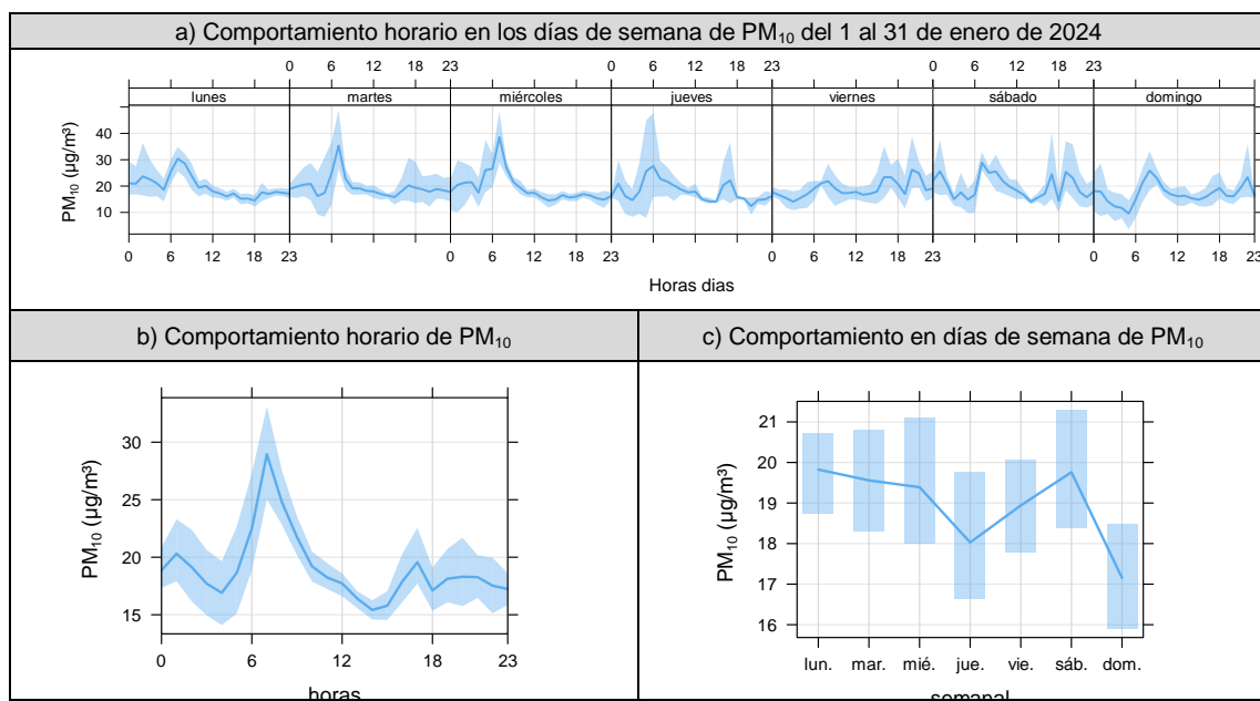
Figura 3.3. Concentraciones promedio (a) horario y por días de la semana, b) horario y c) por días de la semana de PM 10 en la estación de monitoreo CA-TAL-01 (ubicada en Tala), del mes de enero de 2024
