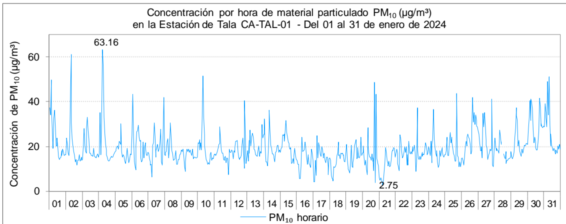
Figura 3.2. Concentración hora de PM 10 en la estación de Tala, del 1 al 31 de enero de 2024
