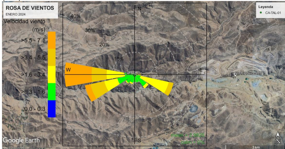
Figura 3.1. Rosa de vientos de la estación de monitoreo CA-TAL-01 (ubicada en Tala), del mes de enero de 2024
