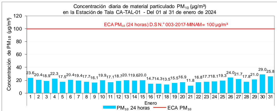
Figura 3.4. Concentración de 24 horas de PM 10 en estación de Tala, 1 al 31 de enero de 2024.
