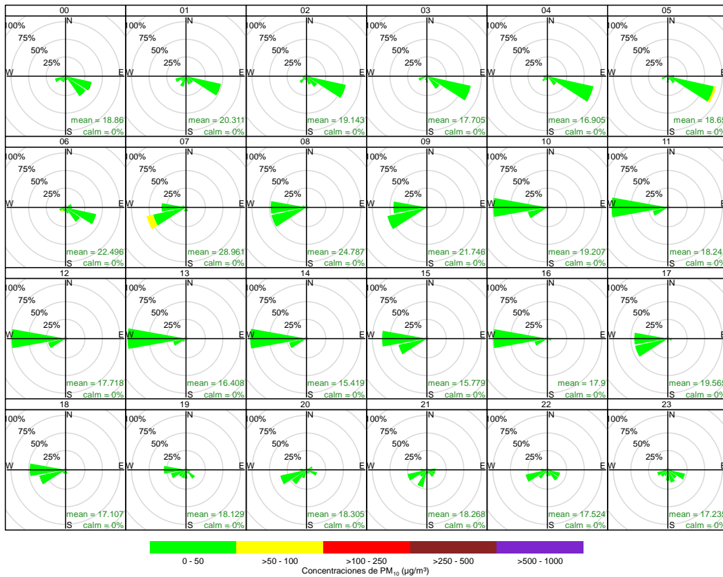
Figura 3.5. Rosas de concentración por horas para el PM 10 , de las 00:00 hasta las 23:00 horas, del mes de enero de 2024.
