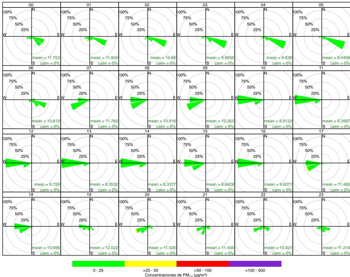
Figura 3.9. Rosas de concentración por horas para PM_{2.5} , de 00:00 a 23:00 horas, enero de 2024
