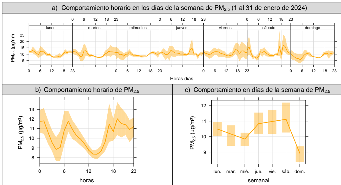
Figura 3.7. Concentraciones promedio (a) horario y por días de la semana, b) horario y c) por días de la semana de PM_{2,5} en la estación de monitoreo CA-TAL-01 (ubicada en Tala), del mes de enero de 2024.
