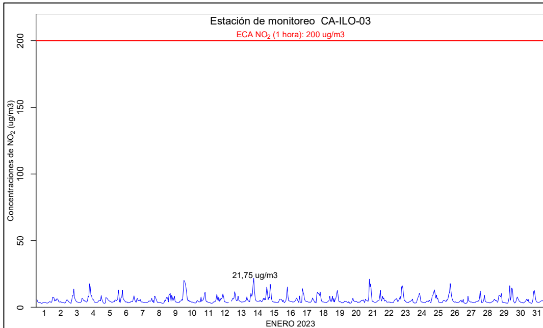
Figura 3.6.3. Concentraciones de horarias de NO 2 en la estación de monitoreo CA-ILO-03, enero de 2023.
