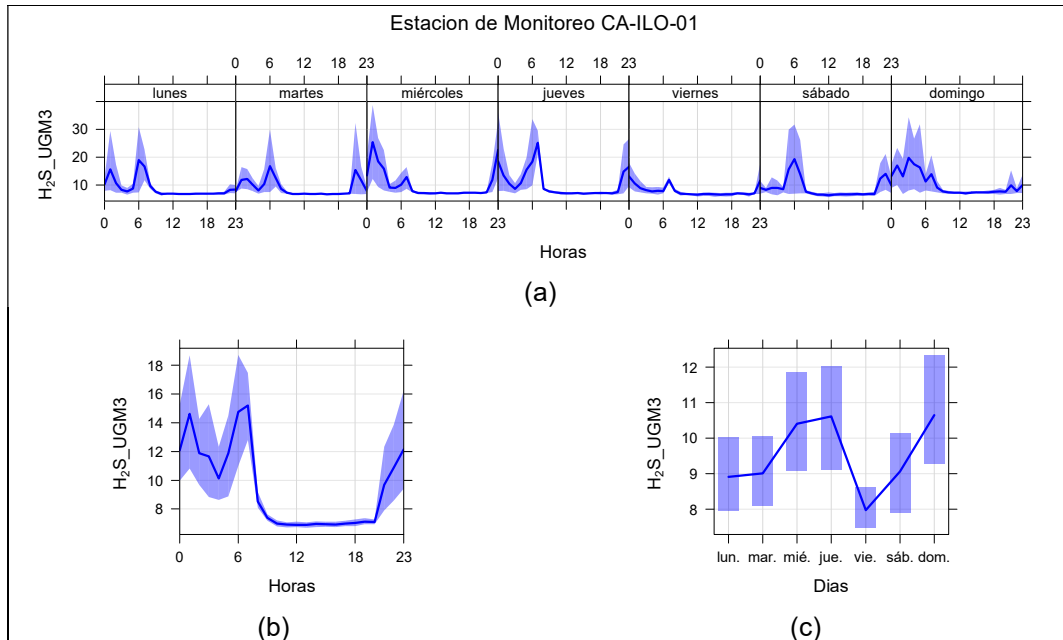
Figura 3.9.8. Concentraciones promedio horarios de H 2 S en la estación de monitoreo CA-ILO-01, de enero de 2023
