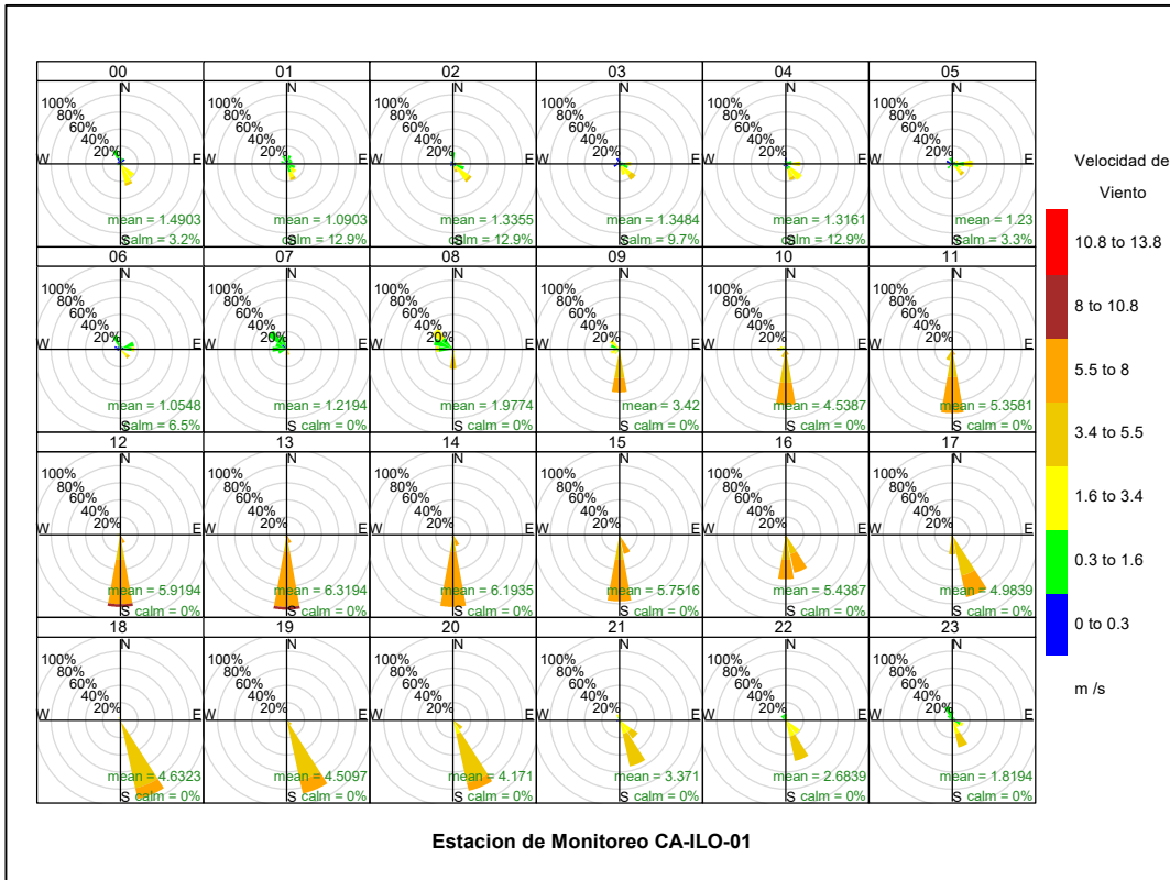
Figura 3.1.3. Rosa de viento horaria de la estación de monitoreo CA-ILO-01, enero de 2023
