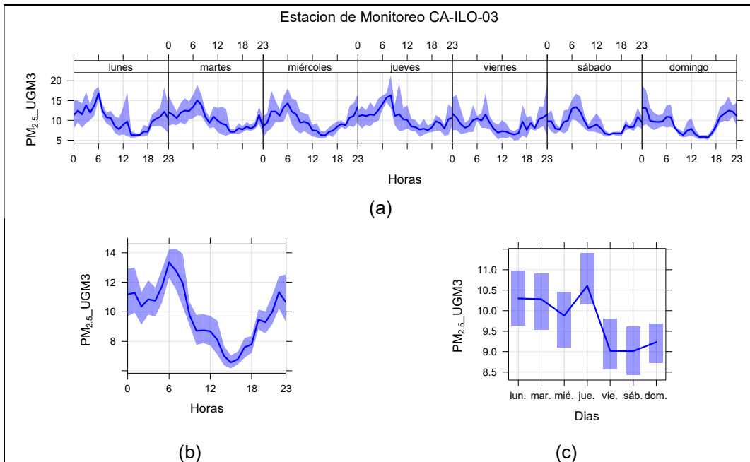
Figura 3.9.2. Concentraciones promedio horarios de PM_{2.5} en la estación de monitoreo CA-ILO-03, de enero de 2023
