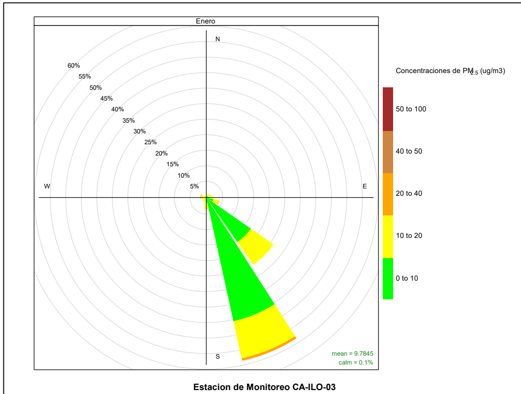
Figura 3.8.2. Rosa de concentración del PM_{2.5} en la estación de monitoreo CA-ILO-03, enero de 2023
