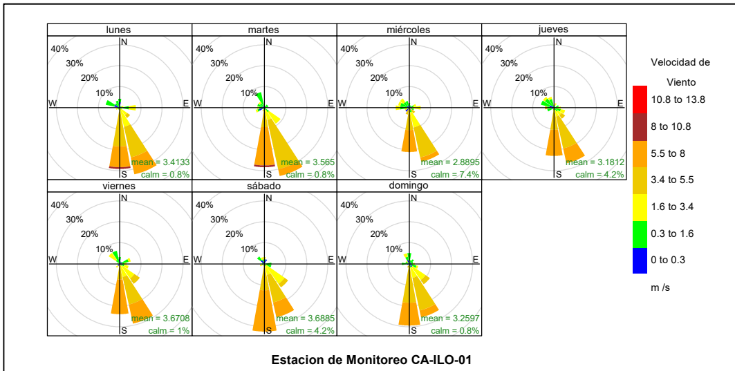
Figura 3.1.2. Rosa de viento por días de la semana de la estación de monitoreo CA-ILO-01, enero de 2023
