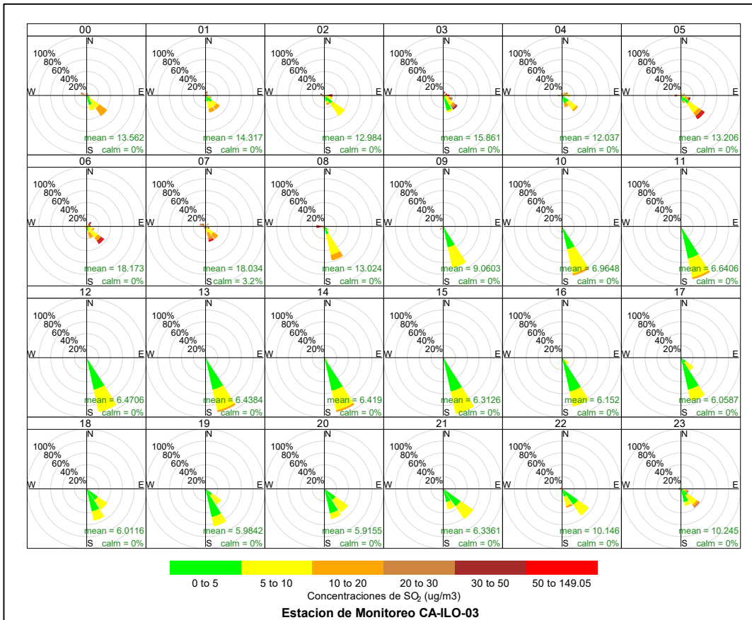
Figura 3.8.14. Rosa de concentración horaria del SO 2 en la estación de monitoreo CA-ILO-03, enero de 2023
