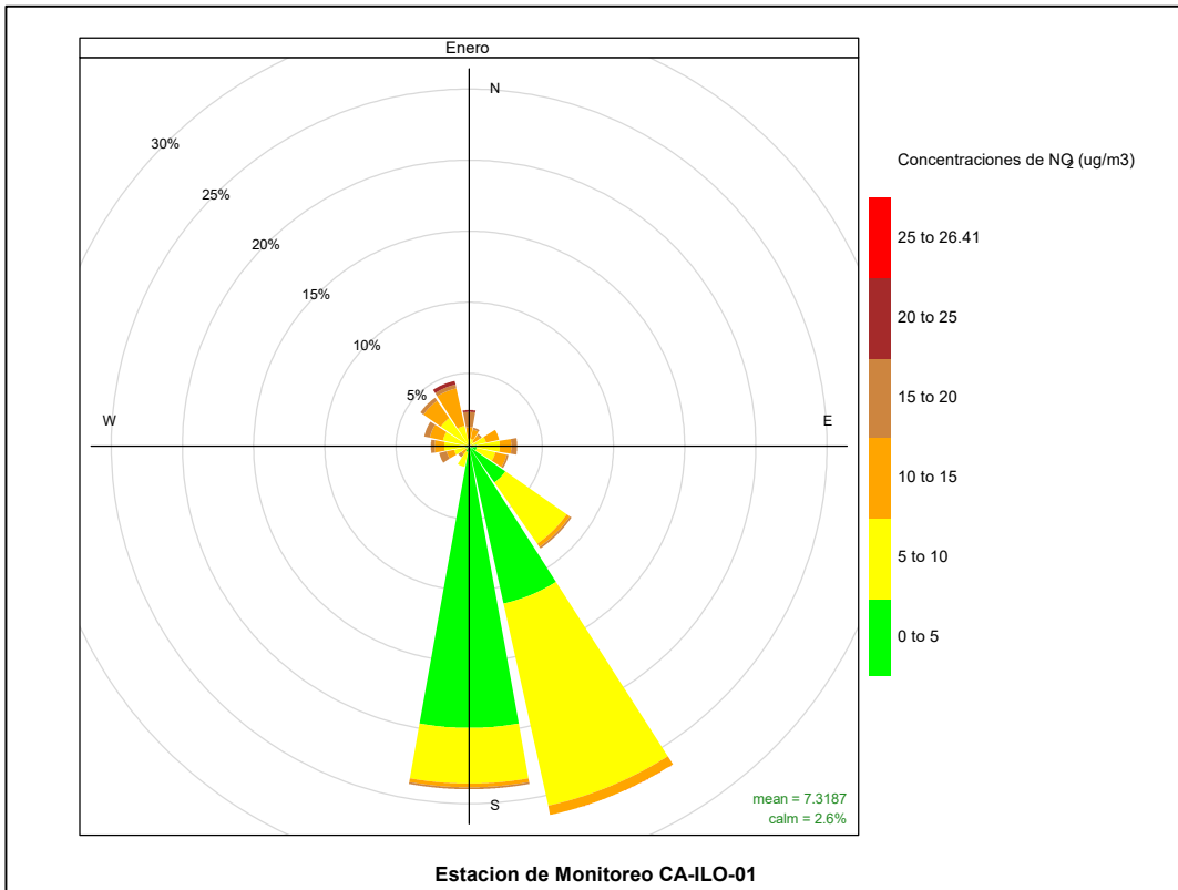
Figura 3.8.21. Rosa de concentración del NO 2 en la estación de monitoreo CA-ILO-01, enero de 2023
