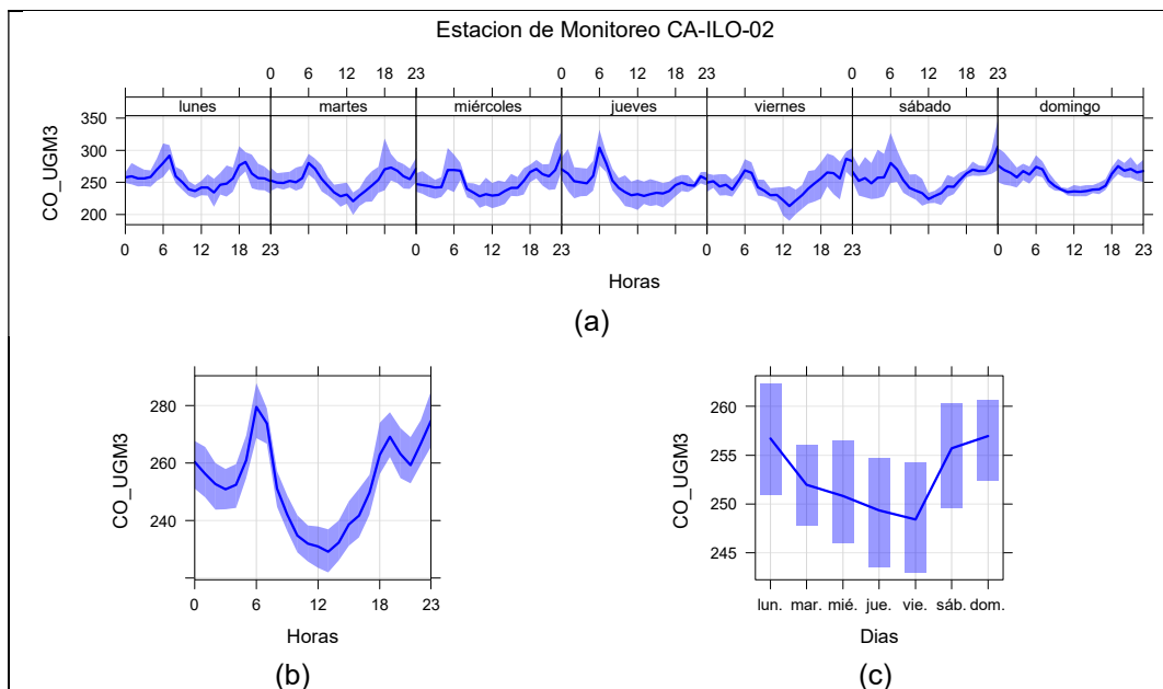
Figura 3.9.15. Concentraciones promedio horarios de CO en la estación de monitoreo CA-ILO-02, de enero de 2023
