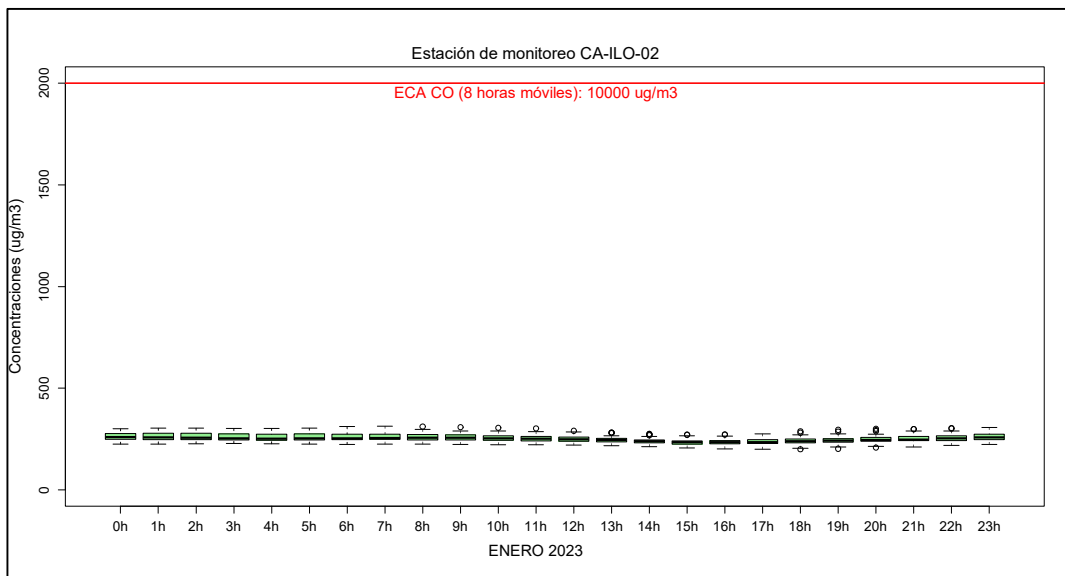
Figura 3.7.5. Concentraciones de promedio móvil de 8 horas de CO en la estación de monitoreo CA-ILO-02, enero de 2023
