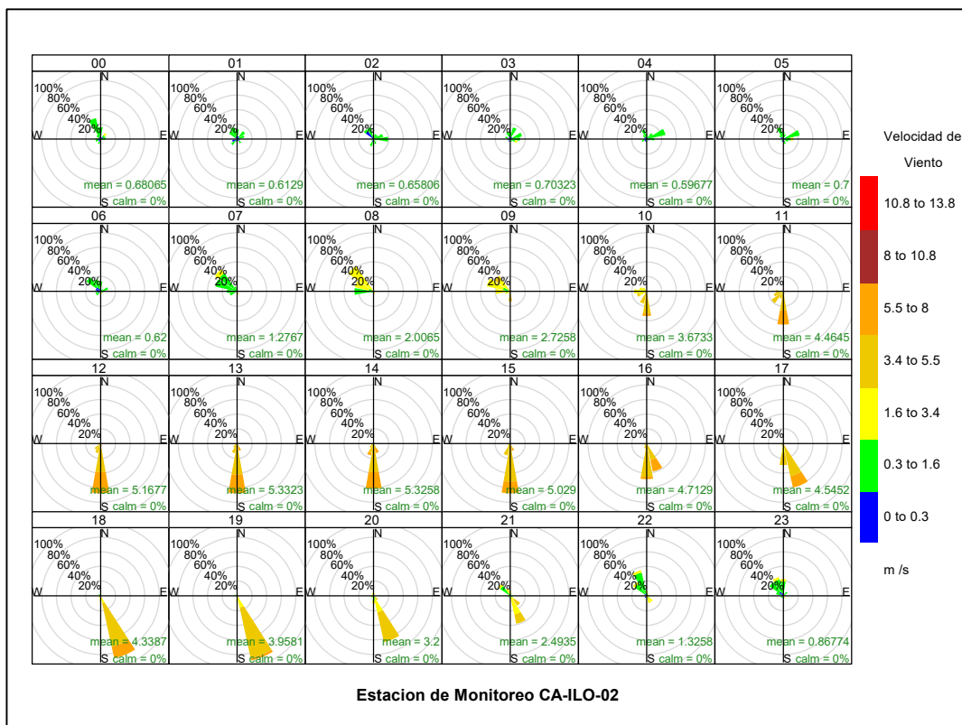
Figura 3.1.6. Rosa de viento horaria de la estación de monitoreo CA-ILO-02, enero de 2023
