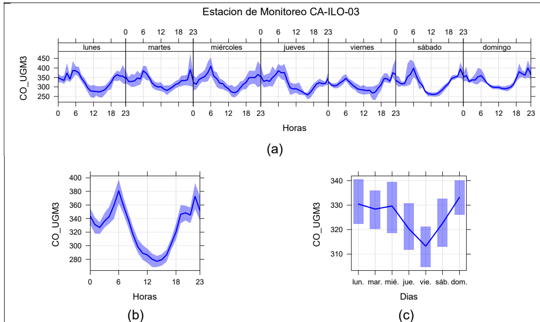
Figura 3.9.16. Concentraciones promedio horarios de CO en la estación de monitoreo CA-ILO-03, de enero de 2023
