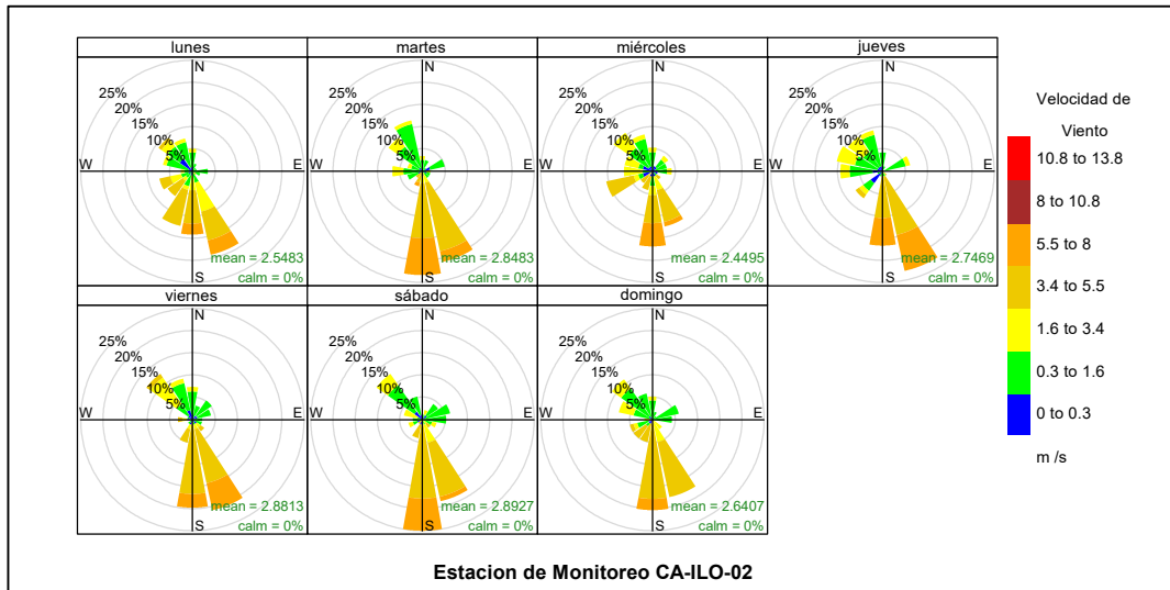
Figura 3.1.5. Rosa de viento por días de la semana de la estación de monitoreo CA-ILO-02, enero de 2023
