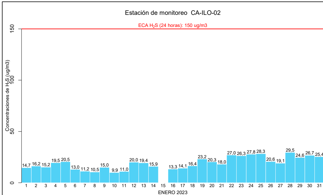
Figura 3.5.2. Concentraciones de 24 horas de H 2 S en la estación de monitoreo CA-ILO-02, enero de 2023
