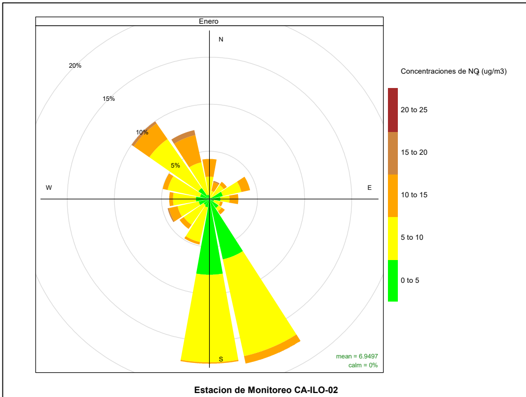
Figura 3.8.22. Rosa de concentración del NO 2 en la estación de monitoreo CA-ILO-02, enero de 2023
