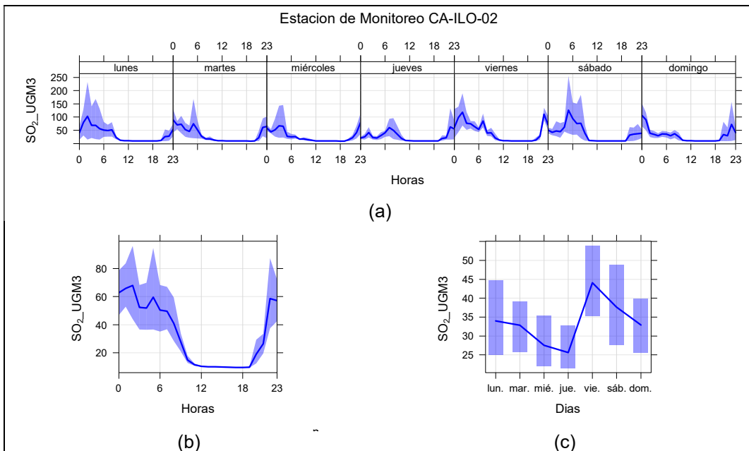
Figura 3.9.6. Concentraciones promedio horarios de SO 2 en la estación de monitoreo CA-ILO-02, de enero de 2023
