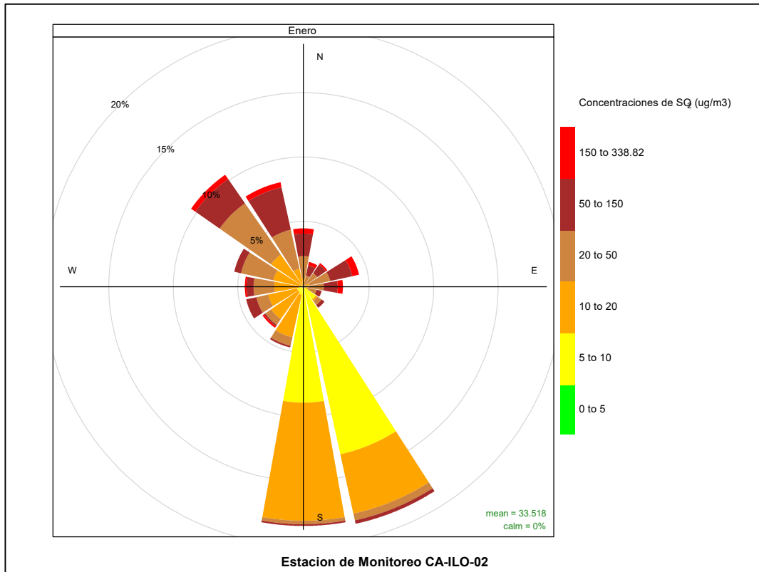
Figura 3.8.10. Rosa de concentración del SO 2 en la estación de monitoreo CA-ILO-02, enero de 2023
