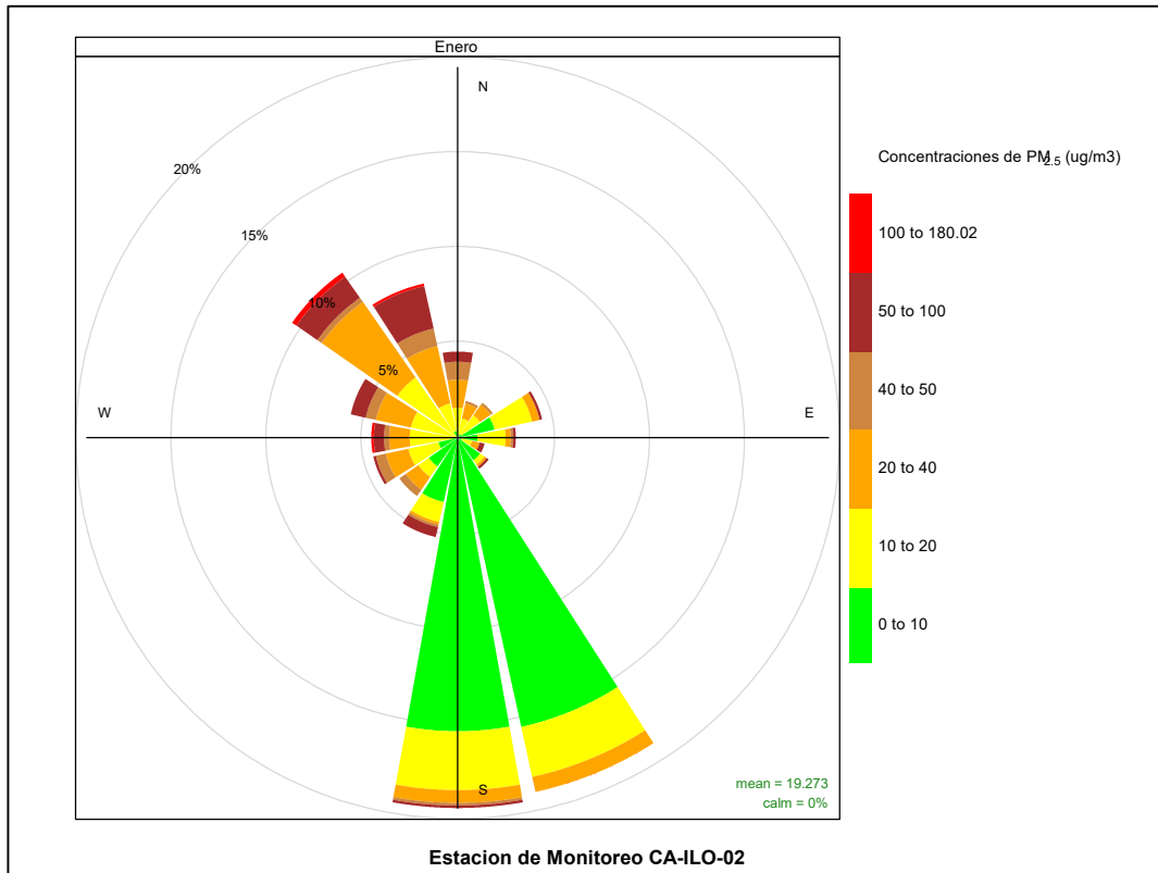
Figura 3.8.1. Rosa de concentración del PM 2.5 en la estación de monitoreo CA-ILO-02, enero del 2023
