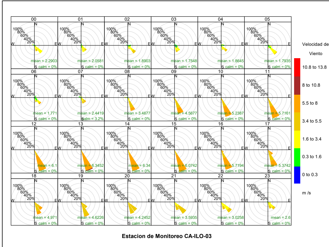
Figura 3.1.9. Rosa de viento horaria de la estación de monitoreo CA-ILO-03, enero de 2023
