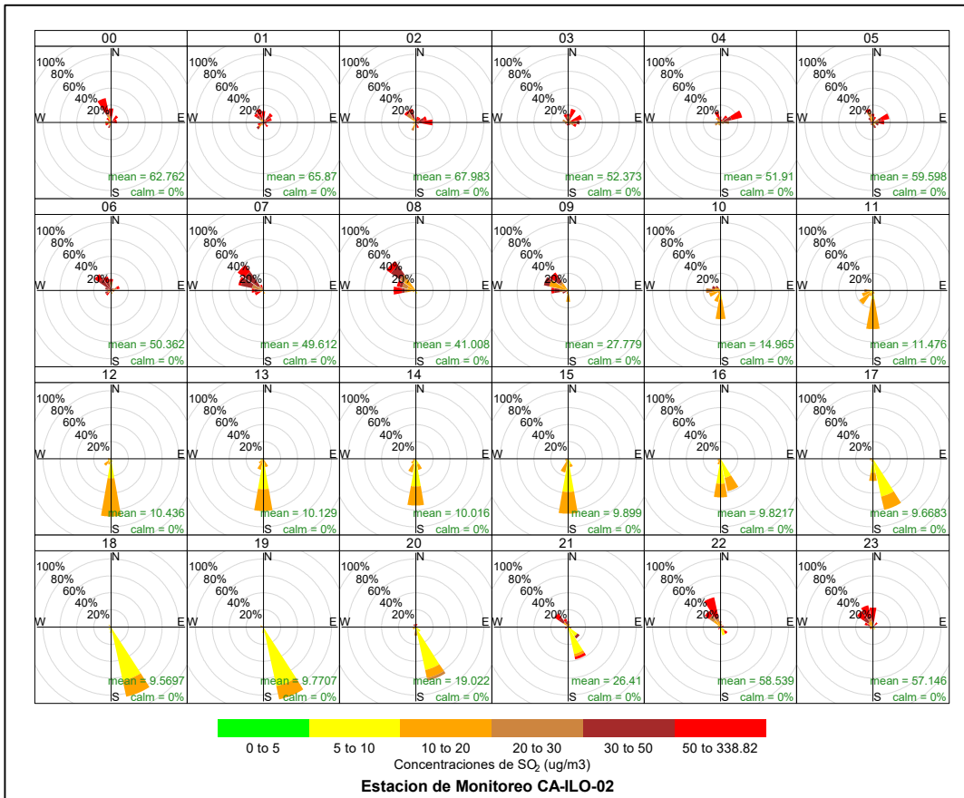
Figura 3.8.13. Rosa de concentración horaria del SO 2 en la estación de monitoreo CA-ILO-02, enero de 2023
