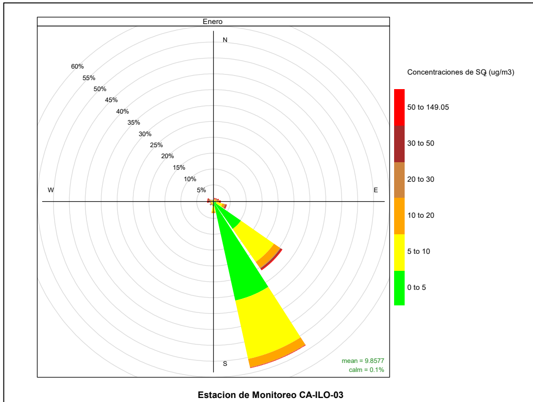
Figura 3.8.11. Rosa de concentración del SO 2 en la estación de monitoreo CA-ILO-03, enero de 2023
