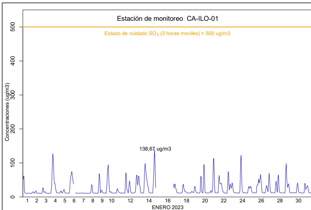
Figura 3.10.1. Concentraciones de promedio móvil de 3 horas de \text{SO}_2 en la estación de monitoreo CA-ILO-01, en enero de 2023
