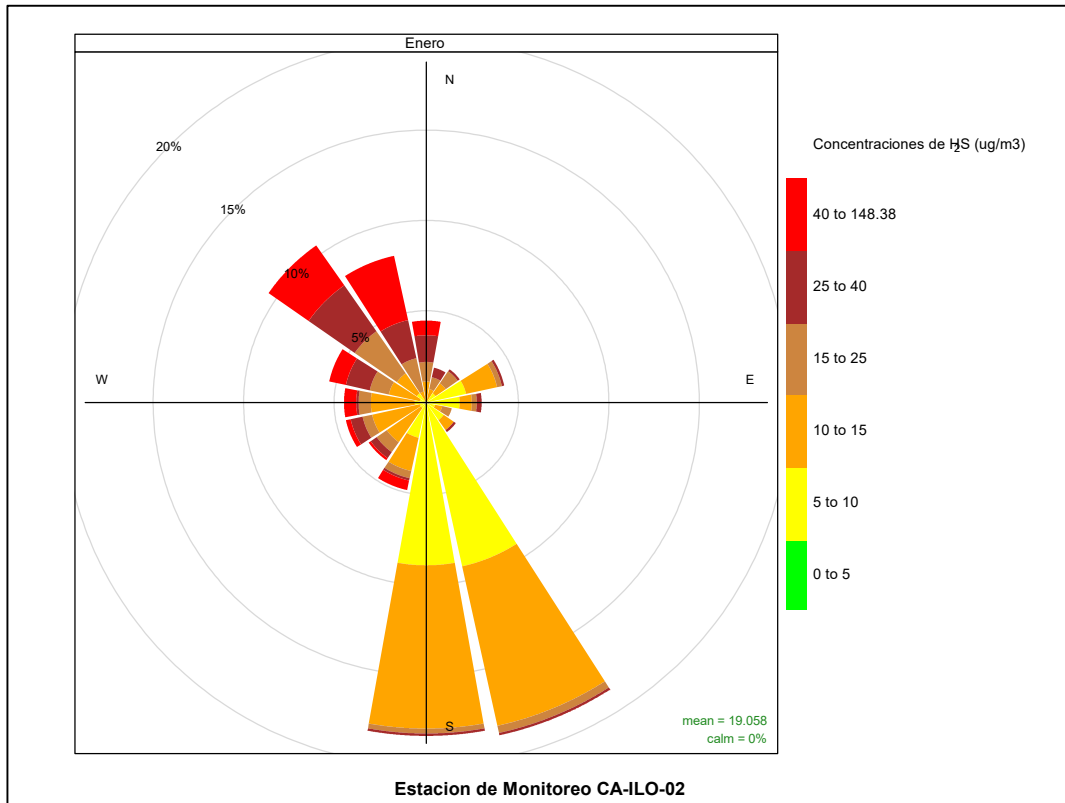
Figura 3.8.16. Rosa de concentración del H 2 S en la estación de monitoreo CA-ILO-02, enero de 2023
