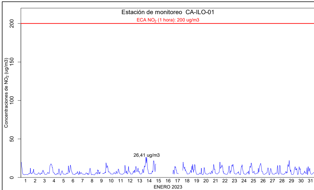
Figura 3.6.1. Concentraciones de horarias de NO 2 en la estación de monitoreo CA-ILO-01, enero de 2023.
