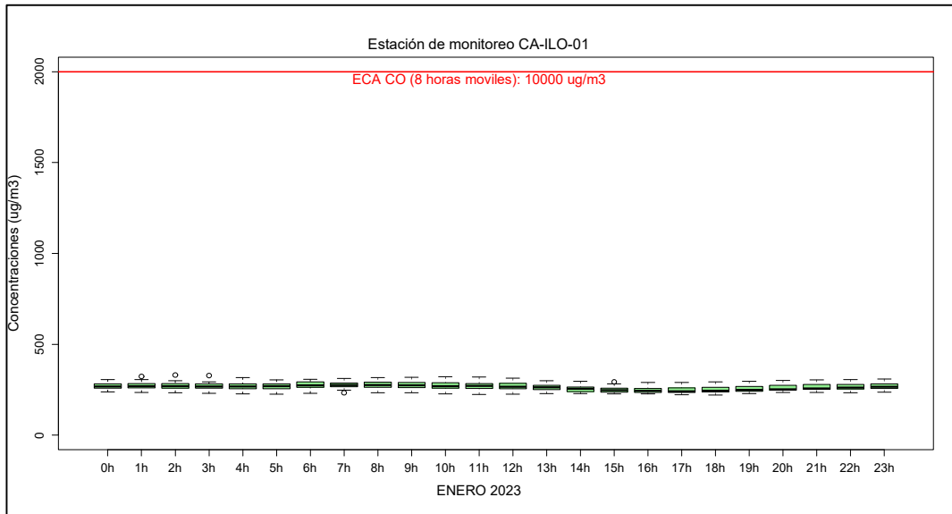
Figura 3.7.4. Concentraciones de promedio móvil de 8 horas de CO en la estación de monitoreo CA-ILO-01, enero de 2023
