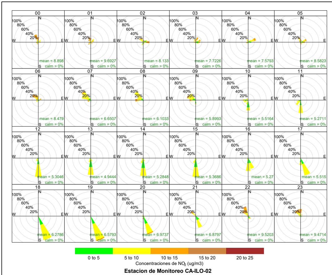
Figura 3.8.25. Rosa de concentración horaria del NO 2 en la estación de monitoreo CA-ILO-02, enero de 2023
