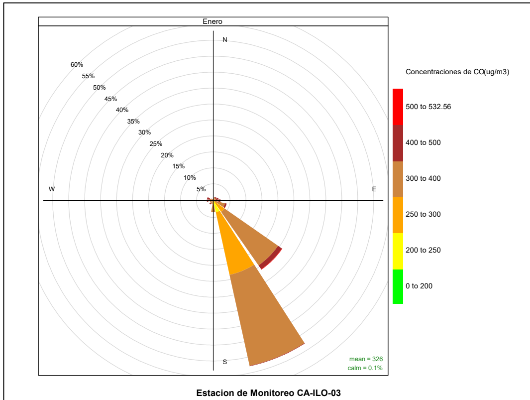
Figura 3.8.29. Rosa de concentración del CO en la estación de monitoreo CA-ILO-03, enero de 2023
