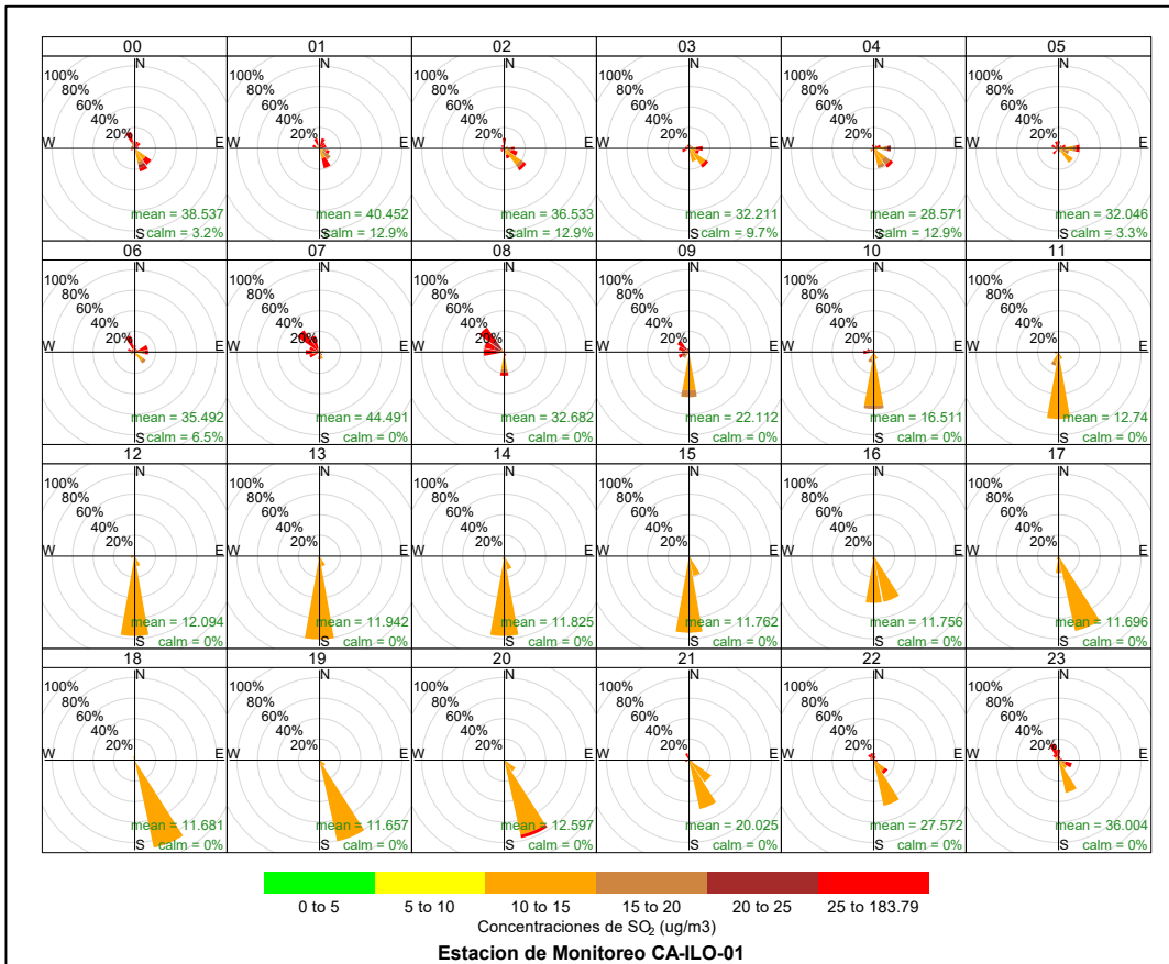
Figura 3.8.12. Rosa de concentración horaria del SO 2 en la estación de monitoreo CA-ILO-01, enero de 2023
