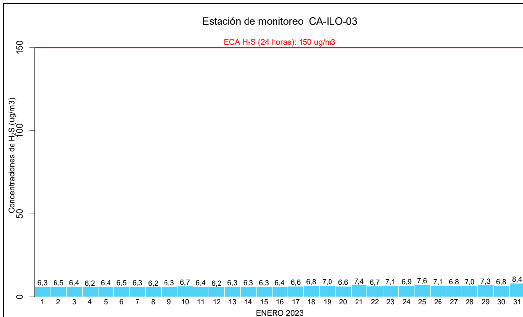
Figura 3.5.3. Concentraciones de 24 horas de H 2 S en la estación de monitoreo CA-ILO-03, enero de 2023.
