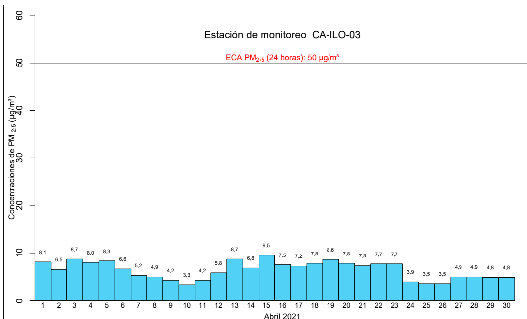
Figura 4.6. Concentraciones de 24 horas de PM 2.5 en la estación de monitoreo CA-ILO-03, en Abril de 2021
