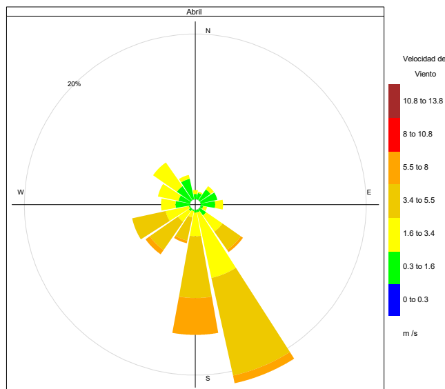
Figura 4.2. Rosa de viento de la estación de monitoreo CA-ILO-02, en Abril de 2021
