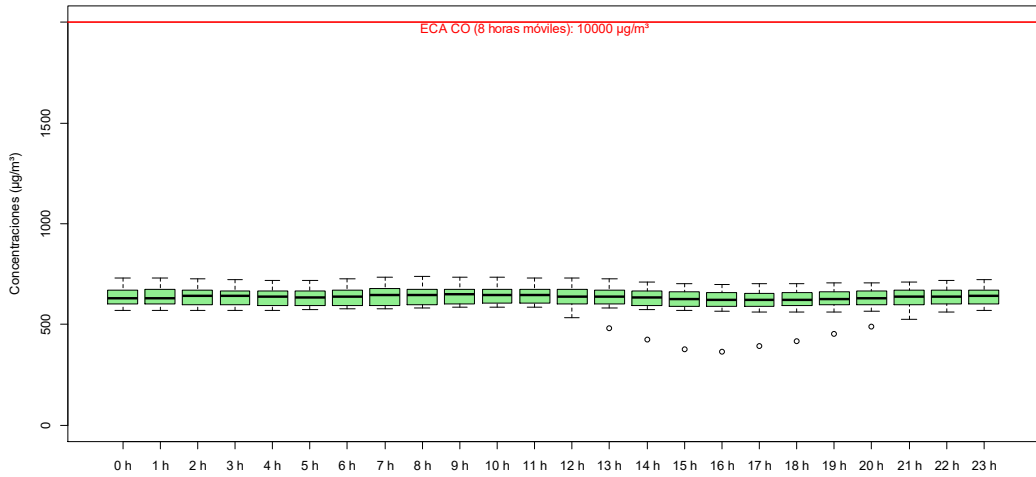
Figura 4.22. Concentraciones de promedio móvil de 8 horas de CO en la estación de monitoreo CA-ILO-01, en Abril de 2021
