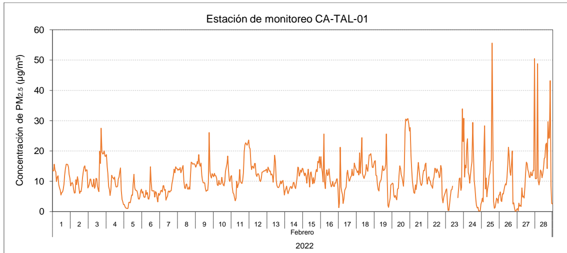
Figura 3.5. Concentraciones horarias de PM 2,5 en la estación de monitoreo Tala (CA-TAL-01) de febrero de 2022
