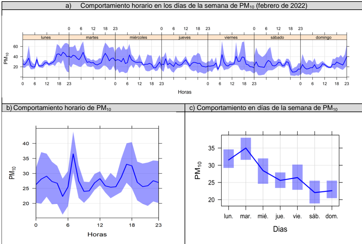
Figura 3.3. Concentraciones promedio horarios, diarios y semanales de PM 10 en la estación de monitoreo Tala (CA-TAL-01), de febrero de 2022
