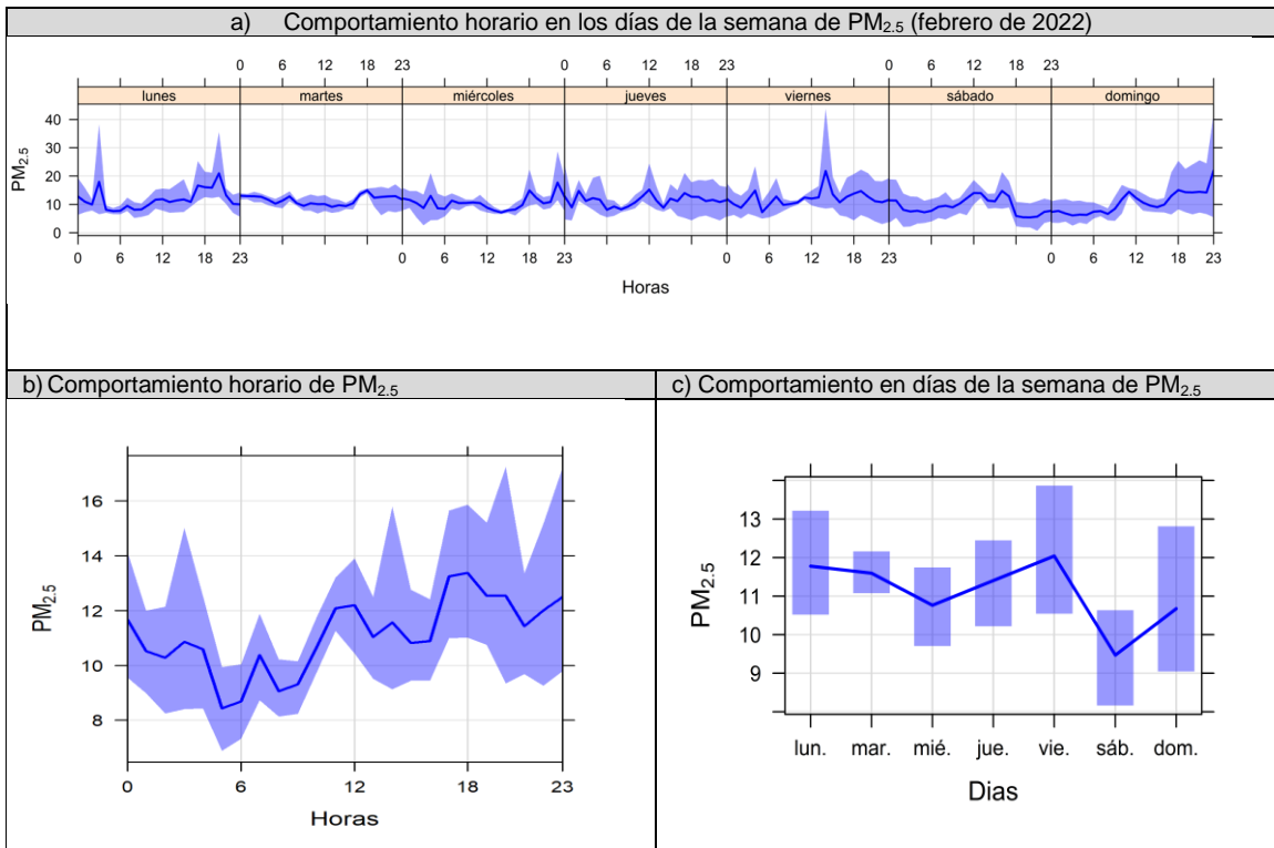
Figura 3.6. Concentraciones promedio horarias, diarias y semanales de PM 2.5 en la estación de monitoreo Tala (CA-TAL-01) de febrero de 2022.
