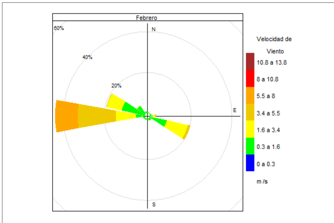
Figura 3.1. Rosa de vientos de la estación de monitoreo Tala (CA-TAL-01), febrero de 2022
