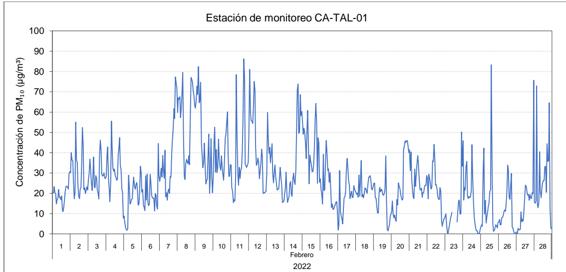
Figura 3.2. Concentración horaria de PM 10 en la estación de monitoreo Tala (CA-TAL-01), de febrero de 2022
