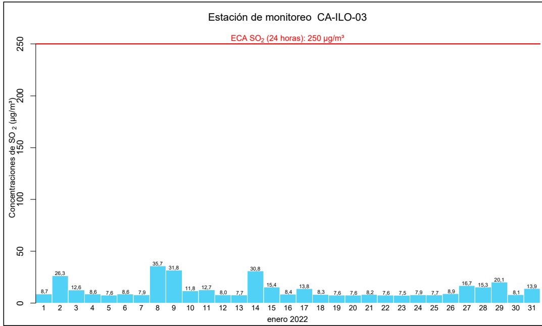
Figura 4.10. Concentraciones de 24 horas de SO 2 en la estación de monitoreo CA-ILO-03, en enero de 2022
