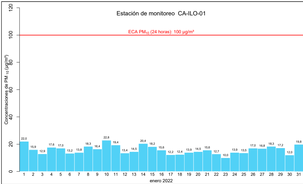
Figura 4.6. Concentraciones de 24 horas de PM 10 en la estación de monitoreo CA-ILO-01, en enero de 2022
