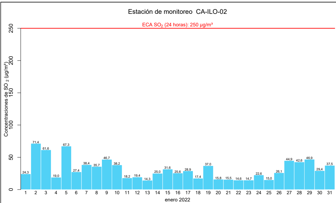
Figura 4.9. Concentraciones de 24 horas de SO 2 en la estación de monitoreo CA-ILO-02, en enero de 2022
