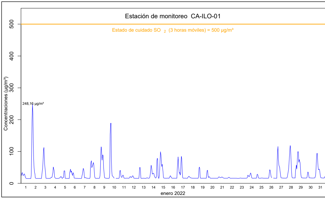
Figura 4.23. Concentraciones de promedio móvil de 3 horas de SO 2 en la estación de monitoreo CA-ILO-01, en enero de 2022
