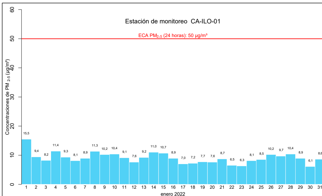
Figura 4.4. Concentraciones de 24 horas de PM 2,5 en la estación de monitoreo CA-ILO-01, en enero de 2022
