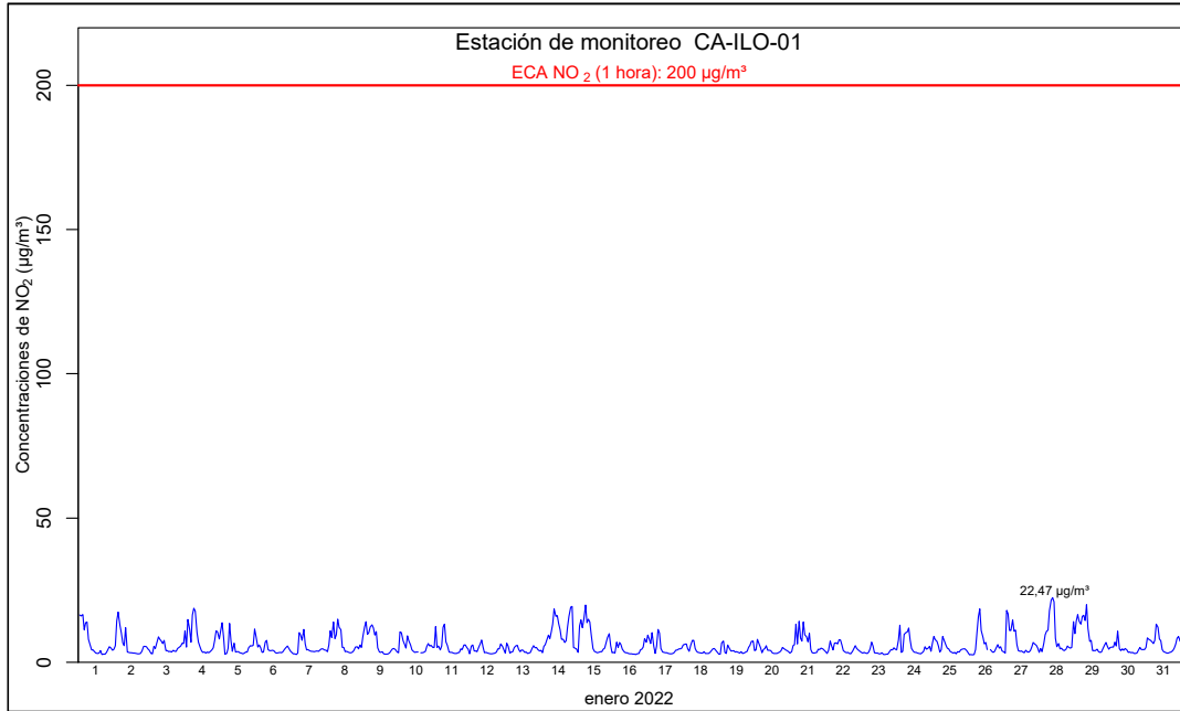
Figura 4.14. Concentraciones de horarias de NO 2 en la estación de monitoreo CA-ILO-01, en enero de 2022
