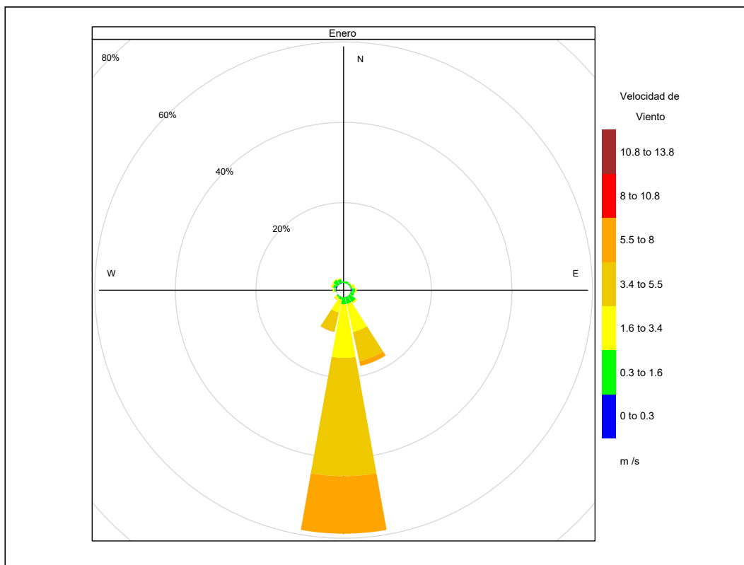
Figura 4.3. Rosa de viento de la estación de monitoreo CA-ILO-03, en enero de 2022
