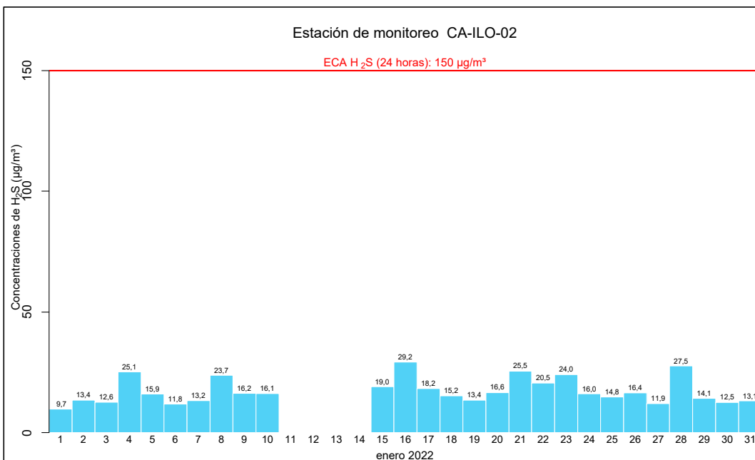
Figura 4.12. Concentraciones de 24 horas de H 2 S en la estación de monitoreo CA-ILO-02, en enero de 2022 1
