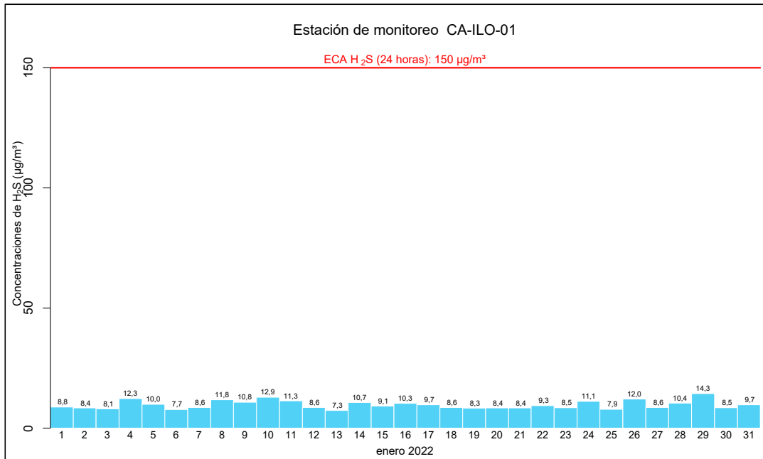
Figura 4.11. Concentraciones de 24 horas de H 2 S en la estación de monitoreo CA-ILO-01, en enero de 2022
