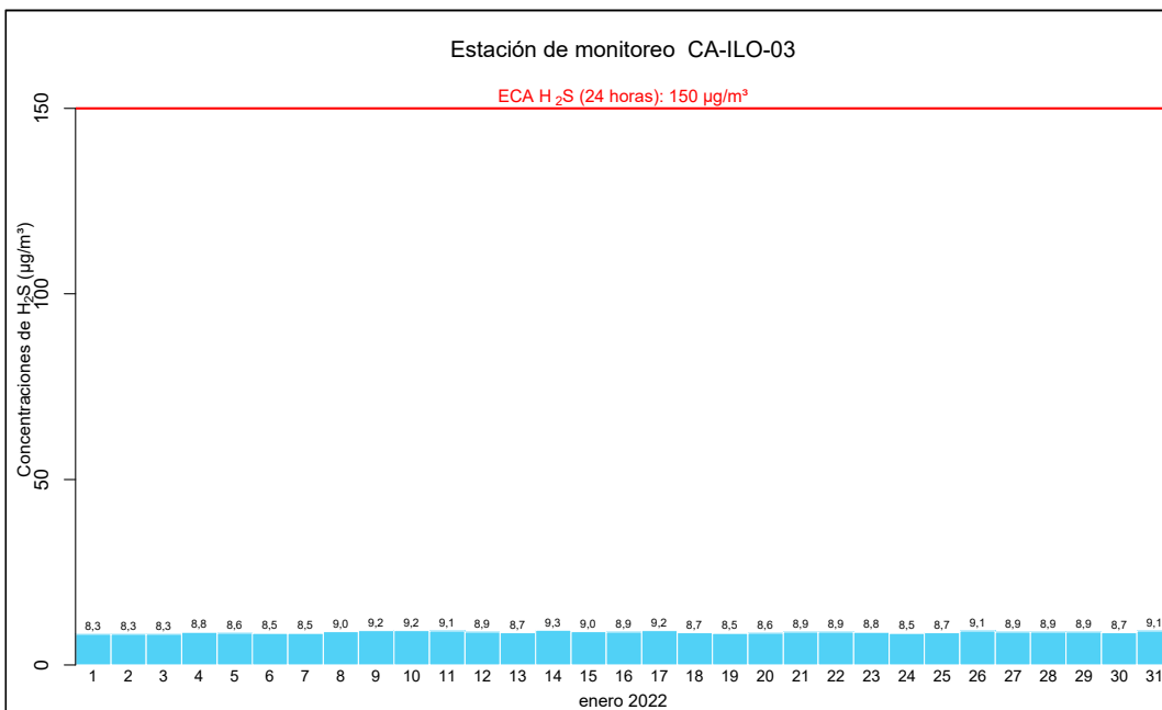
Figura 4.13. Concentraciones de 24 horas de H 2 S en la estación de monitoreo CA-ILO-03, en enero de 2022
