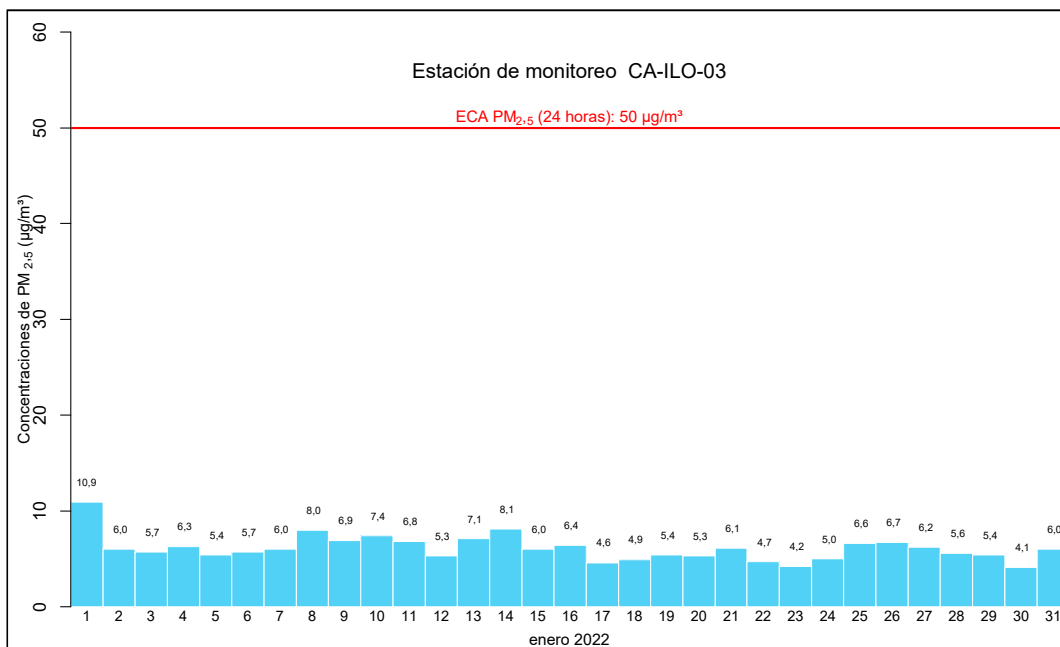
Figura 4.5. Concentraciones de 24 horas de PM 2,5 en la estación de monitoreo CA-ILO-03, en enero de 2022
