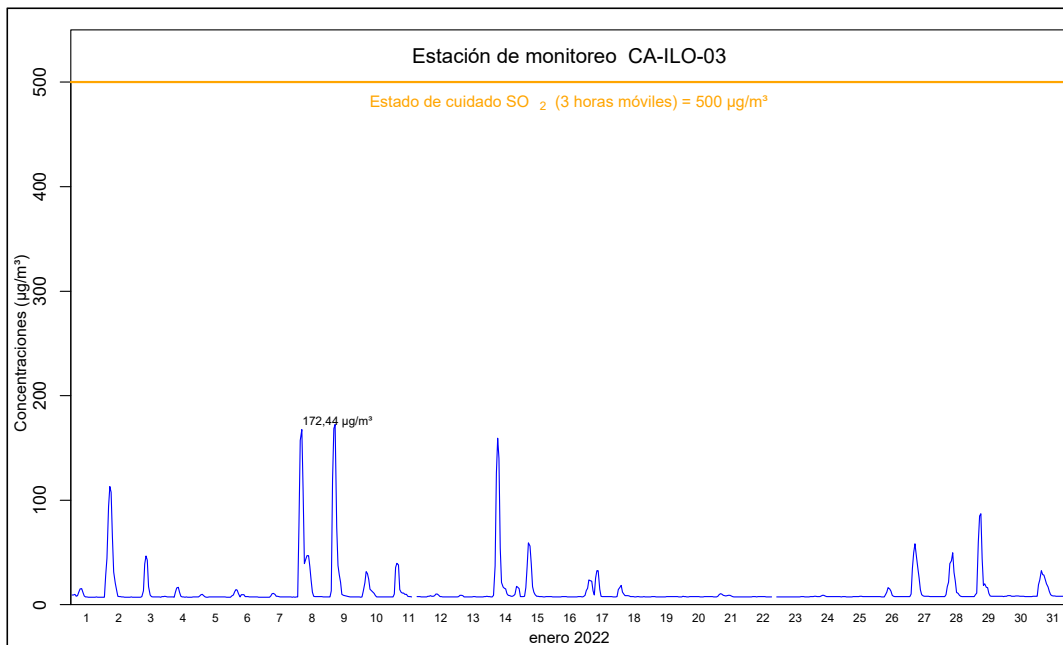
Figura 4.25. Concentraciones de promedio móvil de 3 horas de SO 2 en la estación de monitoreo CA-ILO-03, en enero de 2022
