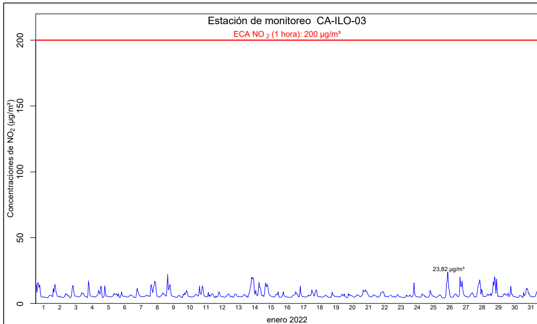
Figura 4.16. Concentraciones de horarias de NO 2 en la estación de monitoreo CA-ILO-03, en enero de 2022
