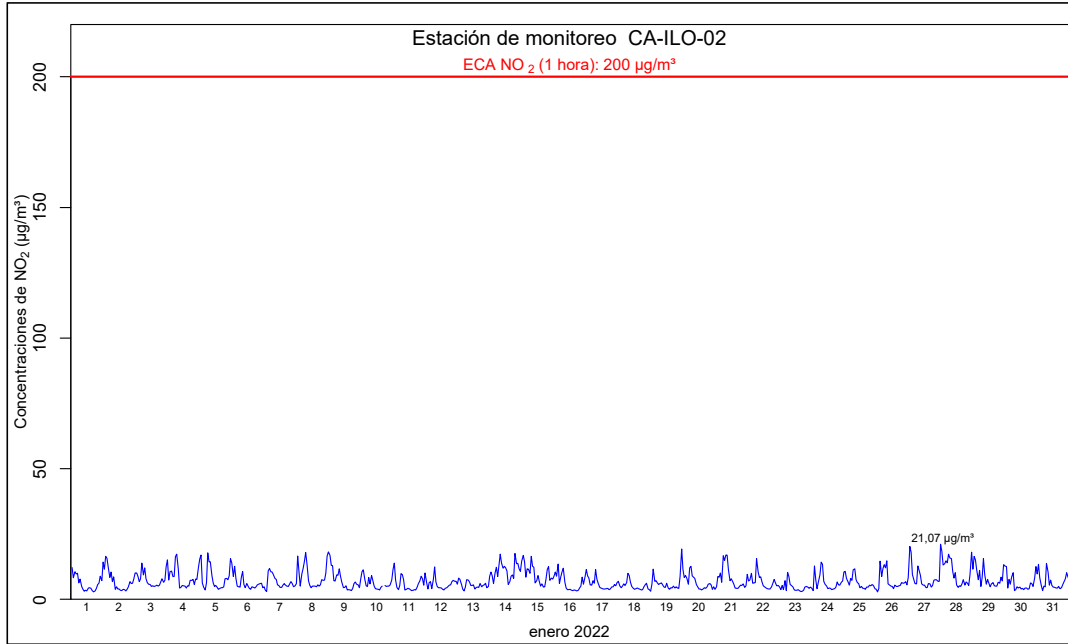
Figura 4.15. Concentraciones de horarias de NO 2 en la estación de monitoreo CA-ILO-02, en enero de 2022
