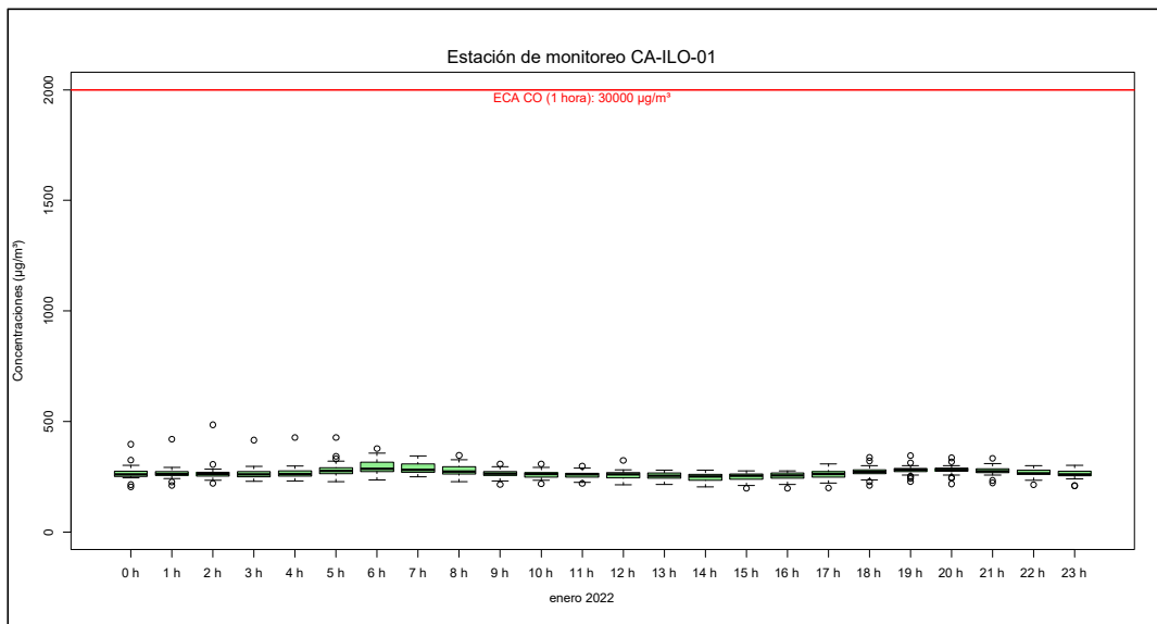
Figura 4.17. Concentraciones de horarias de CO en la estación de monitoreo CA-ILO-01, en enero de 2022
