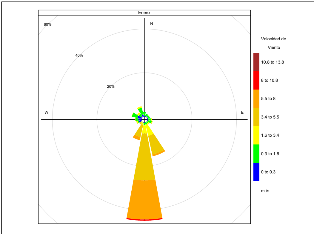
Figura 4.1. Rosa de viento de la estación de monitoreo CA-ILO-01, en enero de 2022
