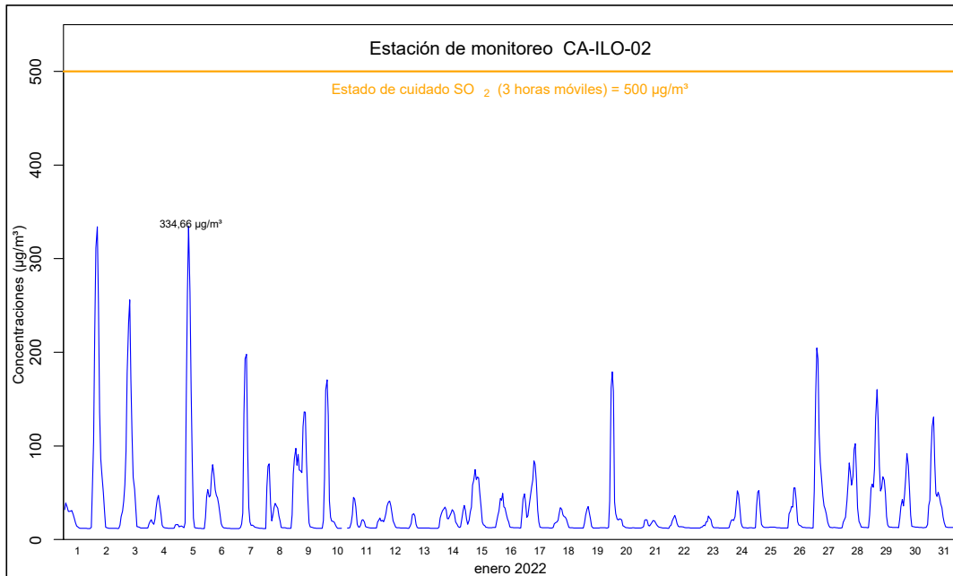
Figura 4.24. Concentraciones de promedio móvil de 3 horas de SO 2 en la estación de monitoreo CA-ILO-02, en enero de 2022
