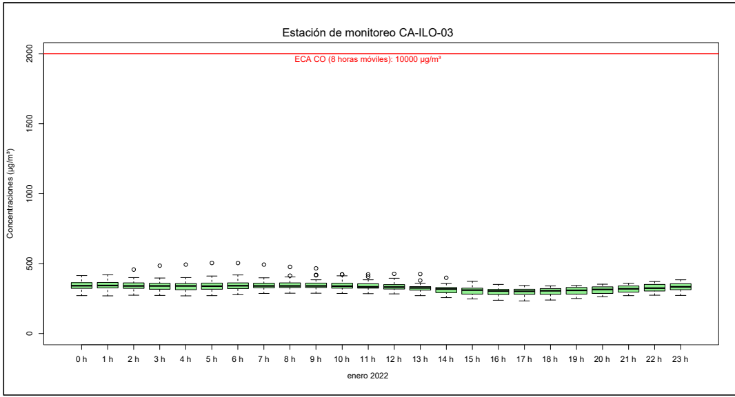
Figura 4.22. Concentraciones de promedio móvil de 8 horas de CO en la estación de monitoreo CA-ILO-03, en enero de 2022
