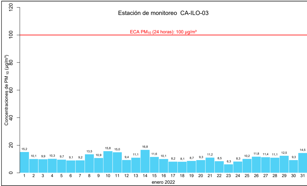
Figura 4.7. Concentraciones de 24 horas de PM 10 en la estación de monitoreo CA-ILO-03, en enero de 2022
