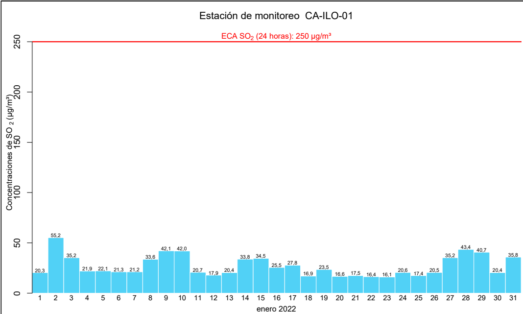
Figura 4.8. Concentraciones de 24 horas de SO 2 en la estación de monitoreo CA-ILO-01, en enero de 2022
