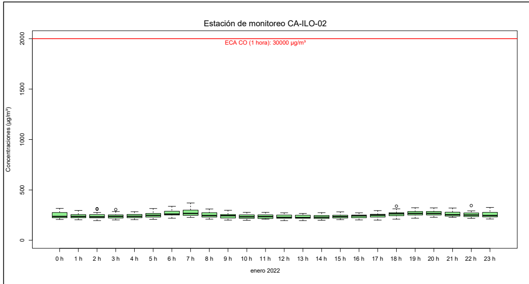
Figura 4.18. Concentraciones de horarias de CO en la estación de monitoreo CA-ILO-02, en enero de 2022
