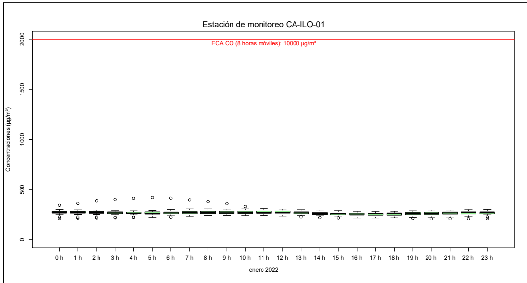
Figura 4.20. Concentraciones de promedio móvil de 8 horas de CO en la estación de monitoreo CA-ILO-01, en enero de 2022
