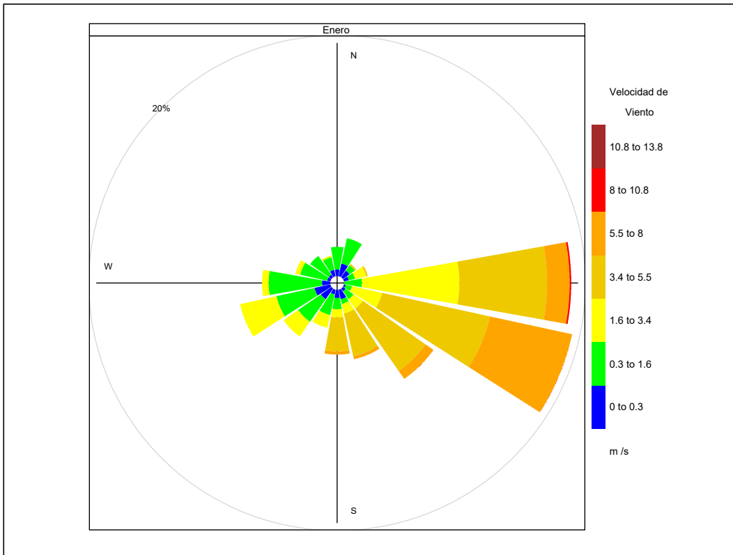
Figura 4.2. Rosa de viento de la estación de monitoreo CA-ILO-02, en enero de 2022
