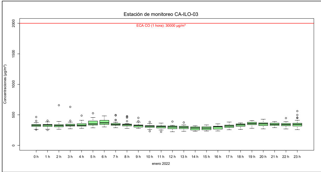
Figura 4.19. Concentraciones de horarias de CO en la estación de monitoreo CA-ILO-03, en enero de 2022
