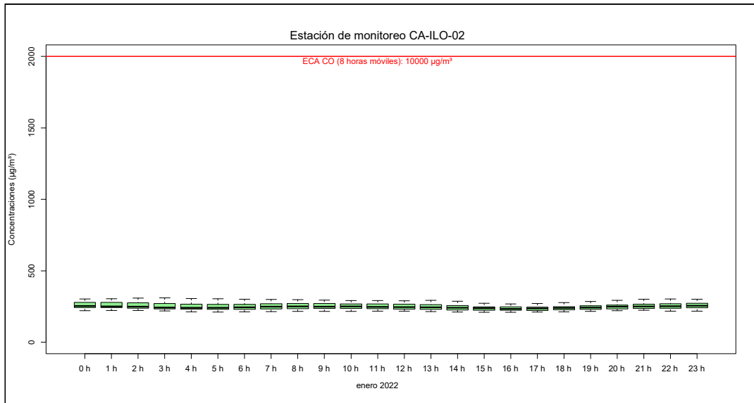
Figura 4.21. Concentraciones de promedio móvil de 8 horas de CO en la estación de monitoreo CA-ILO-02, en enero de 2022
