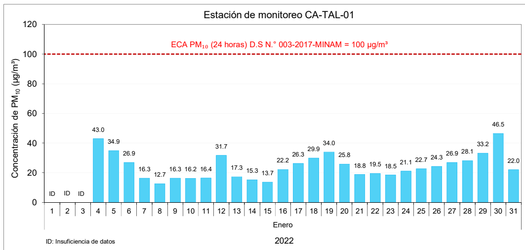
Figura 3.4. Concentraciones de 24 horas de PM 10 en la estación de monitoreo Tala (CA-TAL-01), de enero 2022 ID: Insuficiencia de datos
