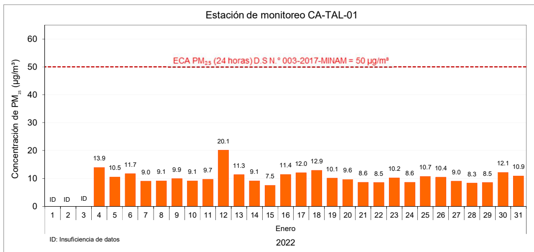
Figura 3.7. Concentraciones de 24 horas de PM_{2.5} en la estación de monitoreo Tala (CA-TAL-01), de enero de 2022 ID: Insuficiencia de datos
