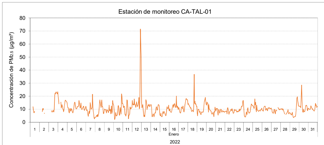
Figura 3.5. Concentraciones horarias de PM 2.5 en la estación de monitoreo Tala (CA-TAL-01) de enero de 2022
