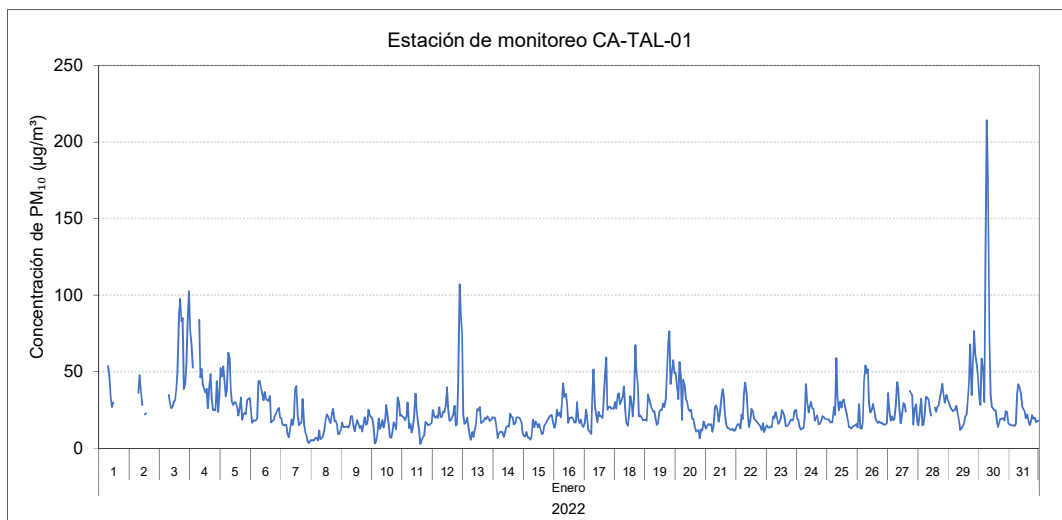
Figura 3.2. Concentración horaria de PM 10 en la estación de monitoreo Tala (CA-TAL-01), de enero de 2022
