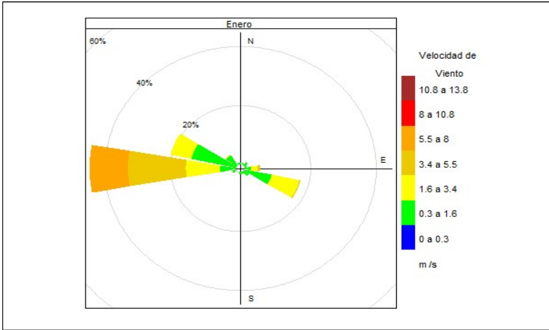
Figura 3.1. Rosa de vientos de la estación de monitoreo Tala (CA-TAL-01), enero de 2022
