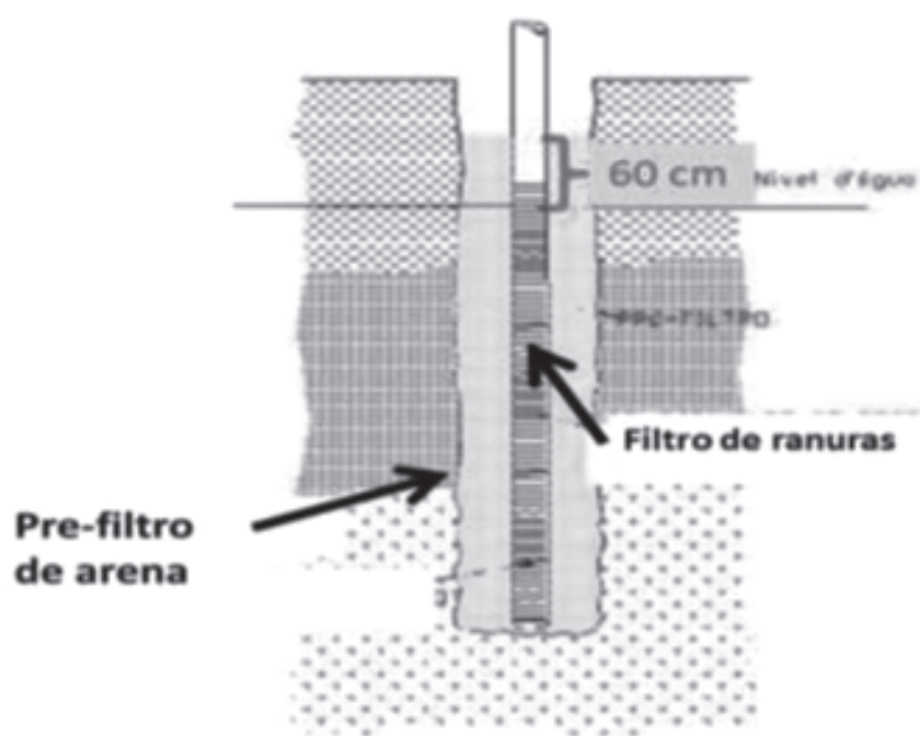
Imagen N° 2: Posición del pre-filtro de arena en relación al filtro de ranuras
